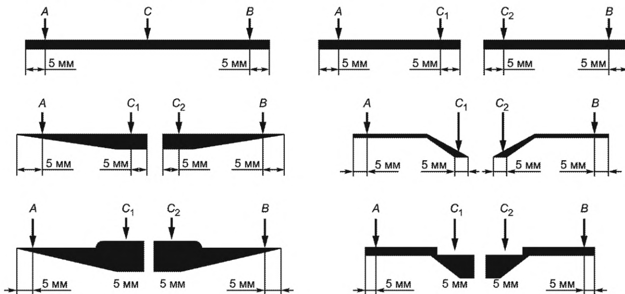
А и В — места измерения толщины с двух сторон по периферии; С, С 1 и С 2 — места измерения толщины в центре
