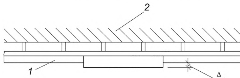
Рисунок Б.12 — Провисание полотна потолка
