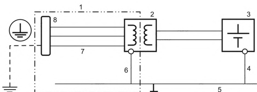
Рисунок 4 — Соединение между защитным проводником и электрическим шасси (пример для варианта 1)
