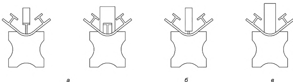
а — гибка по ребру; б — гибка по выступу; в — гибка по полотну
