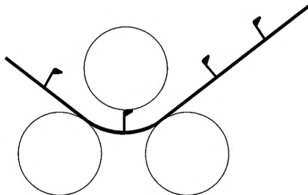
Рисунок 11 — Схема гибки слома панели по ребру жесткости в вальцах
