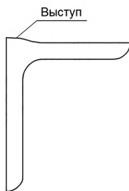
Рисунок 14 — Выступ на внешнем угле профиля
