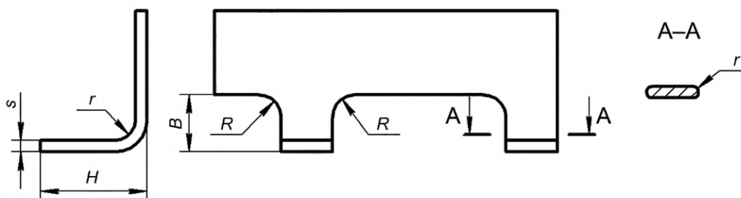
Рисунок 3 — Отбортовка выступающих участков
