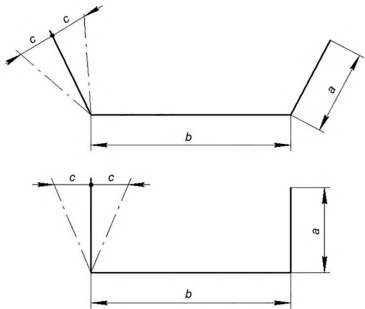
Рисунок 13 — Схема измерений отклонений угловой детали
