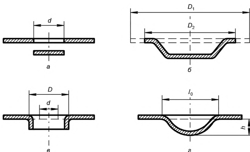
а — вырубка (пробивка); б — вытяжка; в — отбортовка; г — формообразование рифтов
