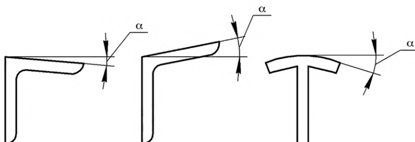
Рисунок 16 — Малка при высадке и малковке
