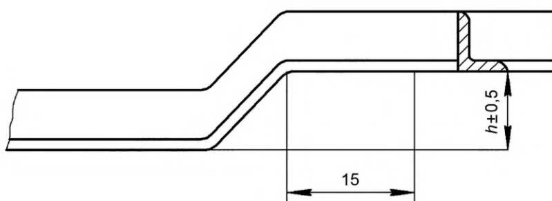
Рисунок 15 — Отклонение от параллельности высадки
