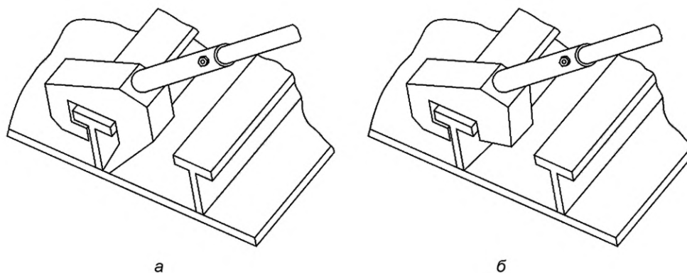
а — правка завалов стенок; б — правка завалов полок
