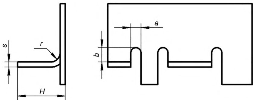
Рисунок 4 — Местная отбортовка
