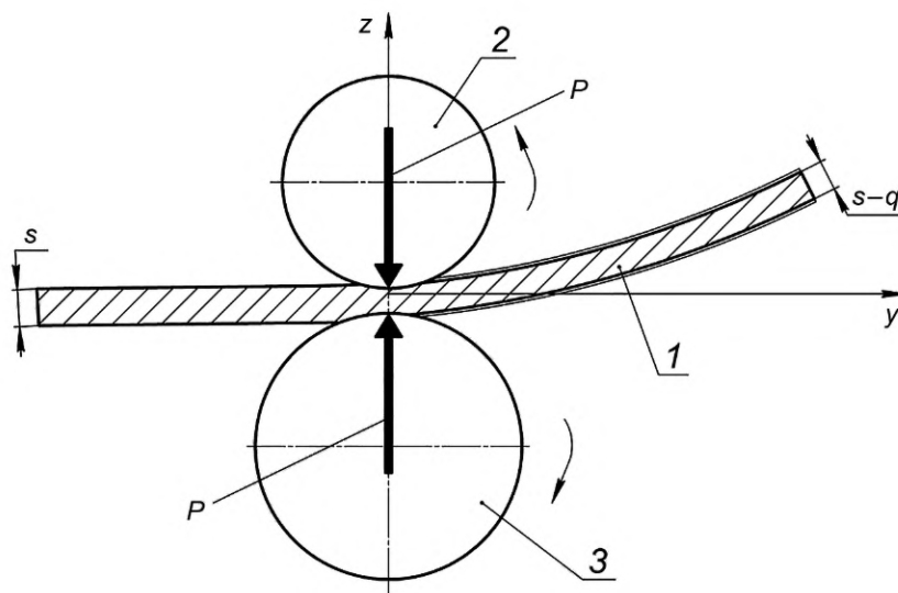
1 — заготовка, 2 — верхний ролик, 3 — нижний ролик, P — усилие гибки, s — толщина заготовки, q — утонение
