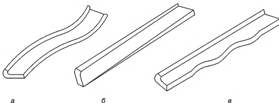
а — ребровая кривизна; б — винтообразное искривление; в — гофры на стенке
