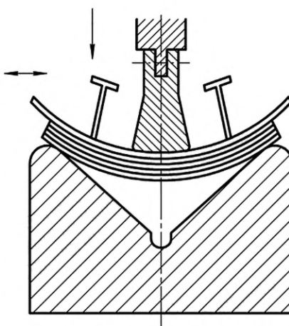
Рисунок 10 — Схема гибки панелей под прессом
