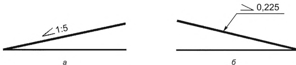
Рисунок 9 — Примеры обозначения уклона
