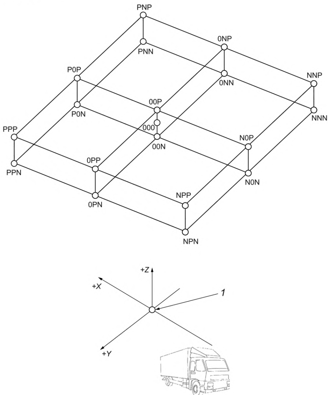
1 — точка выравнивания СЦЭТ Рисунок 6 — Точки выравнивания
