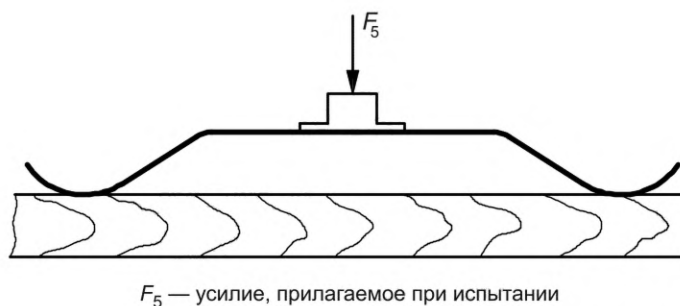
Рисунок Н.3 — Направление приложения испытательной силы F к прижимной защитной накладке для измерения прогиба — Вид сверху
