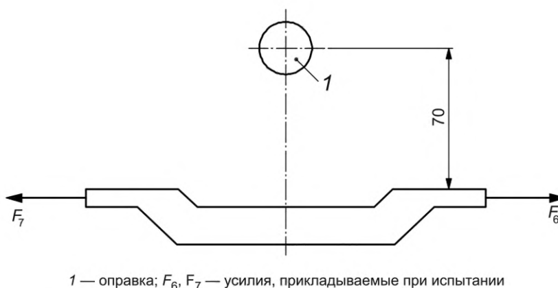
Рисунок Н.5 — Точки измерения прогиба накладки прижима к столу и направления приложения испытательных сил - Вид сверху
