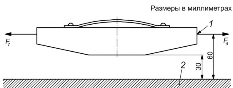
1 — точка приложения измеряемой силы; 2 — стол станка; F_6 , F_7 — усилия, прилагаемые при испытании
