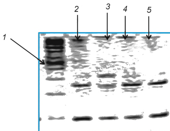
1 — маркер молекулярного веса; 2—5 — образцы
