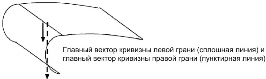
Рисунок 10 — Разрыв G2 вследствие разницы величин вектора кривизны
