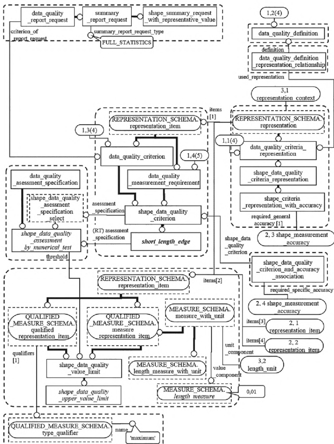
Рисунок F.8 — Примеры экземпляров, образующих информацию о качестве, используемую для обеспечения уверенности в качестве относительно критерия short length edge (1 из 6)
