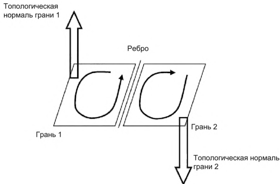
Рисунок 17 — Несогласованные топологические нормали смежных граней
