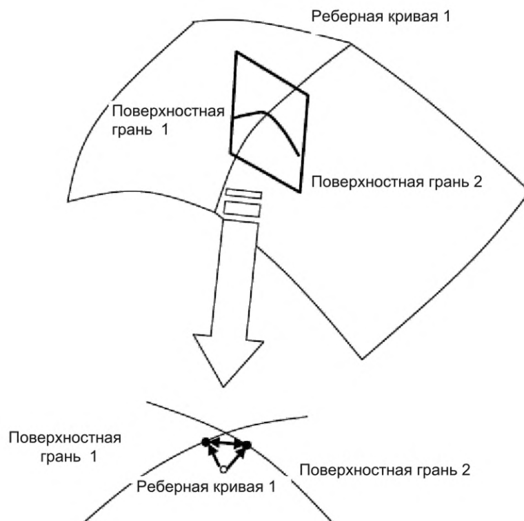
Рисунок 15 — Измерение зазора между гранями, связанными с ребром
