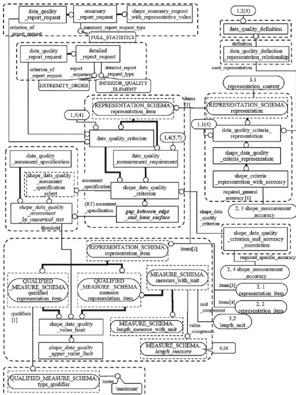
Рисунок F.21 — Примеры экземпляров, образующих информацию о качестве, используемую для улучшения качества относительно критерия gap_between_edge_and_base_surface (1 из 7)
