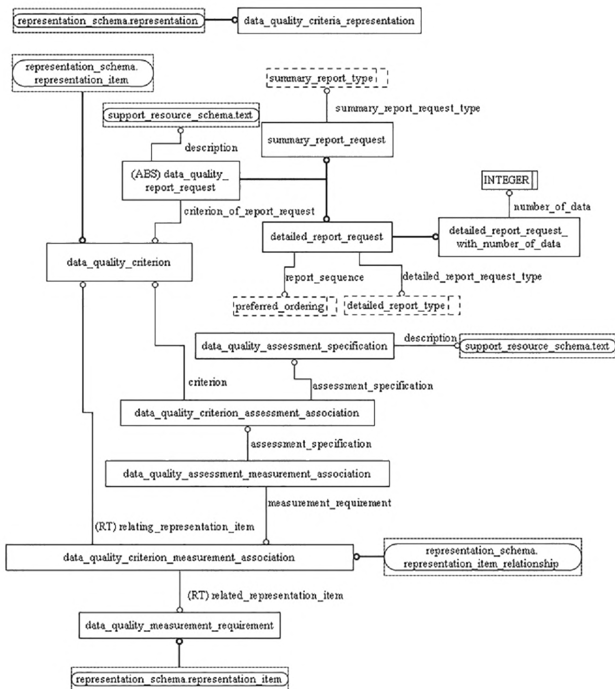
Рисунок D.4 — EXPRESS-G диаграмма схемы product_data_quality_criteria_schema (диаграмма 2 из 2)
