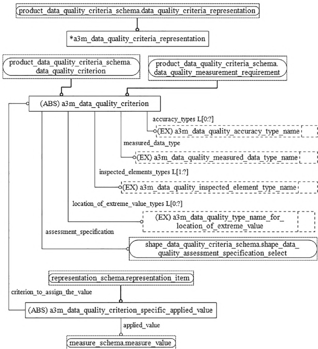
Рисунок D.22 — EXPRESS-G диаграмма схемы annotated_3d_model_data_quality_criteria_schema (диаграмма 2 из 3)
