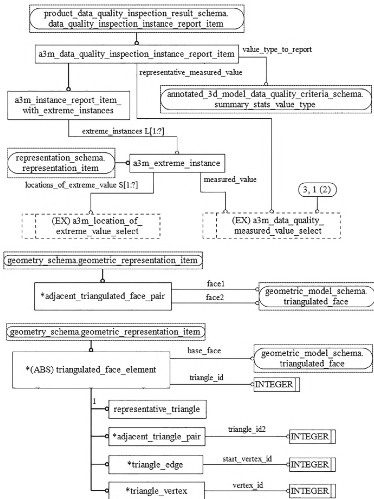
Рисунок D.26 — EXPRESS-G диаграмма схемы annotated_3d_model_data_quality_inspection_result_schema (диаграмма 3 из 3)
