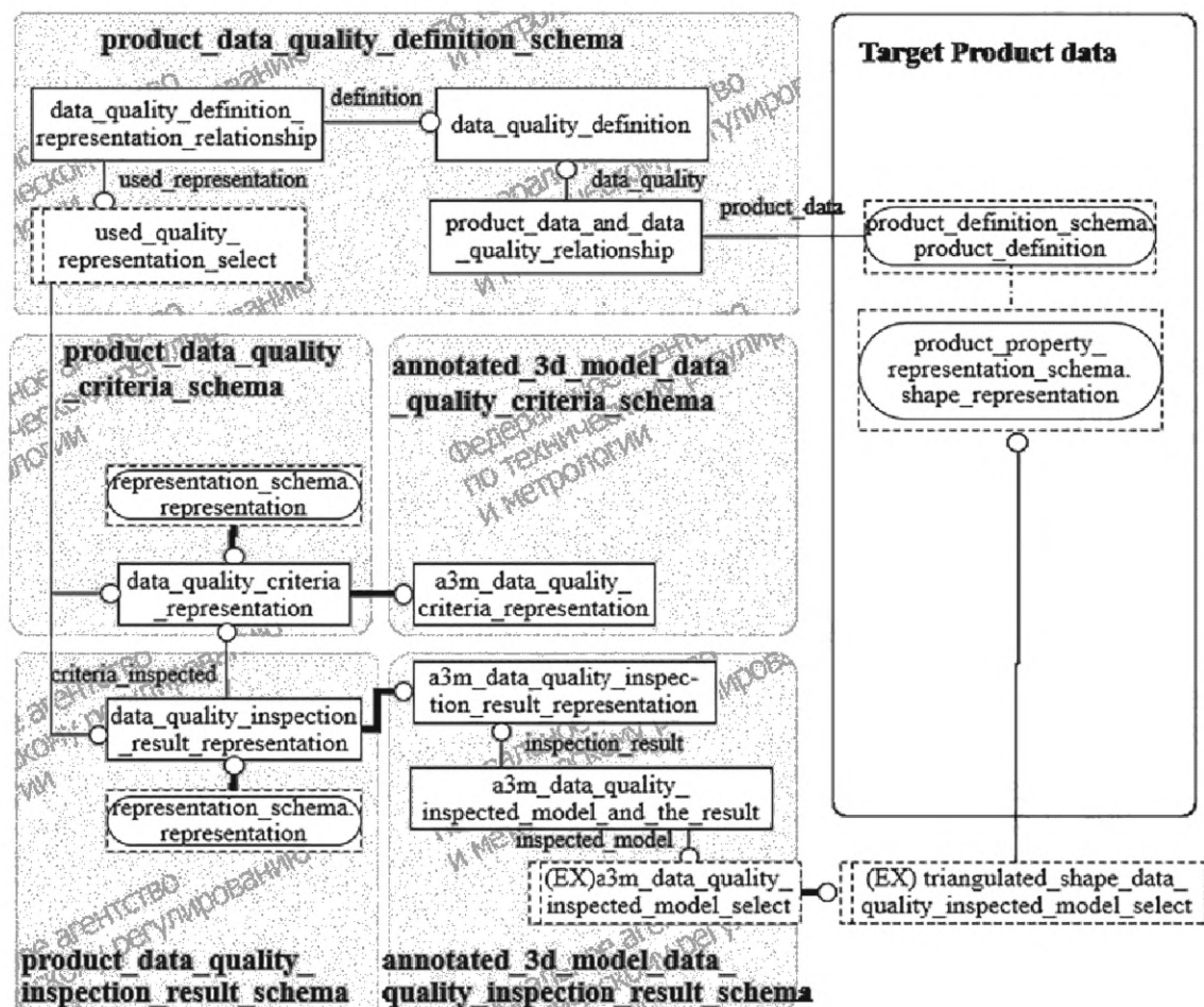
Рисунок Е.2 — Отношения между схемами третьего издания настоящего стандарта и подлежащими обработке данными об изделии
