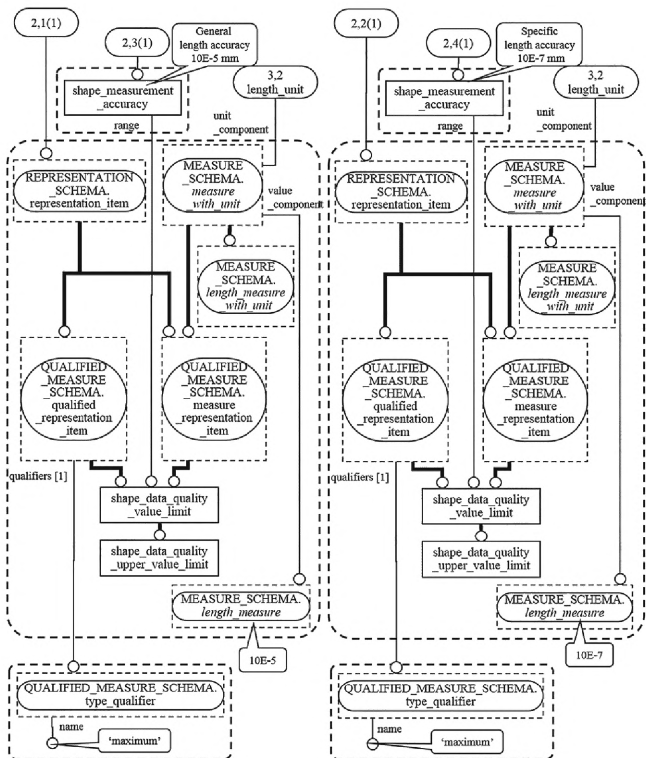
Рисунок F.22 — Примеры экземпляров, образующих информацию о качестве, используемую для улучшения качества относительно критерия gap_between_edge_and_base_surface (2 из 7)
