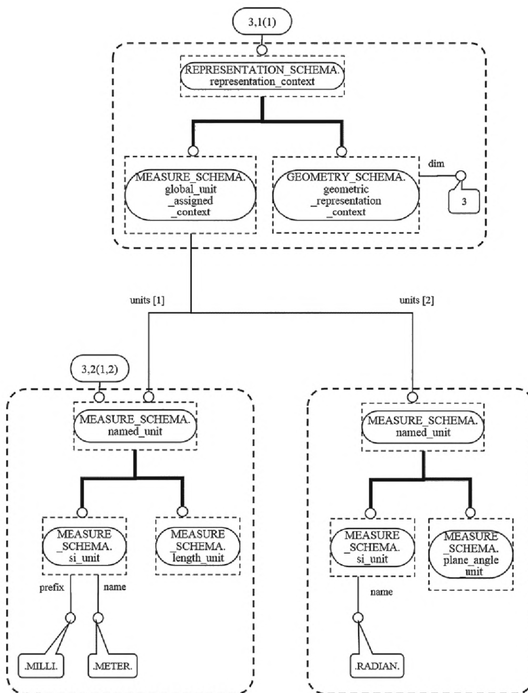
Рисунок F.10 — Примеры экземпляров, образующих информацию о качестве, используемую для обеспечения уверенности в качестве относительно критерия short_length_edge (3 из 6)
