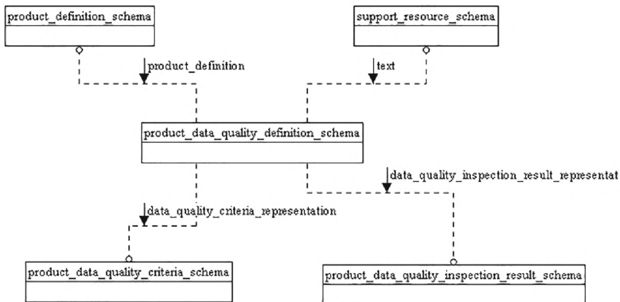
Рисунок D.1 — EXPRESS-G диаграмма схемы product_data_quality_definition_schema (диаграмма 1 из 2)
