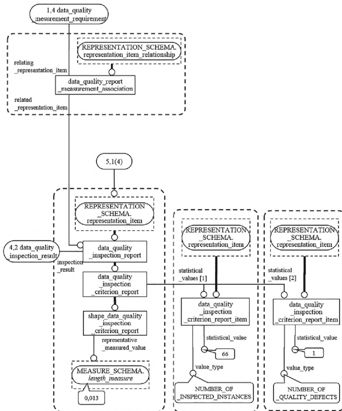
Рисунок F.25 — Примеры экземпляров, образующих информацию о качестве, используемую для улучшения качества относительно критерия gap_between_edge_and_base_surface (5 из 7)
