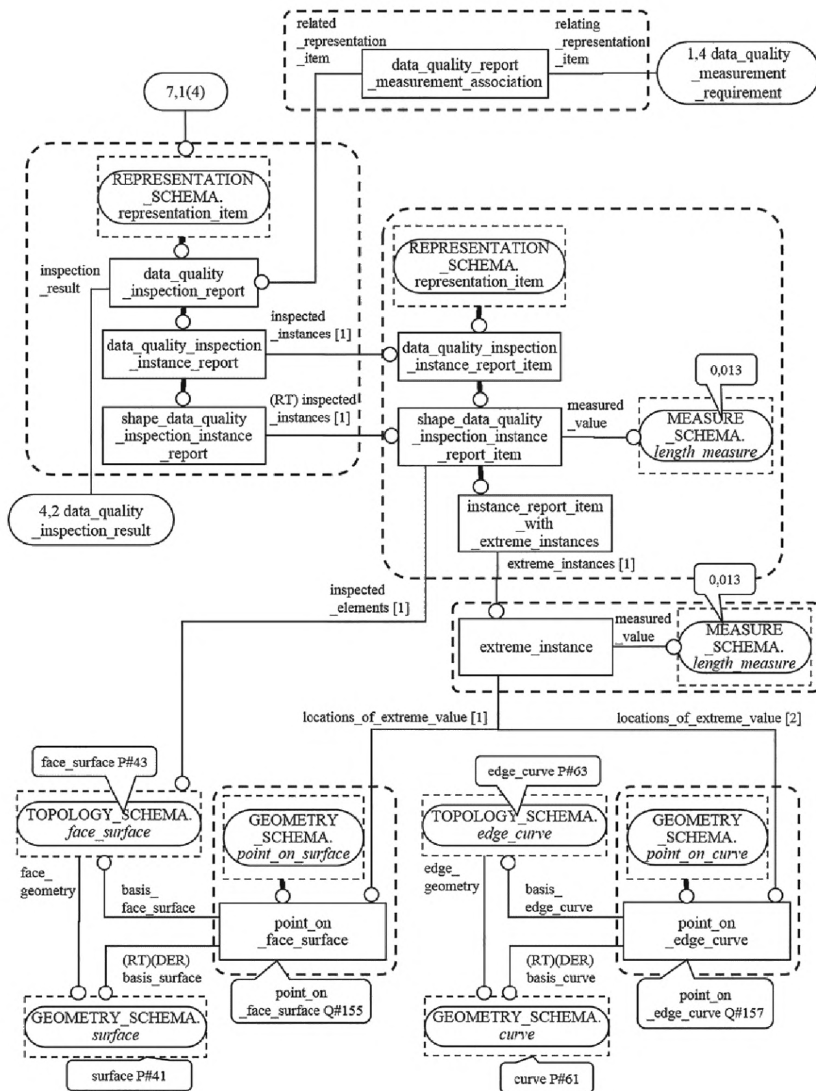
Рисунок F.27 — Примеры экземпляров, образующих информацию о качестве, используемую для улучшения качества относительно критерия gap_between_edge_and_base_surface (7 из 7)
