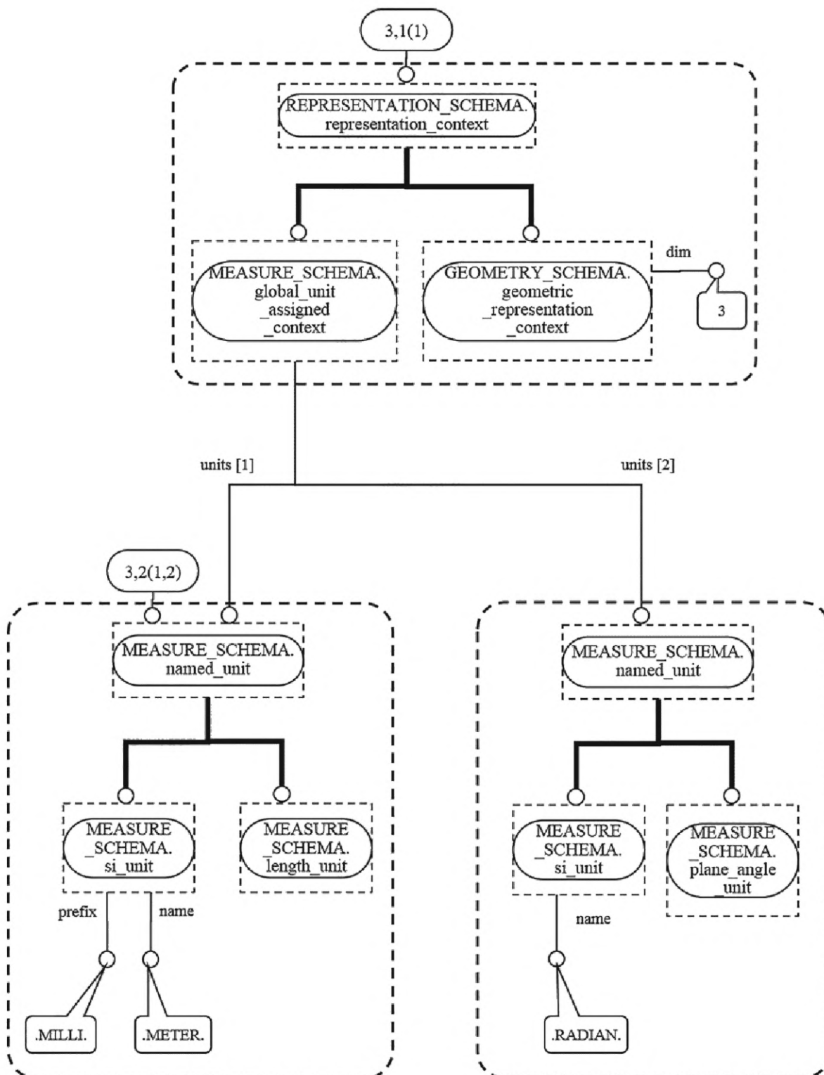
Рисунок F.7 — Пример экземпляров объектов, представляющих информацию о качестве, используемых для представления требований/заявления с заданием точности (3 из 3)
