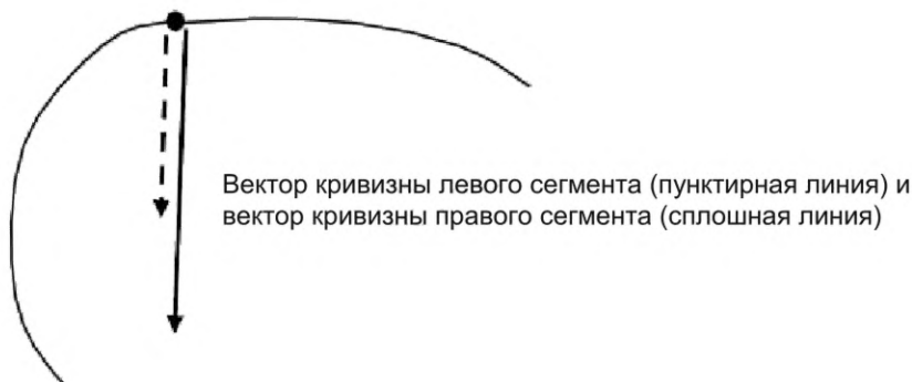
Рисунок 12 — Разрыв G2 вследствие разности значений радиусов кривизны
