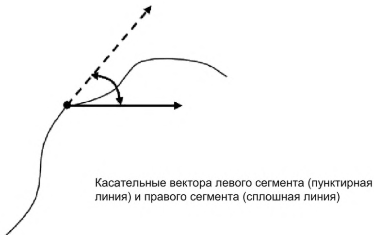
Рисунок 9 — Кривая, имеющая разрыв G1
