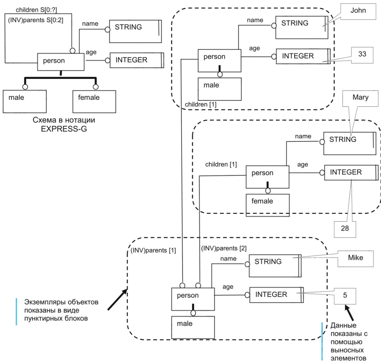
Рисунок F.1 — Пример использования нотации
