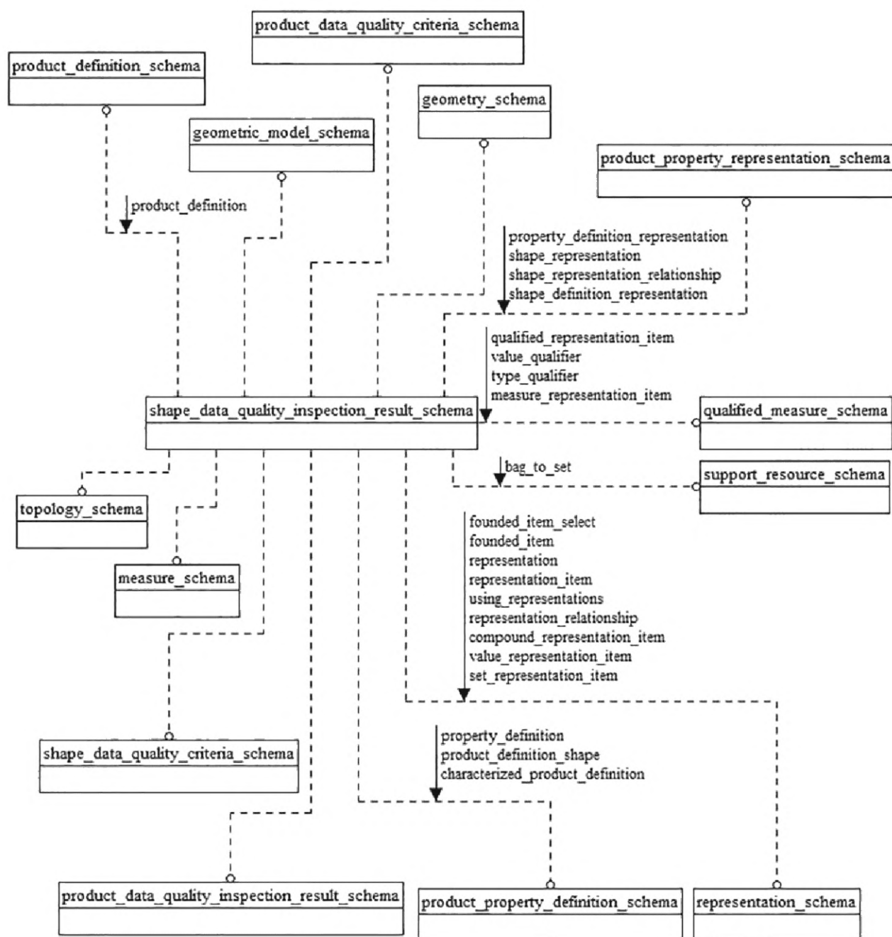
Рисунок D.16 — EXPRESS-G диаграмма схемы shape_data_quality_inspection_result_schema (диаграмма 1 из 5)
