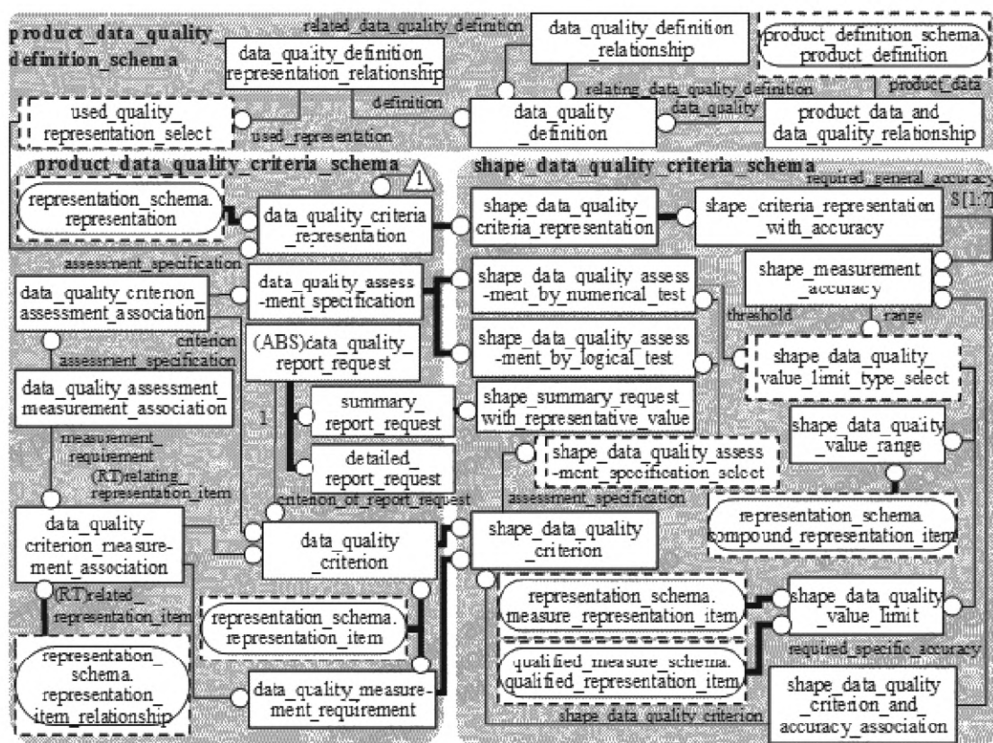
Рисунок Е.12 — Информация о качестве, используемая при задании требований к качеству данных и для заявления о качестве данных
