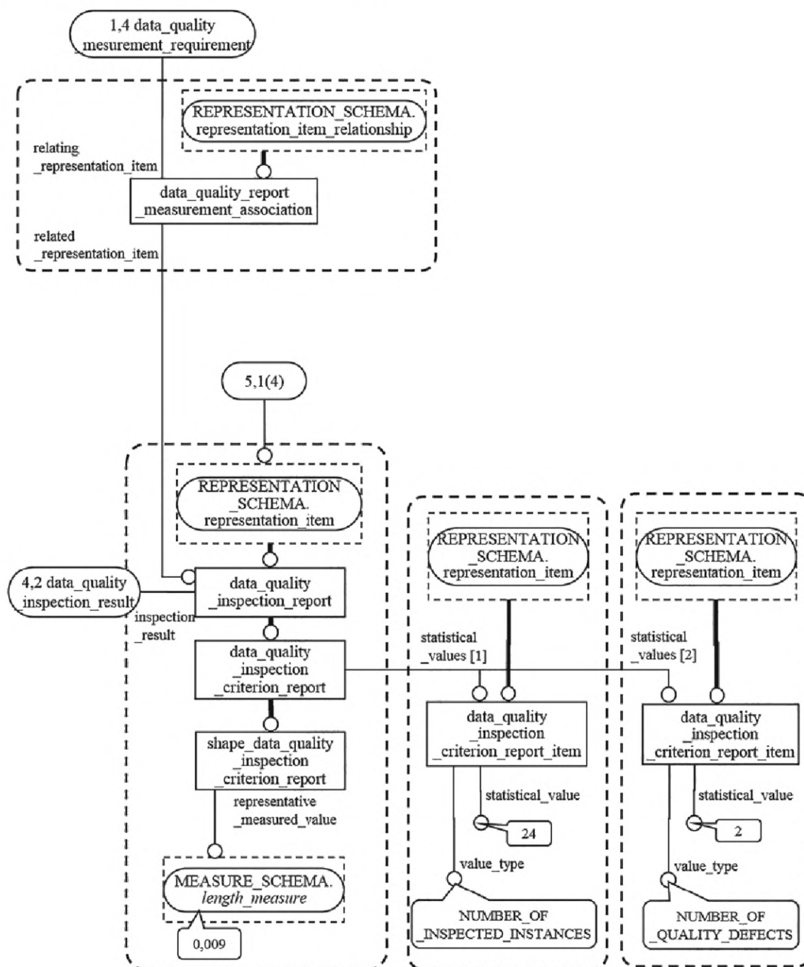
Рисунок F.12 — Примеры экземпляров, образующих информацию о качестве, используемую для обеспечения уверенности в качестве относительно критерия short_length_edge (5 из 6)
