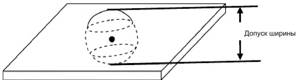
Рисунок 5 — Измерение полностью узкого твердого тела
