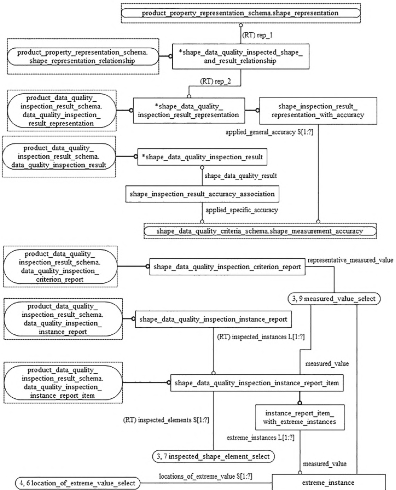
Рисунок D.17 — EXPRESS-G диаграмма схемы shape_data_quality_inspection_result_schema (диаграмма 2 из 5)
