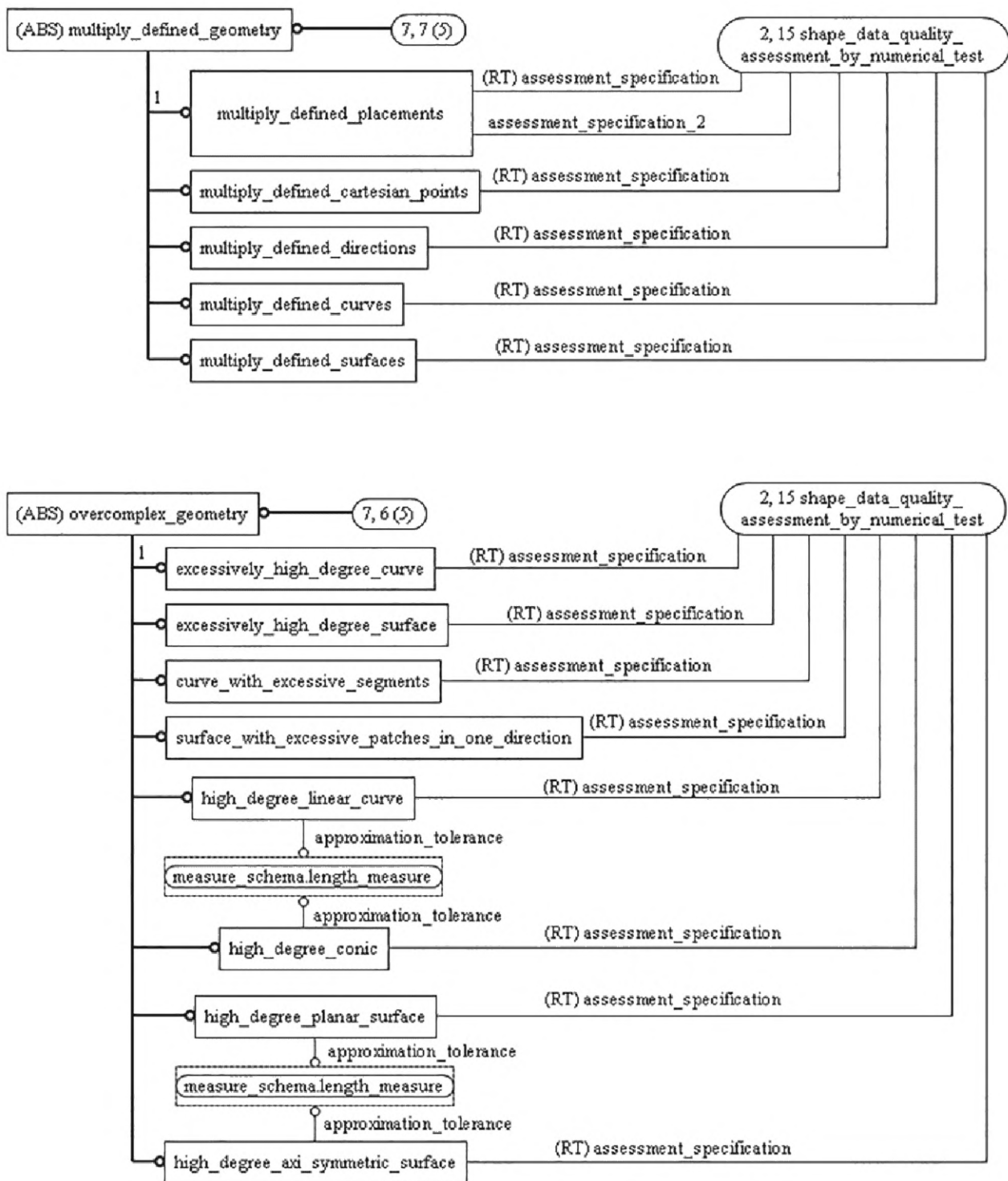
Рисунок D.13 — EXPRESS-G диаграмма схемы shape_data_quality_criteria_schema (диаграмма 7 из 9)
