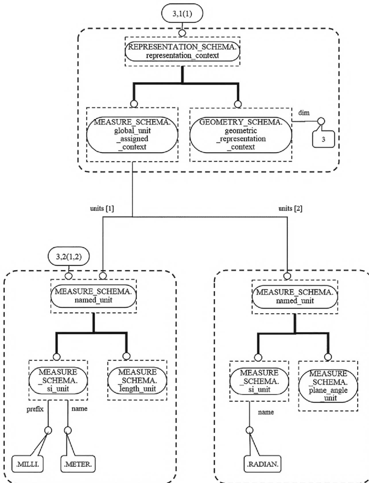
Рисунок F.23 — Примеры экземпляров, образующих информацию о качестве, используемую для улучшения качества относительно критерия gap_between_edge_and_base_surface (3 из 7)
