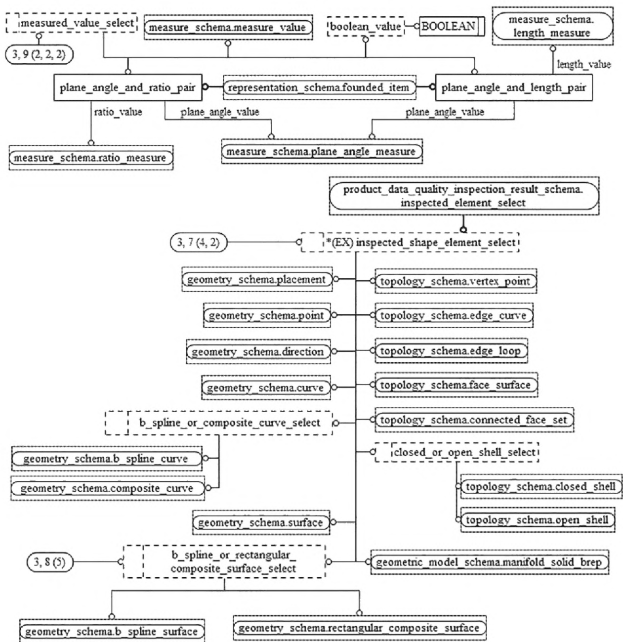
Рисунок D.18 — EXPRESS-G диаграмма схемы shape_data_quality_inspection_result_schema (диаграмма 3 из 5)
