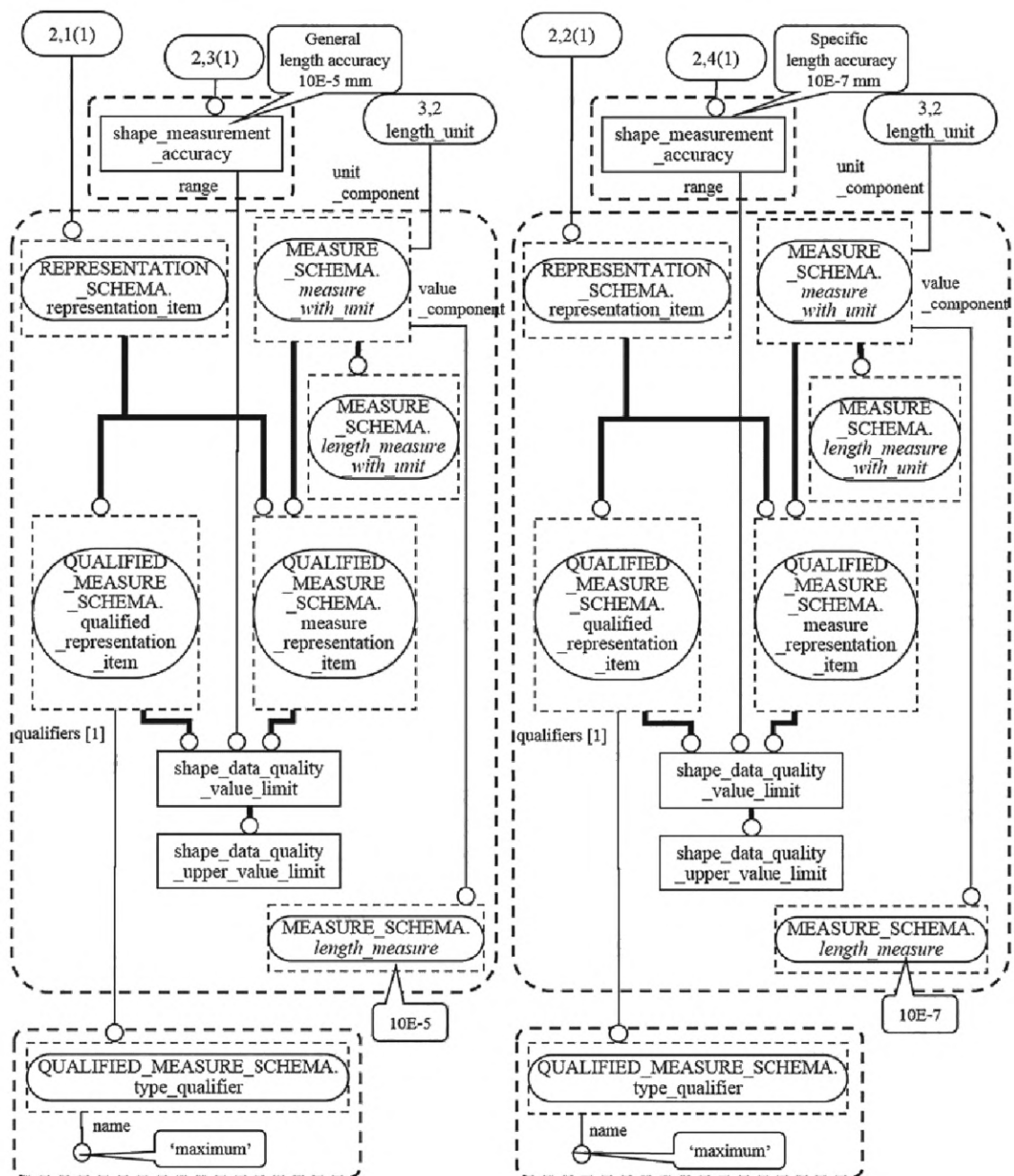
Рисунок F.15 — Примеры экземпляров, образующих информацию о качестве, используемую для улучшения качества относительно критерия short_length_edge (2 из 7)
