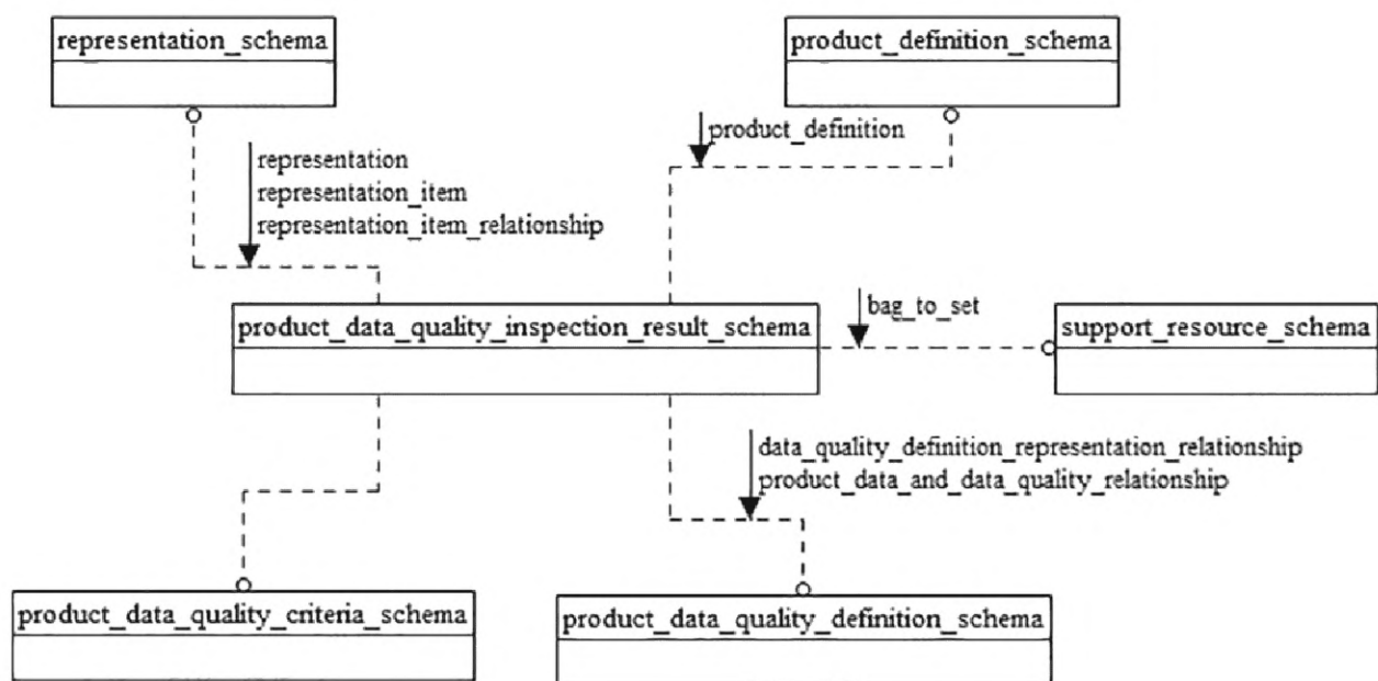
Рисунок D.5 — EXPRESS-G диаграмма схемы product_data_quality_inspection_result_schema (диаграмма 1 из 2)
