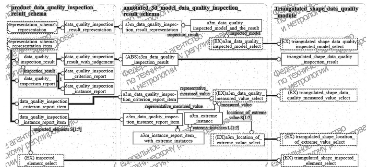
Рисунок Е.4 — Схема EXPRESS-G, показывающая связь ресурсов результатов проверки с модулем качества данных триангулированной формы
