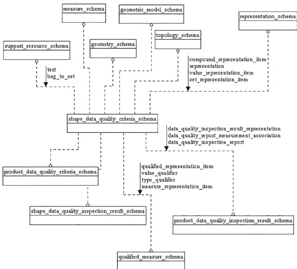
Рисунок D.7 — EXPRESS-G диаграмма схемы shape_data_quality_criteria_schema (диаграмма 1 из 9)
