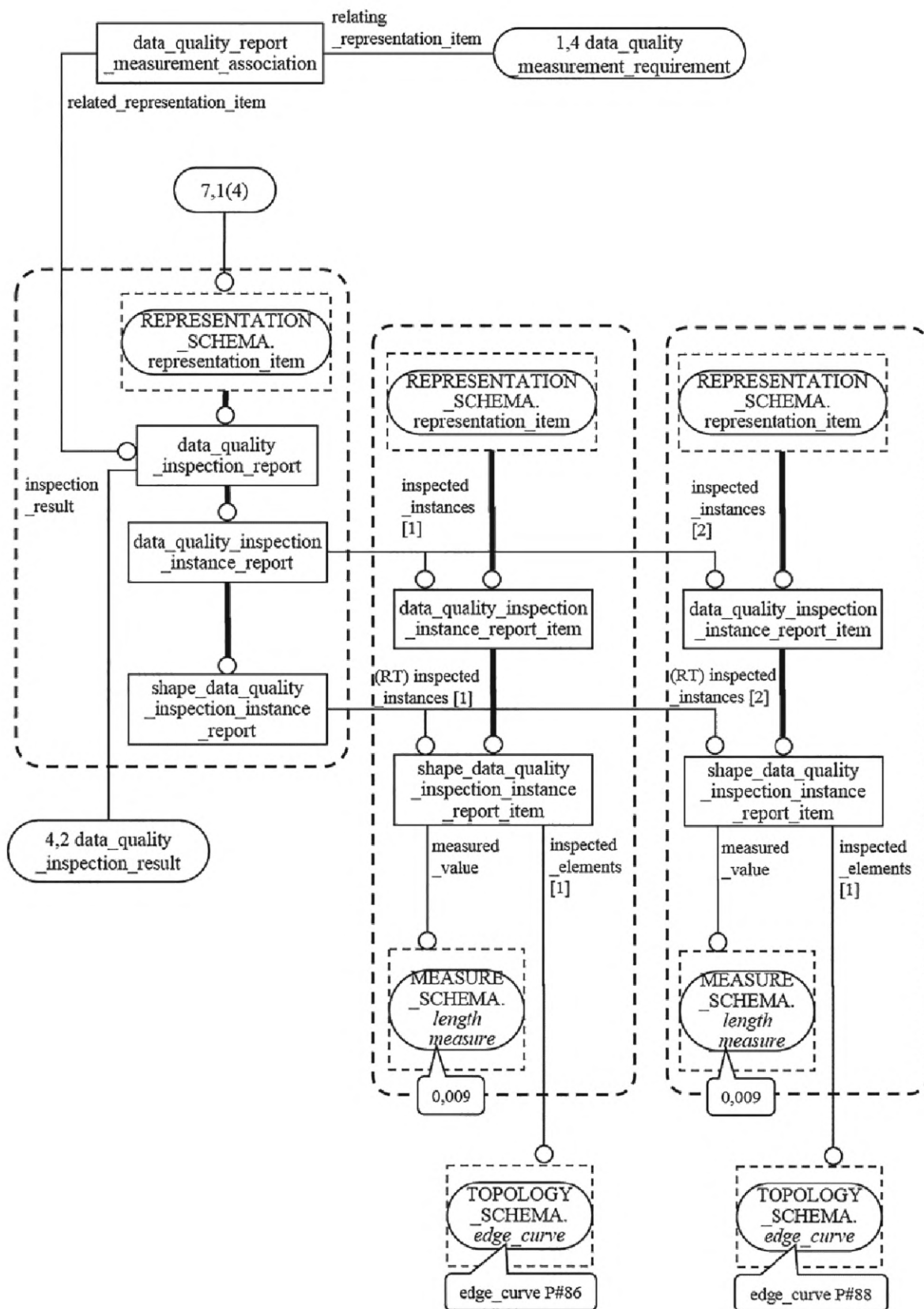
Рисунок F.20 — Примеры экземпляров, образующих информацию о качестве, используемую для улучшения качества относительно критерия short_length_edge (7 из 7)
