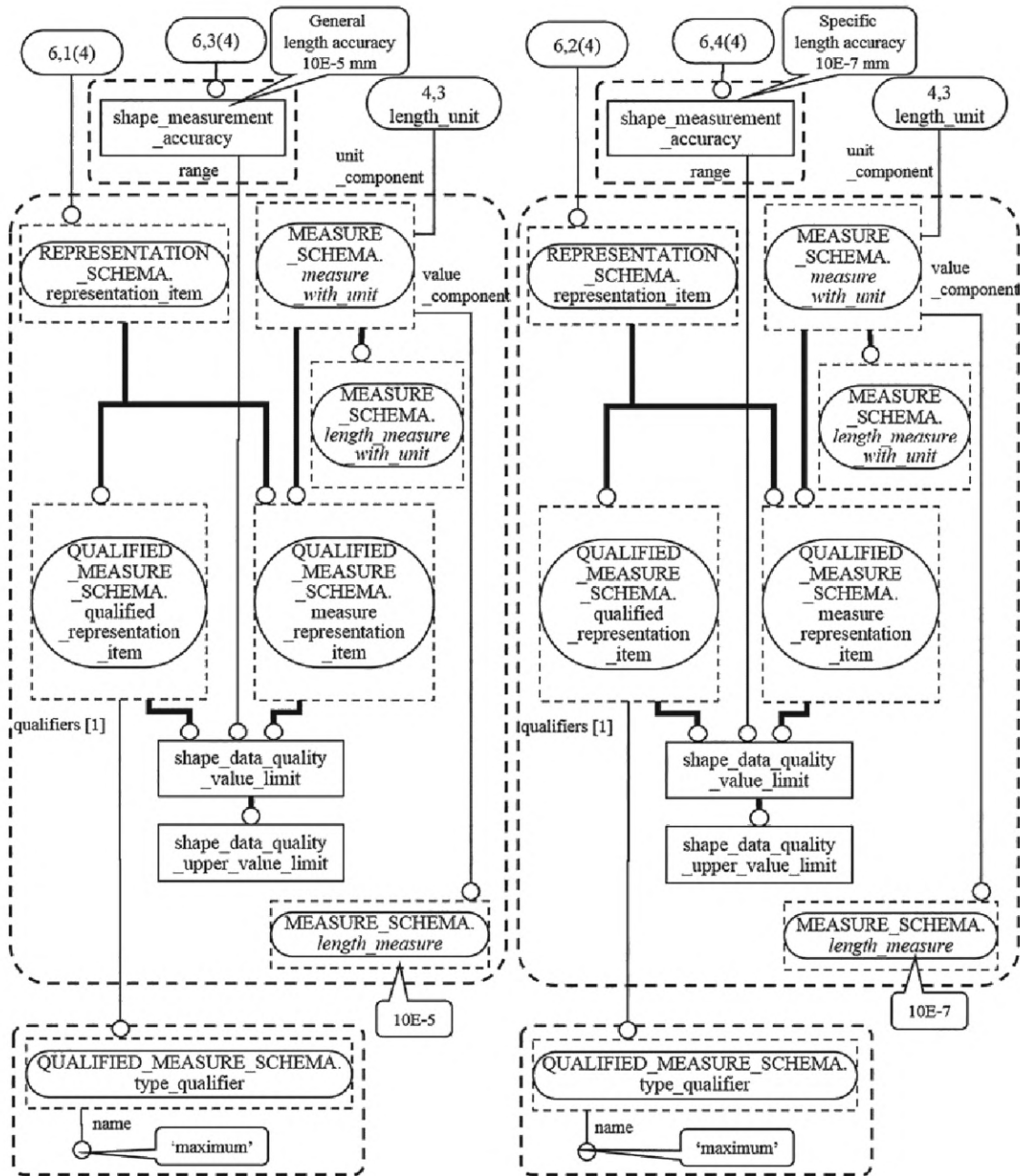
Рисунок F.13 — Примеры экземпляров, образующих информацию о качестве, используемую для обеспечения уверенности в качестве относительно критерия short_length_edge (6 из 6)
