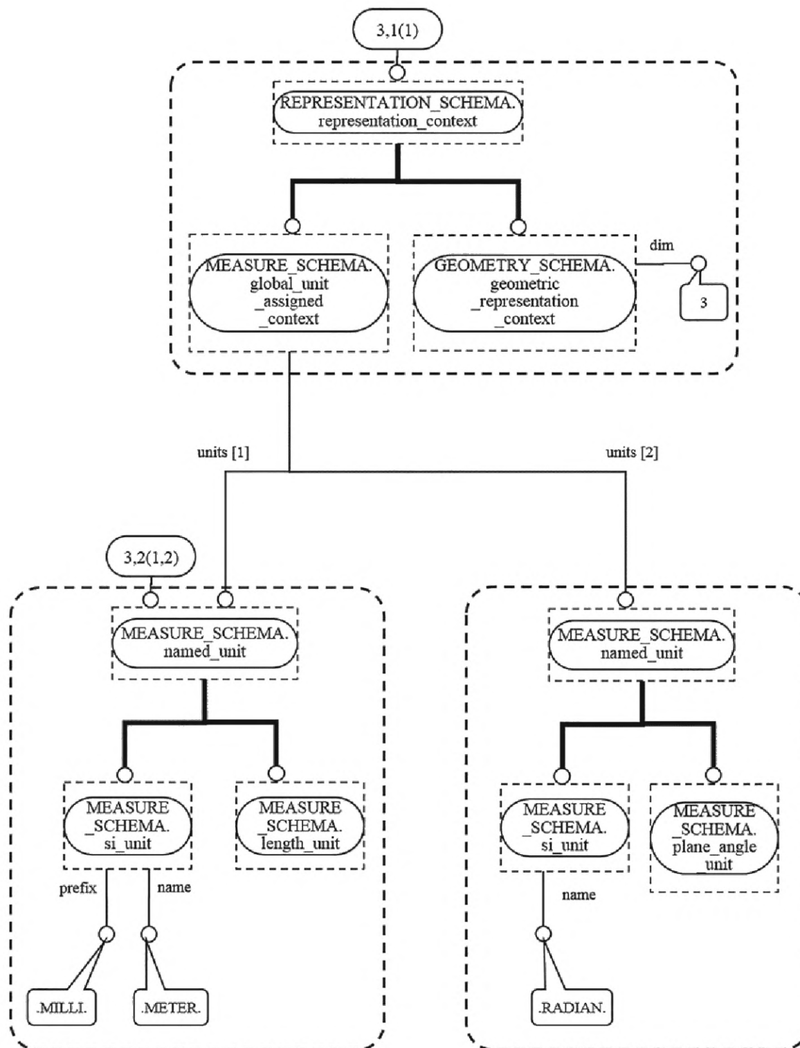
Рисунок F.16 — Примеры экземпляров, образующих информацию о качестве, используемую для улучшения качества относительно критерия short_length_edge (3 из 7)
