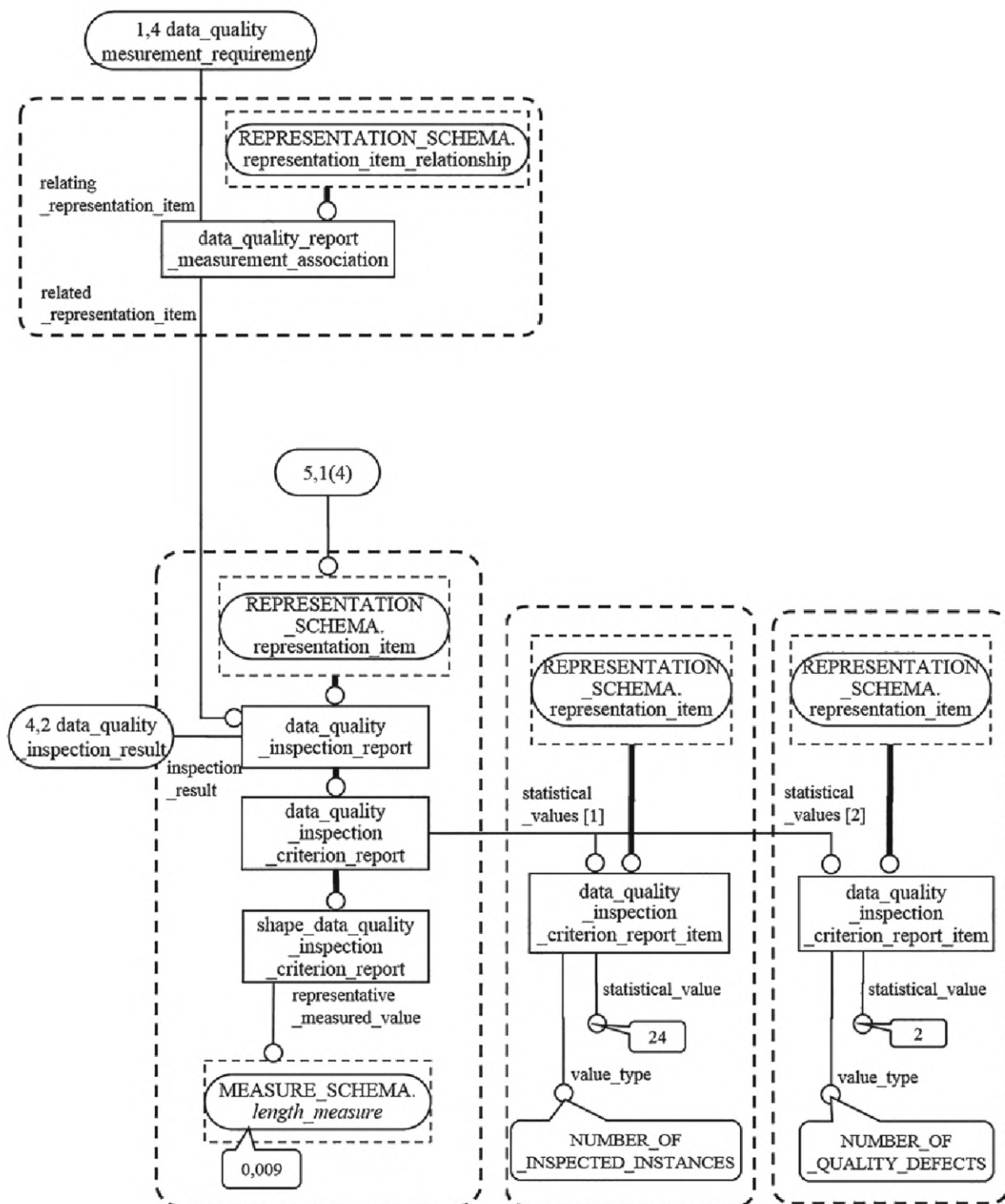
Рисунок F.18 — Примеры экземпляров, образующих информацию о качестве, используемую для улучшения качества относительно критерия short_length_edge (5 из 7)
