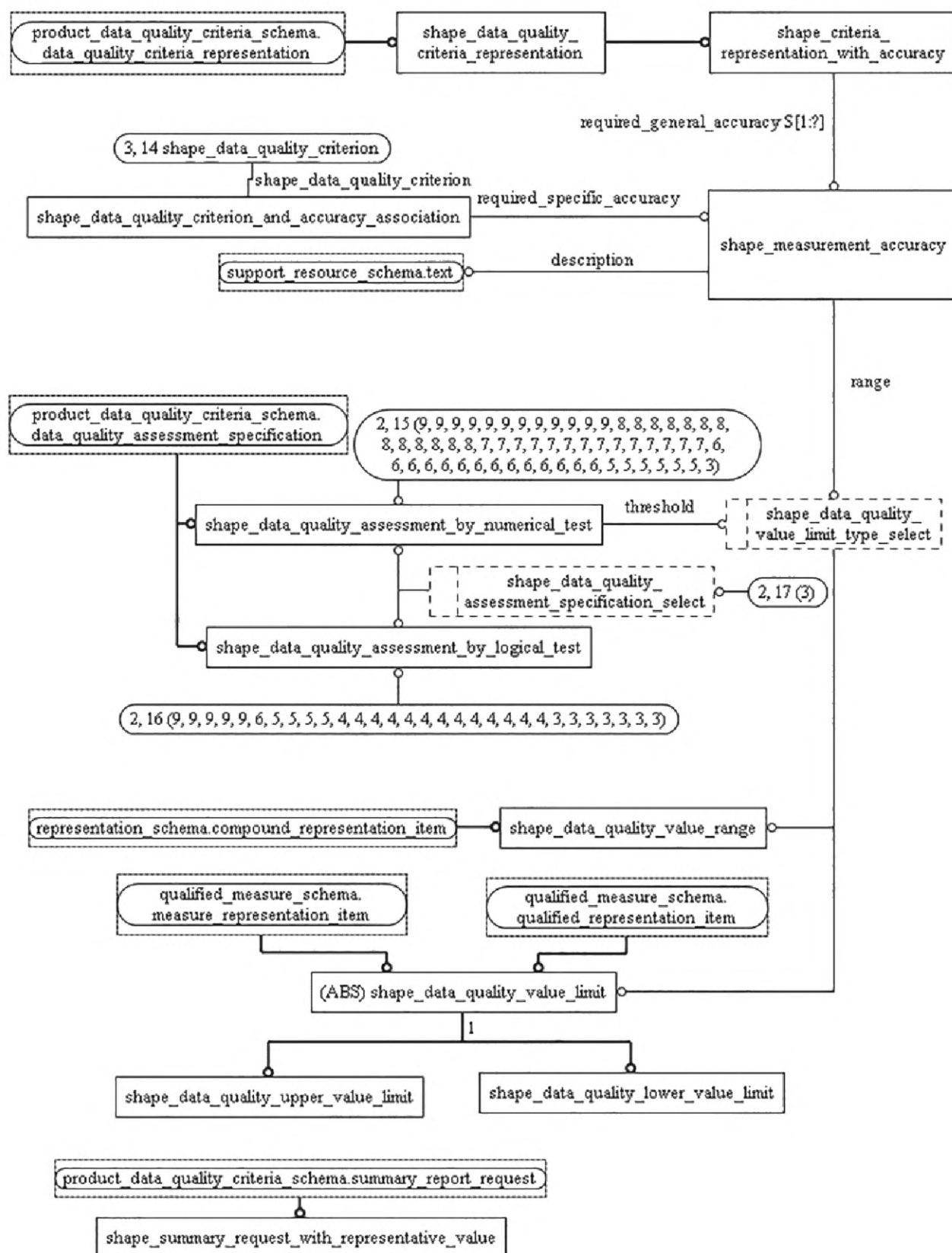
Рисунок D.8 — EXPRESS-G диаграмма схемы shape_data_quality_criteria_schema (диаграмма 2 из 9)
