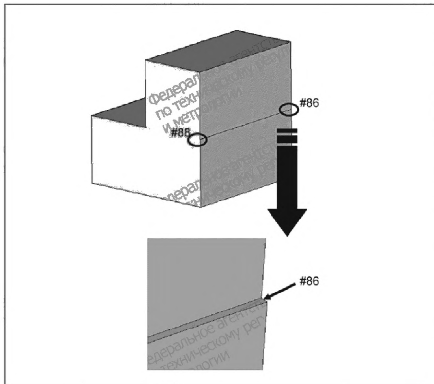
Рисунок F.2 — Типичный пример ребра короткой длины
