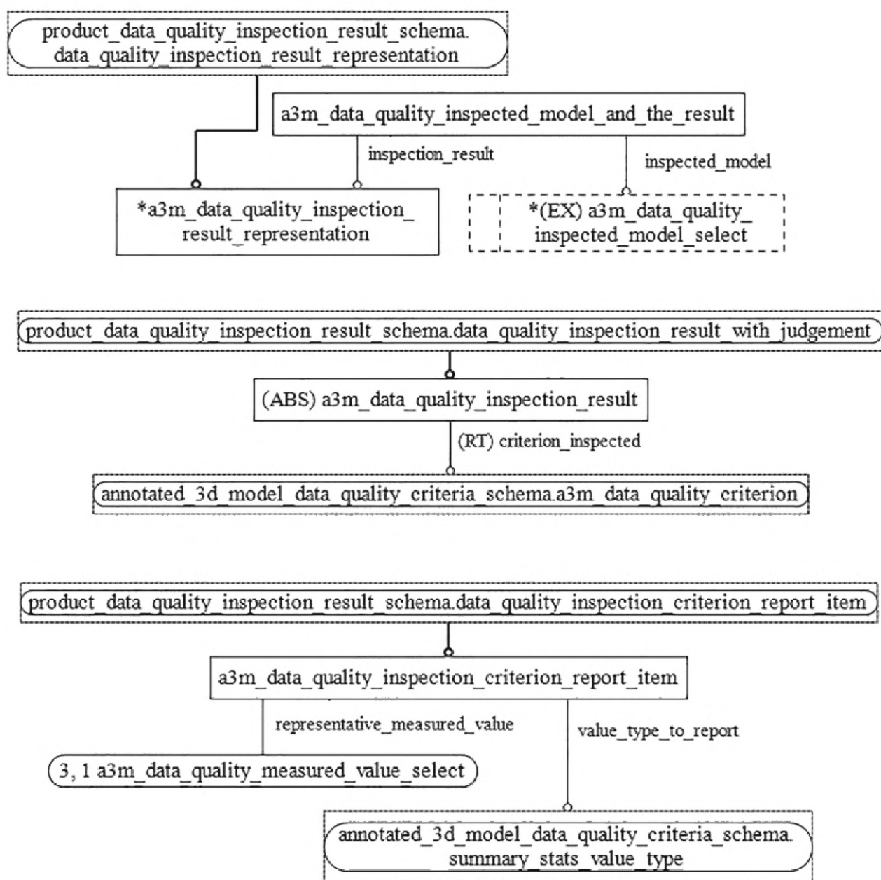
Рисунок D.25 — EXPRESS-G диаграмма схемы annotated_3d_model_data_quality_inspection_result_schema (диаграмма 2 из 3)
