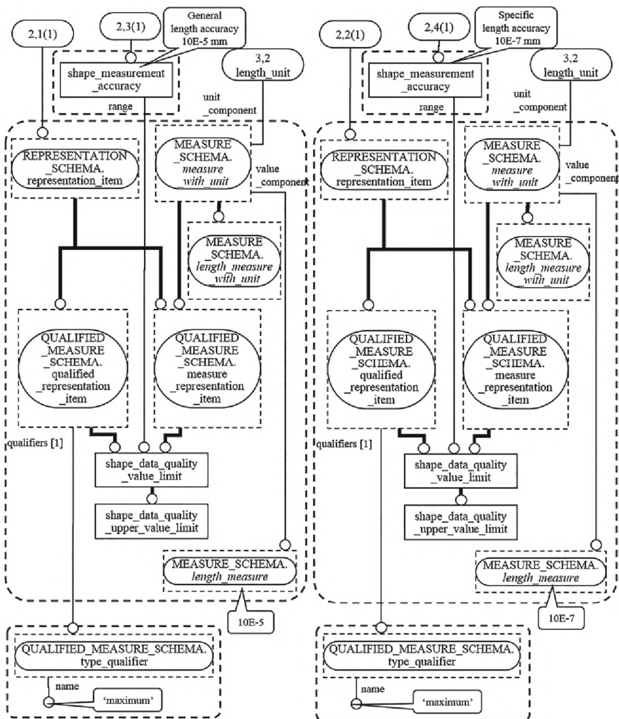
Рисунок F.9 — Примеры экземпляров, образующих информацию о качестве, используемую для обеспечения уверенности в качестве относительно критерия short_length_edge (2 из 6)
