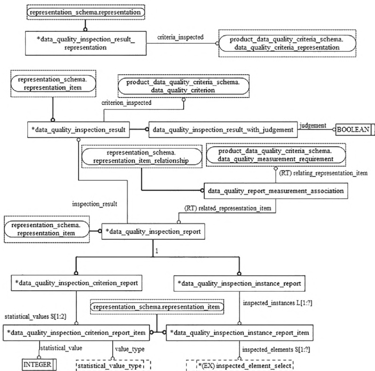
Рисунок D.6 — EXPRESS-G диаграмма схемы product_data_quality_inspection_result_schema (диаграмма 2 из 2)
