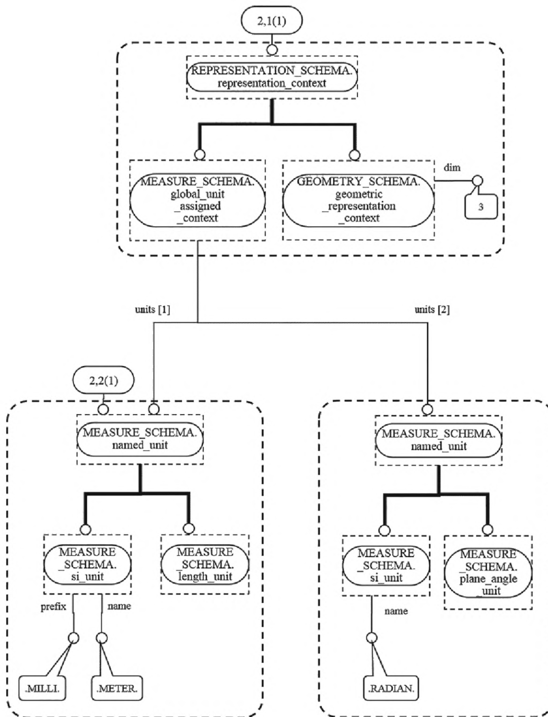
Рисунок F.4 — Пример экземпляров объектов, представляющих информацию о качестве, используемых для представления требований/заявления без задания точности (2 из 2)
