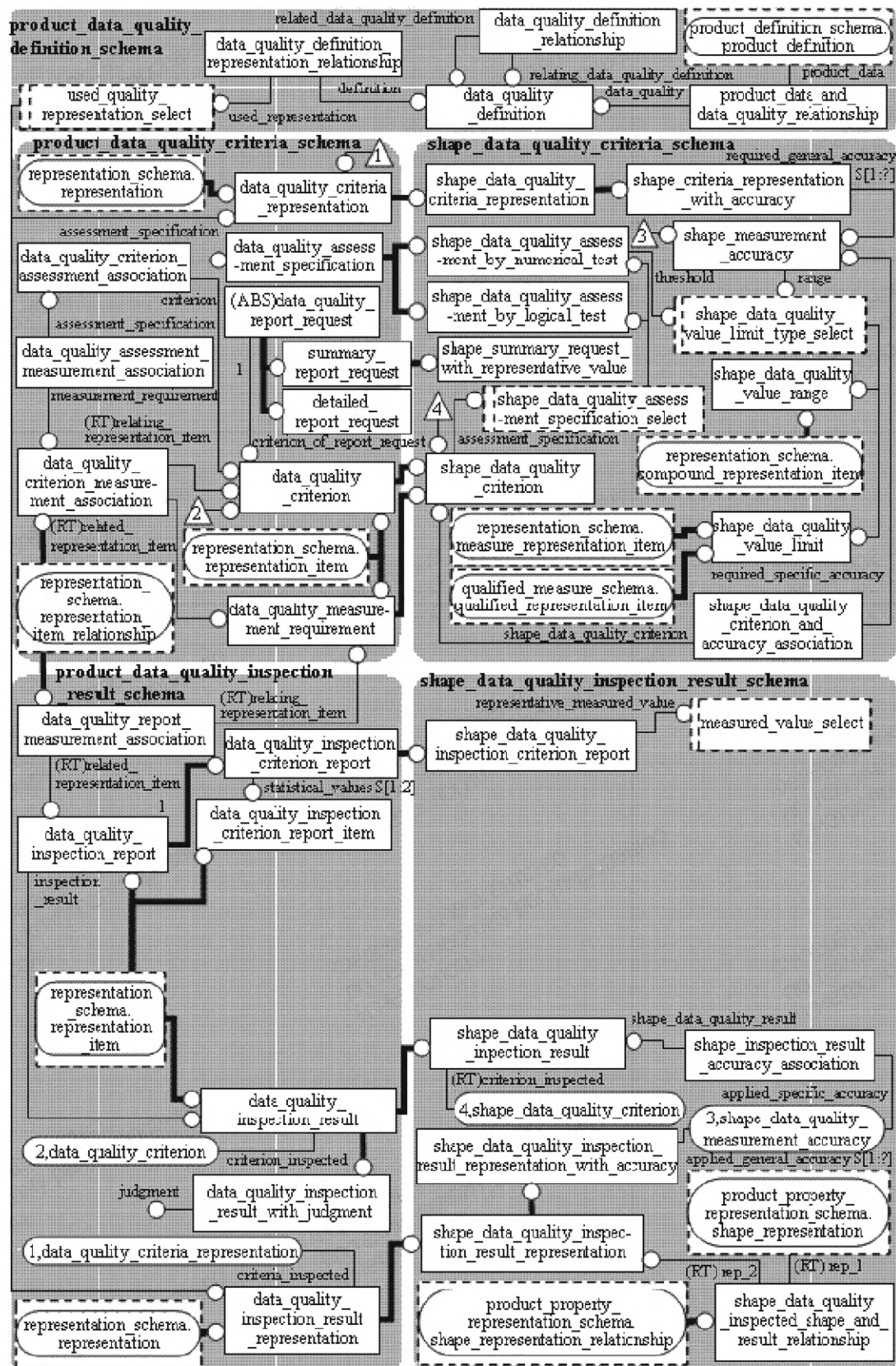
Рисунок Е.13 — Информация о качестве, используемая для обеспечения уверенности в качестве данных
