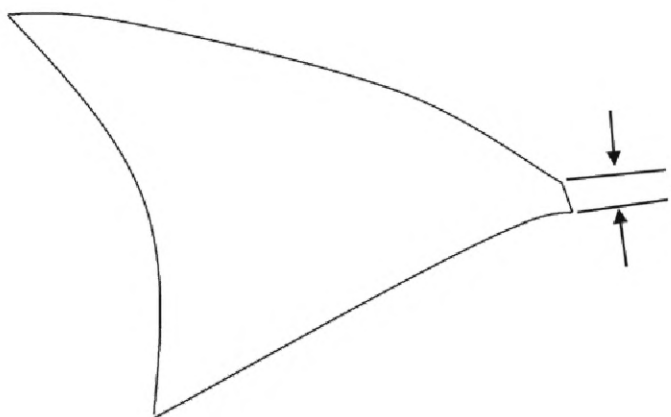
Рисунок 23 — Близкая к вырождению граница поверхности
