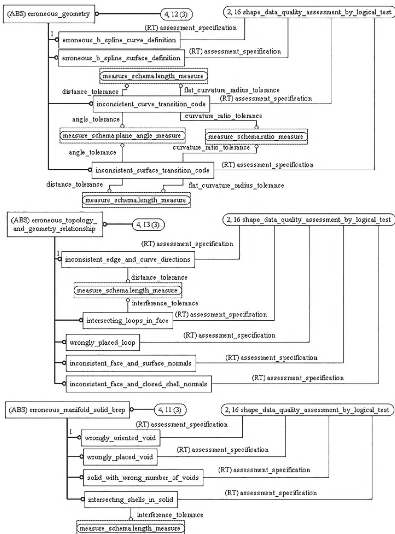
Рисунок D.10 — EXPRESS-G диаграмма схемы shape_data_quality_criteria_schema (диаграмма 4 из 9)
