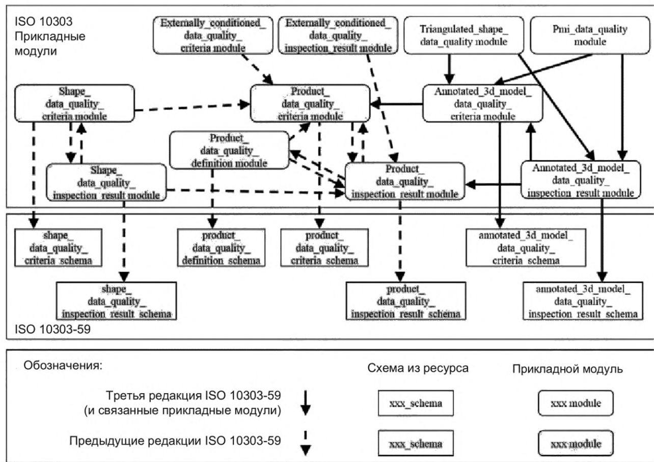
Рисунок Е.1 — Структурное отношение между относящимися к PDQ схемам и соответствующими прикладными модулями
