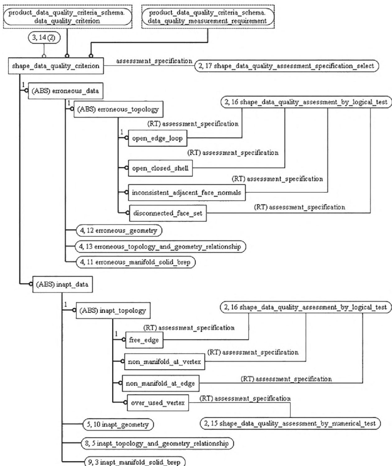
Рисунок D.9 — EXPRESS-G диаграмма схемы shape_data_quality_criteria_schema (диаграмма 3 из 9)
