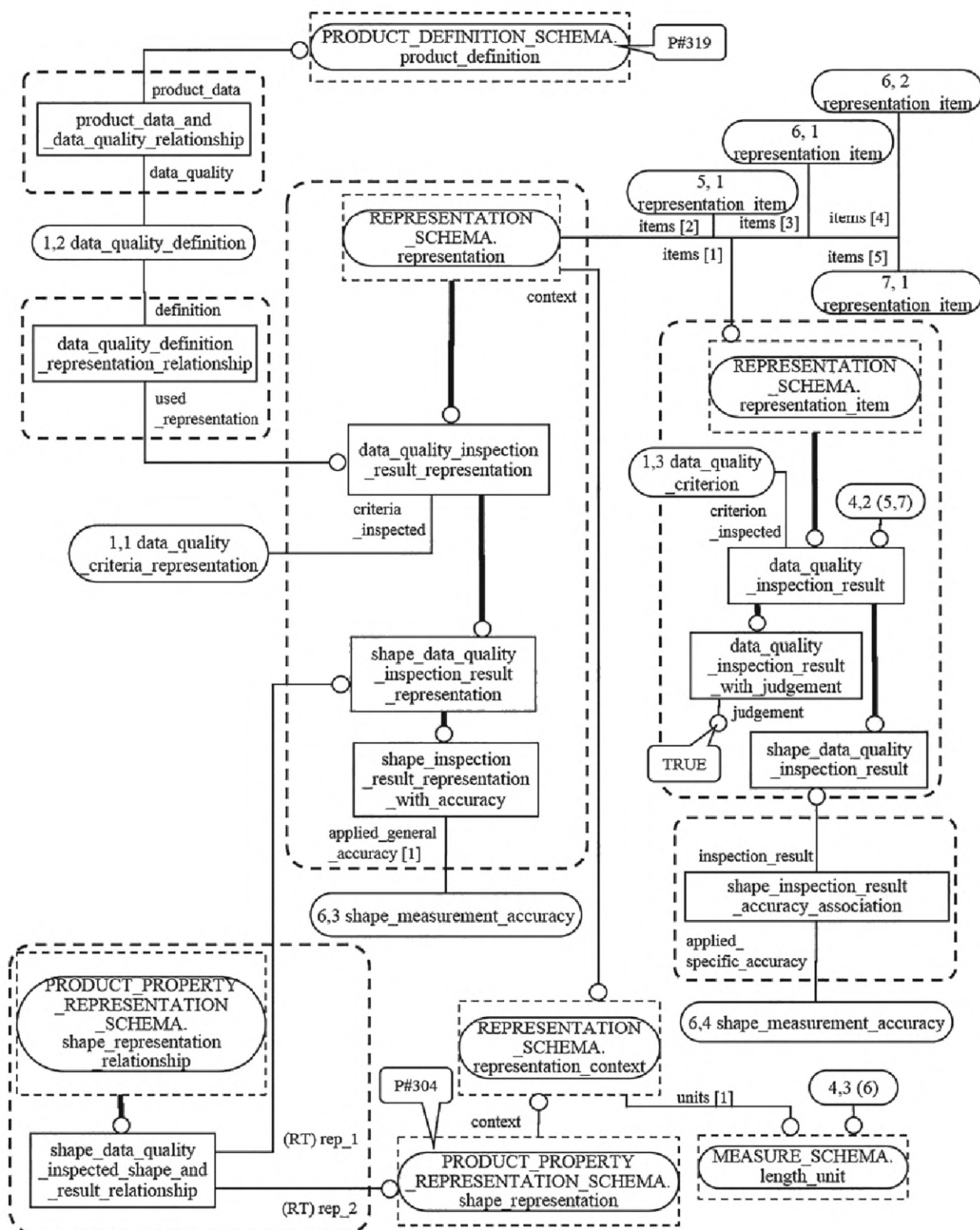
Рисунок F.17 — Примеры экземпляров, образующих информацию о качестве, используемую для улучшения качества относительно критерия short_length_edge (4 из 7)
