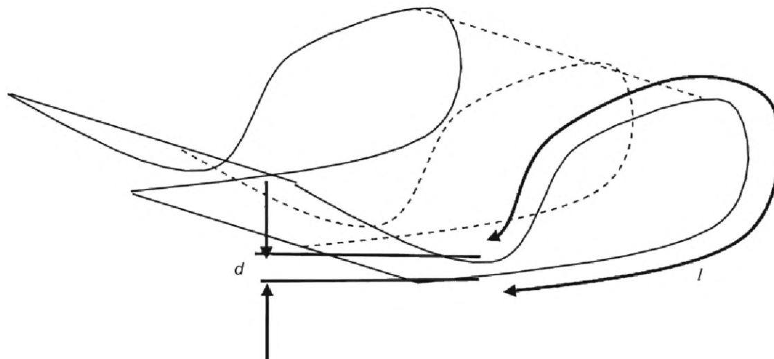
Рисунок 34 — Самопересекающаяся поверхность
