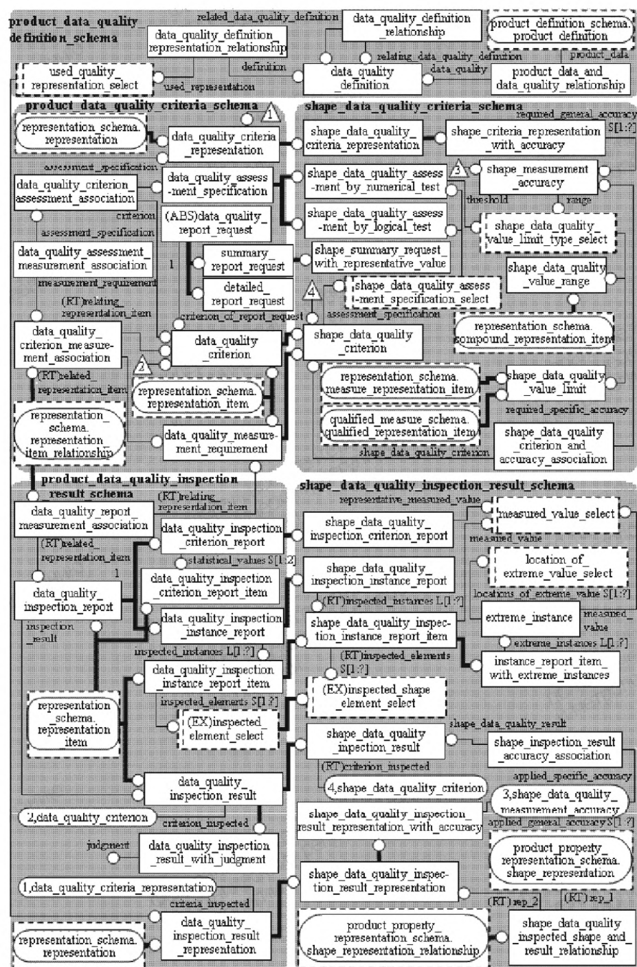
Рисунок Е.14 — Информация о качестве, используемая для улучшения качества
