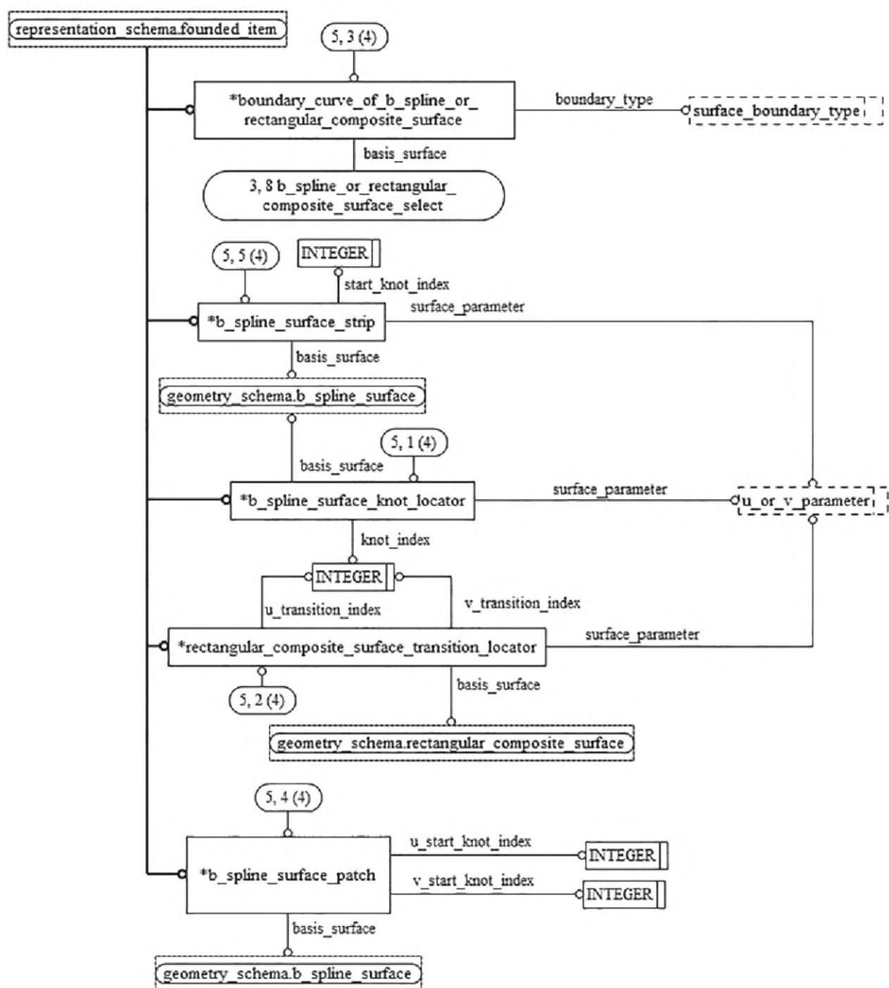
Рисунок D.20 — EXPRESS-G диаграмма схемы shape_data_quality_inspection_result_schema (диаграмма 5 из 5)
