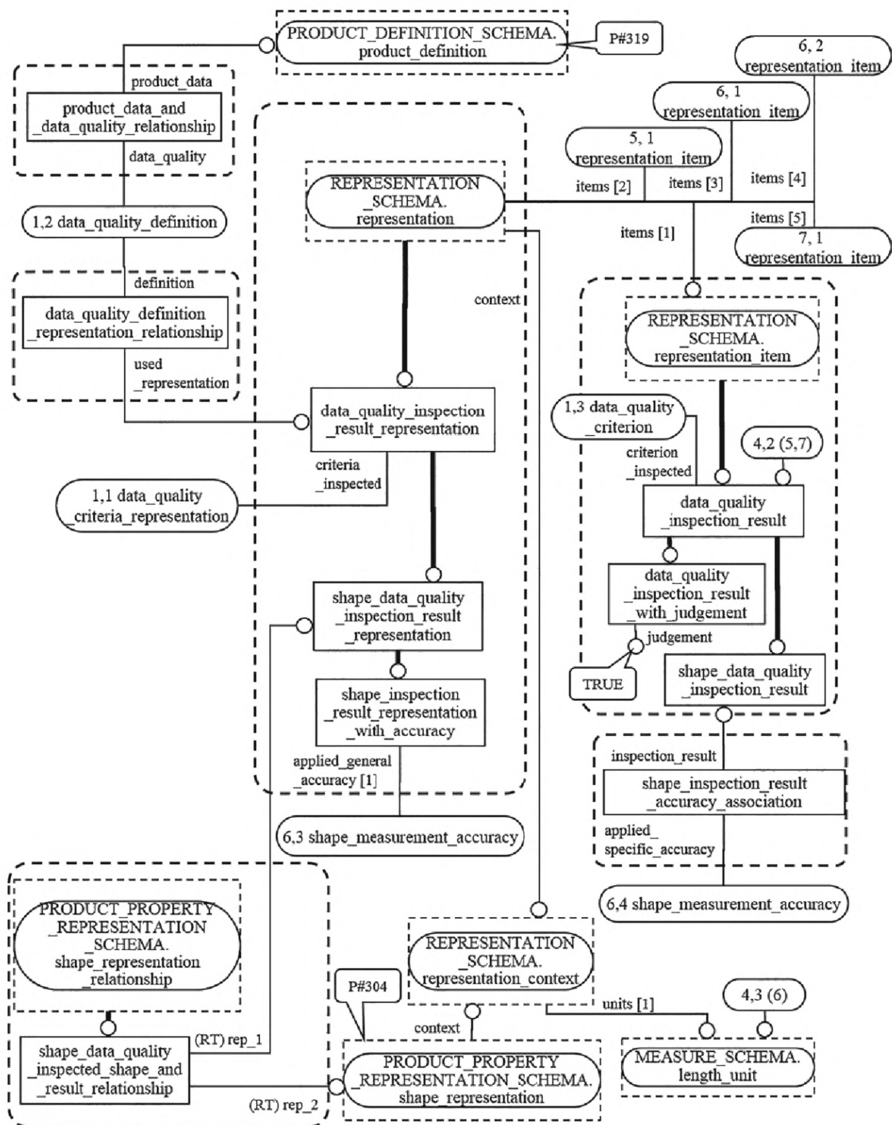
Рисунок F.24 — Примеры экземпляров, образующих информацию о качестве, используемую для улучшения качества относительно критерия gap between edge and base surface (4 из 7)
