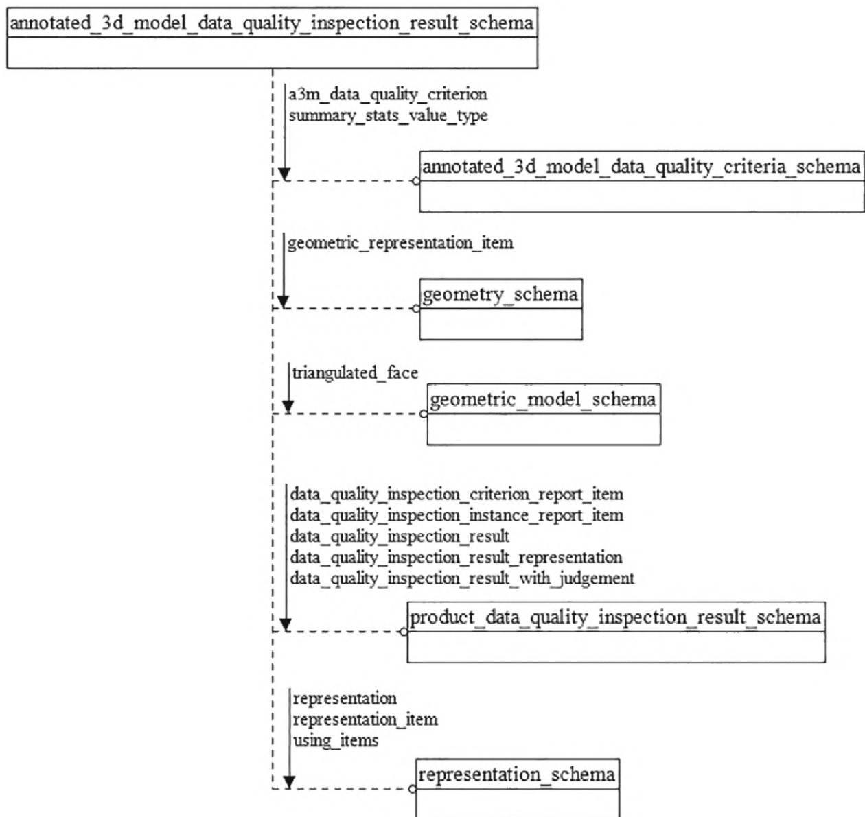
Рисунок D.24 — EXPRESS-G диаграмма схемы annotated_3d_model_data_quality_inspection_result_schema (диаграмма 1 из 3)
