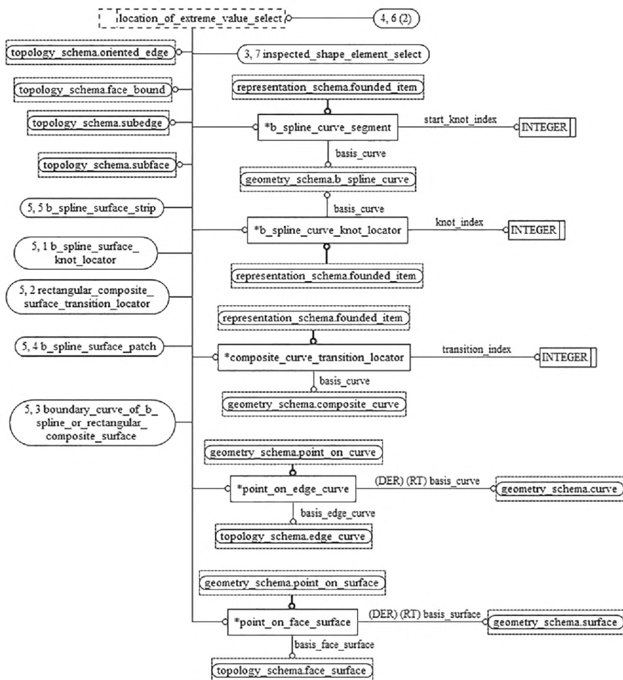
Рисунок D.19 — EXPRESS-G диаграмма схемы shape_data_quality_inspection_result_schema (диаграмма 4 из 5)
