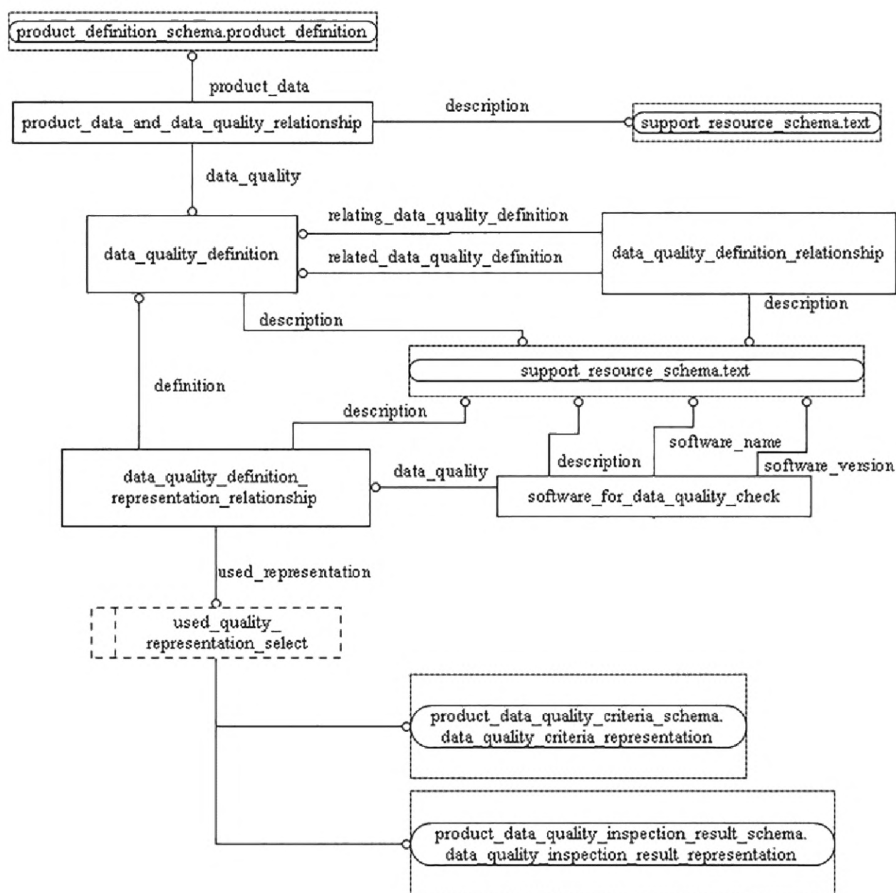
Рисунок D.2 — EXPRESS-G диаграмма схемы product_data_quality_definition_schema (диаграмма 2 из 2)
