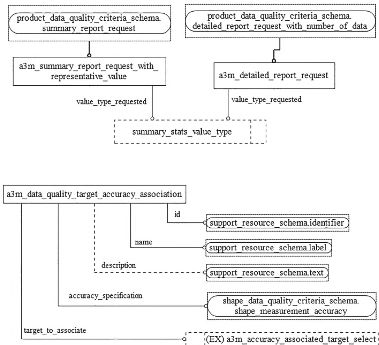
Рисунок D.23 — EXPRESS-G диаграмма схемы annotated_3d_model_data_quality_criteria_schema (диаграмма 3 из 3)
