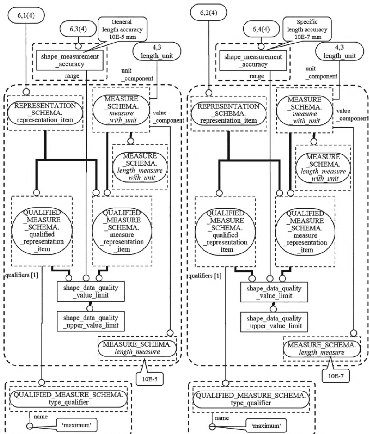
Рисунок F.26 — Примеры экземпляров, образующих информацию о качестве, используемую для улучшения качества относительно критерия gap_between_edge_and_base_surface (6 из 7)
