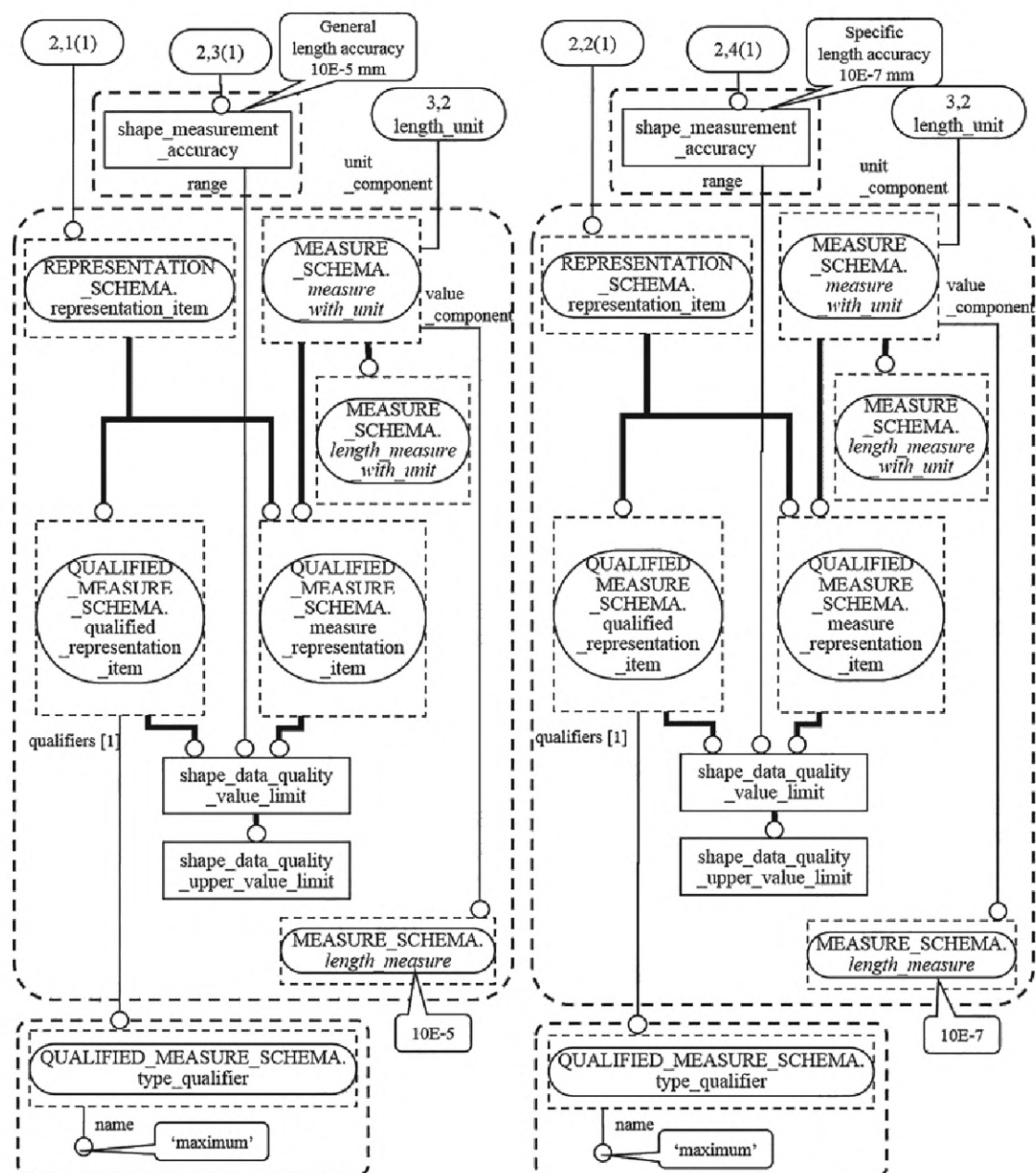
Рисунок F.6 — Пример экземпляров объектов, представляющих информацию о качестве, используемых для представления требований/заявления с заданием точности (2 из 3)
