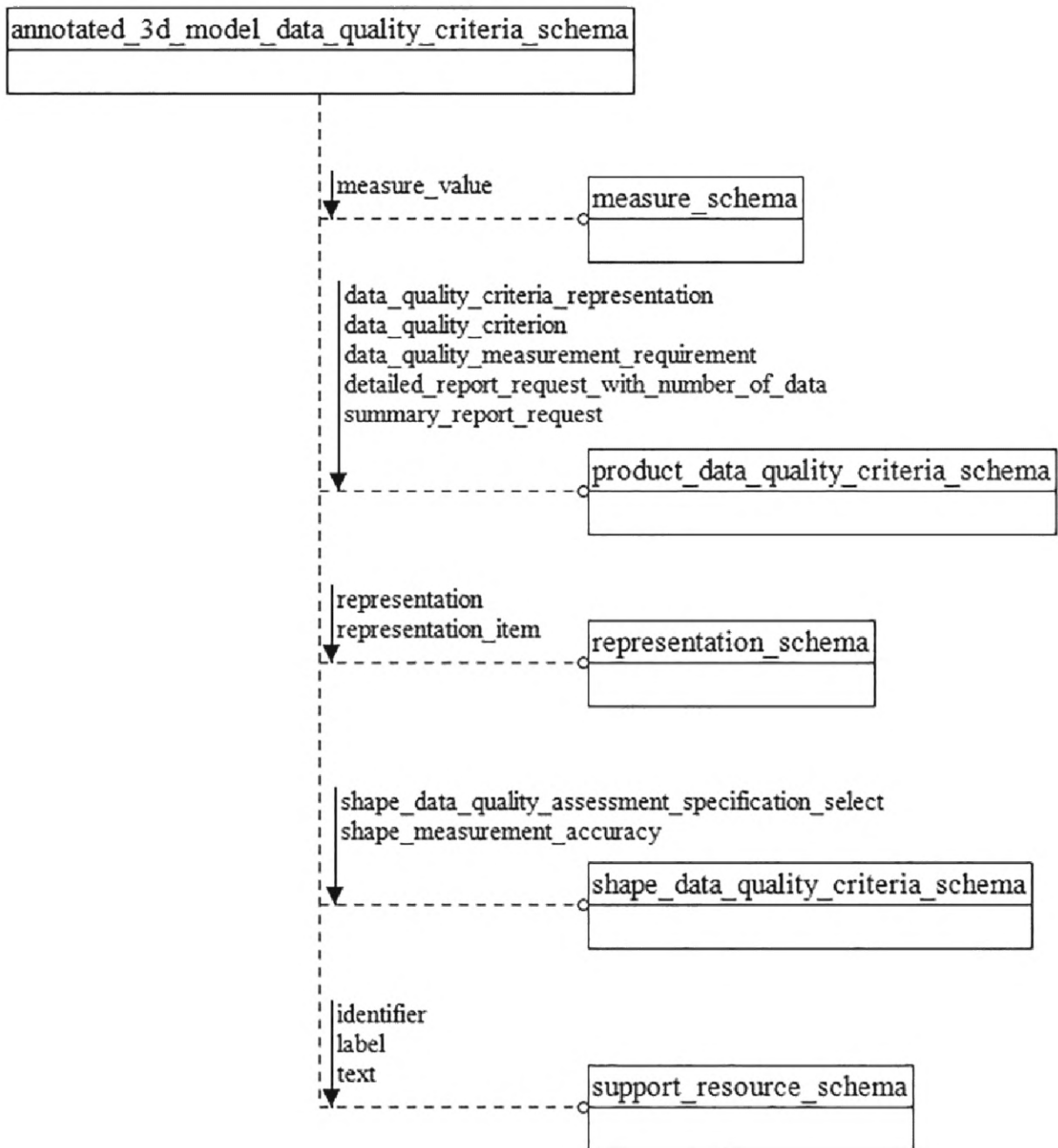
Рисунок D.21 — EXPRESS-G диаграмма схемы annotated_3d_model_data_quality_criteria_schema (диаграмма 1 из 3)
