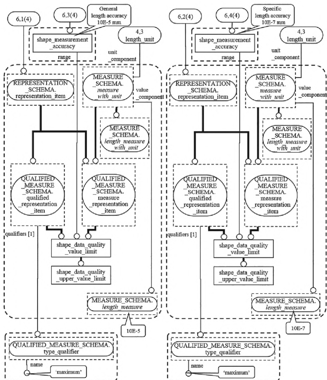
Рисунок F.19 — Примеры экземпляров, образующих информацию о качестве, используемую для улучшения качества относительно критерия short_length_edge (6 из 7)
