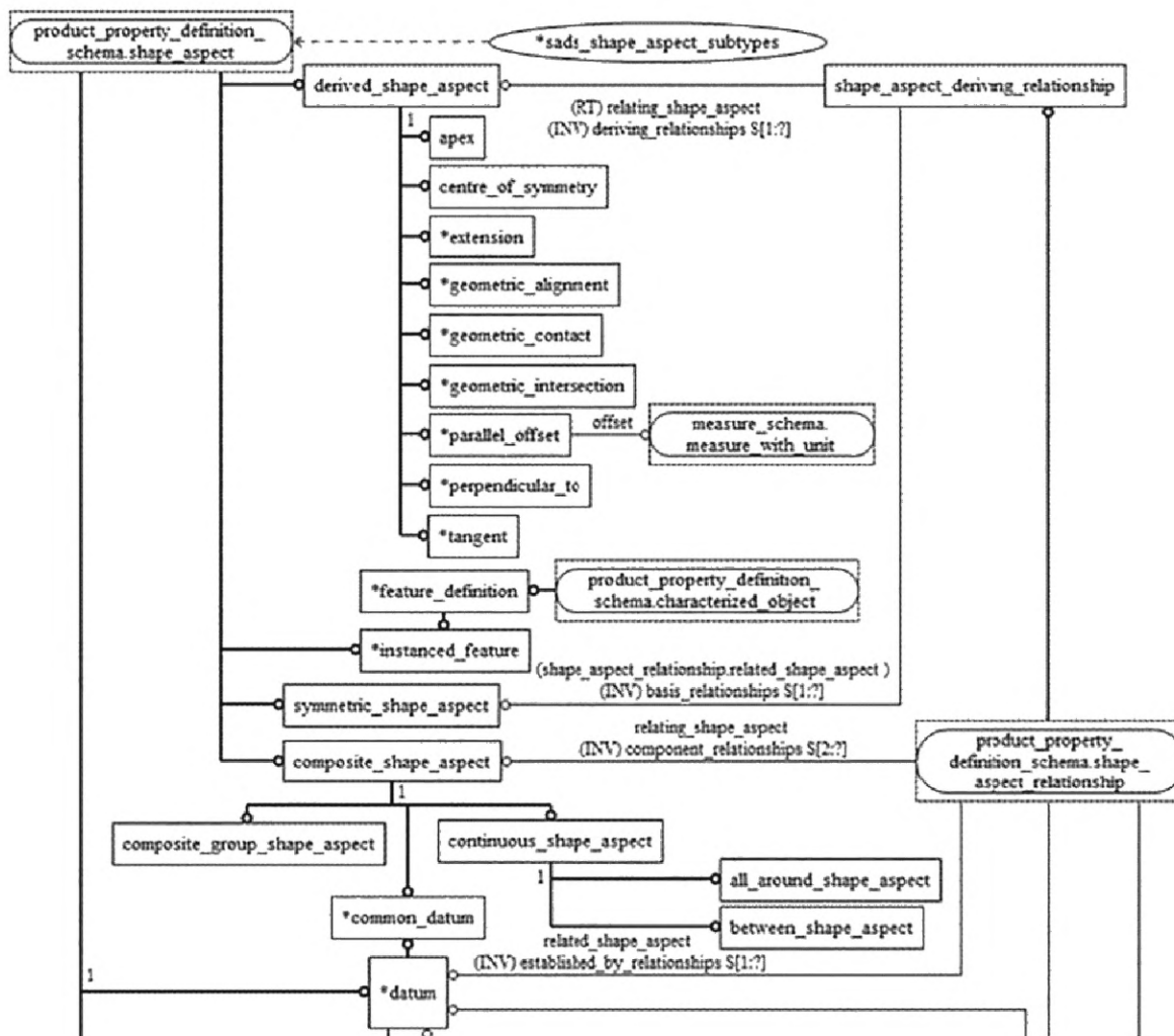
Рисунок Е.9 — Изображение подмножества информационной модели изделия в формате ИСО 10303 с использованием нотации, описанной в ИСО 10303-11
