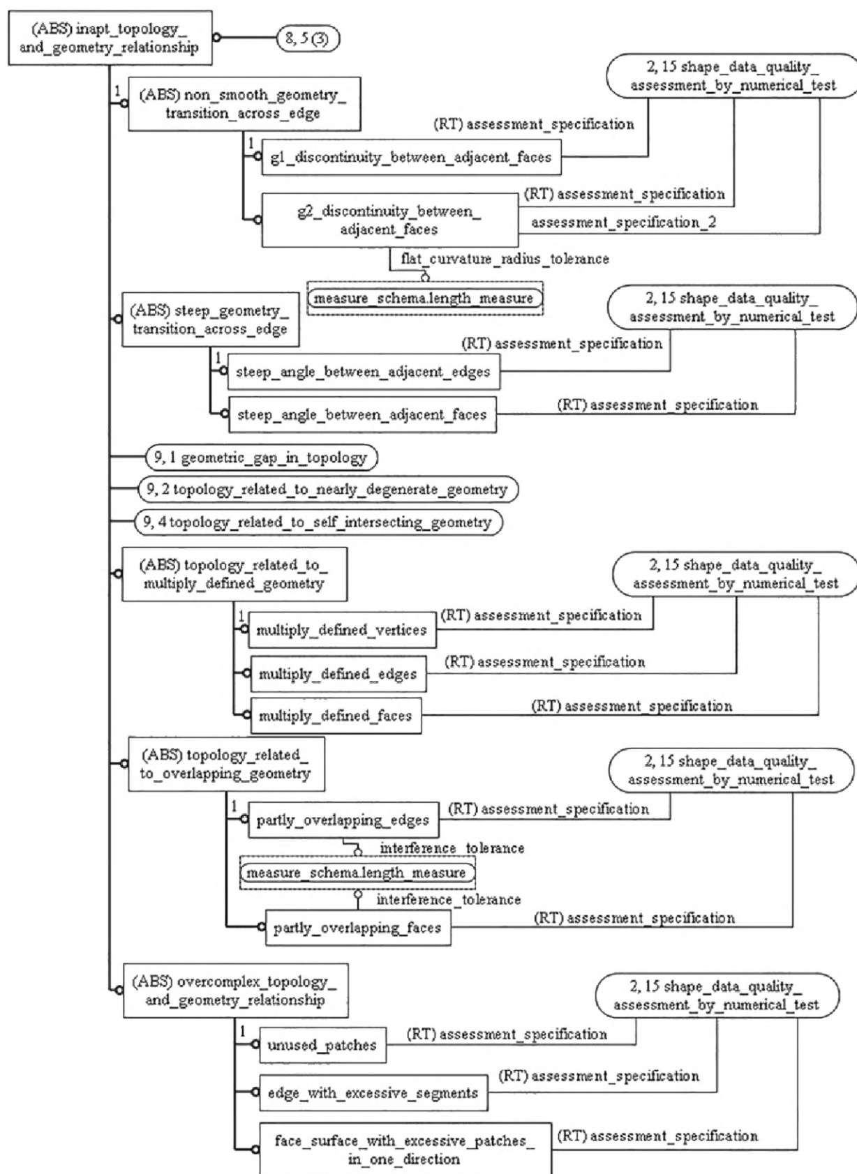
Рисунок D.14 — EXPRESS-G диаграмма схемы shape_data_quality_criteria_schema (диаграмма 8 из 9)
