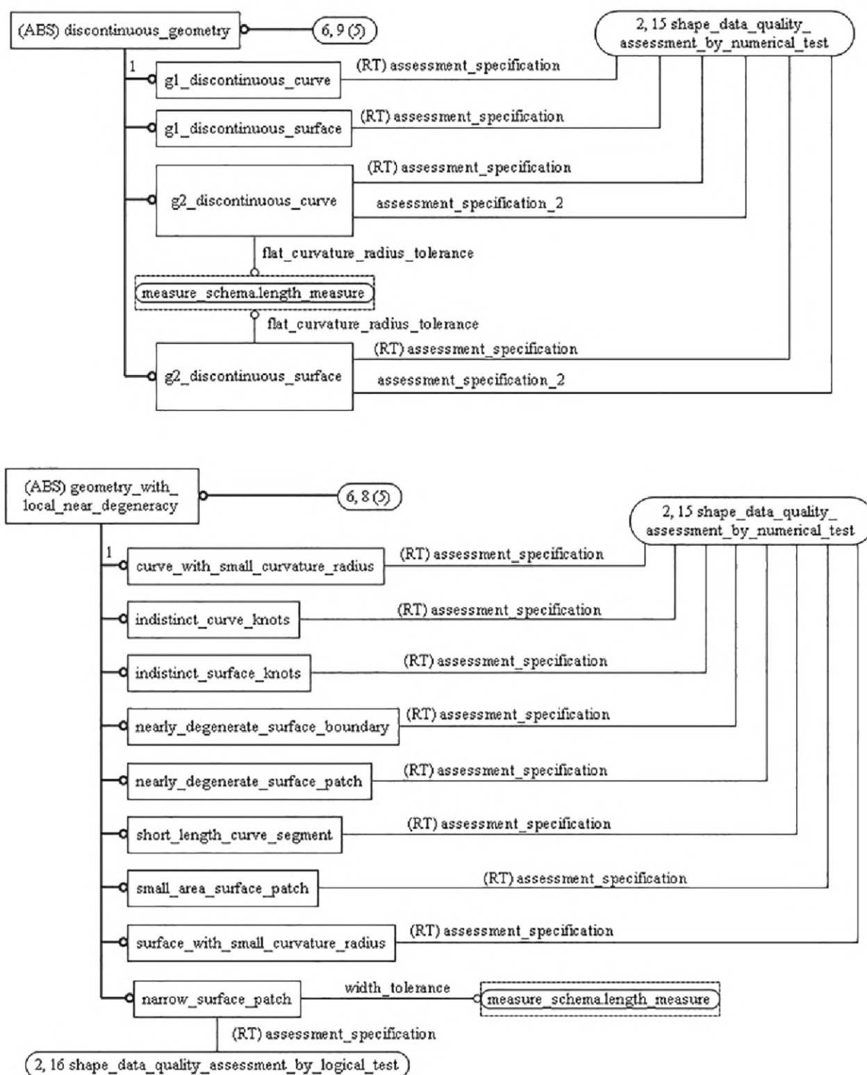
Рисунок D.12 — EXPRESS-G диаграмма схемы shape_data_quality_criteria_schema (диаграмма 6 из 9)
