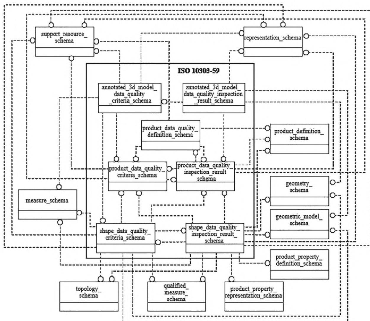
Рисунок 1 — Диаграмма уровня схем, показывающая отношения между схемами, специфицированными в настоящем стандарте (внутри прямоугольника), и другими схемами, относящимися к информационным ресурсам
