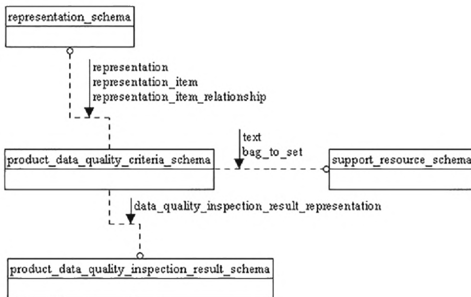
Рисунок D.3 — EXPRESS-G диаграмма схемы product_data_quality_criteria_schema (диаграмма 1 из 2)
