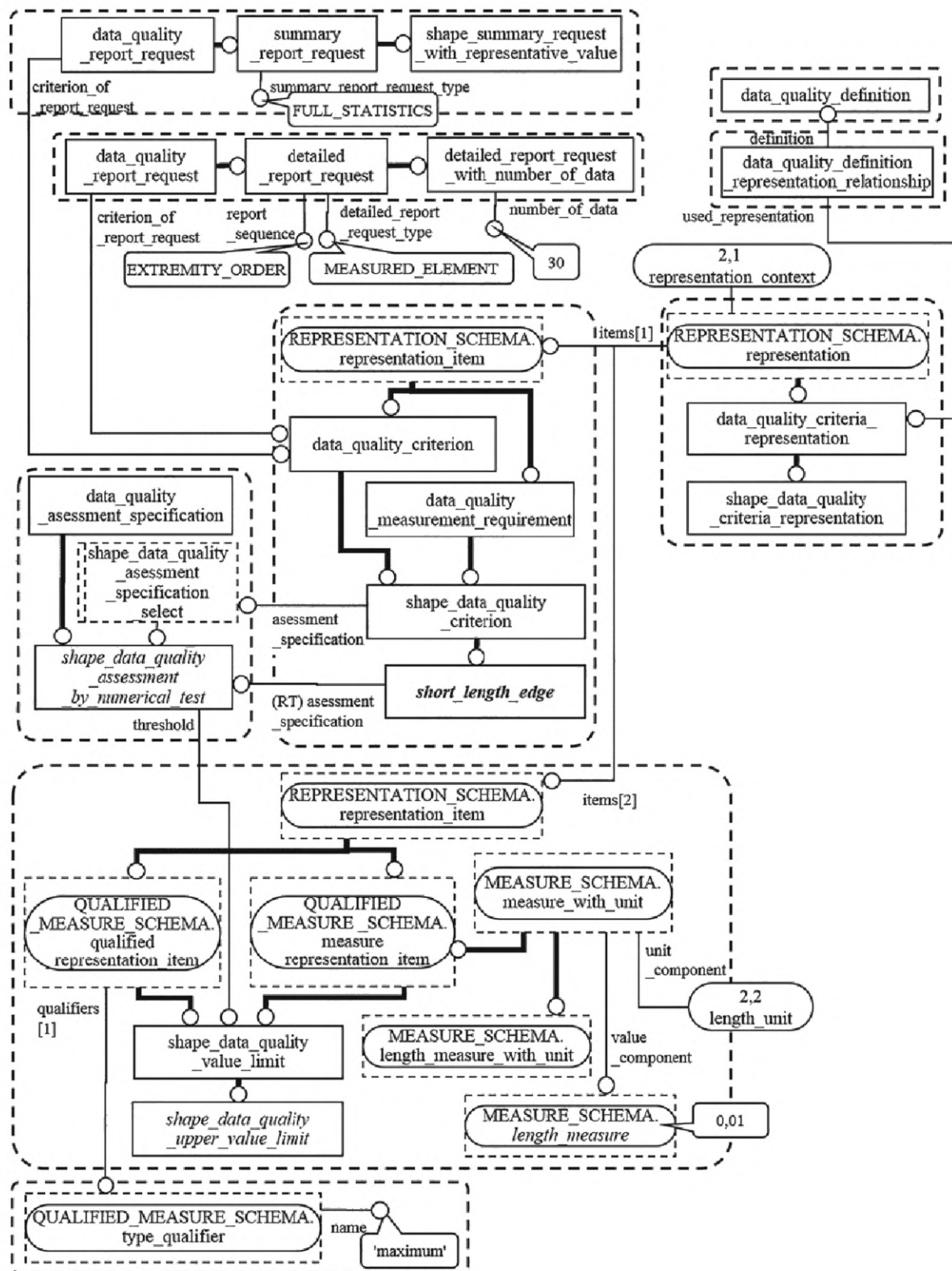
Рисунок F.3 — Пример экземпляров объектов, представляющих информацию о качестве, используемых для представления требований/заявления без задания точности (1 из 2)
