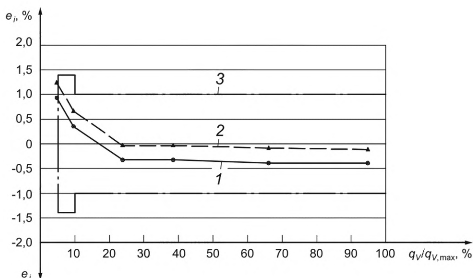
Рисунок В.1 — График результатов калибровки без корректировки (линия 1) и скорректированных на FWME (линия 2) для USM DN200 (линия 3 — предел допускаемой погрешности)
