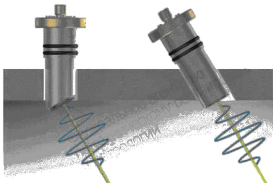
Рисунок 5 — Характерные схемы расположения ультразвуковых преобразователей
