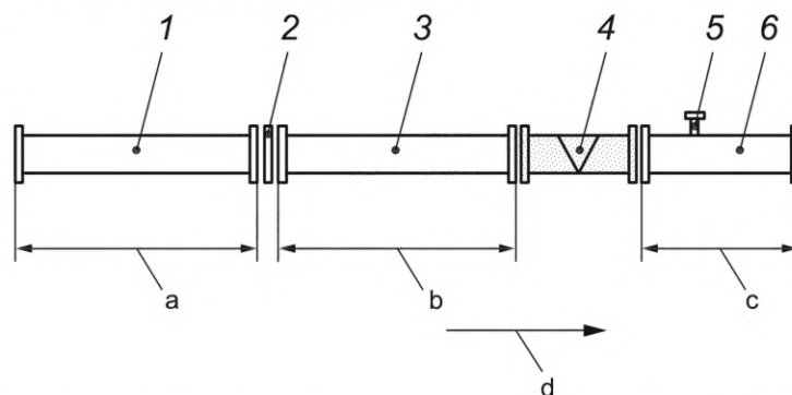
1 — входной трубопровод формирователя потока; 2 — формирователь потока (FC); 3 — входной трубопровод счетчика; 4 — ультразвуковой счетчик (USM); 5 — выходной трубопровод; 6 — датчик температуры (TS); а — длина участка не менее 2D (предпочтительно 3D); b — длина участка не менее XD (указывается изготовителем); c — расположение датчика температуры TS на расстоянии от 2D до 5D от выходного торца USM (длина выходного трубопровода от 3D до не менее 6D соответственно); d — основное направление потока (прямое)
