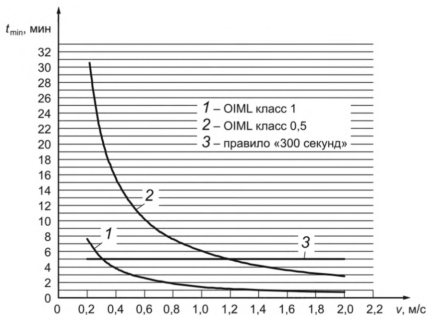
Рисунок D.4 — Минимальное время усреднения для счетчика DN800
