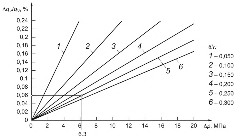
Рисунок 16 — Максимальная ожидаемая погрешность измерения расхода \Delta q_v/q_v , связанная с разностью давления \Delta p , для различных соотношений \delta/r
