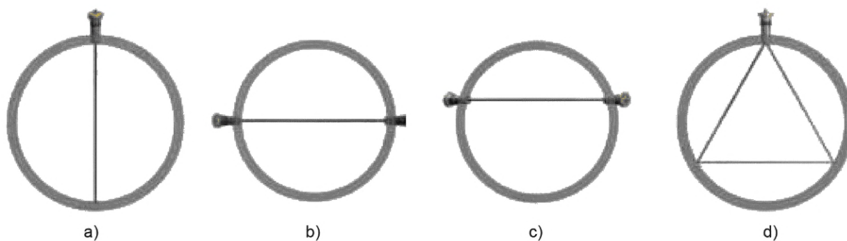
Рисунок 6 — Основные типы акустических траекторий для многолучевых счетчиков
