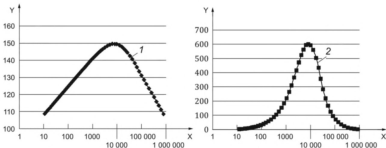
X — частота, Гц; Y — акустический уровень; 1 — L_{pi}(f) , дБ; 2 — P_i(f) , Па
