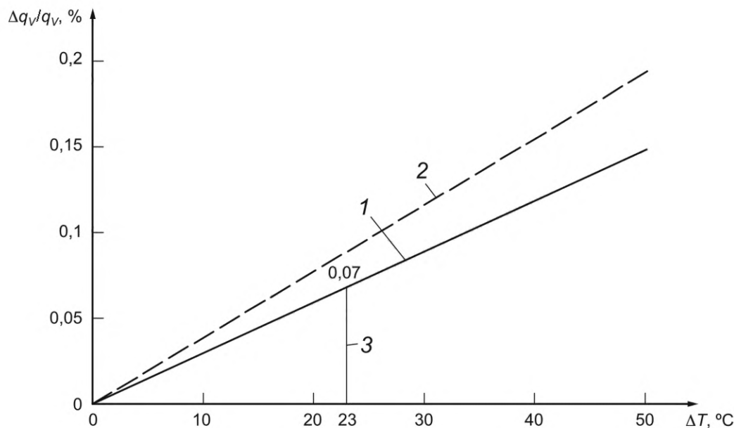
Рисунок 15 — Погрешность измерения расхода \Delta q_V/q_V , связанная с разницей температур \Delta T , для двух видов материала
