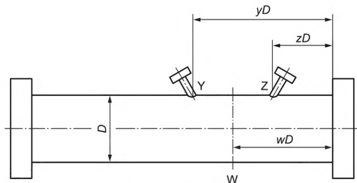
Рисунок Е.1 — Места установки ультразвуковых преобразователей относительно фланцев
