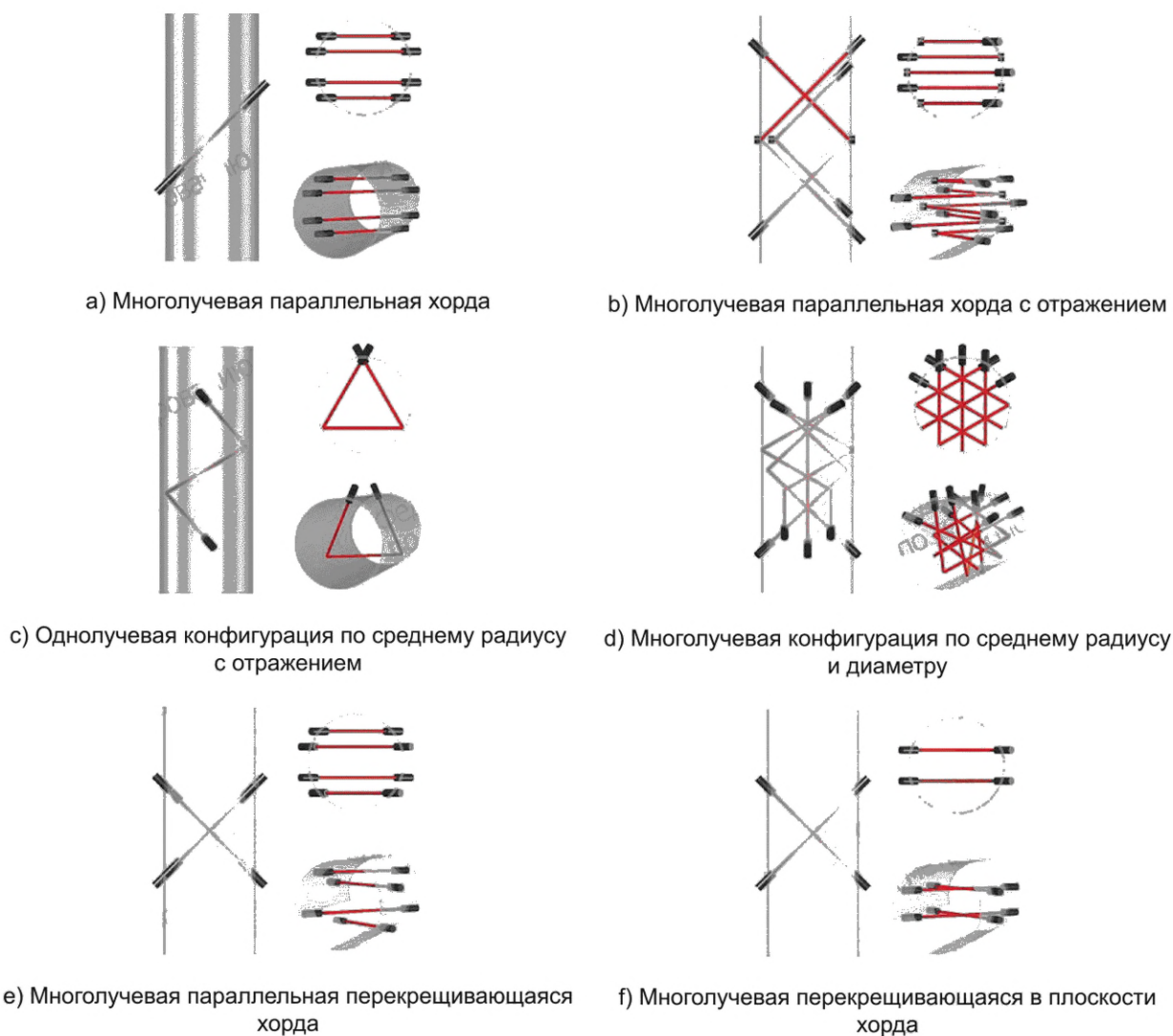
Рисунок 7 — Варианты часто встречающихся конфигураций расположения акустических траекторий
