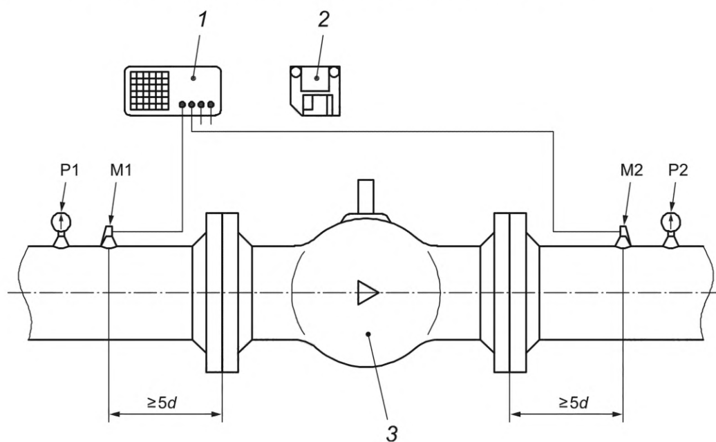
1 — осциллограф; 2 — запоминающее устройство для записи бинарных данных; 3 — регулирующий клапан; M1, M2 — микрофоны; P1, P2 — датчики давления; d — внутренний диаметр трубопровода
