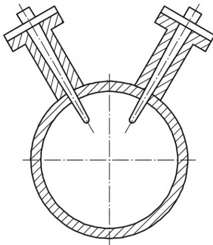
Рисунок 9 — Гильзы термометров расположены не на одной линии с акустическими траекториями
