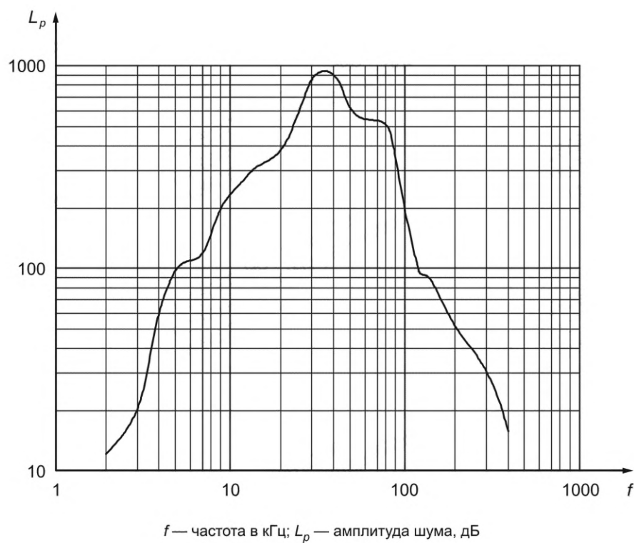
Рисунок С.1 — Характерный спектр акустического шума, генерируемого клапаном
