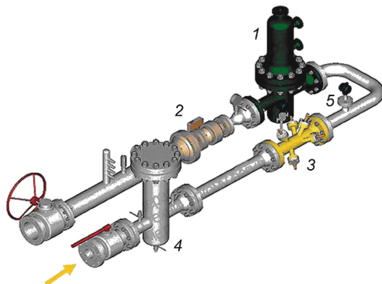
1 — теплообменник; 2 — регулирующий клапан; 3 — УСМ; 4 — фильтр; 5 — гильза термометра
