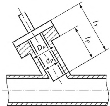
Рисунок Е.3 — Размеры монтажного канала ультразвукового преобразователя
