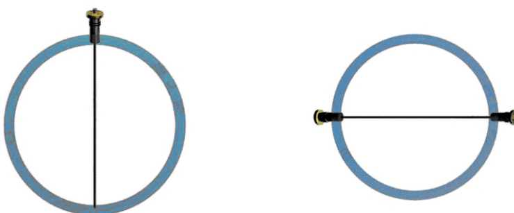
Рисунок 2 — Диаметральные траектории акустического сигнала
