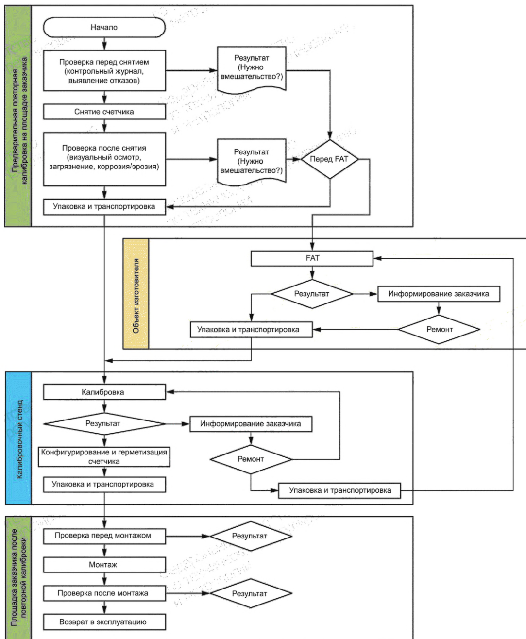
Рисунок 13 — Процесс повторной калибровки
