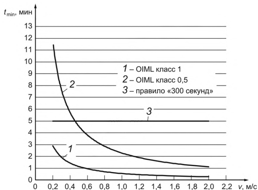
Рисунок D.3 — Минимальное время усреднения для счетчика DN300
