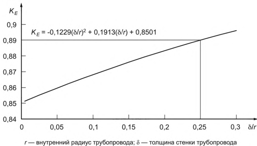
Рисунок 17 — Поправочный коэффициент торцевой нагрузки и крепления K_E
