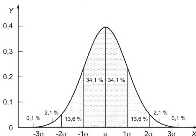
Рисунок D.2 — Распределение вероятностей Гаусса
