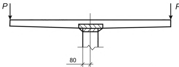
Рисунок В.2 — Схема испытания ступеней типоразмеров ЛСС 12 и ЛСС 15
