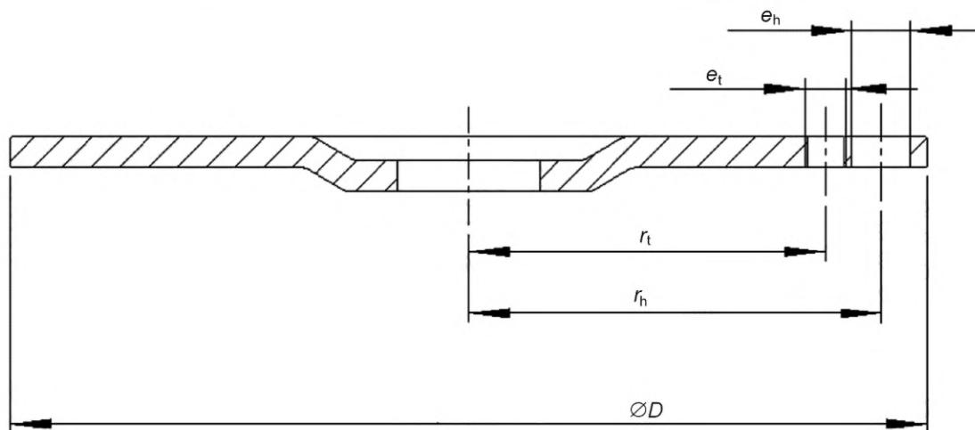
Рисунок С.4 — Размеры отверстий для альтернативного варианта круга типа 27
