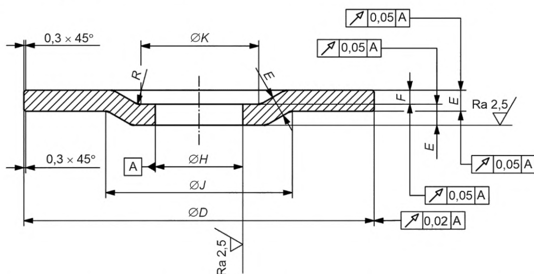
Рисунок С.1 — Геометрические размеры и допуски на изготовление для испытательных кругов типа 27
