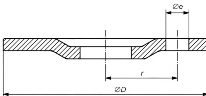
Рисунок С.3 — Размеры отверстий для создания неуравновешенности испытательных кругов типа 27
