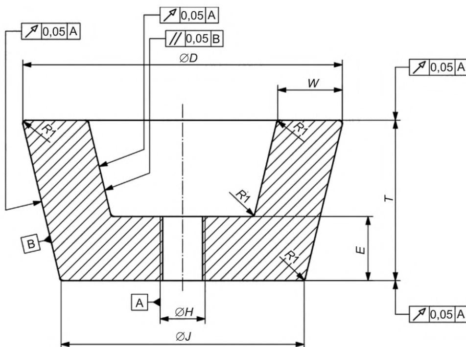
Рисунок С.2 — Геометрические размеры и допуски на изготовление для испытательных кругов типа 11
