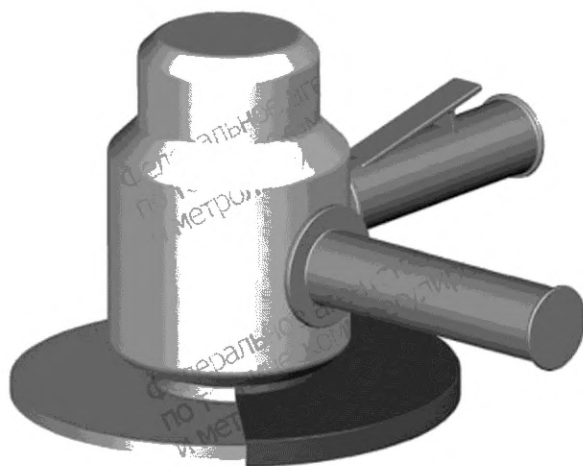
Рисунок 5 — Пневматическая вертикальная шлифовальная машина
