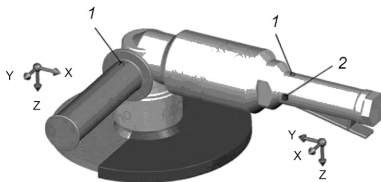
Рисунок 10 — Точки и направления измерений для пневматической угловой шлифовальной машины с обособленной основной рукояткой
