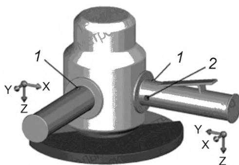
Рисунок 11 — Точки и направления измерений для пневматической вертикальной шлифовальной машины
