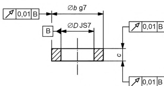
Рисунок С.6 — Геометрические размеры и допуски на изготовление промежуточной втулки для испытательных кругов типа 27
