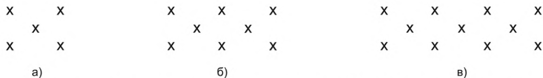
Рисунок 1 — Схемы отбора точечных образцов от партии или с площади методом одиночного, двойного или тройного «конверта»
