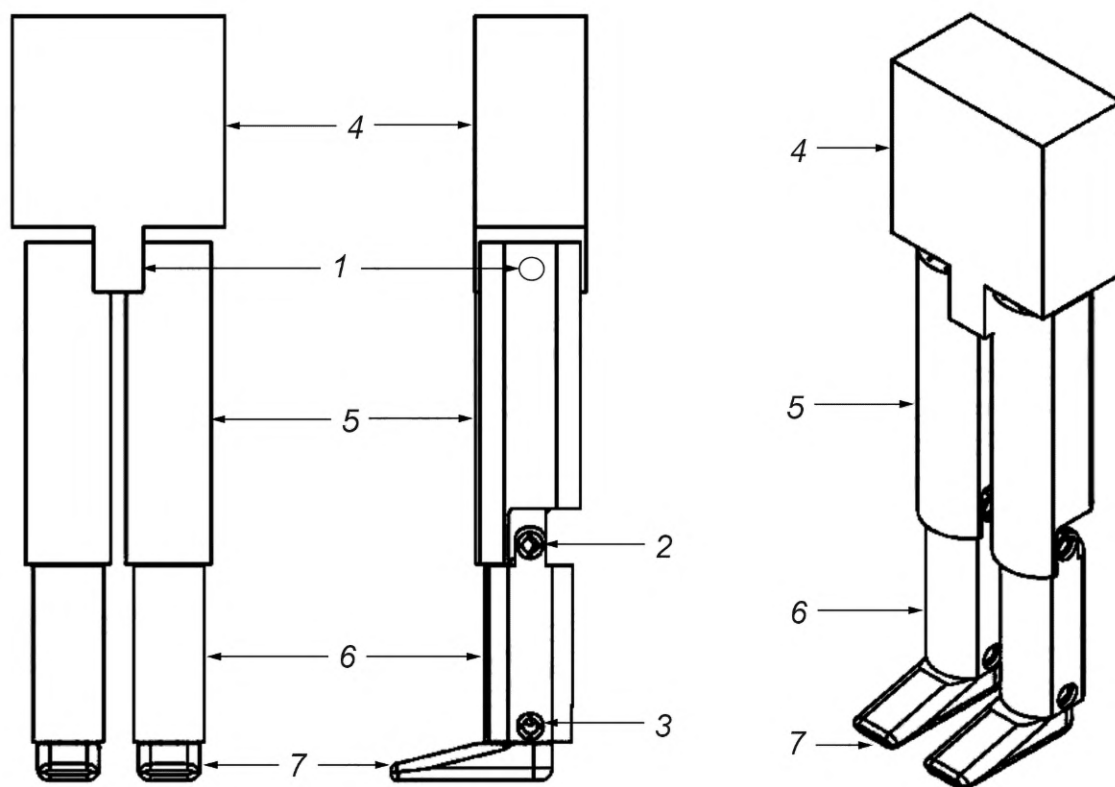
1 — тазобедренный шарнир; 2 — коленный шарнир; 3 — голеностопный шарнир; 4 — таз и верхняя часть туловища; 5 — бедро; 6 — голень; 7 — ступня
