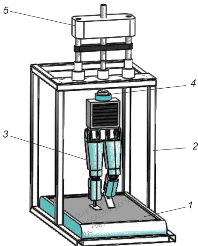
1 — беговая дорожка; 2 — каркас испытательного оборудования; 3 — тестовый манекен; 4 — датчик усилия; 5 — исполнительный модуль
