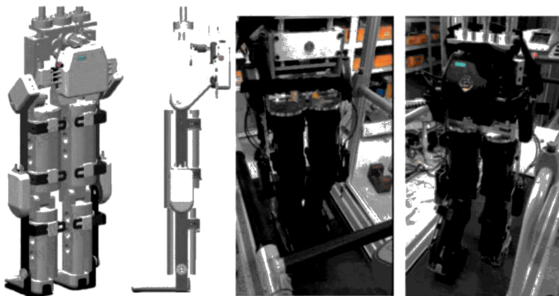
Рисунок 4 — Пример реализации испытательного стенда
