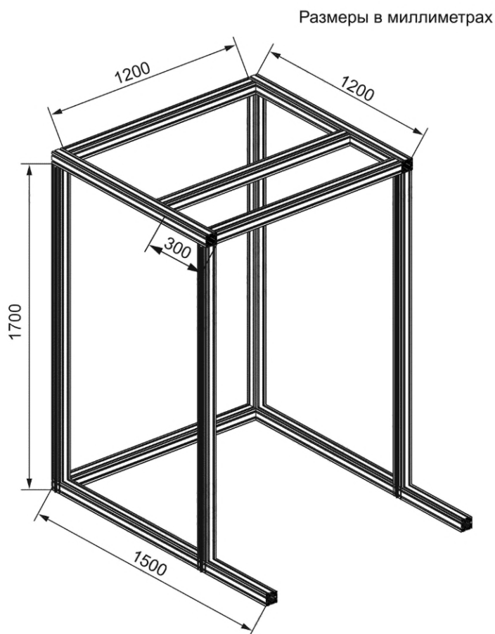
Рисунок 3 — Пример конструкции и размеров каркаса испытательного оборудования
