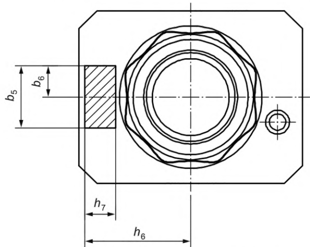
Рисунок Е.1 — Расположение и размеры области для передачи энергии и данных
