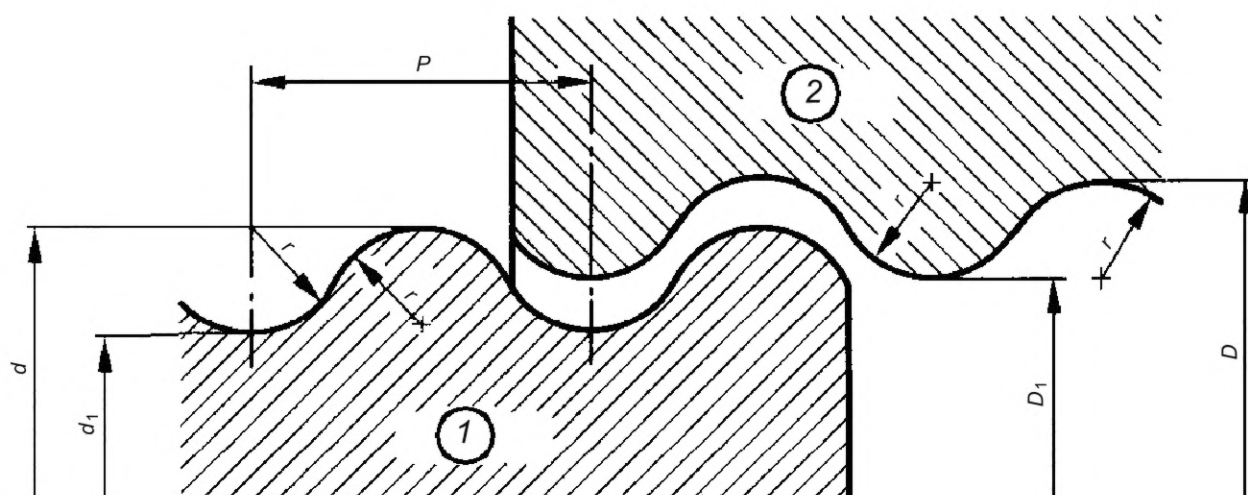
1 — болт; 2 — гайка
