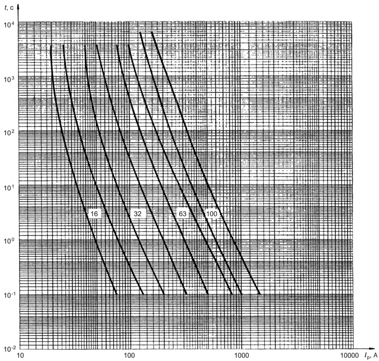
Рисунок 305 — Зоны времятоковых характеристик для плавких вставок «gG»
