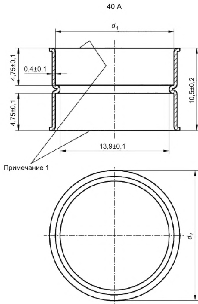
Калибровочная втулка 40 А
