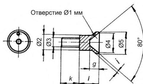
Втулка
