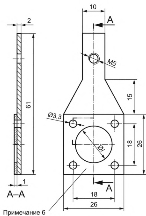
Типоразмеры D01...D03, DII и DIII
