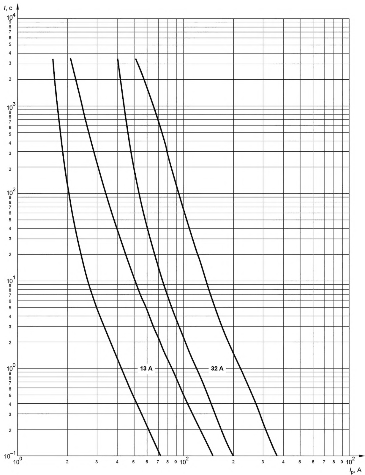
Рисунок 103 — Зоны времятоковых характеристик для плавких вставок «gG» для номинальных токов 13 и 32 А
