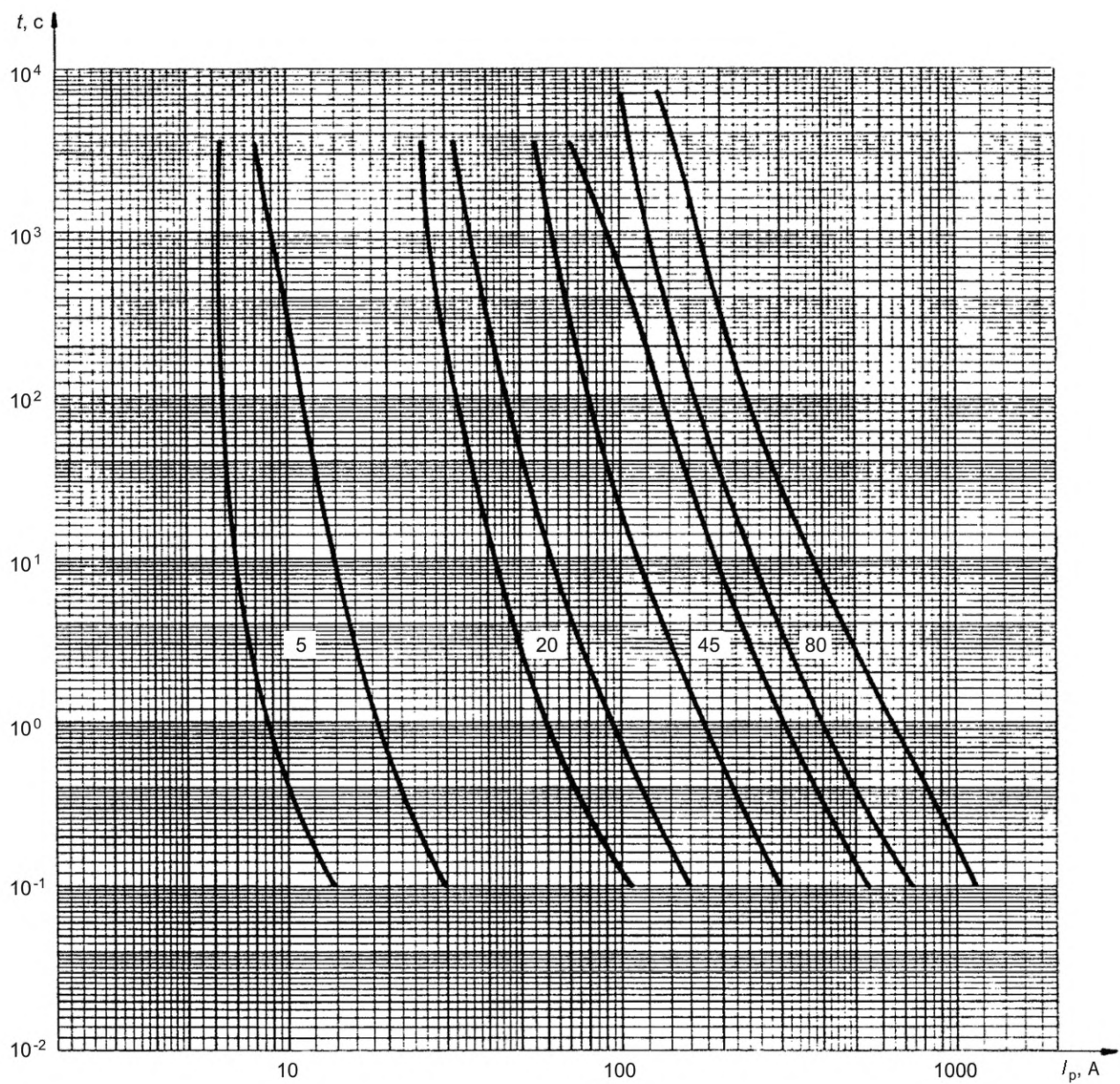
Рисунок 304 — Зоны времятоковых характеристик для плавких вставок «gG»
