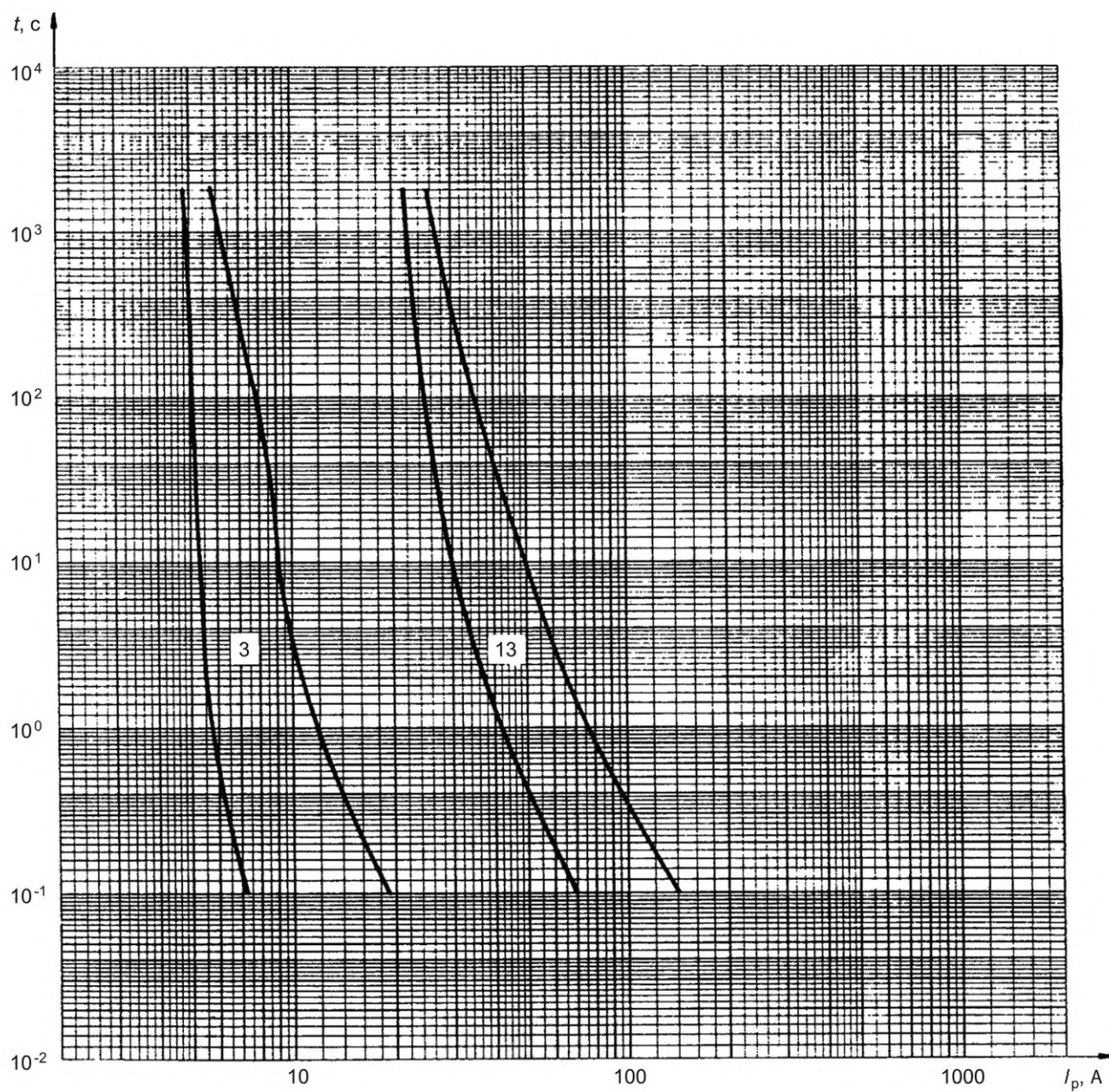
Рисунок 602 — Зоны времятоковых характеристик для плавких вставок «gG»
