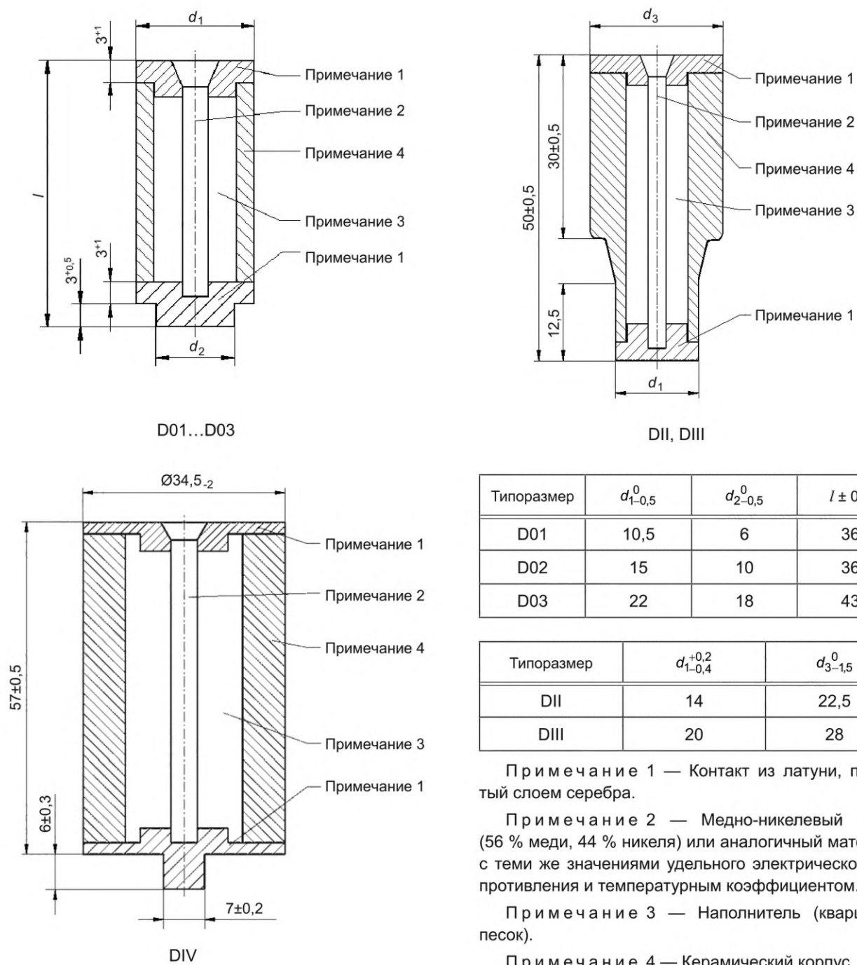
Рисунок 104 — Макетные плавкие вставки в соответствии с 8.3 и 8.9.1.1
