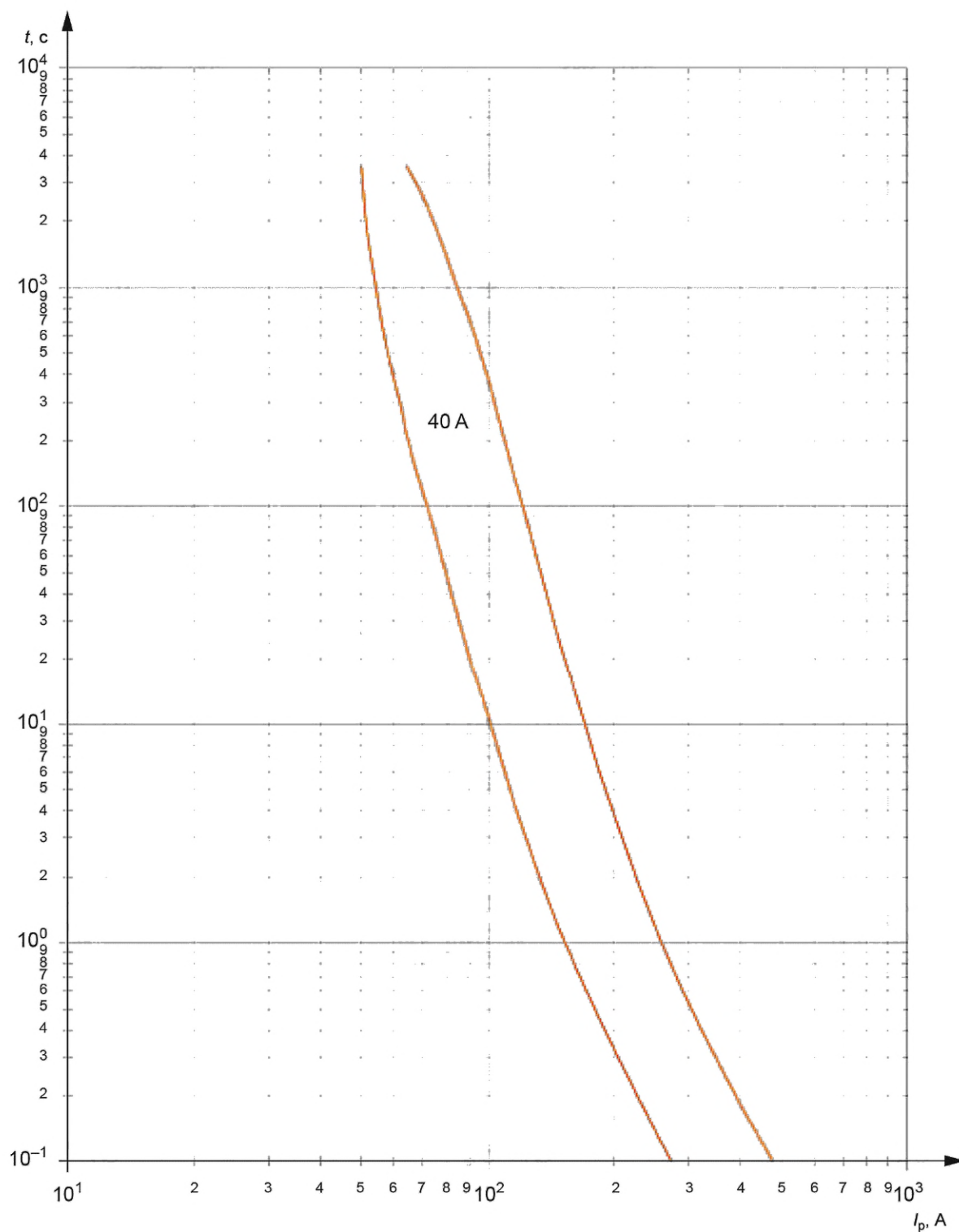
Рисунок 127 — Зоны времятоковых характеристик для плавких вставок «gG» для номинального тока 40 А
