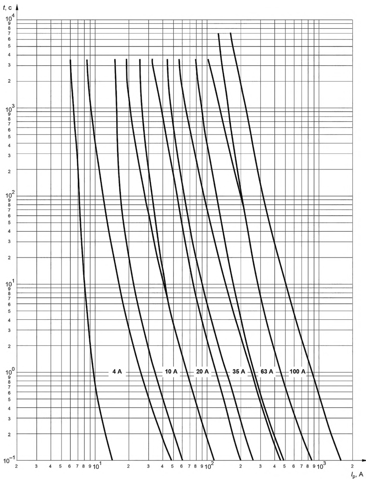
Рисунок 102 — Зоны времятоковых характеристик для плавких вставок «gG»
