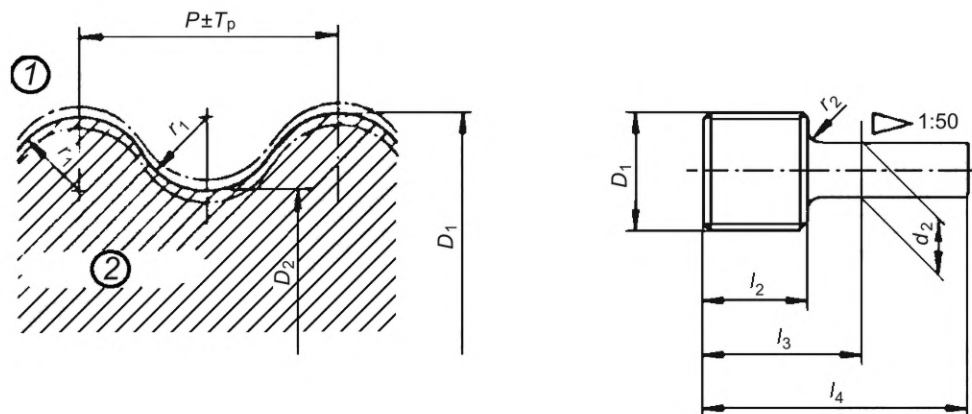
1 — профиль резьбы; 2 — калибр-пробка
