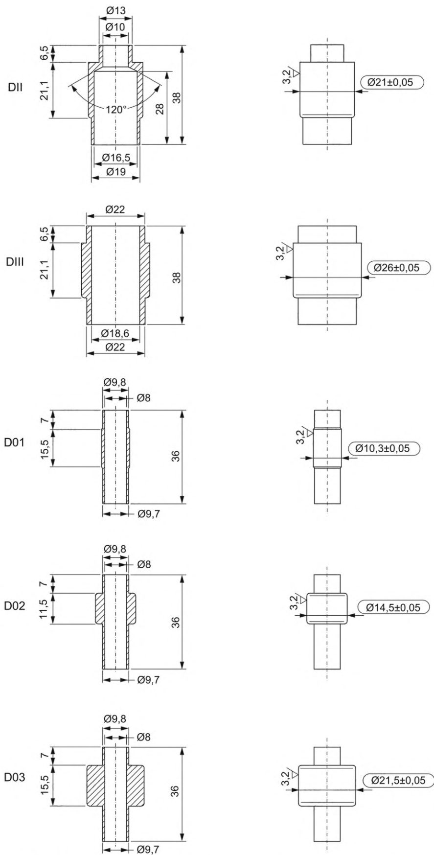
Рисунок 126 — Испытательные калибровочные втулки типоразмеров DII, DIII, D01, D02 и D03 для испытания держателей плавких вставок
