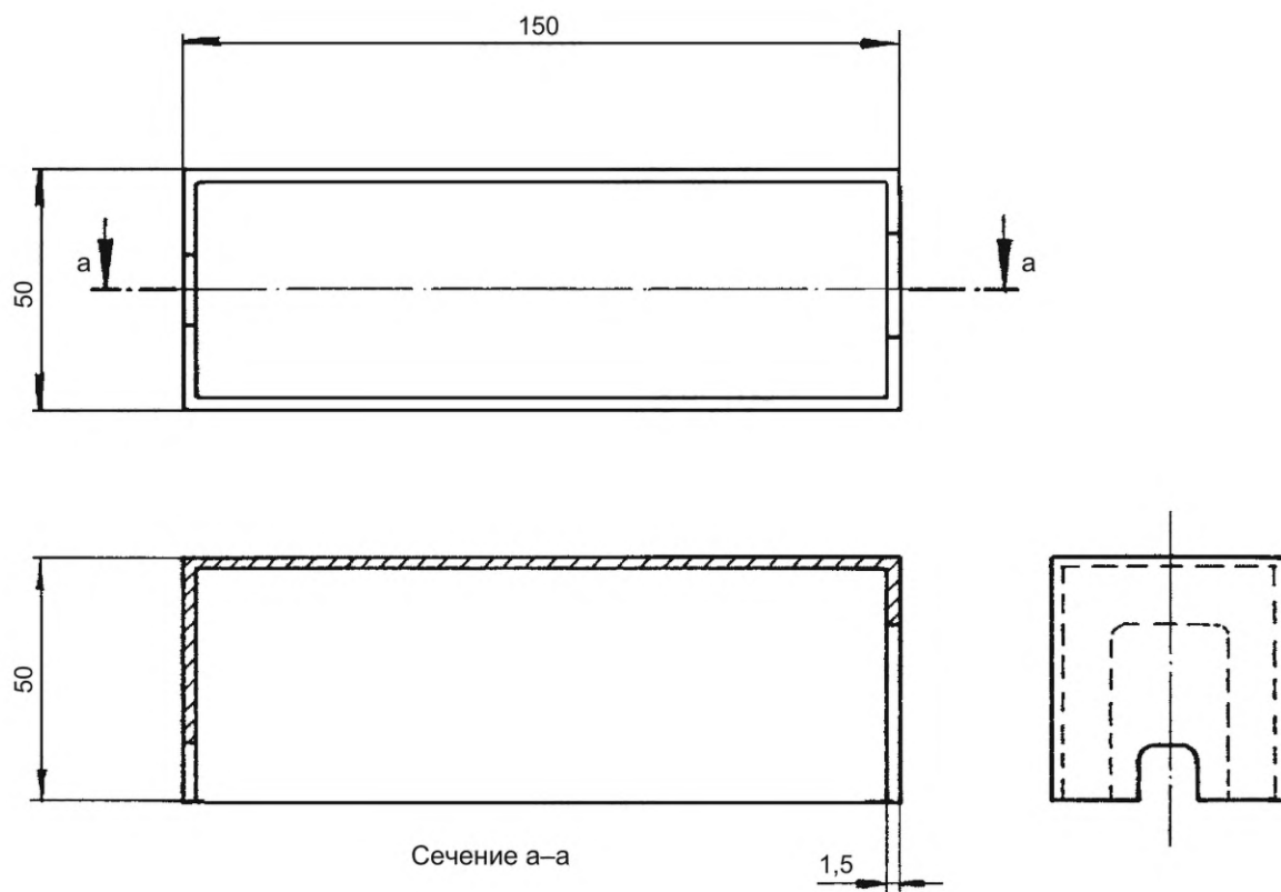
Рисунок 205 — Кожух для проверки срабатывания плавких вставок с испытательным стендом по рисунку 203
