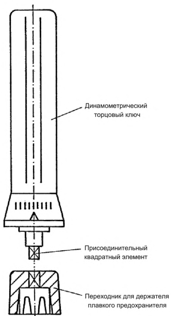
Рисунок 108 — Пример динамометрического торцового ключа в соответствии с 8.9.2
