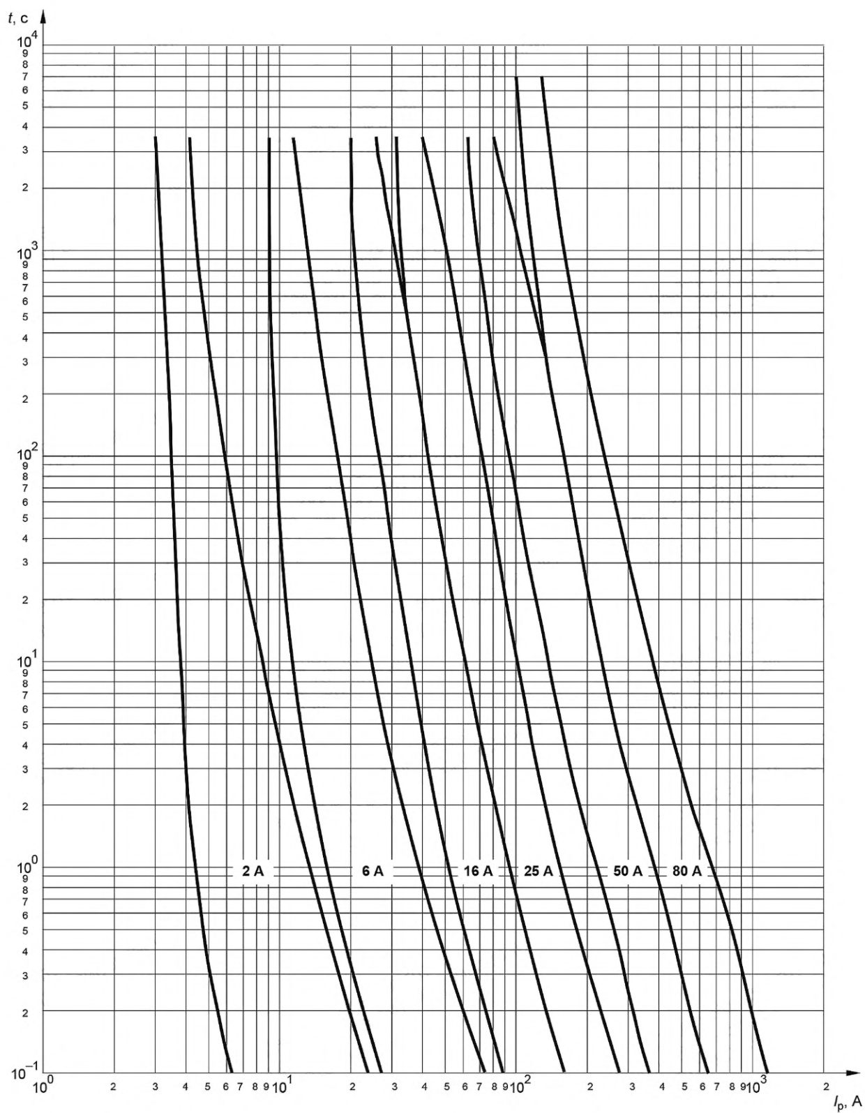
Рисунок 101 — Зоны времятоковых характеристик для плавких вставок «gG»
