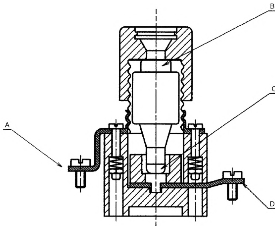
Рисунок 109 — Точки измерения для серии плавких предохранителей А в соответствии с 8.3.3, 8.3.4.1 и 8.10.2
