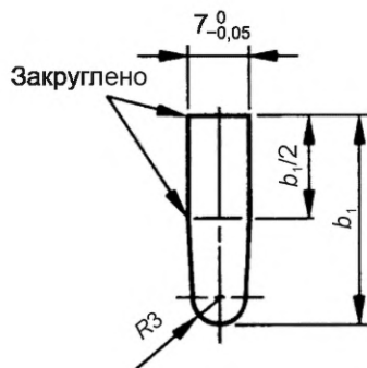
Рисунок 107 — Испытательный нож согласно 8.5.5.1.2
