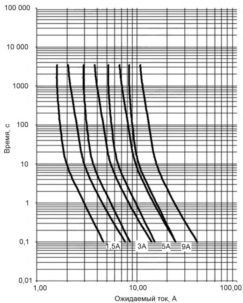
Рисунок 1005 — Зоны времятоковых характеристик для предохранителей gN класса CC
