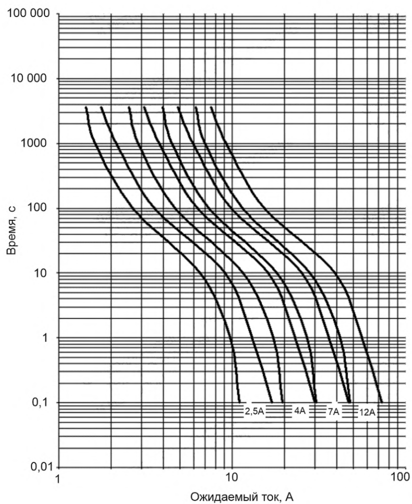
Рисунок 1010 — Зоны времятоковых характеристик для предохранителей gD класса CC
