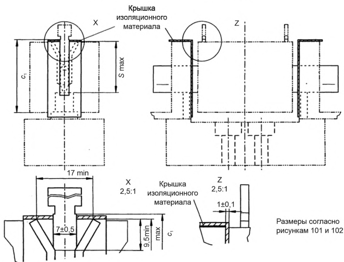
Рисунок 110 — Точки измерения согласно 8.10.2
