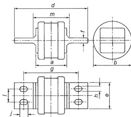
Плавкая вставка, типоразмер D
