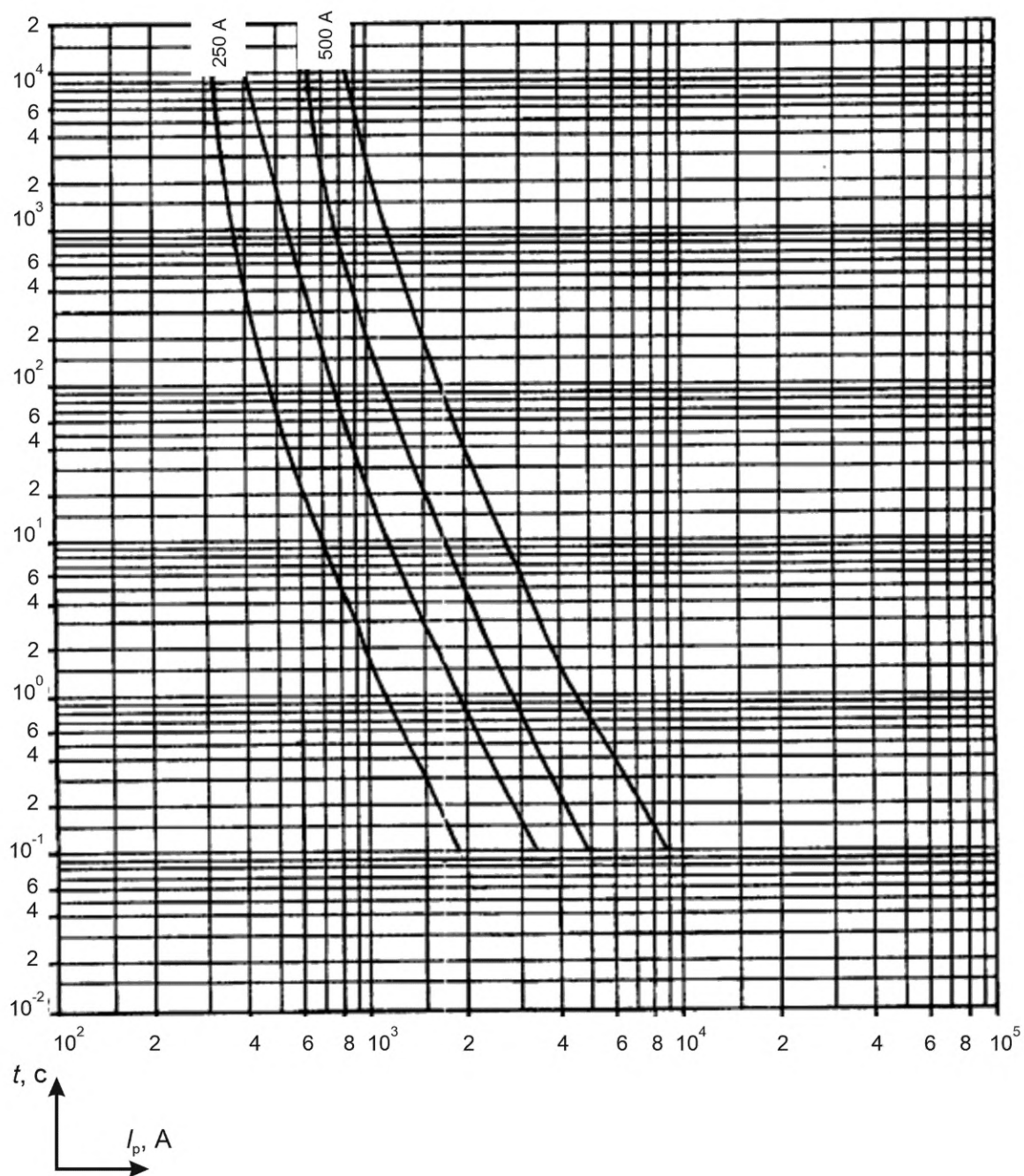
Рисунок 903 — Зоны времятоковых характеристик для номинальных токов 250 А и 500 А
