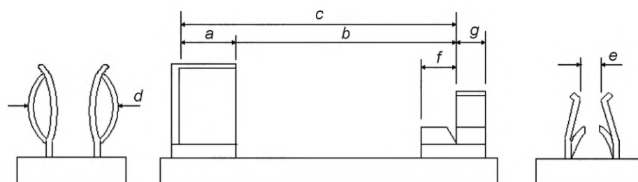
Рисунок 1001 — Плавкие вставки класс CC (1—30 А)
