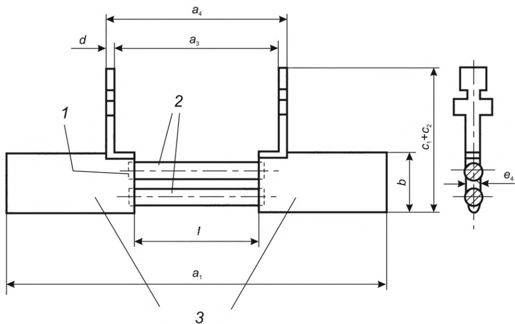
1 — пайка; 2 — CuMn12Ni; 3 — посеребренный медный сплав
