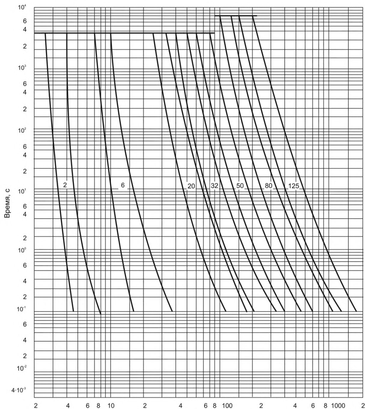
Рисунок 704 — Зоны времятоковых характеристик для плавких вставок gG
