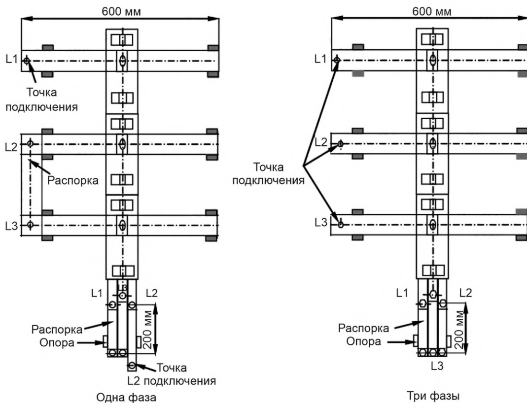
Чертеж групп В и С
