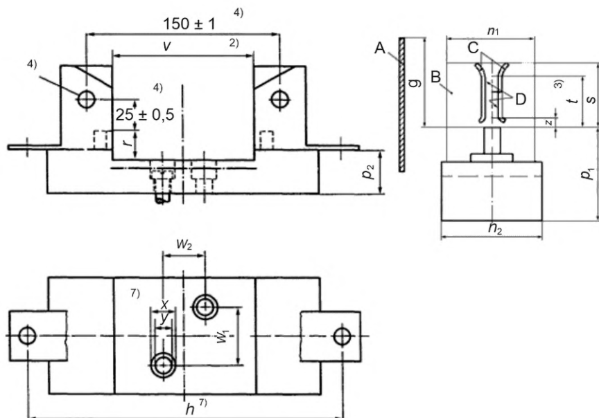
Рисунок 102 — Основания для плавких вставок с ножевыми контактами
