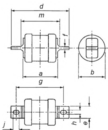
Плавкая вставка, типоразмер В
