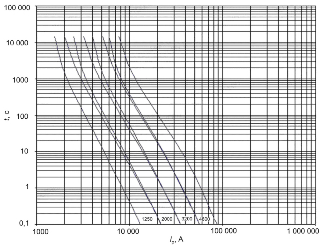
Рисунок 1104 — Зоны времятоковых характеристик для плавких вставок gK серии предохранителей К (1 из 2)
