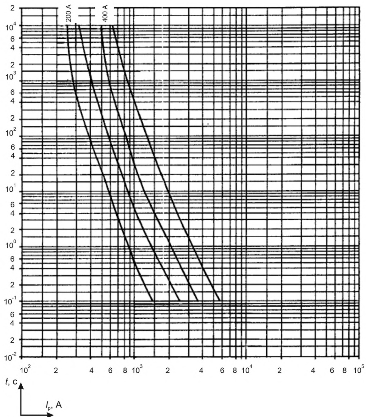
Рисунок 904 — Зоны времятоковых характеристик для номинальных токов 200 и 400 А
