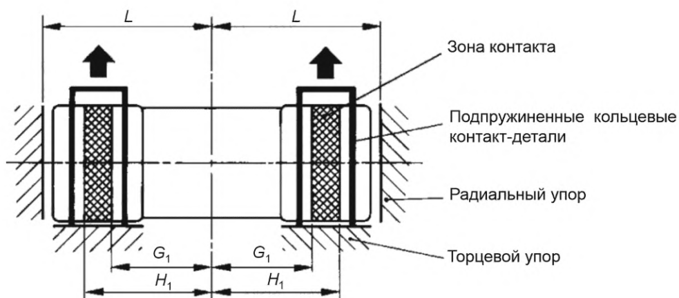
Основание А. Контакт на двух цилиндрических головках
