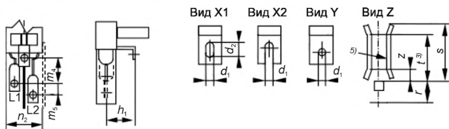
Рисунок 301 — Планочные предохранители для плавких вставок с ножевыми контактами (1 из 3)
