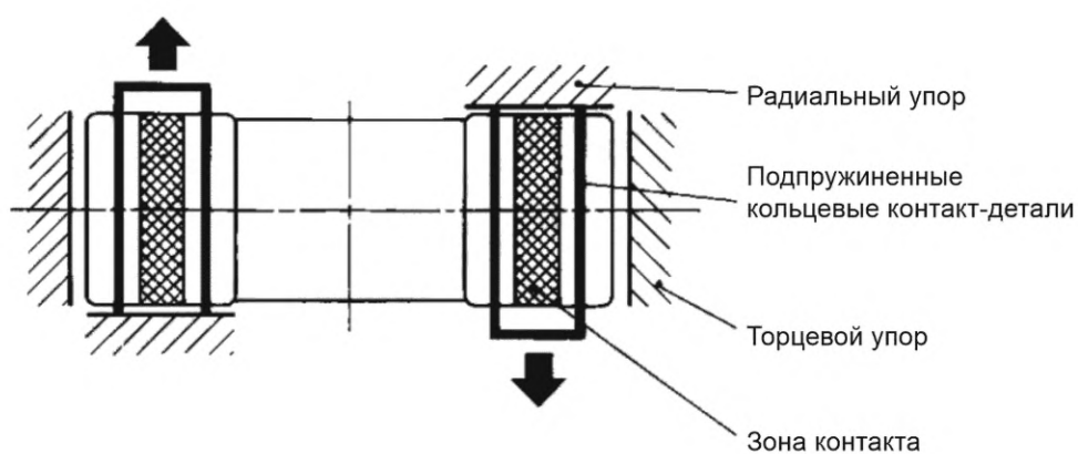
Основание В. Контакт на двух цилиндрических головках
