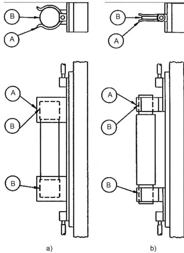
Рисунок 807 — Конструкция стенда для испытаний на нагрев
