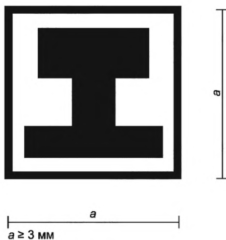
Рисунок 112 — Маркировочный знак для изолированных креплений
