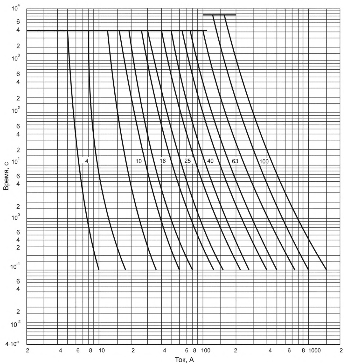
Рисунок 703 — Зоны времятоковых характеристик для плавких вставок gG
