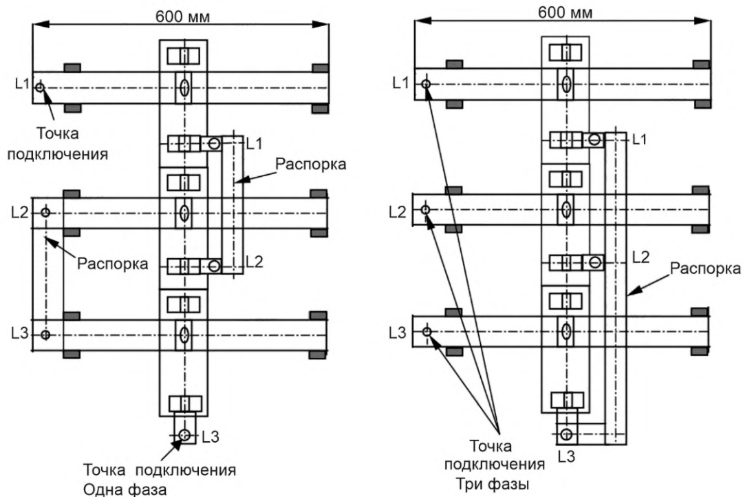
Чертеж группы А
