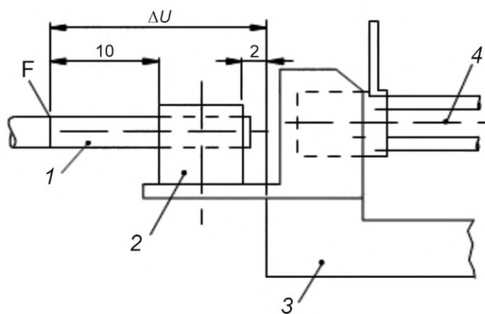
Рисунок 110 — Точки измерения согласно 8.10.2
