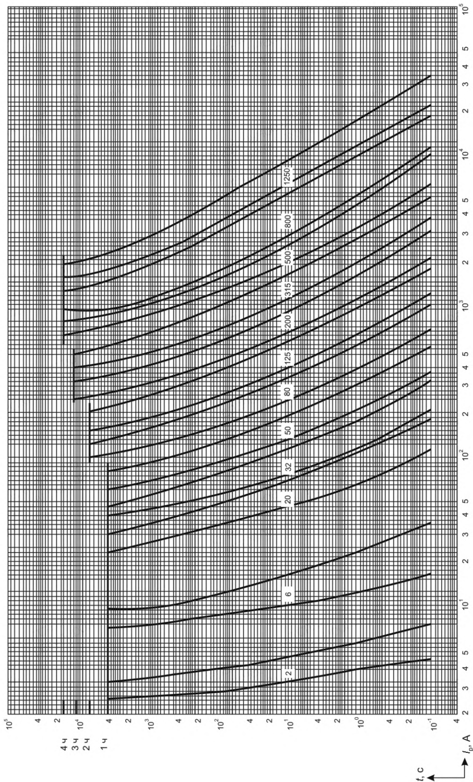
Рисунок 503 — Зоны времятоковых характеристик для плавких вставок gG
