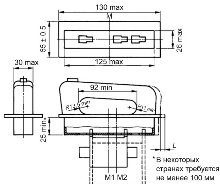
Рисунок 102 — Основания для плавких вставок с ножевыми контактами
