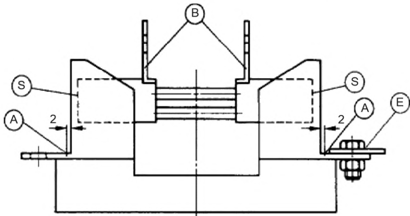
Рисунок 106 — Точки замеров согласно IEC 60269-1, 8.3.4 и серия A: 8.3.4.1, 8.3.4.2 и 8.10.2
