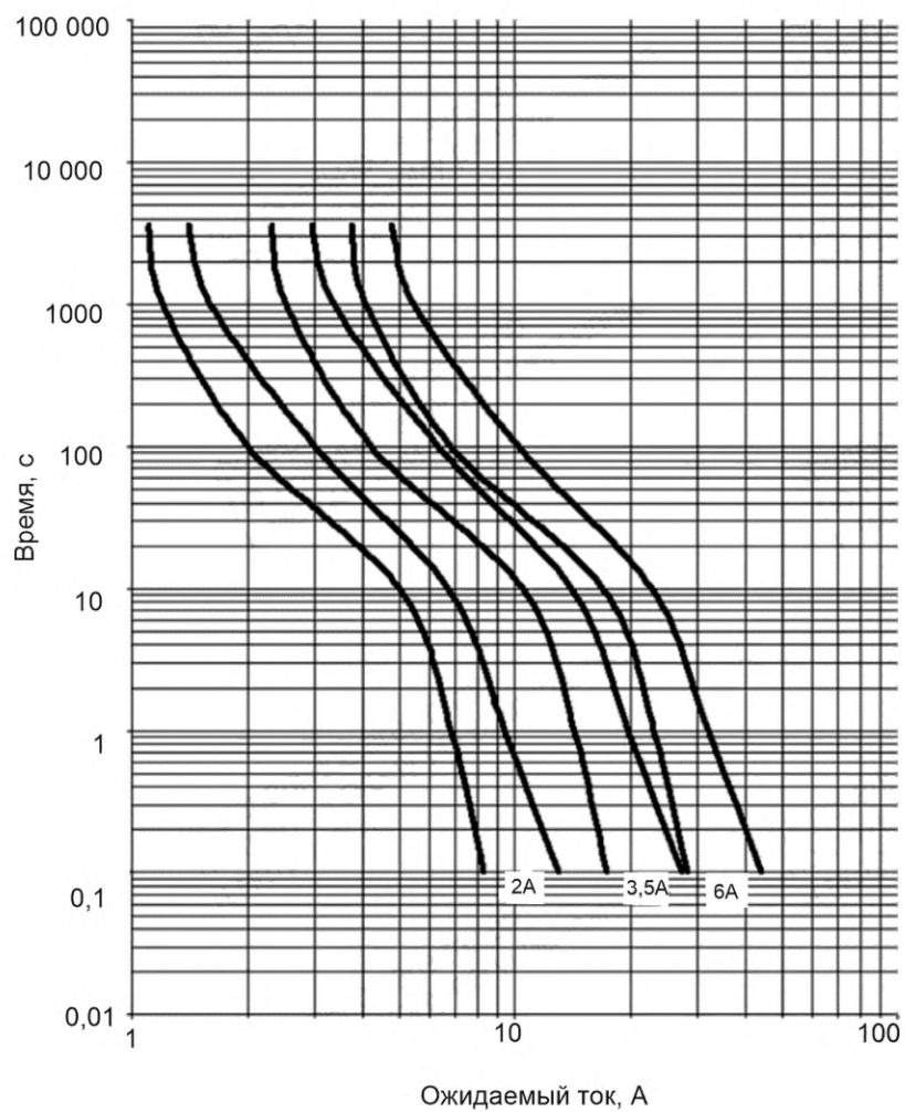
Рисунок 1008 — Зоны времятоковых характеристик для предохранителей gD класса CC
