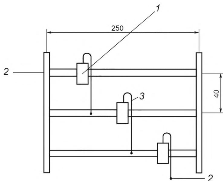
Рисунок 404 — Испытательный стенд для однополюсных и трехполюсных оснований для монтажа на систему шин в соответствии с 8.3.1
