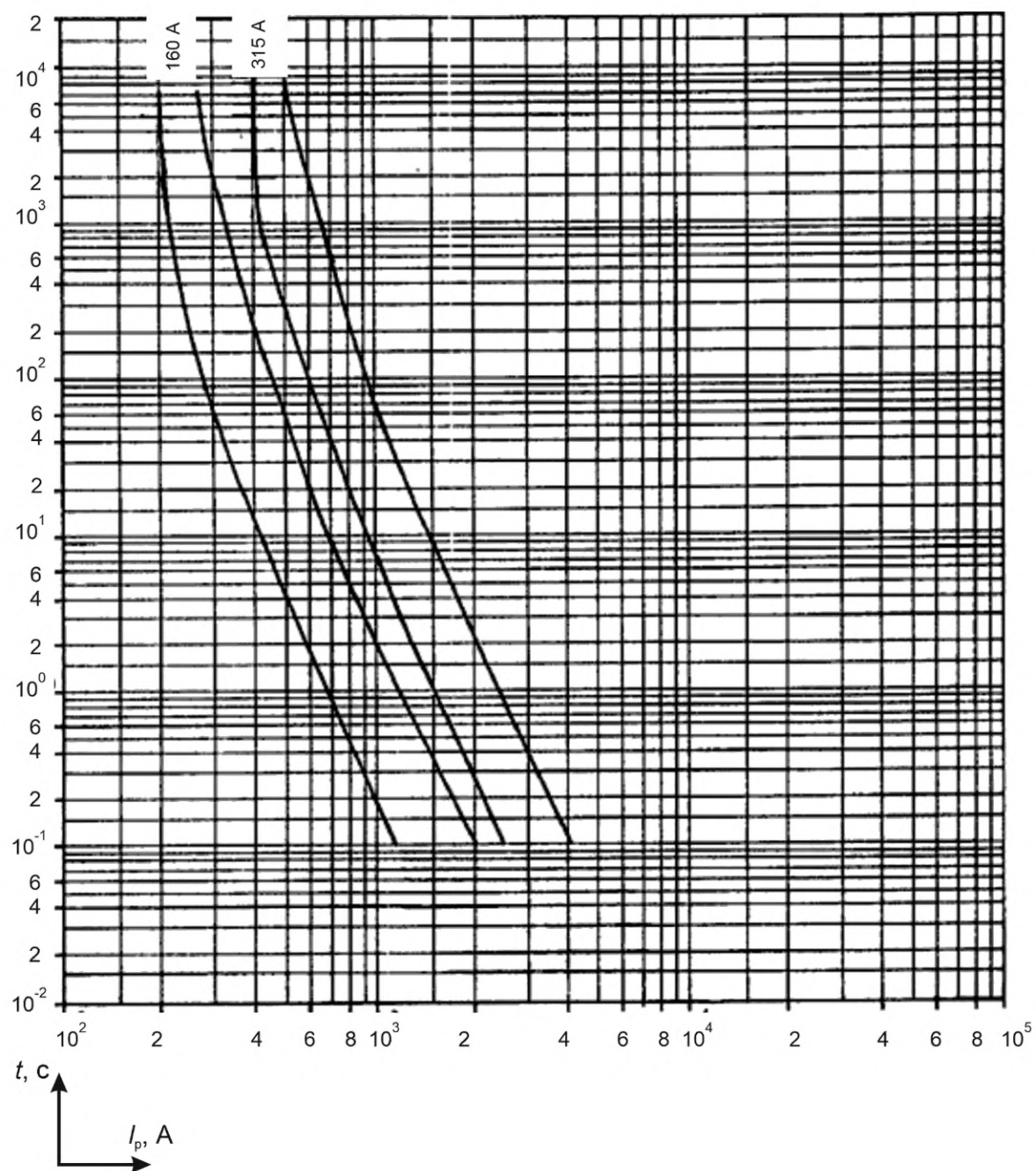
Рисунок 902 — Зоны времятоковых характеристик для номинальных токов 160 и 315 А
