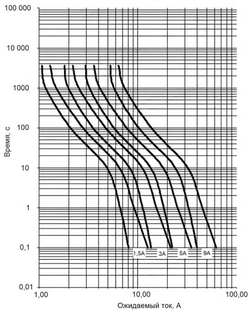
Рисунок 1009 — Зоны времятоковых характеристик для предохранителей gD класса CC
