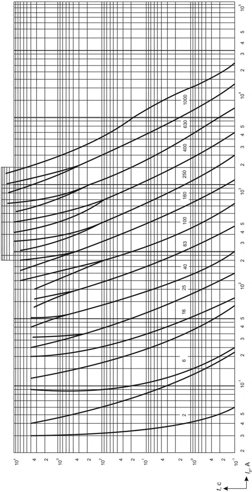
Рисунки 104 — Зоны времятоковых характеристик для плавких вставок gG (1 из 5)
