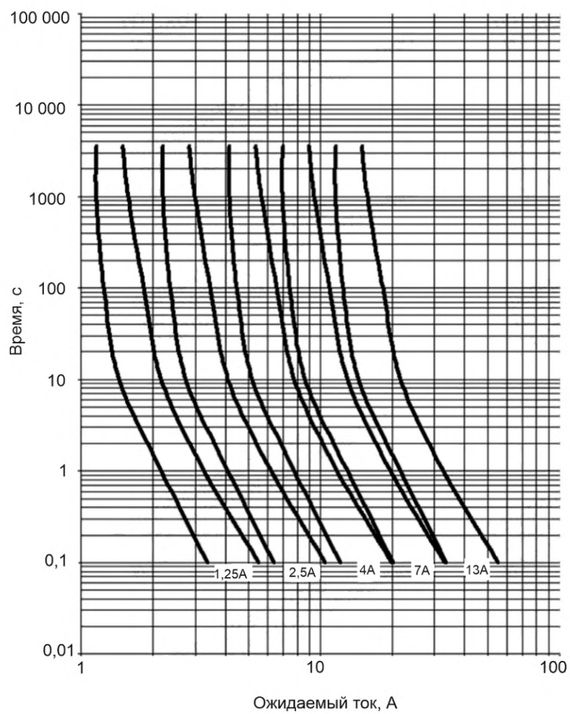
Рисунок 1006 — Зоны времятоковых характеристик для предохранителей gN класса CC
