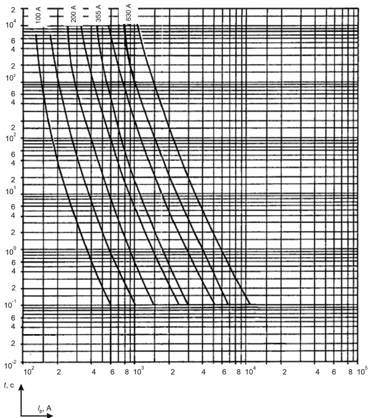
Рисунок 901 — Зоны времятоковых характеристик для номинальных токов 100, 200, 355 и 630 А
