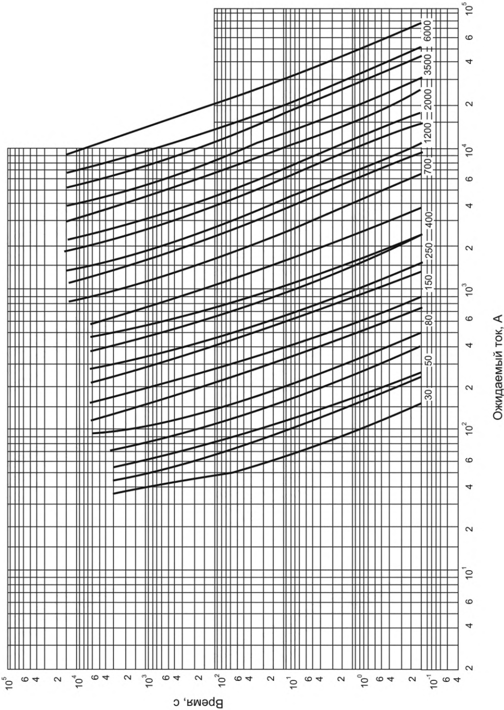
Рисунок 810 — Зоны времятоковых характеристик для плавких вставок gN
