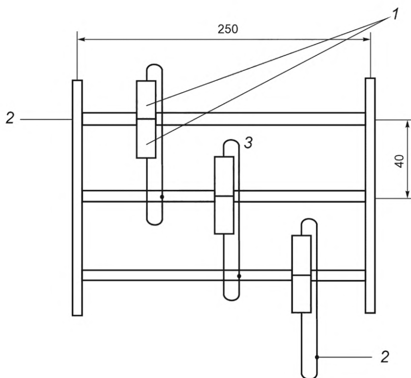
Рисунок 404 — Испытательный стенд для однополюсных и трехполюсных оснований для монтажа на систему шин в соответствии с 8.3.1
