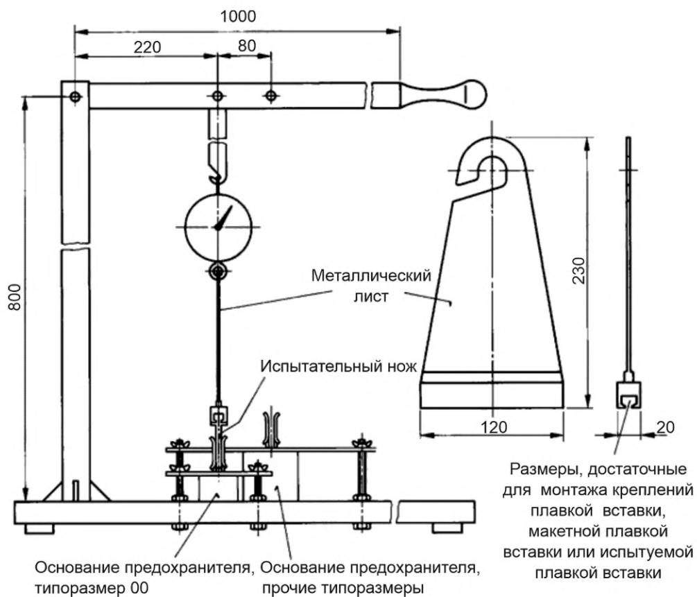
Рисунок 107 — Испытательный нож согласно 8.5.5.1.2
