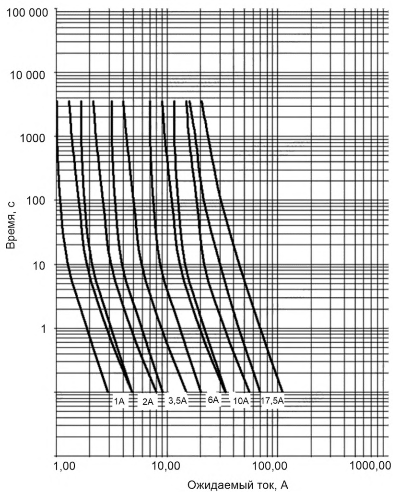
Рисунок 1007 — Зоны времятоковых характеристик для предохранителей gN класса CC
