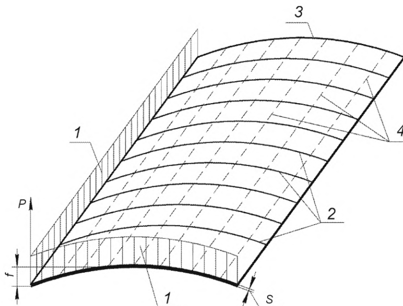
1 — эпюры изменения усилия раскатки P ; 2 — линии прокатки; 3 — короткая кромка листовой заготовки; 4 — образующие поверхности (линиигиба); P — усилие раскатки; f — стрелка погиба листа; S — толщина листа
