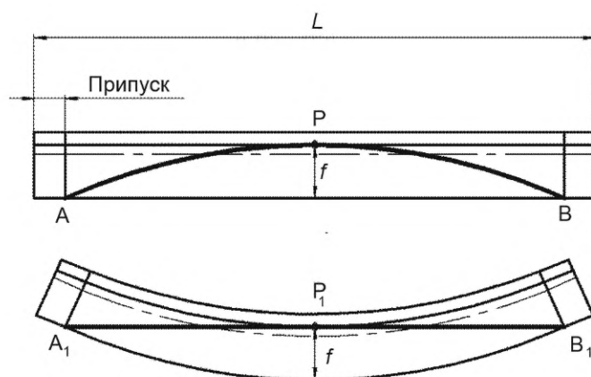
а — деталь с изгибом бульбой внутрь и одной спрямляемой кривой
