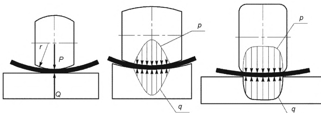
r — поперечный радиус ролика; P — сосредоточенное усилие гибки; p — распределенное усилие гибки; Q, q — сосредоточенные и распределенные реакции опор соответственно
