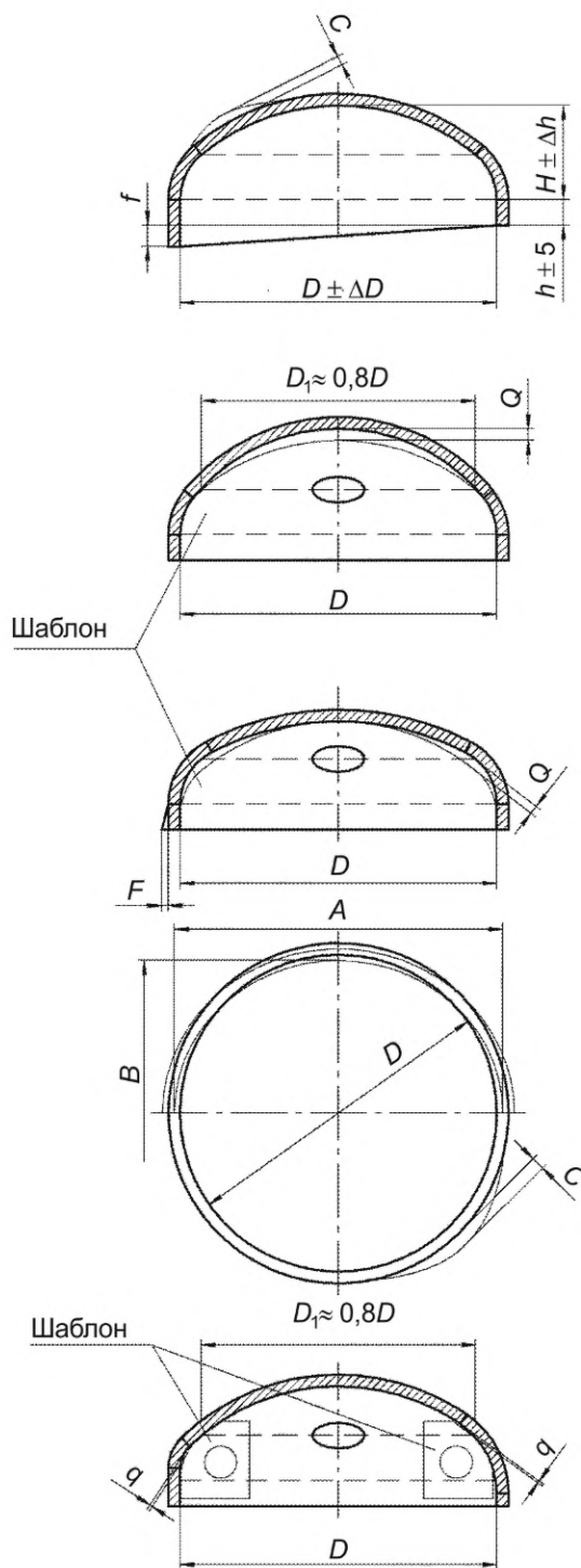
Рисунок 44 — Схемы отклонения размеров цельноштампованных днищ
