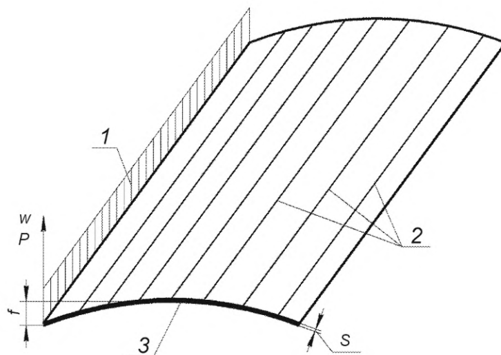
1 — эпюра изменения прогиба листа под роликом w или усилия гибки P ; 2 — линиигиба; 3 — короткая кромка листовой заготовки; w — прогиб листа под роликом; P — усилие гибки; f — стрелка погиба листа; S — толщина листа
