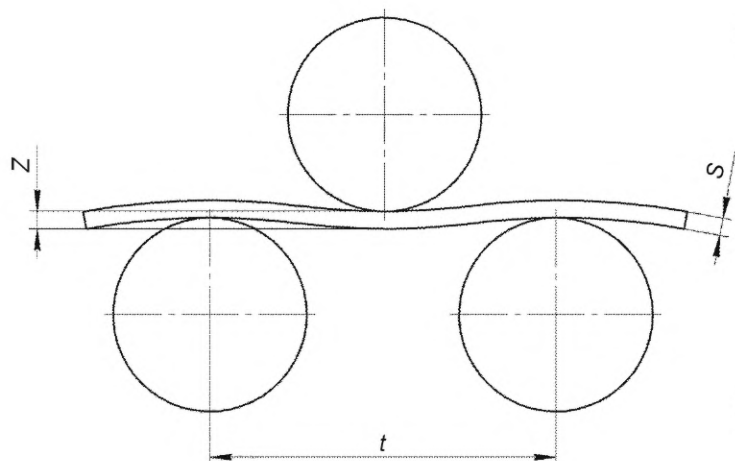
Рисунок 1 — Схема настройки рабочих валков
