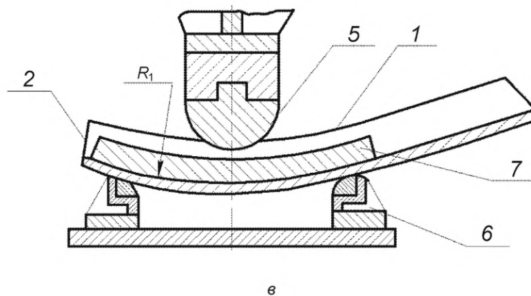
б, в — формообразование в цилиндрическом штампе
