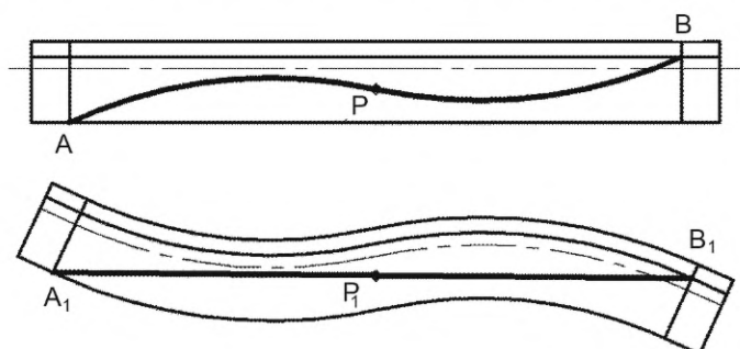
в — деталь S-образной формы с одной спрямляемой кривой
