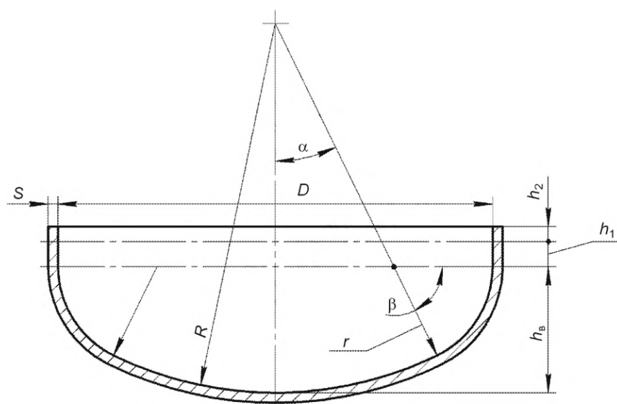
б — торосферические и коробовые
