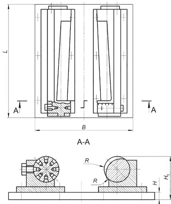
Рисунок 8 — Комбинированный листогибочный штамп для гибки цилиндрических и конических деталей
