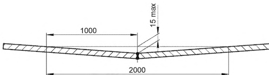
Рисунок 16 — Схема измерений угловатости сварной заготовки
