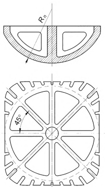
Рисунок 24 — Пуансон для горячей штамповки
