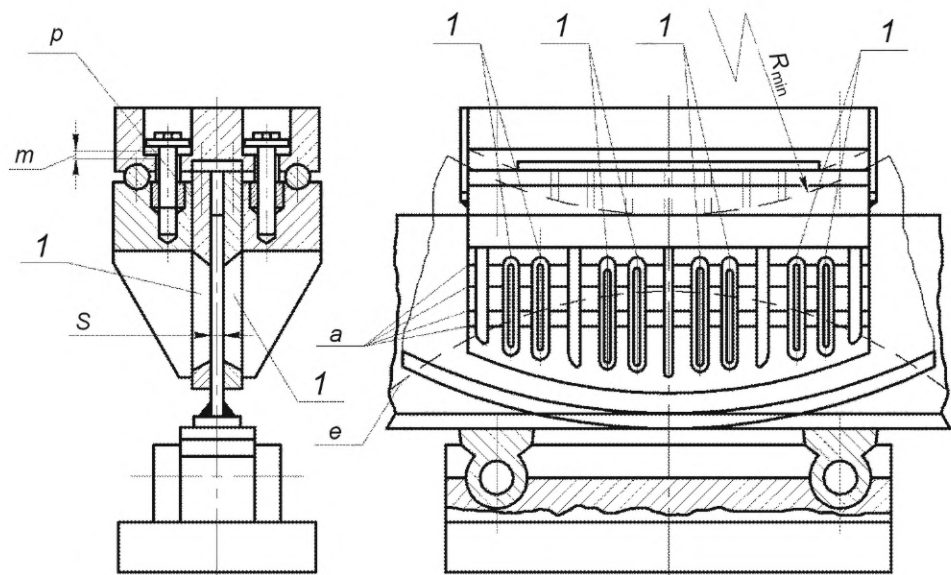
p — поворотные щеки штампа; m — зазор; S — толщина стенки профиля; e — «спрямляемая кривая»; R_{min} — минимальный радиус гибки; a — горизонтальные ориентирные линии; 1 — смотровые щели Рисунок 41 — Типовой штамп для гибки сварных тавровых балок полкой наружу
