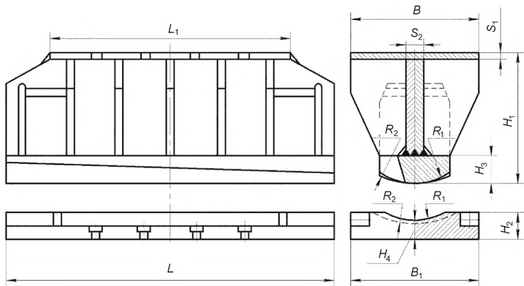
H_1 — высота пуансона; H_2 — толщина матрицы; H_3 — толщина пуансона; H_4 — толщина заглабления матрицы; B — ширина пуансонодержателя; L и L_1 — длина плиты матрицы и пуансонодержателя; B_1 — ширина матрицы; S_1 — толщина плиты пуансонодержателя; S_2 — толщина ребра пуансонодержателя; R_1 и R_2 — радиусы на противоположных концах пуансона и матрицы
