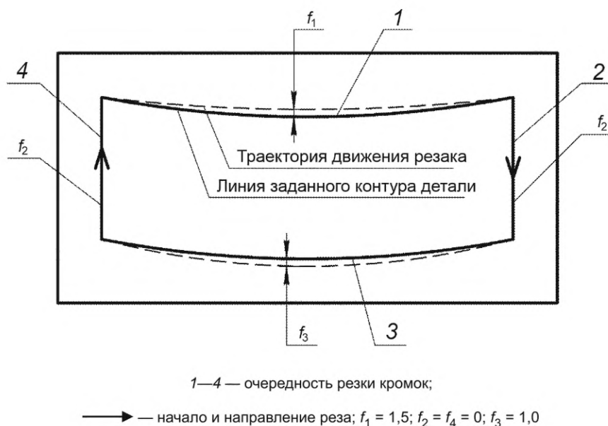
Рисунок 2 — Чертеж для вырезки деталей, близких к размерам листа
