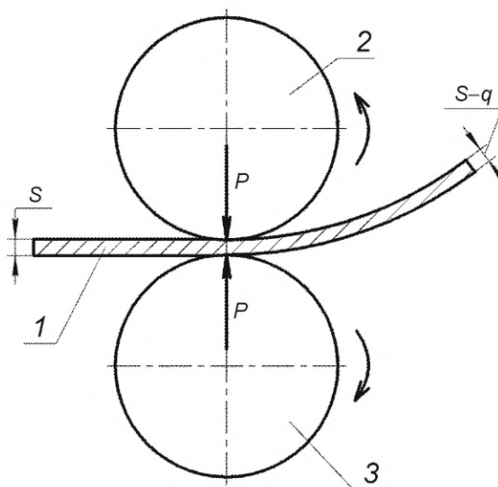
1 — заготовка; 2 — верхний гибочный ролик; 3 — нижний гибочный ролик; P — усилие гибки; S — толщина заготовки; q — утонение
