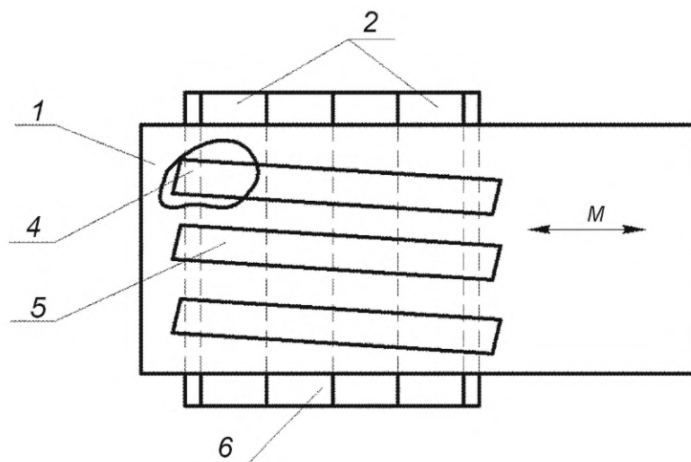
а — укладка прокладок перед формообразованием
