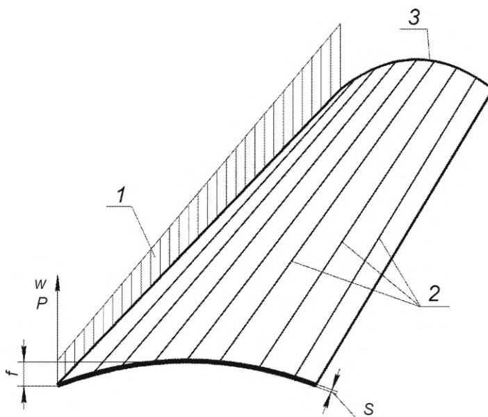
1 — эпюра изменения прогиба листа под роликом w или усилия гибки P ; 2 — линиигиба; 3 — узкая кромка листовой заготовки; w — прогиб листа под роликом; P — усилие гибки; f — стрелка погиба листа; S — толщина листа
