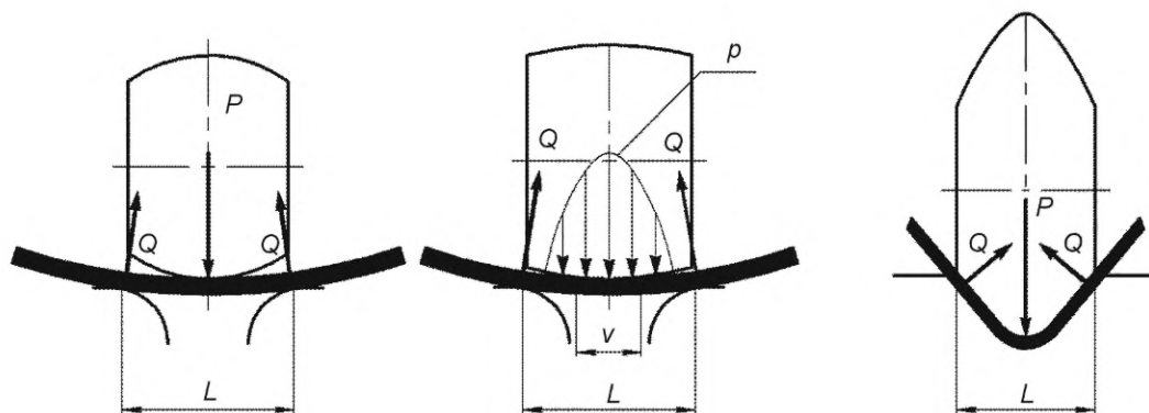
P — сосредоточенное усилие гибки; p — распределенное усилие гибки; Q — реакции опор; L — расстояние между опорами; v — зона облегания
