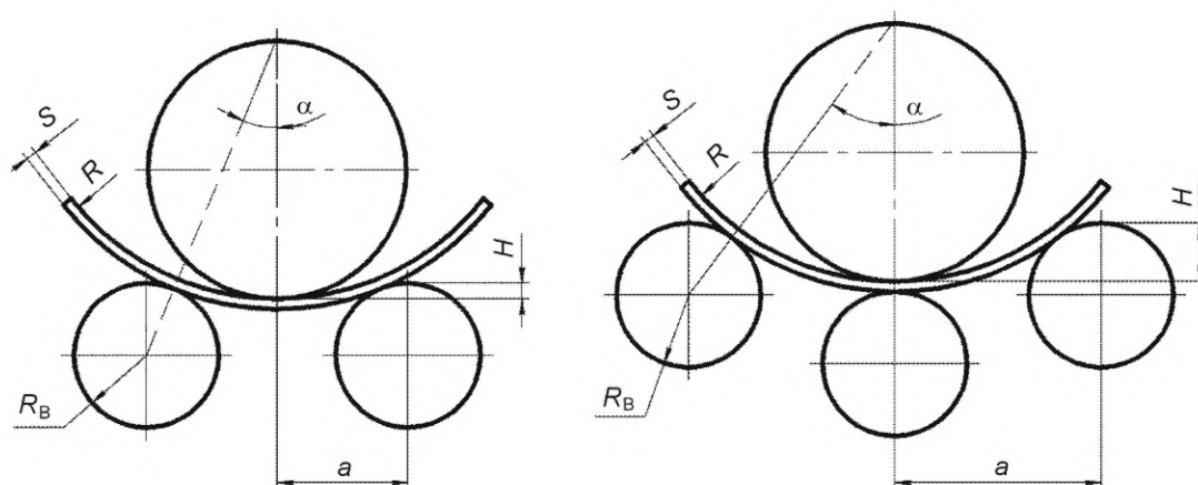
а — трехвалковые вальцы
