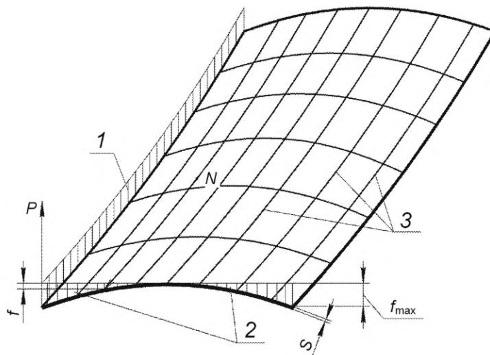
1 — эпюра изменения усилия при прокатке; 2 — эпюра изменения усилия от одной прокатки к другой; 3 — линии прокатки; P — усилие раскатки; f — стрелка прогиба листа; f_{\max} — максимальная стрелка прогиба листа; S — толщина листа
