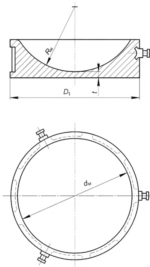
Рисунок 23 — Матрица для горячей штамповки
