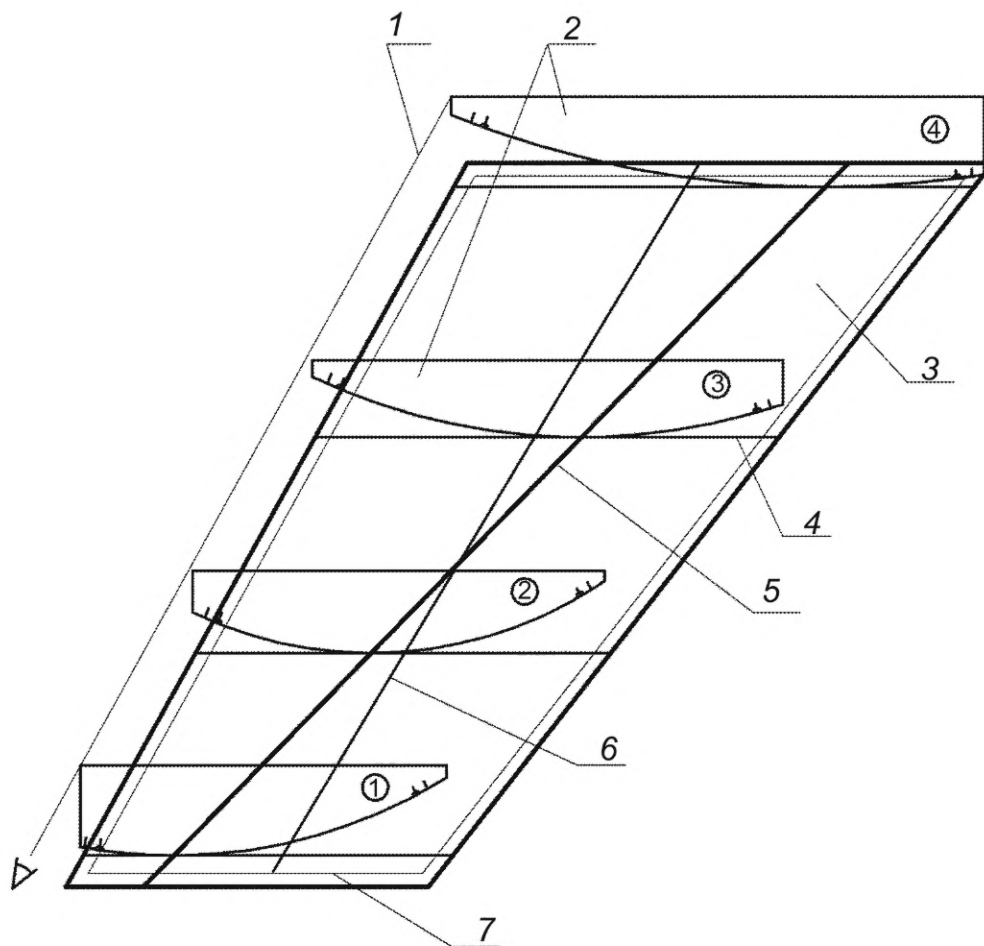
1 — линия горизонтирования шаблонов по базовой кромке; 2 — поперечные шаблоны; 3 — листовая заготовка; 4 — линия приложения поперечного шаблона; 5 — базовая линиягиба; 6 — линия приложения продольного шаблона; 7 — линия припуска
