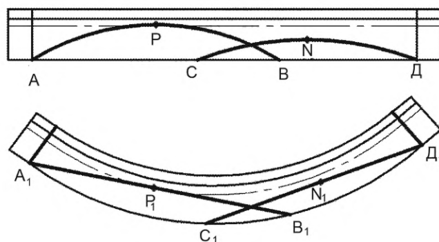
б — деталь с изгибом бульбой внутрь и двумя спрямляемыми кривыми
