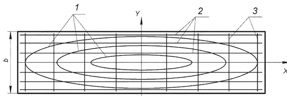
а — изопараметрические линии утонения при гибке раскаткой
