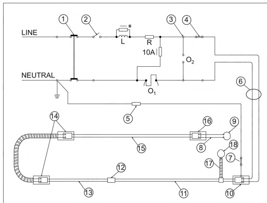
Рисунок 6 — Испытание соединения секций шинопровода статической нагрузкой
