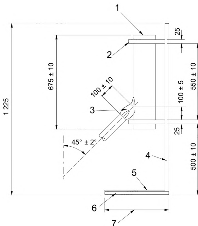
1 — образец, расположенный по центру горизонтальной плоскости; 2 — зажим; 3 — пламя; 4 — задняя стенка; 5 — тонкая бумага; 6 — деревянная доска толщиной 10 мм и шириной 700^{+0}_{-25} ; 7 — глубина 450^{+0}_{-25}
