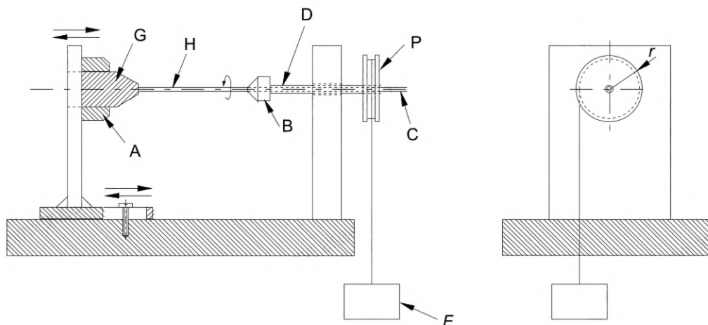
A — устройство фиксации корпуса образца; B — устройство для фиксации кабеля образца; C — конец кабеля; D — вал вращения (полый); r — радиус шкива; F — вес (момент = F \times r ); P — шкив; G — образец; H — кабель
