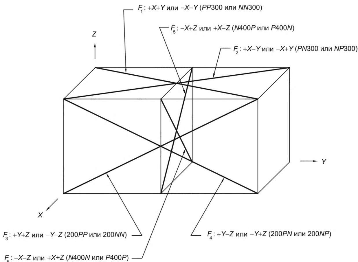
Рисунок 2 — Примеры диагоналей в плоскости фронтальной грани прямоугольной призмы
