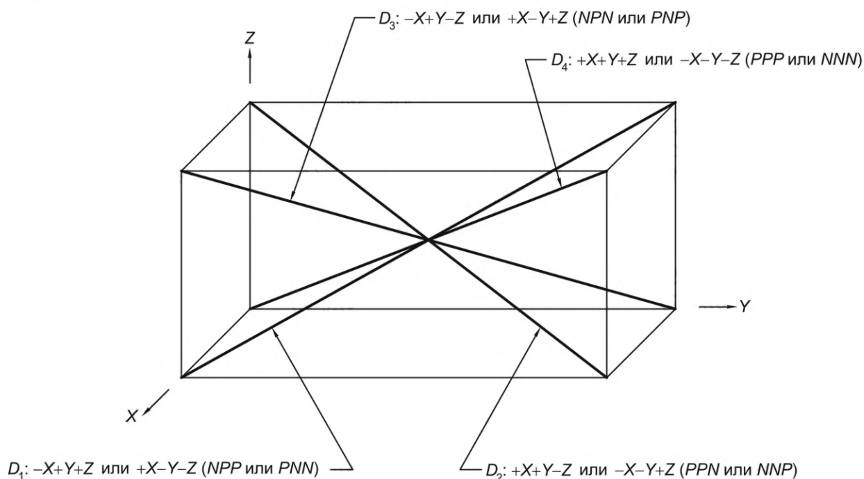
Рисунок 1 — Четыре диагонали в объеме прямоугольной призмы
