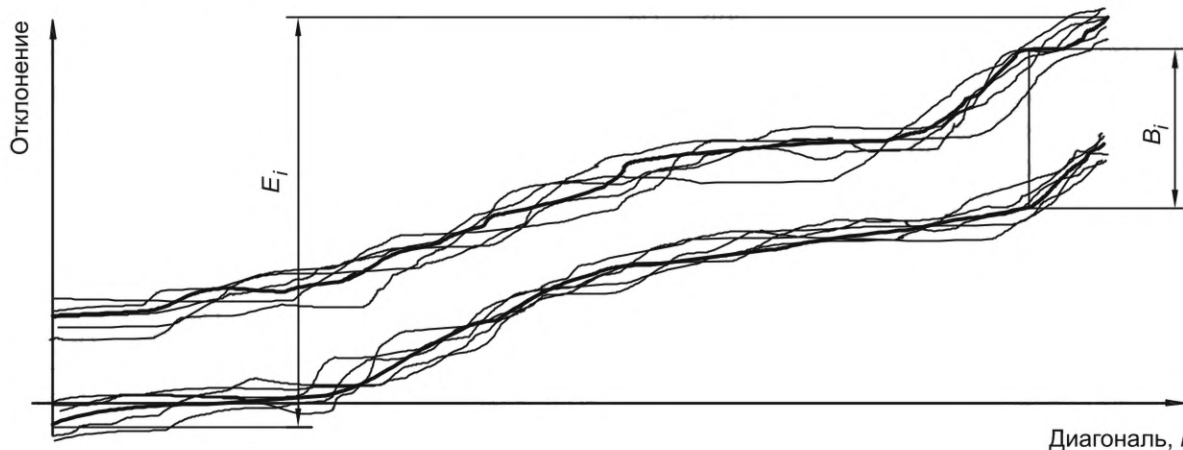
Рисунок 3 — Оценка E_i and B_i
