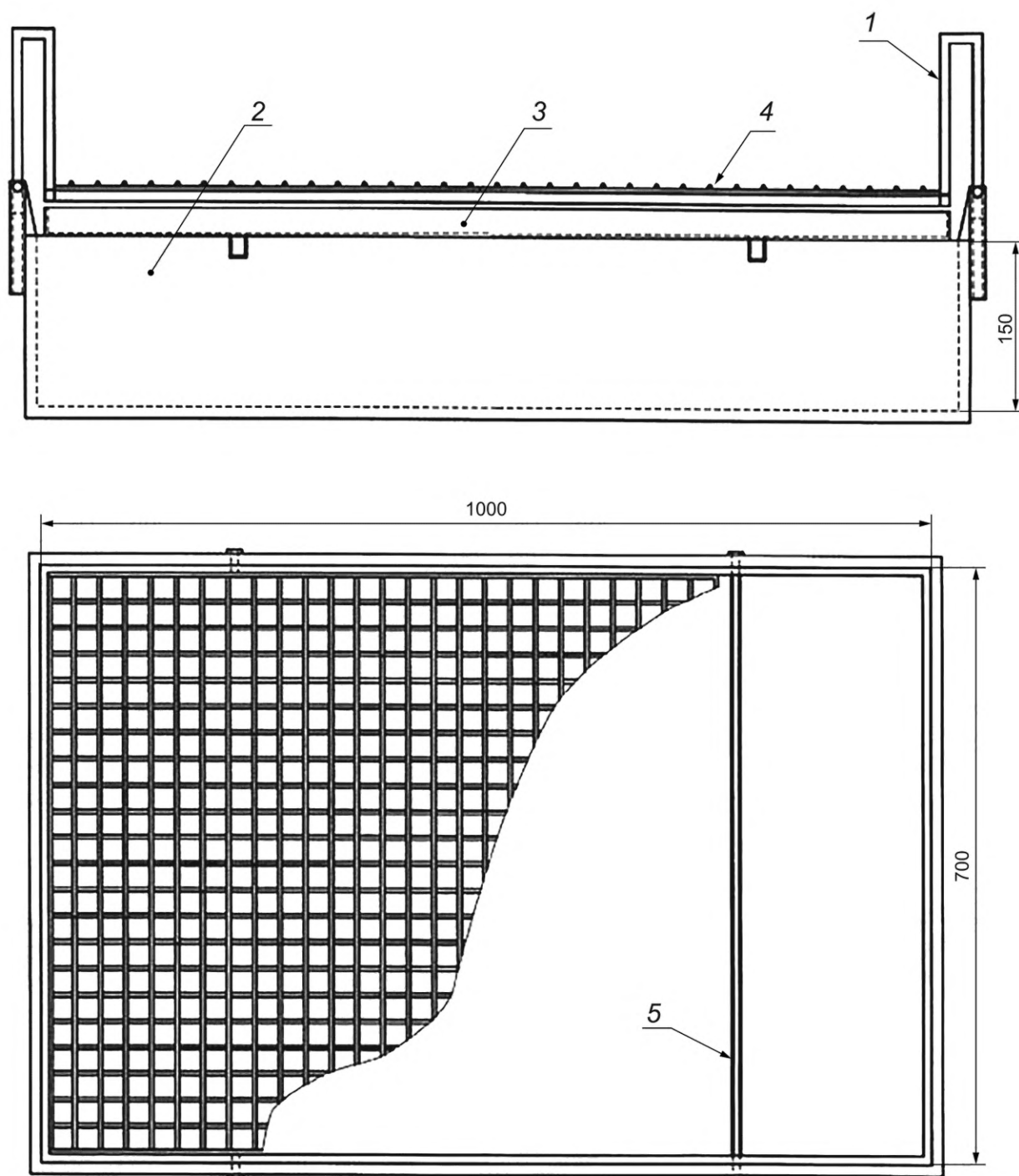
Рисунок 1 — Устройство для определения абсорбционной способности
