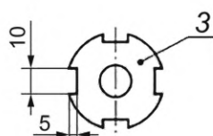
в) Вид пробки 3 сверху
