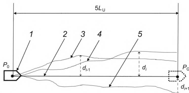
1 — робот; 2 — заданный маршрут; 3 — (i - 1) -й фактический маршрут; 4 — i -й фактический маршрут; 5 — (i + 1) -й фактический маршрут
