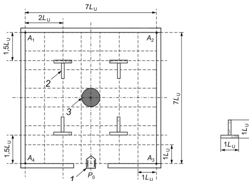
Рисунок 11 — Компоновка стенда для испытаний по картографированию
