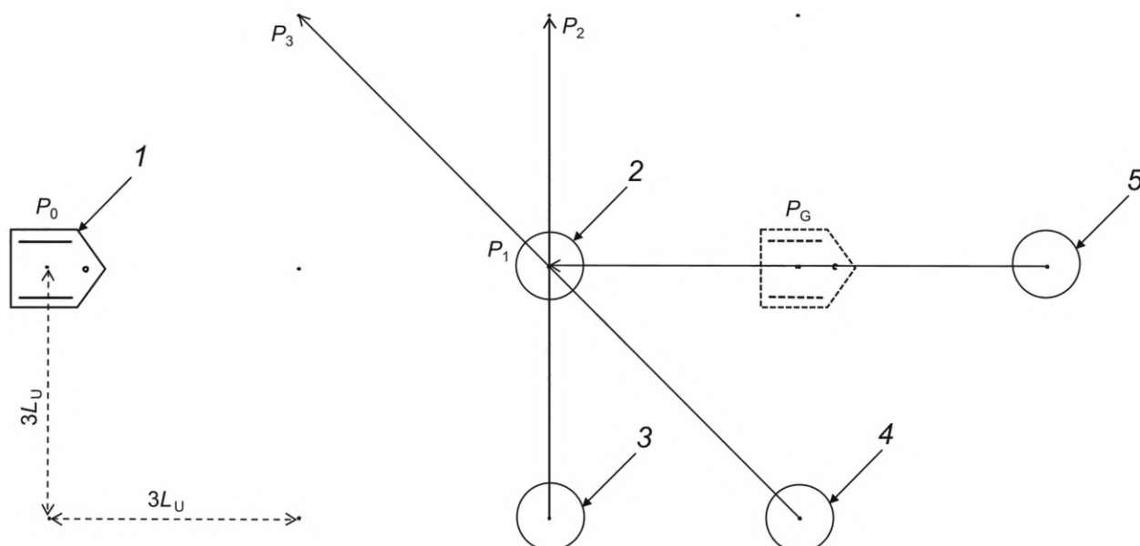
Рисунок 8 — Схема испытательного стенда и алгоритмы поведения препятствия (вид сверху)
