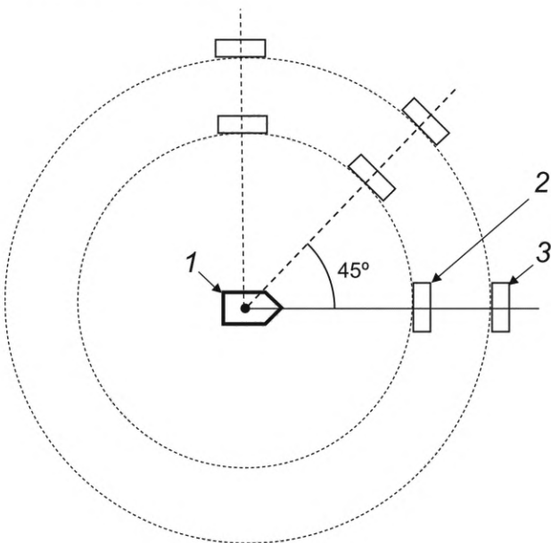
1 — мобильный робот; 2 — препятствия на минимальной дальности; 3 — препятствия на максимальной дальности
