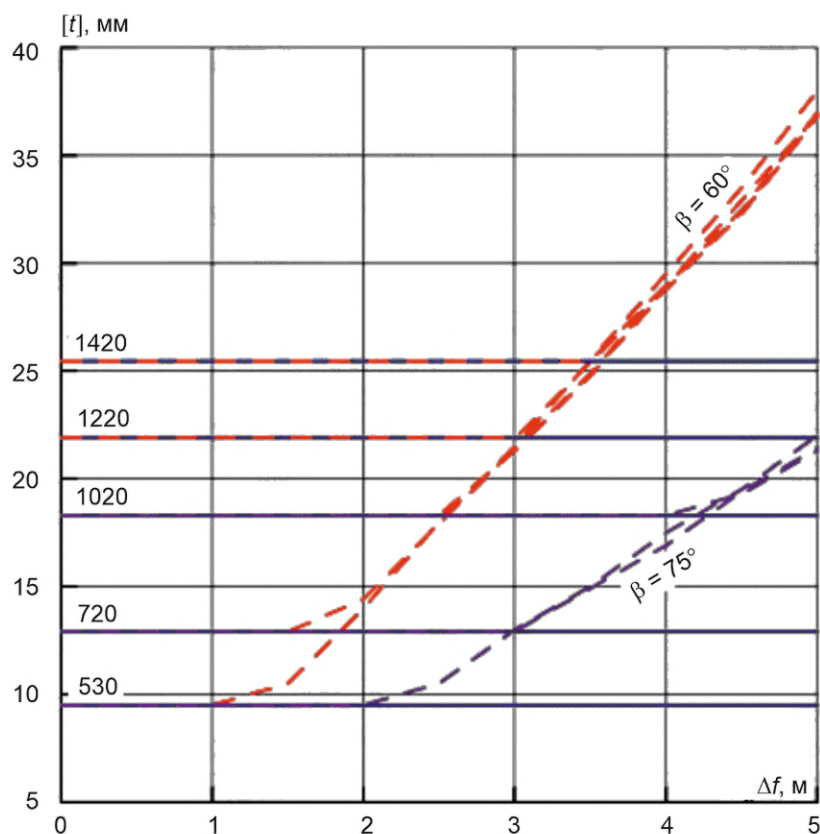
Рисунок В.31 — Сдвиг, глина, К70, p = 11,8 МПа
