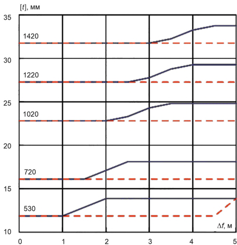
Рисунок В.16 — Сдвиг, песок, К70, p = 14,7 МПа
