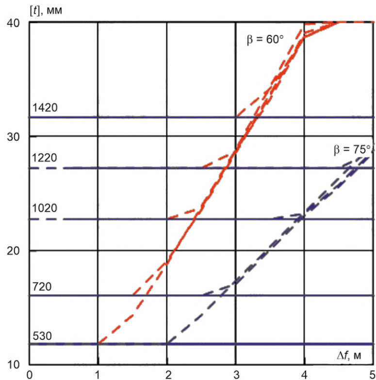
Рисунок В.23 — Сдвиг, глина, К60, p = 11,8 МПа
