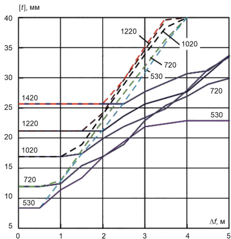
Рисунок В.54 — Сброс, глина, К60, p = 9,8 МПа
