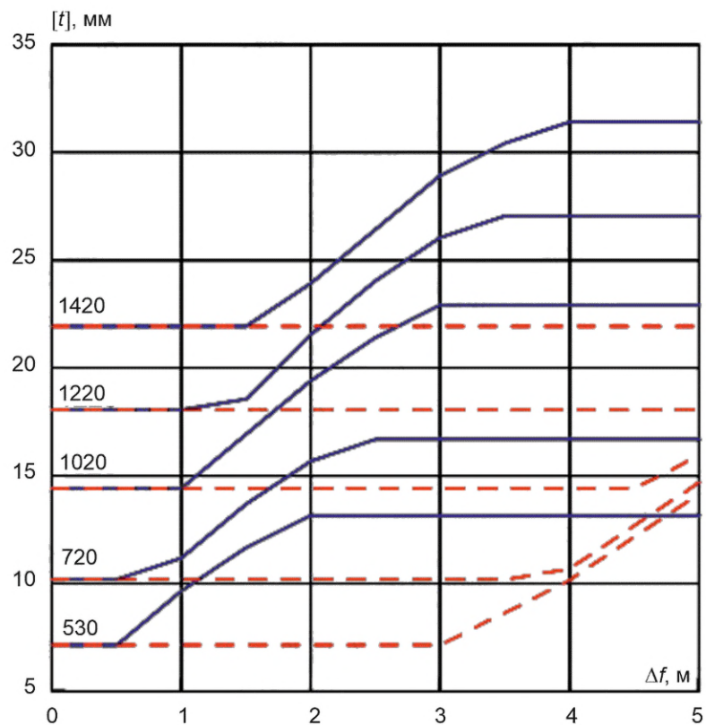
Рисунок В.14 — Сдвиг, песок, K70, p = 9,8 МПа
