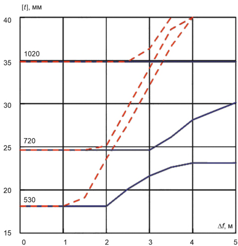
Рисунок В.52 — Сброс, глина, К55, \rho = 14,7 МПа
