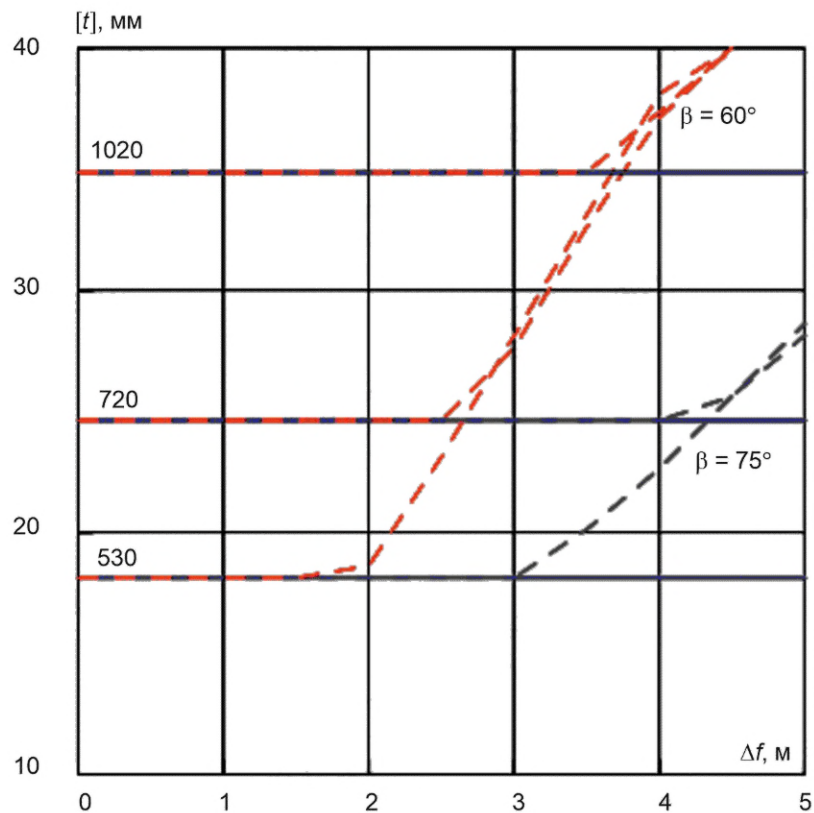
Рисунок В.20 — Сдвиг, глина, К55, p = 14,7 МПа
