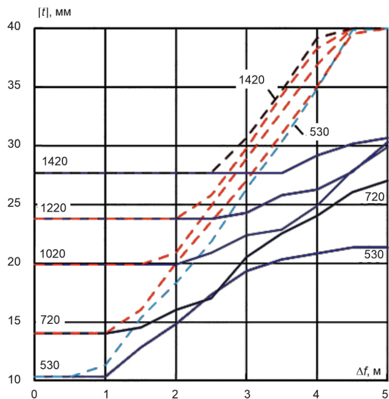
Рисунок В.59 — Сброс, глина, К65, p = 11,8 МПа
