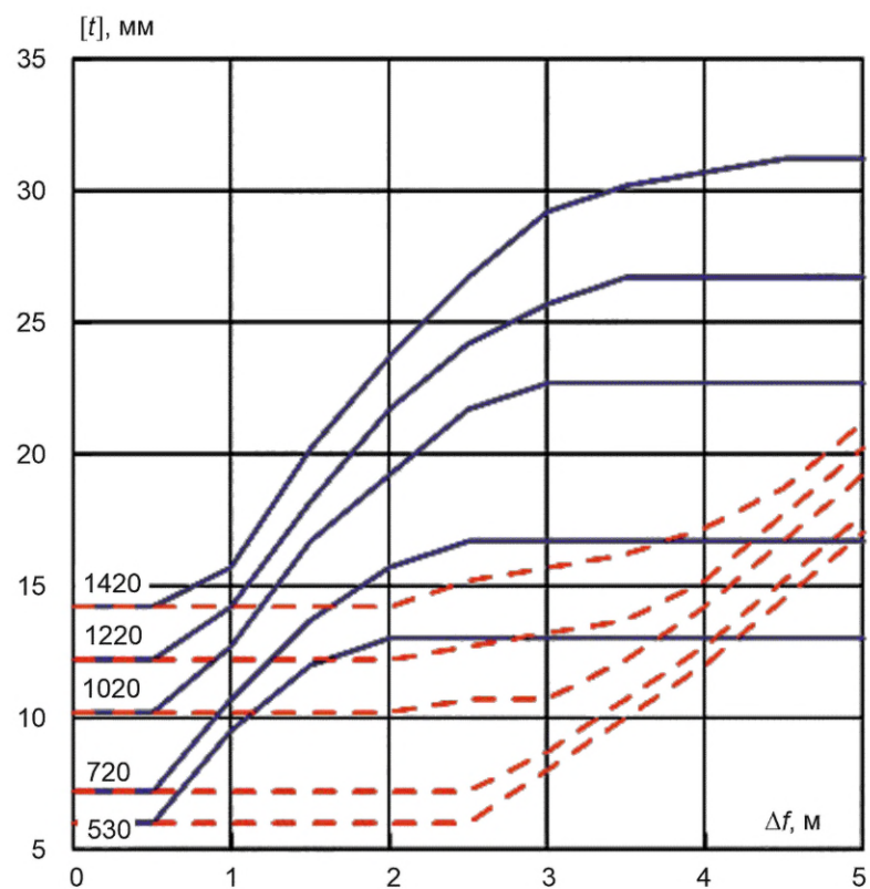
Рисунок В.9 — Сдвиг, песок, K65, p = 5,4 МПа
