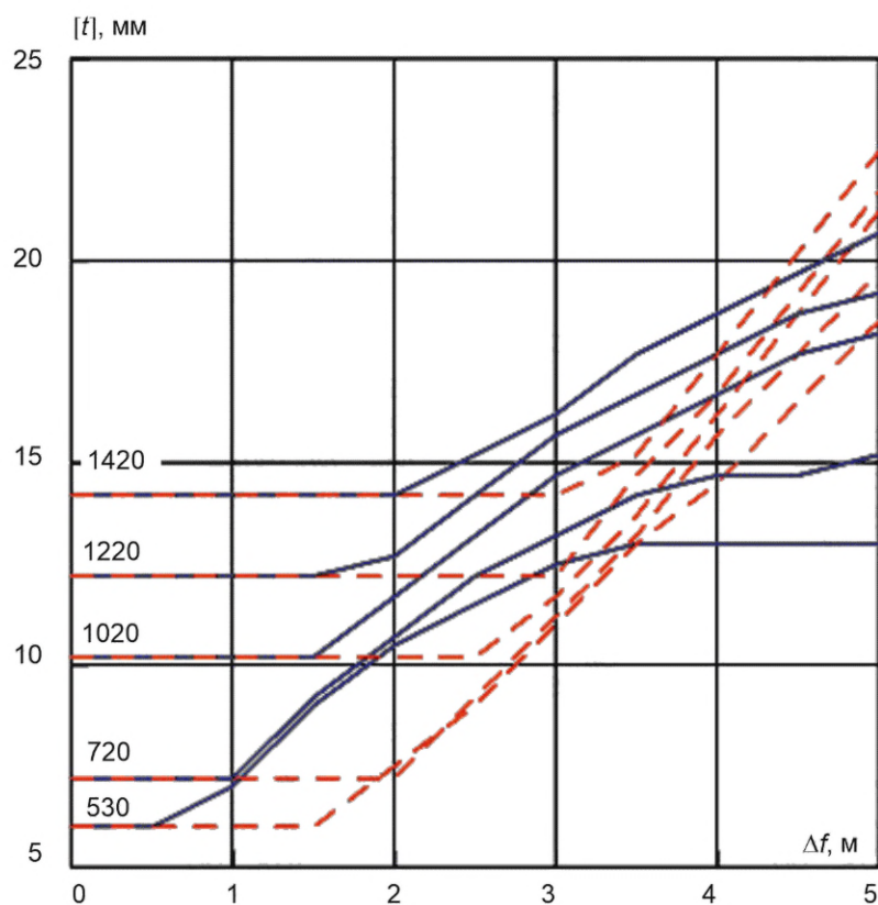
Рисунок В.41 — Сброс, песок, К65, p = 5,4 МПа
