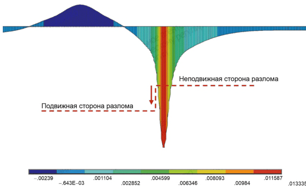
Рисунок Г.2 — Распределение полных продольных деформаций вдоль верхней образующей трубопровода
