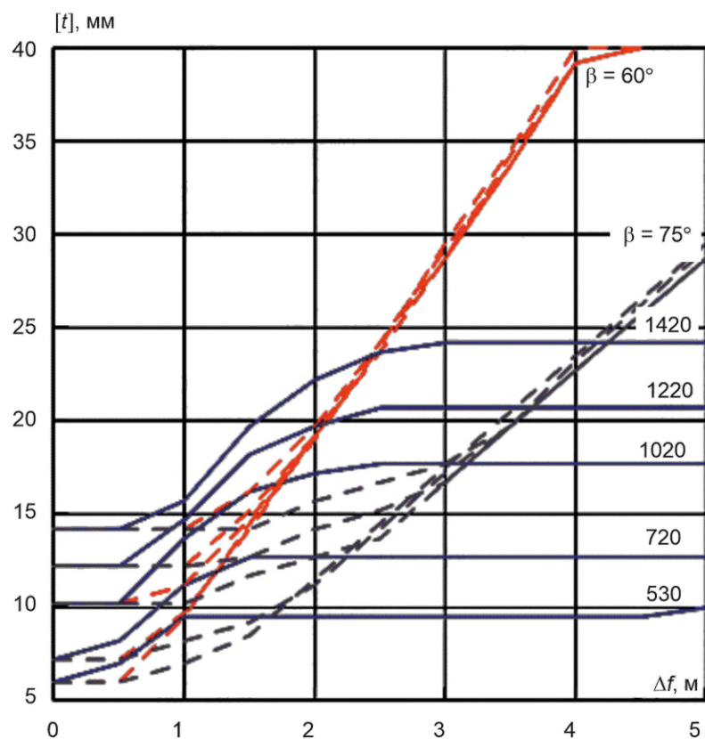
Рисунок В.21 — Сдвиг, глина, К60, p = 5,4 МПа
