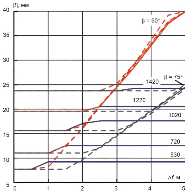
Рисунок В.26 — Сдвиг, глина, К65, p = 9,8 МПа
