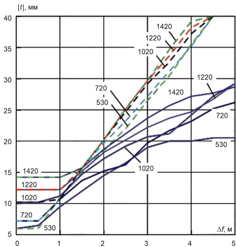
Рисунок В.57 — Сброс, глина, К65, p = 5,4 МПа
