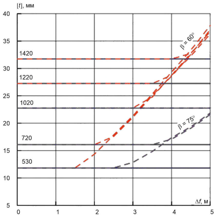
Рисунок В.32 — Сдвиг, глина, К70, p = 14,7 МПа
