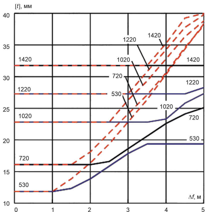
Рисунок В.64 — Сброс, глина, К70, p = 14,7 МПа
