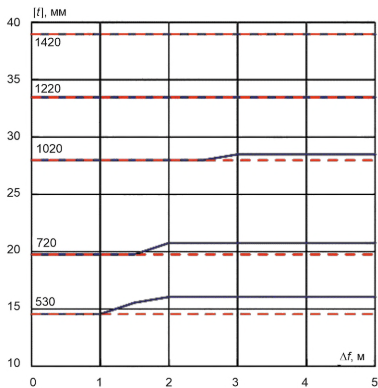
Рисунок В.3 — Сдвиг, песок, К55, p = 11,8 МПа
