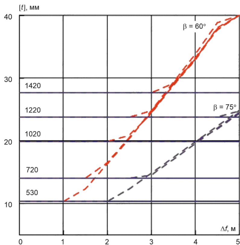
Рисунок В.27 — Сдвиг, глина, К65, p = 11,8 МПа
