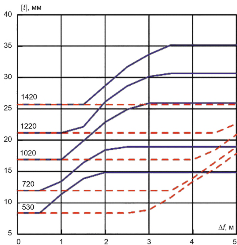
Рисунок В.6 — Сдвиг, песок, К60, \rho = 9,8 МПа
