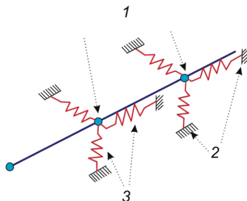
1 — узлы балочной модели; 2 — узлы на концах «грунтовых пружин»; 3 — «грунтовые пружины»
