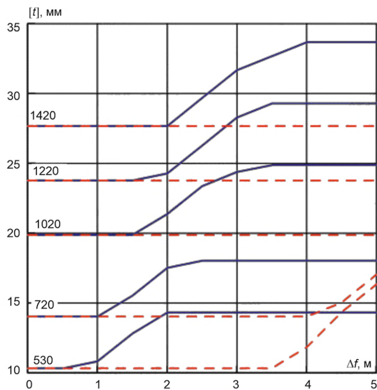
Рисунок В.11 — Сдвиг, песок, К65, p = 11,8 МПа
