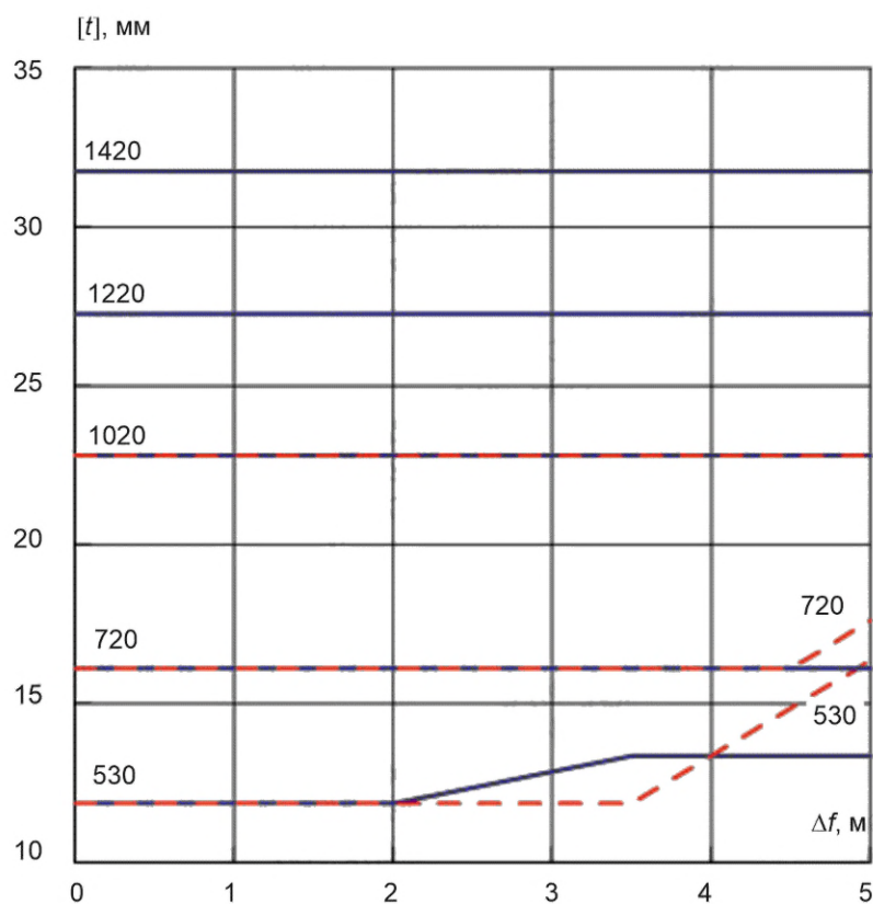
Рисунок В.48 — Сброс, песок, К70, \rho = 14,7 МПа
