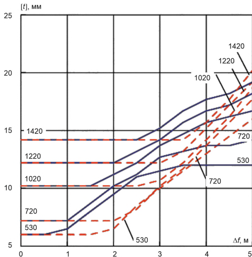
Рисунок В.45 — Сброс, песок, К70, p = 5,4 МПа
