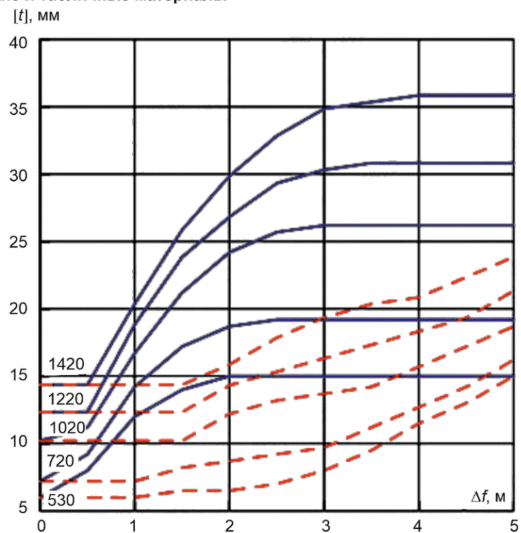
Рисунок В.1 — Сдвиг, песок, К55, p = 5,4 МПа
