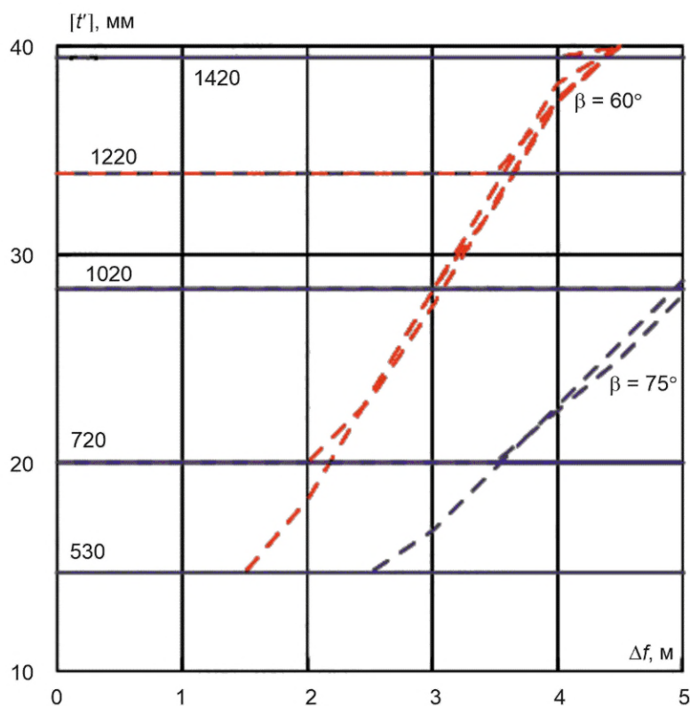
Рисунок В.24 — Сдвиг, глина, К60, p = 14,7 МПа
