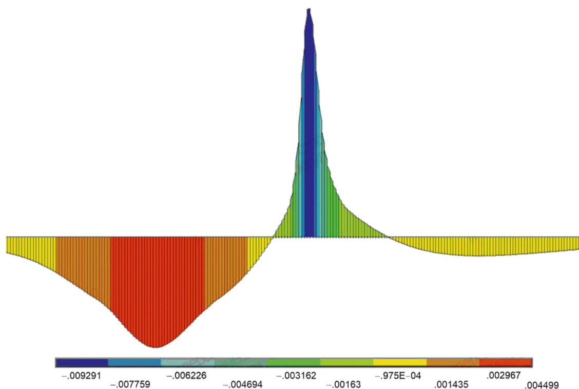
Рисунок Г.3 — Распределение полных продольных деформаций вдоль нижней образующей трубопровода
