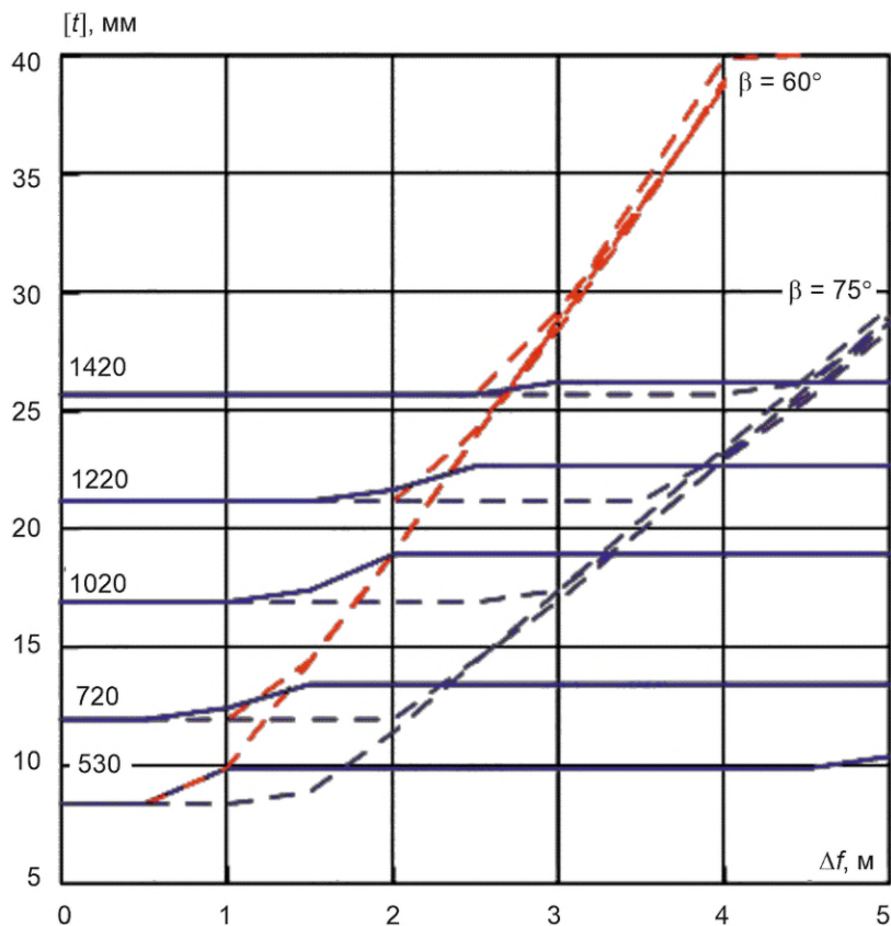
Рисунок В.22 — Сдвиг, глина, К60, p = 9,8 МПа
