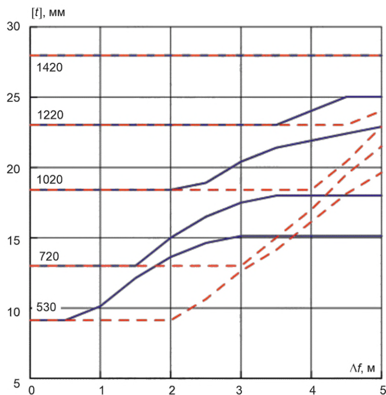
Рисунок В.34 — Сброс, песок, К55, p = 9,8 МПа
