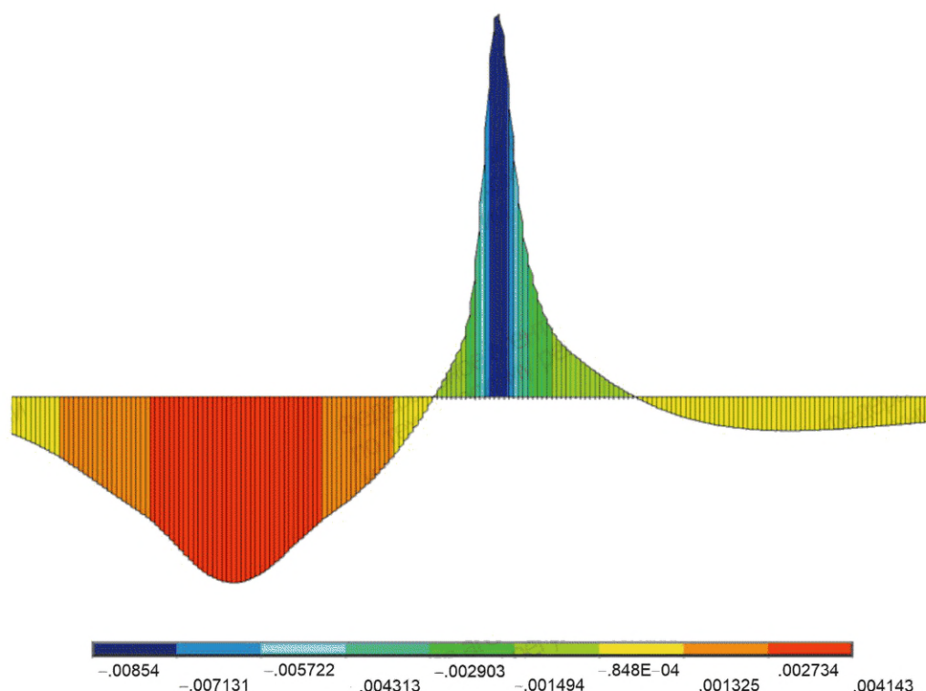
Рисунок Г.5 — Распределение полных продольных деформаций вдоль нижней образующей трубопровода для скорректированной толщины стенки
