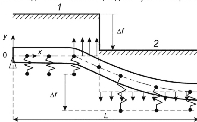
\Delta f — полное прогнозное смещение АТР, м; L — длина расчетного участка газопровода, м; 1 — неподвижная сторона; 2 — подвижная сторона
