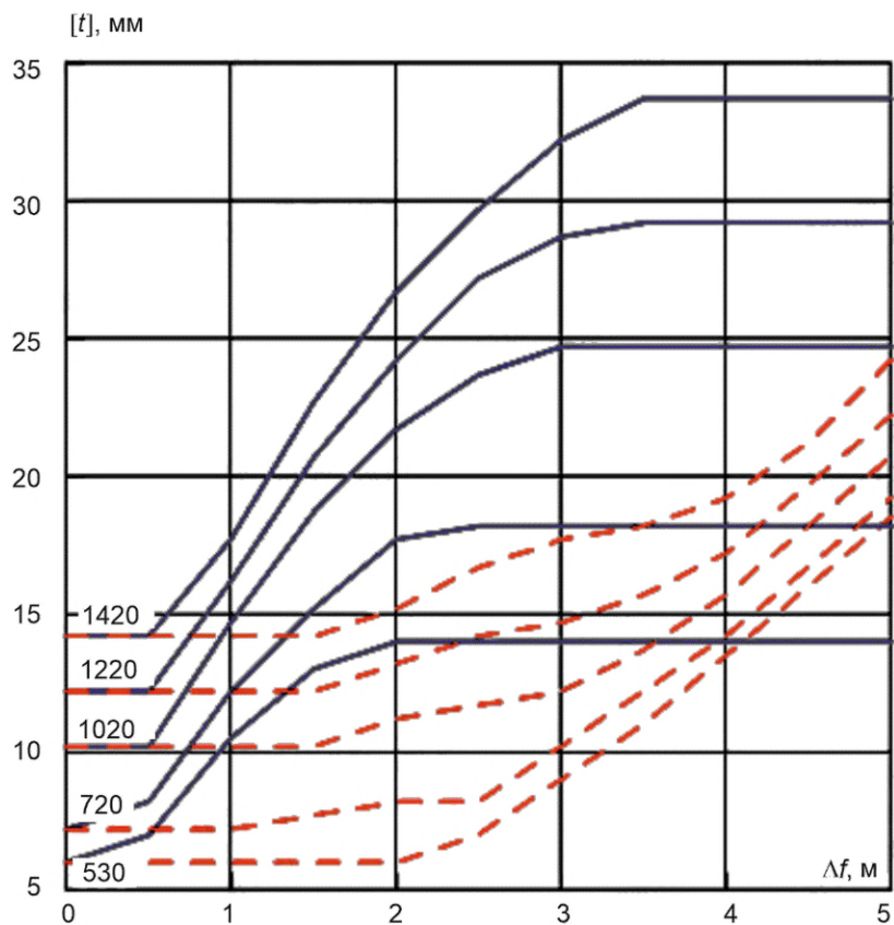
Рисунок В.5 — Сдвиг, песок, K60, p = 5,4 МПа
