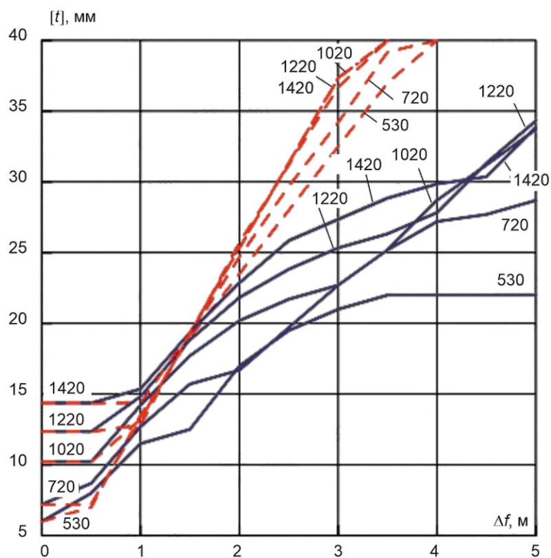
Рисунок В.49 — Сброс, глина, К55, p = 5,4 МПа
