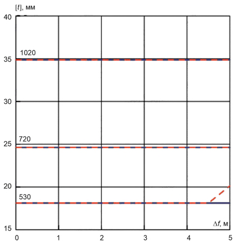
Рисунок В.36 — Сброс, песок, К55, p = 14,7 МПа
