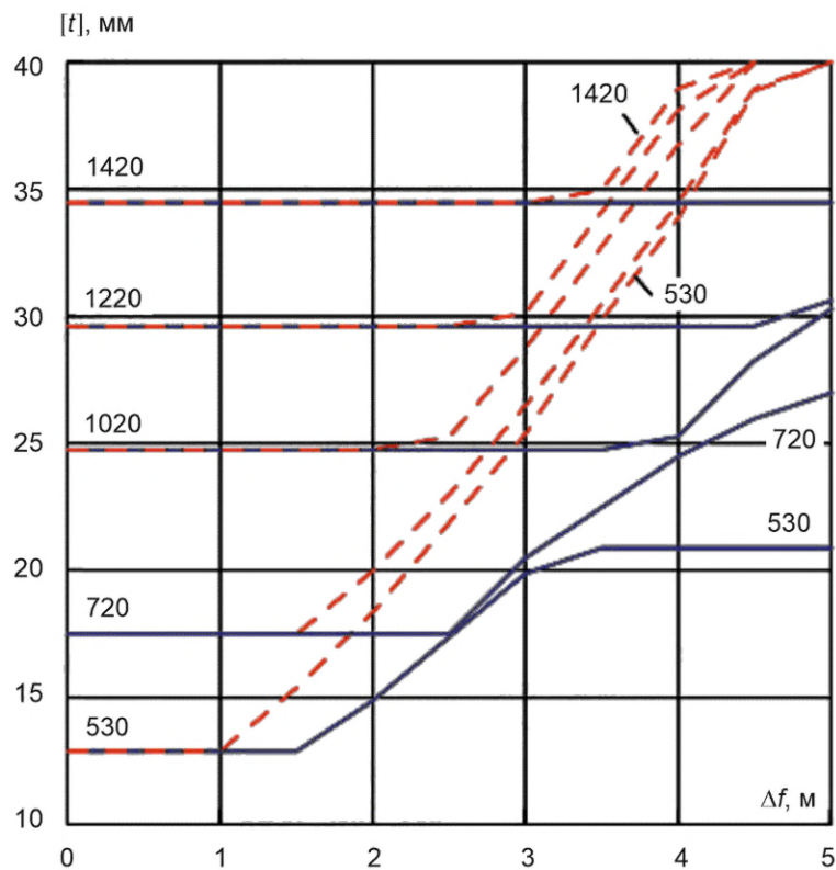
Рисунок В.60 — Сброс, глина, К65, p = 14,7 МПа
