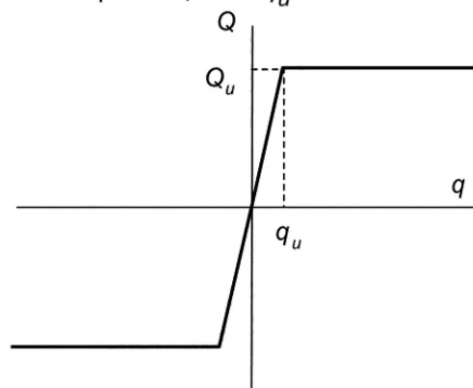
Рисунок 10.3 — Зависимость типа «билинейная диаграмма»
