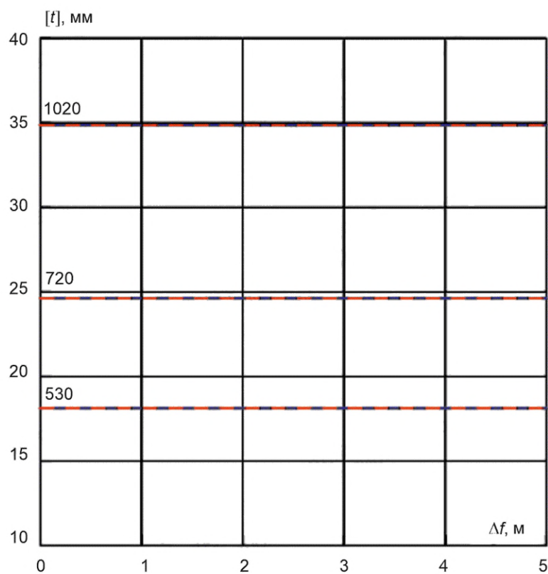
Рисунок В.4 — Сдвиг, песок, К55, p = 14,7 \text{ МПа}
