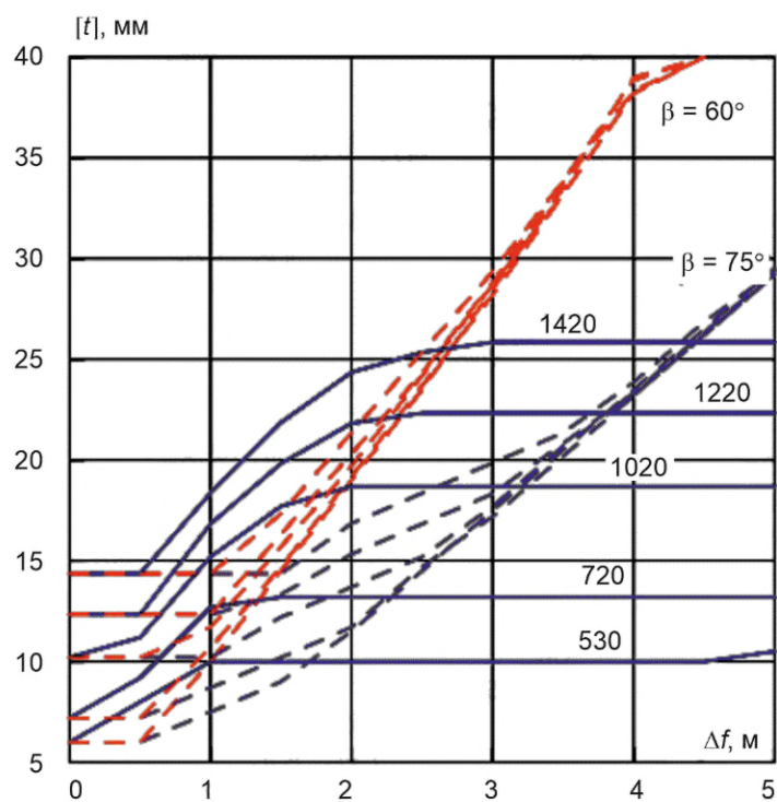
Рисунок В.17 — Сдвиг, глина, К55, p = 5,4 МПа
