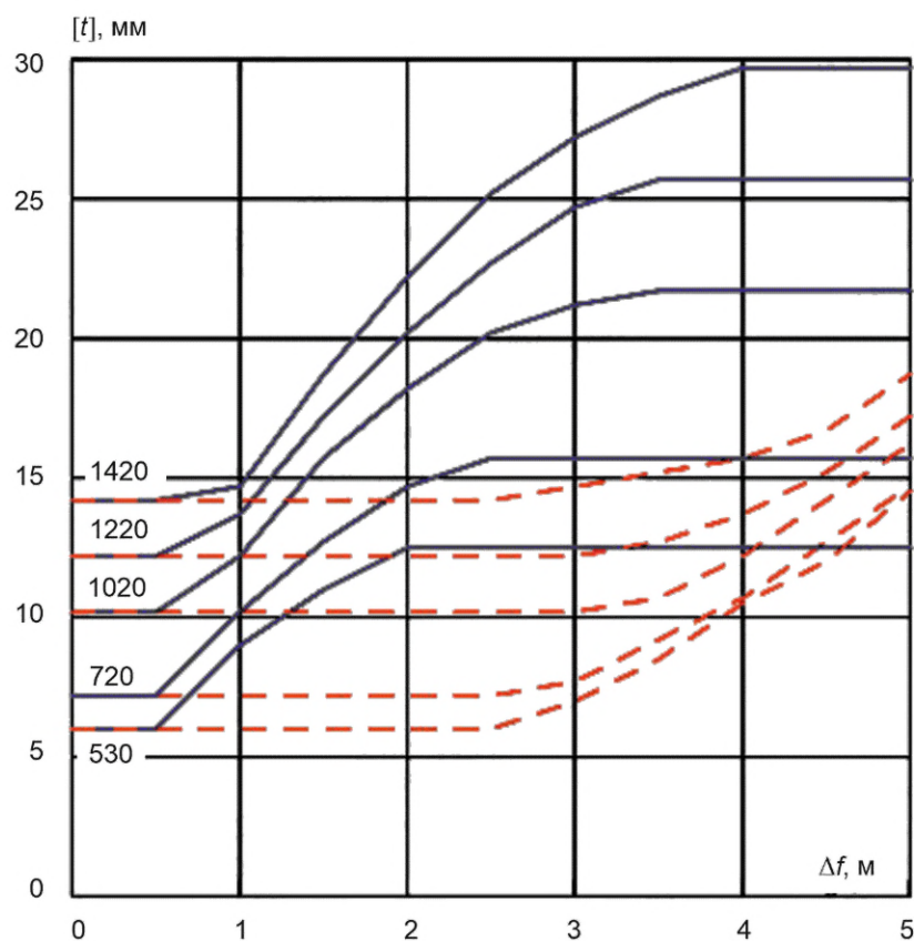
Рисунок В.13 — Сдвиг, песок, К70, p = 5,4 МПа
