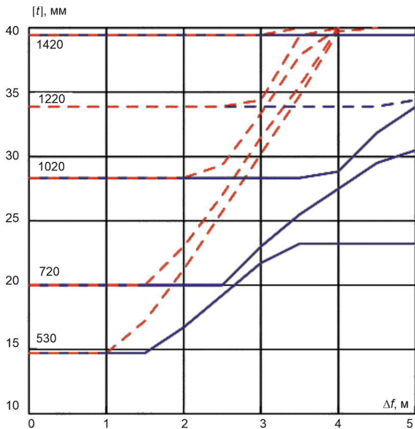
Рисунок В.56 — Сброс, глина, К60, p = 14,7 МПа
