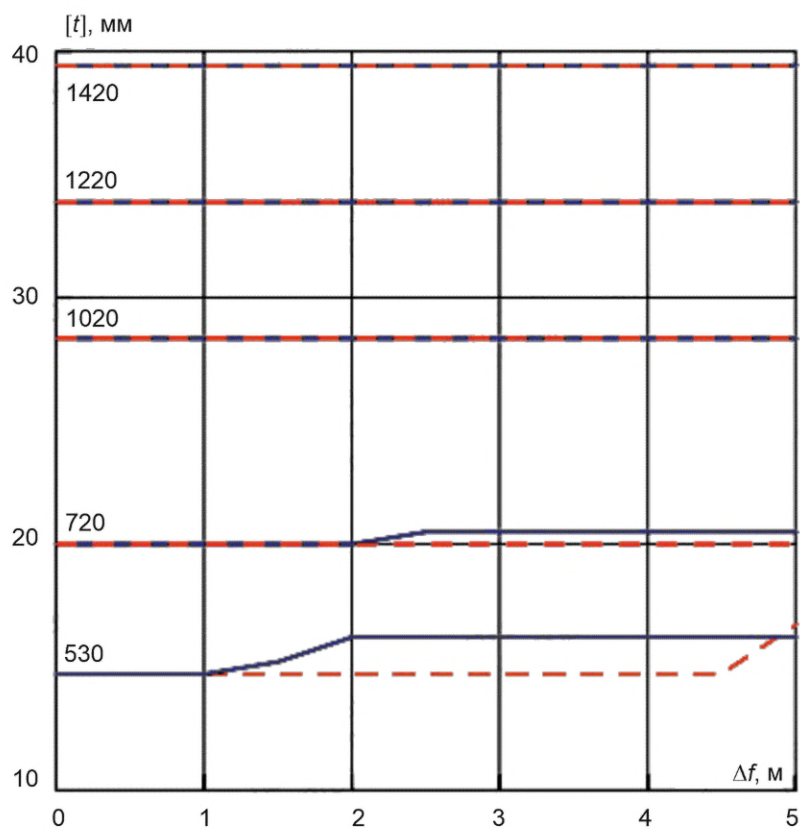
Рисунок В.8 — Сдвиг, песок, К60, p = 14,7 МПа
