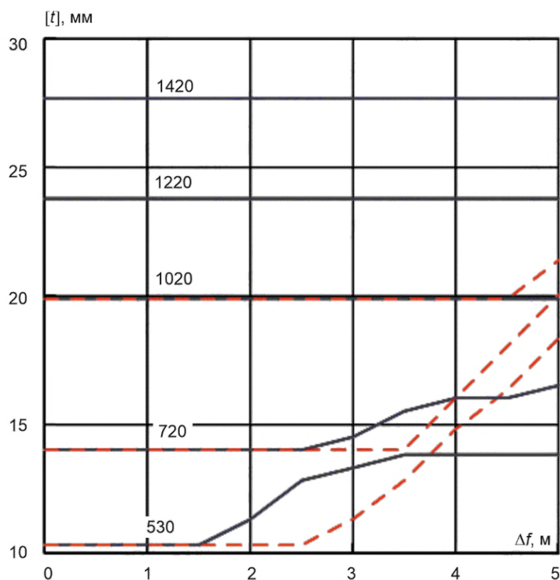
Рисунок В.43 — Сброс, песок, K65, \rho = 11,8 МПа
