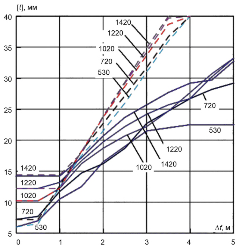
Рисунок В.53 — Сброс, глина, К60, p = 5,4 МПа
