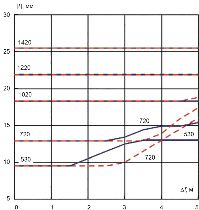
Рисунок В.47 — Сброс, песок, K70, p = 11,8 МПа
