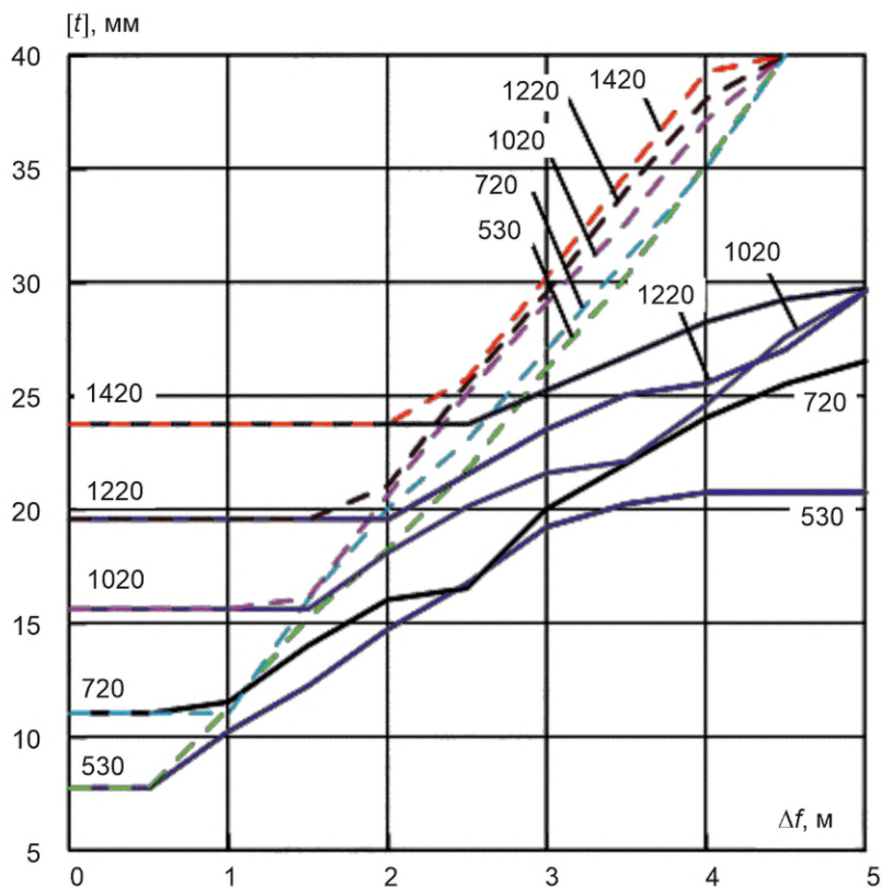
Рисунок В.58 — Сброс, глина, К65, p = 9,8 МПа
