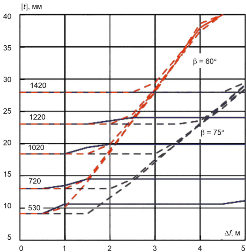
Рисунок В.18 — Сдвиг, глина, К55, p = 9,8 МПа
