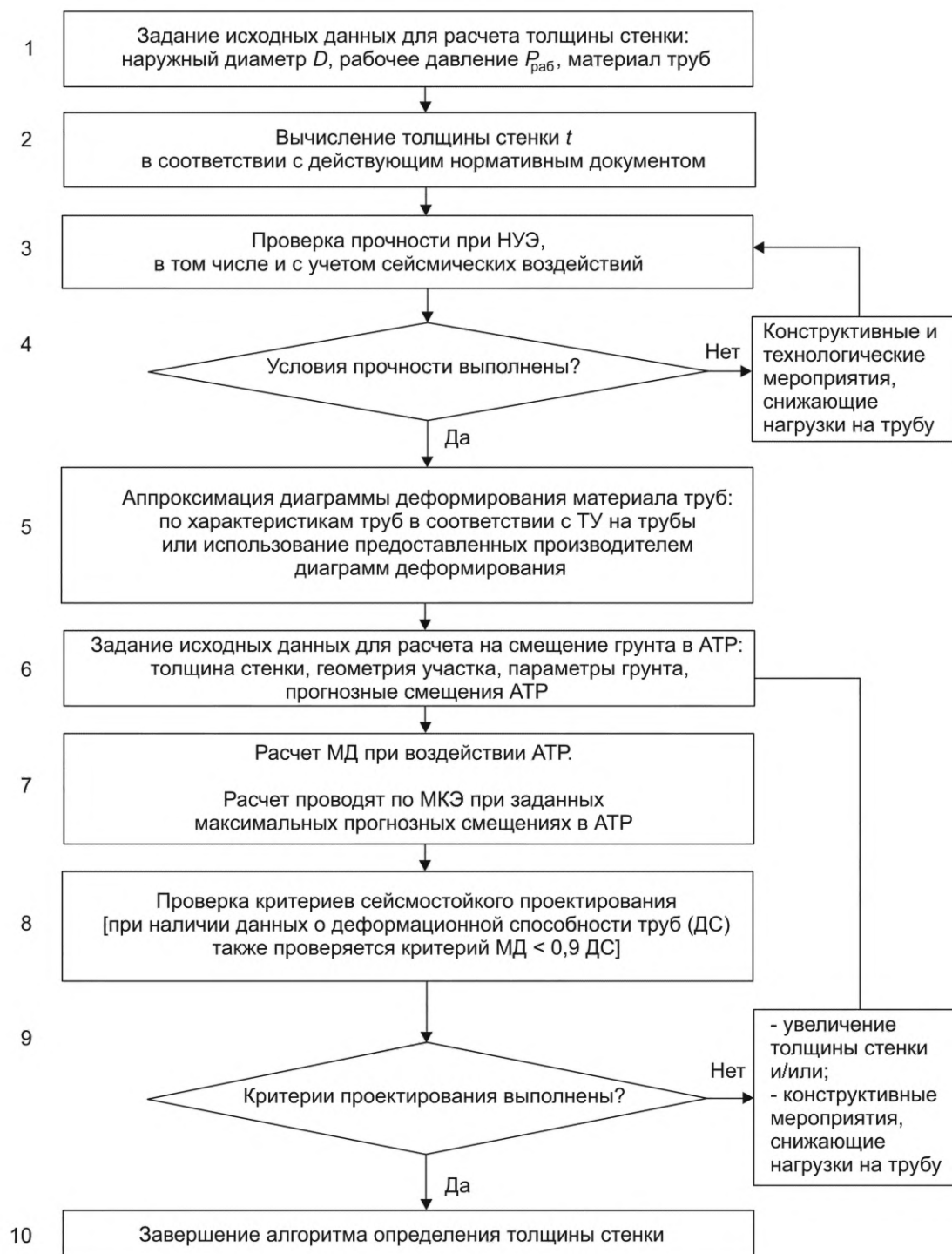
Рисунок 13.1 — Блок-схема алгоритма определения толщины стенки труб для участков пересечения АТР
