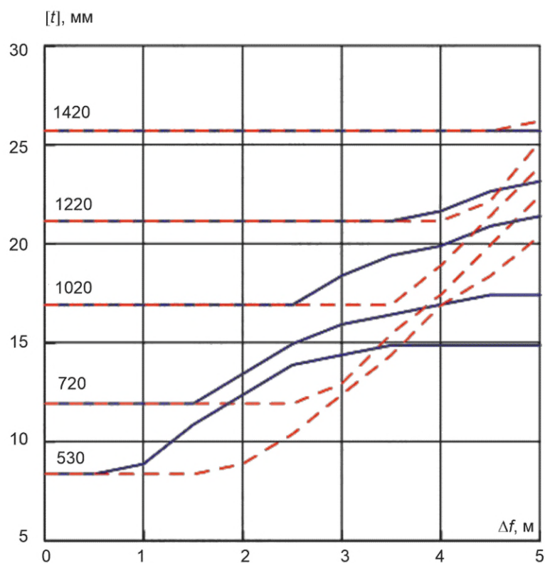
Рисунок В.38 — Сброс, песок, К60, p = 9,8 МПа
