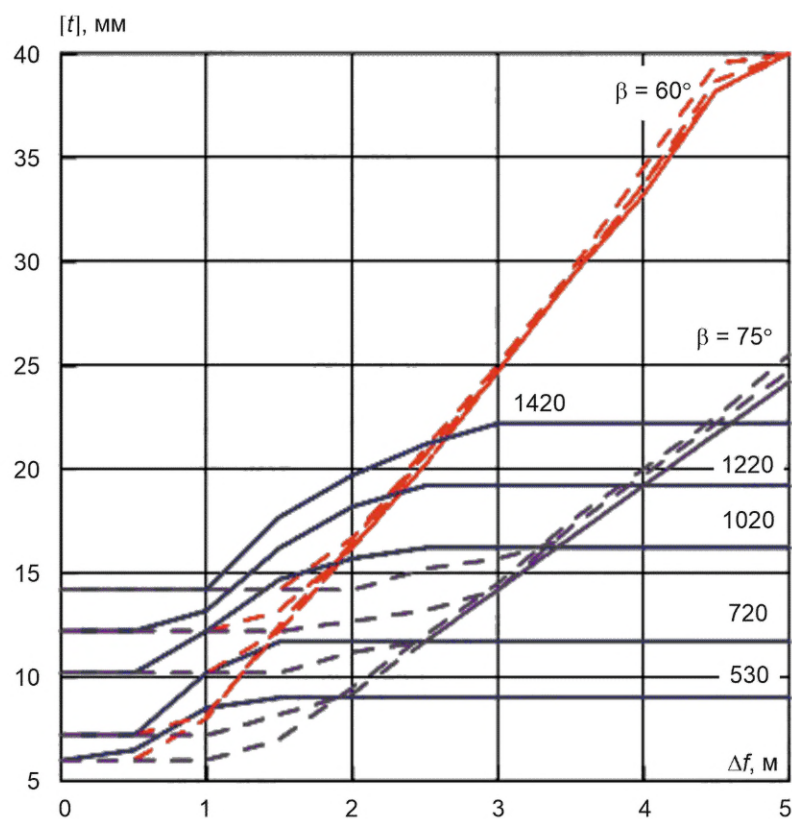
Рисунок В.25 — Сдвиг, глина, К65, p = 5,4 МПа
