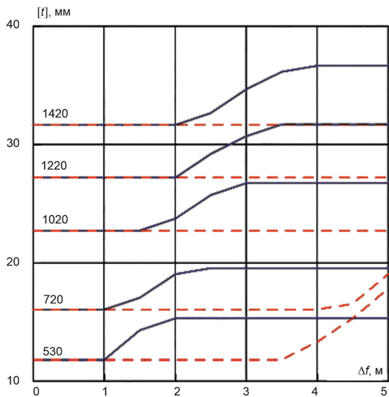
Рисунок В.7 — Сдвиг, песок, К60, p = 11,8 МПа
