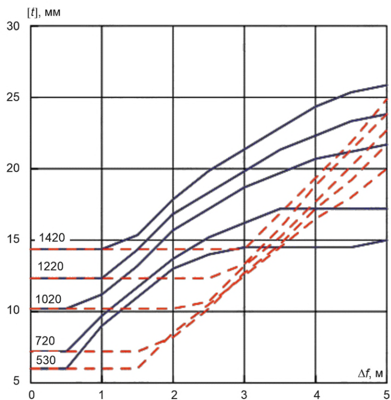
Рисунок В.33 — Сброс, песок, К55, p = 5,4 МПа
