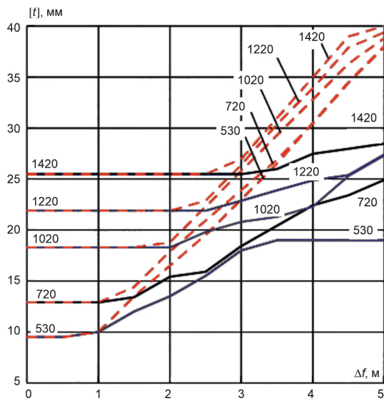
Рисунок В.63 — Сброс, глина, К70, \rho = 11,8 МПа
