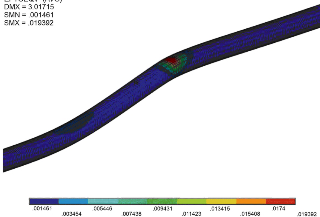
Рисунок Г.1 — Эквивалентные деформации по Мизесу в окрестности точки пересечения АТР
