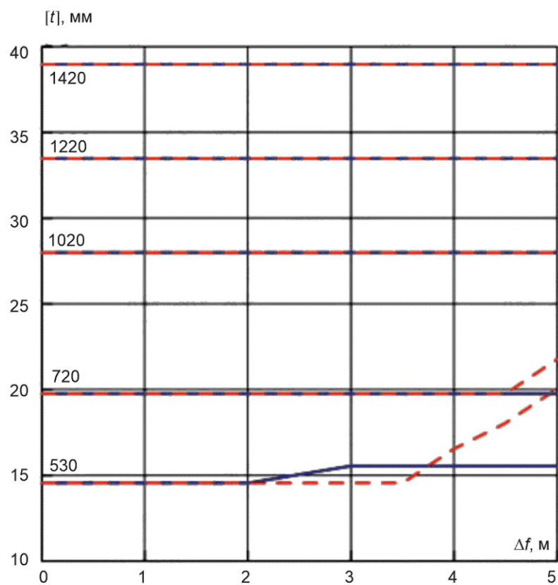
Рисунок В.35 — Сброс, песок, К55, p = 11,8 МПа
