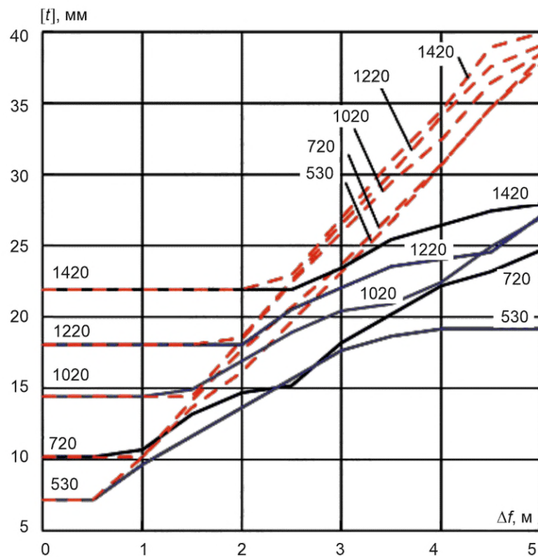
Рисунок В.62 — Сброс, глина, К70, p = 9,8 МПа
