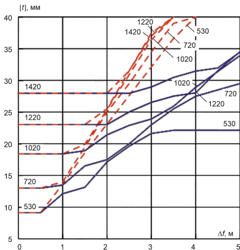
Рисунок В.50 — Сброс, глина, К55, p = 9,8 МПа
