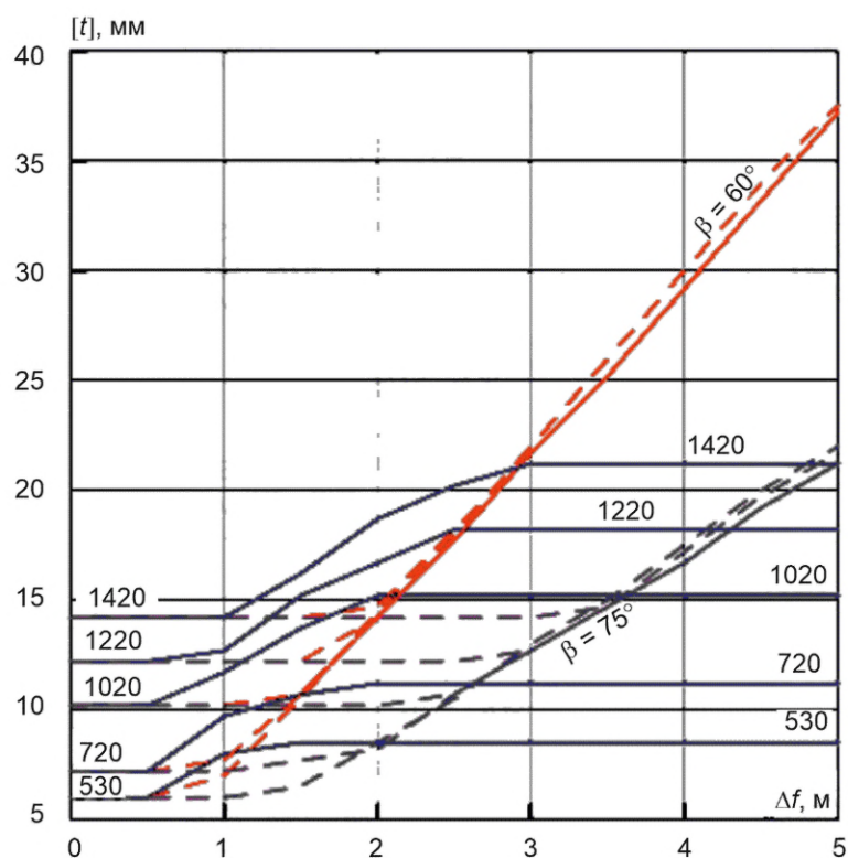
Рисунок В.29 — Сдвиг, глина, К70, p = 5,4 МПа
