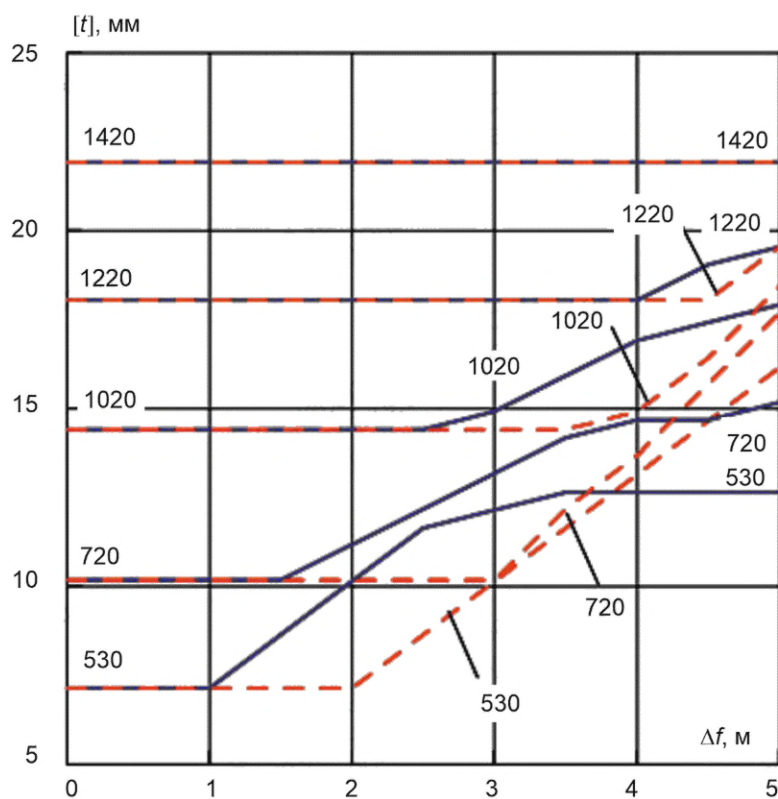
Рисунок В.46 — Сброс, песок, K70, p = 9,8 МПа
