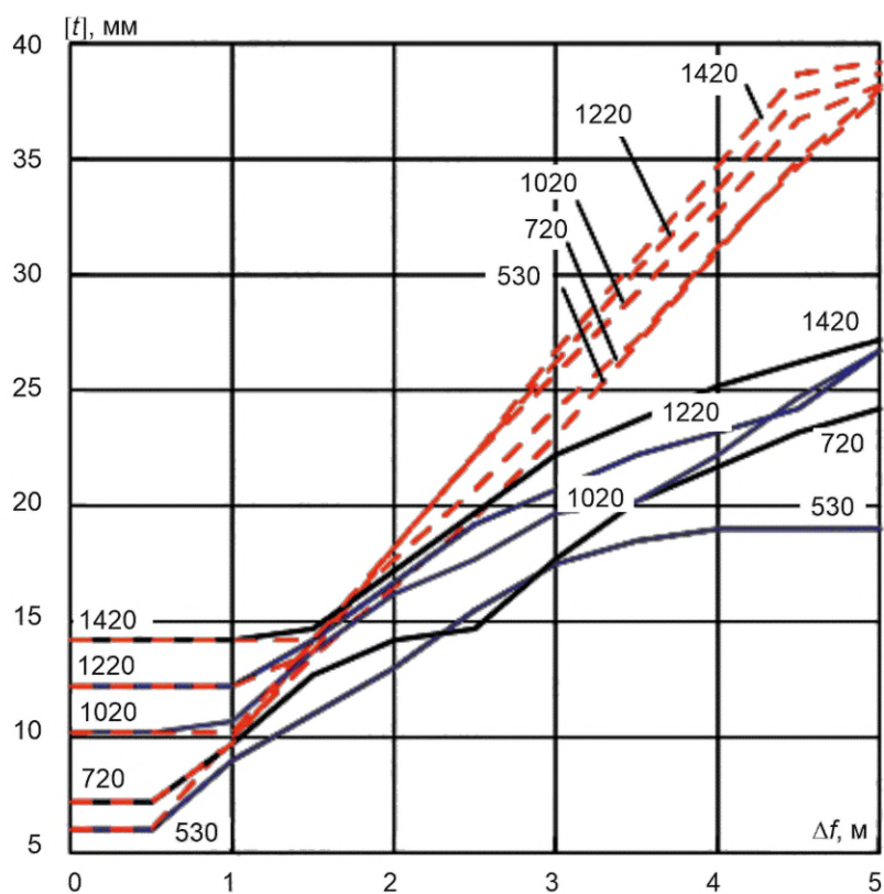
Рисунок В.61 — Сброс, глина, K70, p = 5,4 МПа
