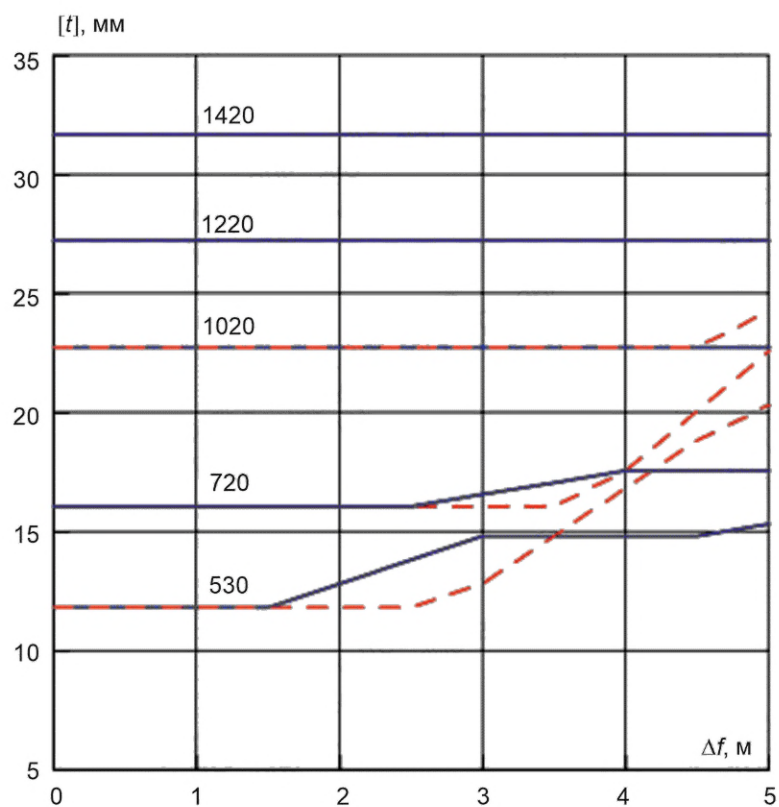
Рисунок В.39 — Сброс, песок, K60, p = 11,8 МПа
