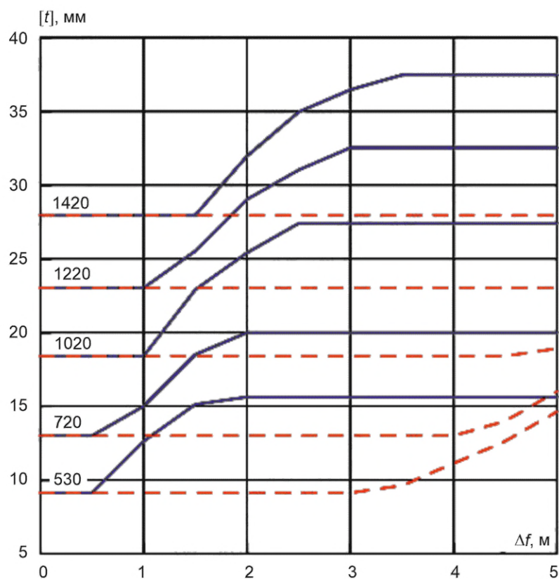
Рисунок В.2 — Сдвиг, песок, К55, p = 9,8 МПа
