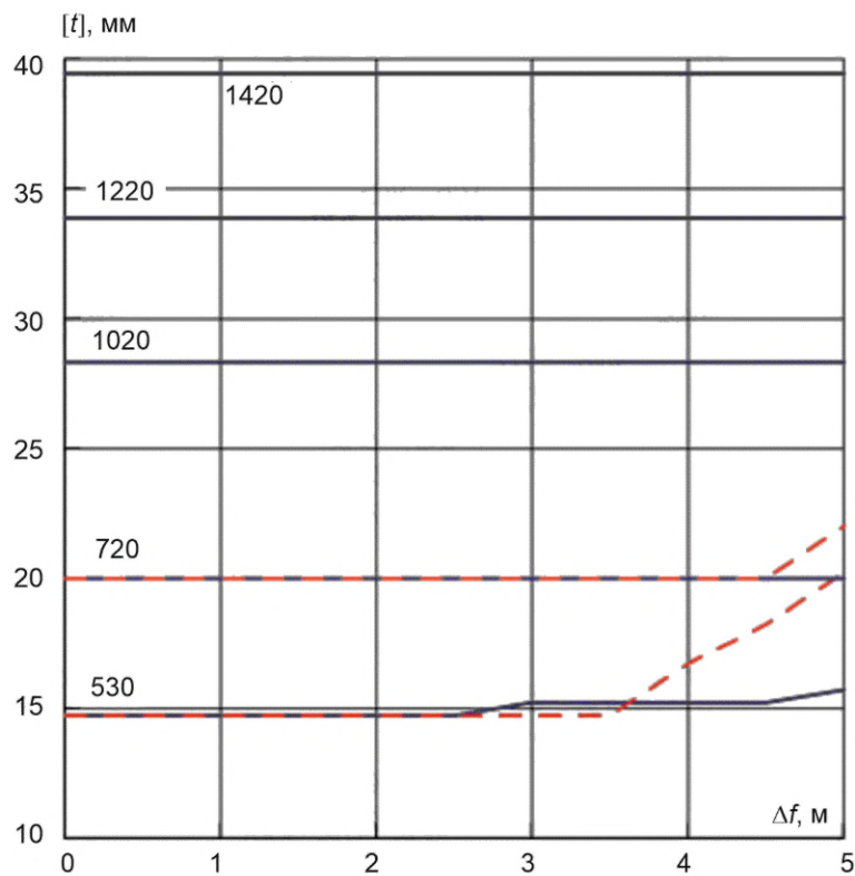
Рисунок В.40 — Сброс, песок, К60, p = 14,7 МПа
