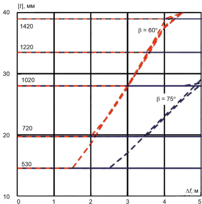
Рисунок В.19 — Сдвиг, глина, К55, p = 11,8 МПа
