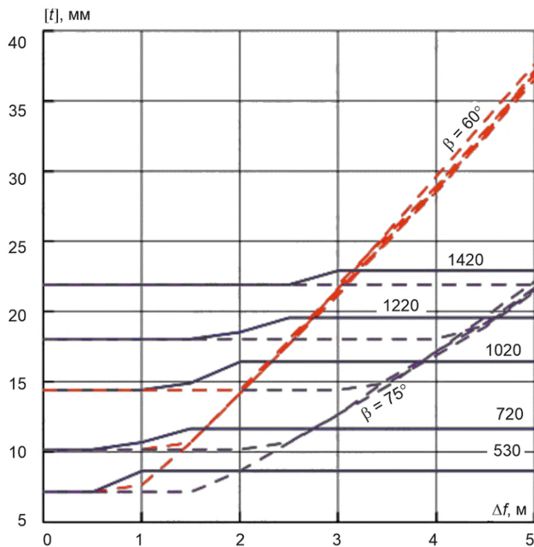
Рисунок В.30 — Сдвиг, глина, К70, p = 9,8 МПа
