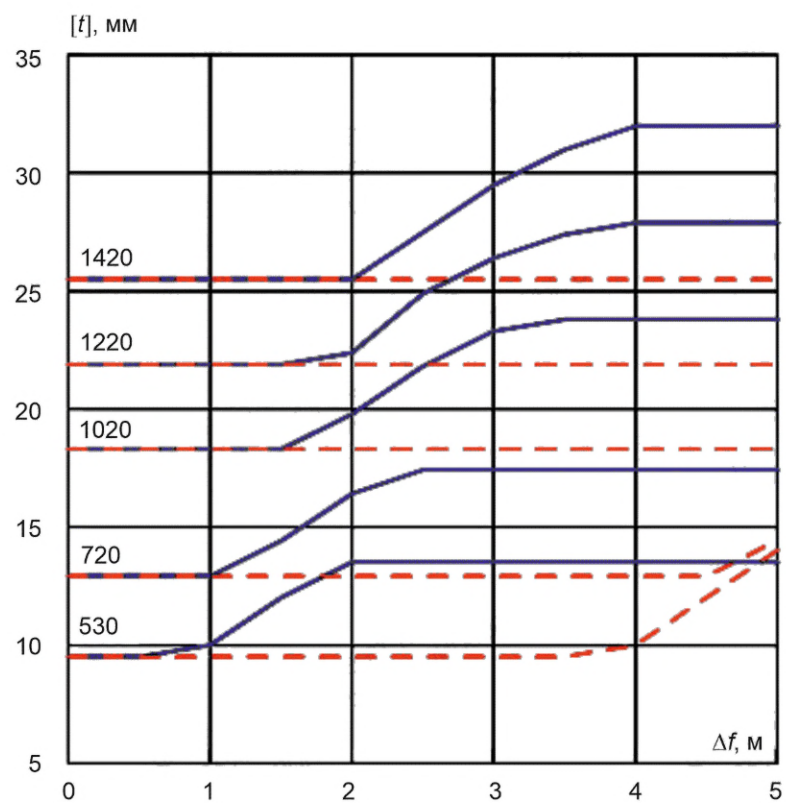
Рисунок В.15 — Сдвиг, песок, K70, p = 11,8 МПа
