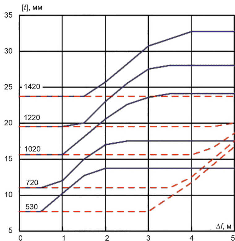
Рисунок В.10 — Сдвиг, песок, К65, p = 9,8 МПа
