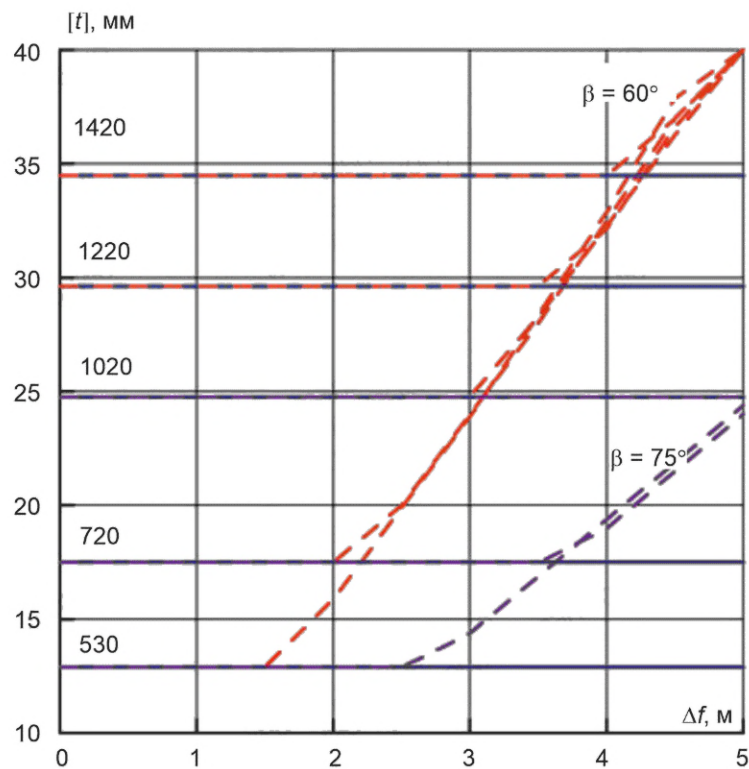
Рисунок В.28 — Сдвиг, глина, К65, p = 14,7 МПа
