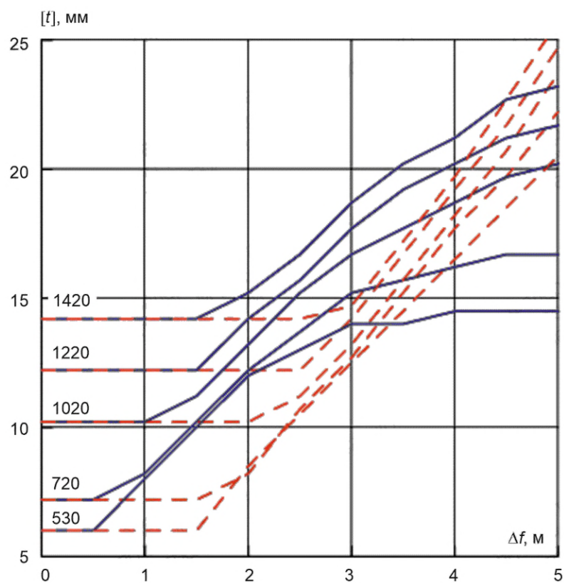
Рисунок В.37 — Сброс, песок, K60, p = 5,4 МПа
