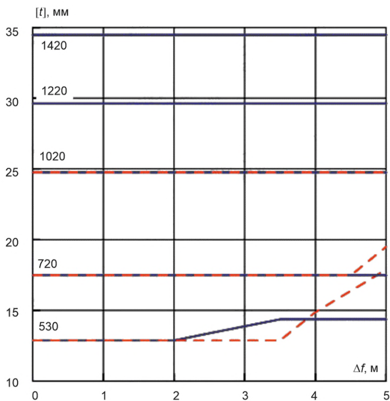
Рисунок В.44 — Сброс, песок, К65, p = 14,7 МПа
