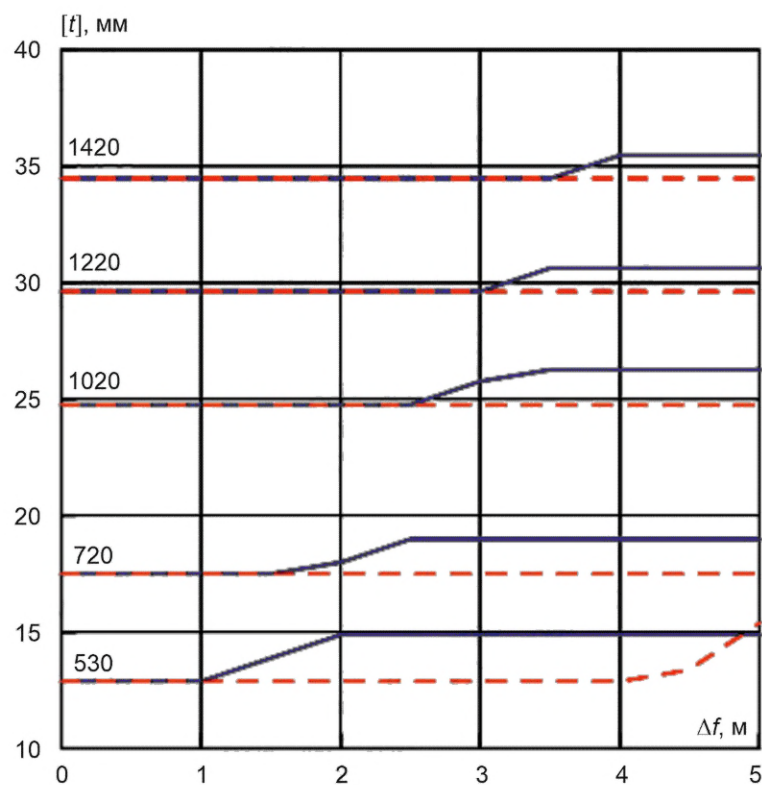
Рисунок В.12 — Сдвиг, песок, К65, \rho = 14,7 МПа
