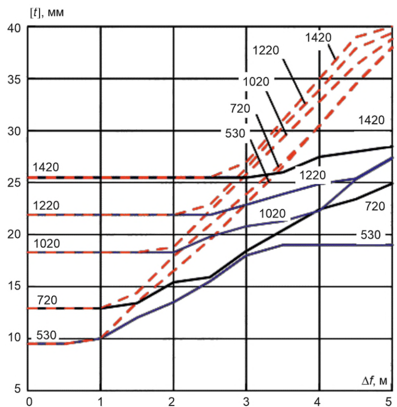
Рисунок В.55 — Сброс, глина, К60, p = 11,8 МПа
