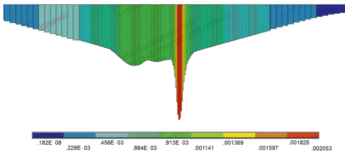
Рисунок Г.4 — Распределение продольных осевых деформаций на участке протяженностью 200 м
