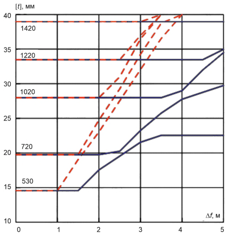
Рисунок В.51 — Сброс, глина, К55, p = 11,8 МПа
