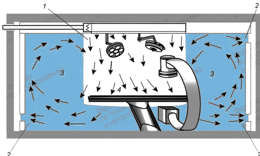
1 — воздухоораспределитель однонаправленного потока (операционный потолок чистого воздуха); 2 — вытяжные отверстия с сепараторами пуха; 3 — зона вне размещения больного; 4 — ангиографическое оборудование (рабочая зона)
