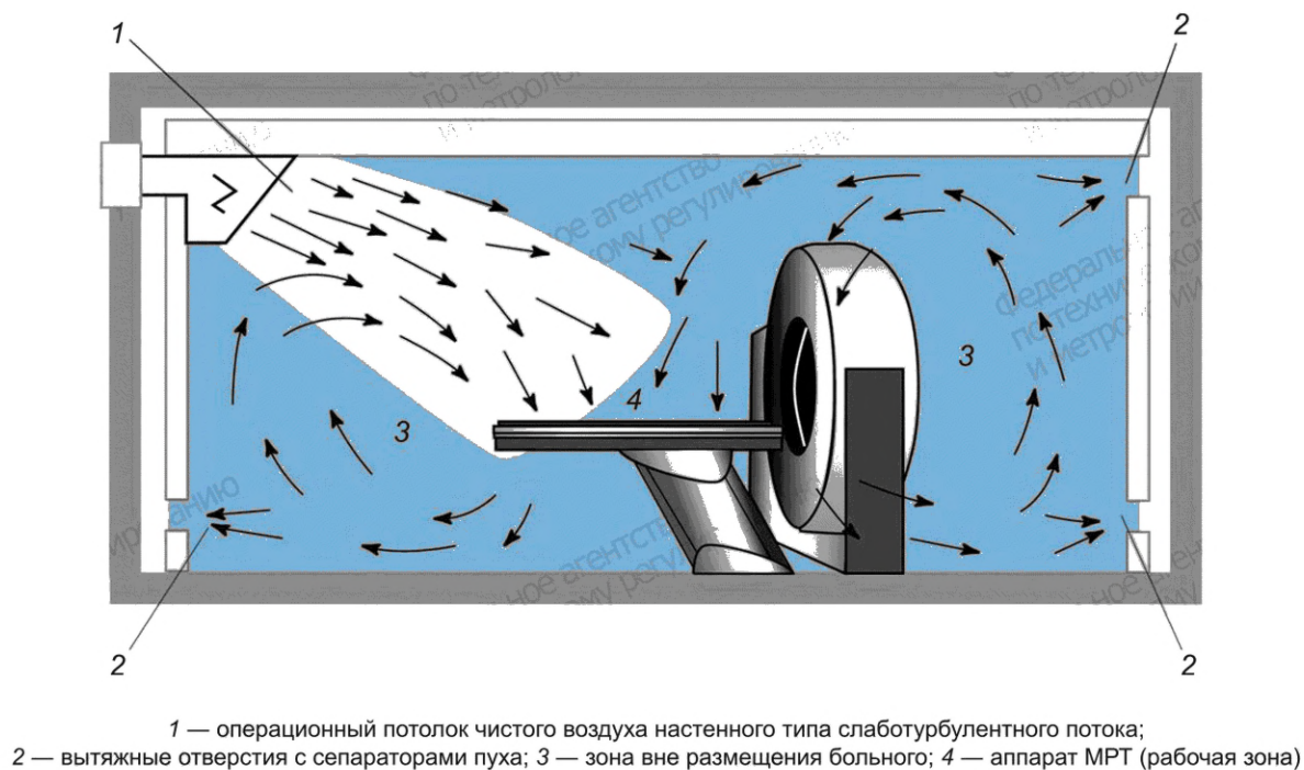
Рисунок 21 — Организация распределения воздуха в кабинете МРТ
