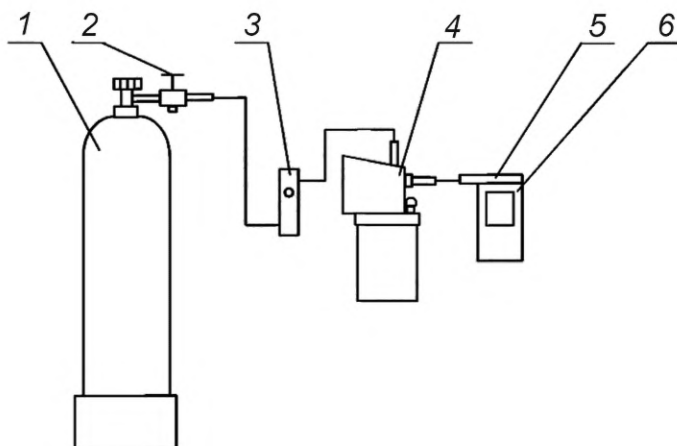
1 — баллон с азотом (воздухом); 2 — вентиль; 3 — ротаметр; 4 — генератор; 5 — мундштук; 6 — индикатор (анализатор)
