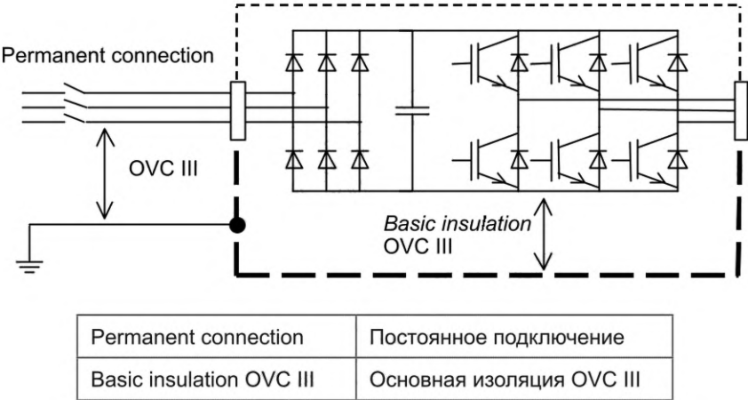
Рисунок В.2 — Оценка основной изоляции для цепей, подключенных напрямую к питающей сети
