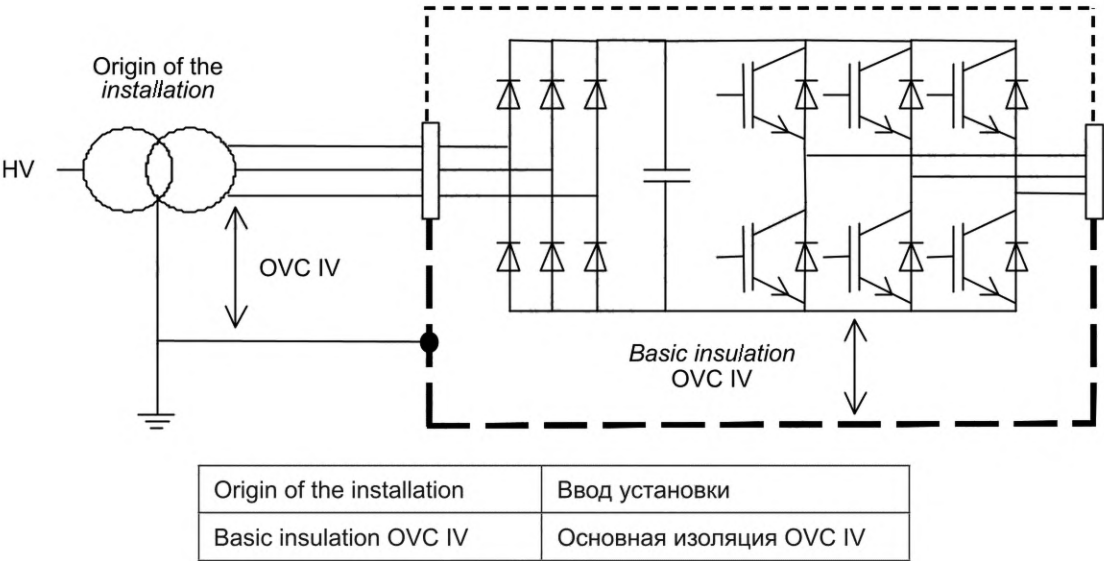
Рисунок В.1 — Оценка основной изоляции для цепей, подключенных напрямую к вводу в установку от питающей сети
