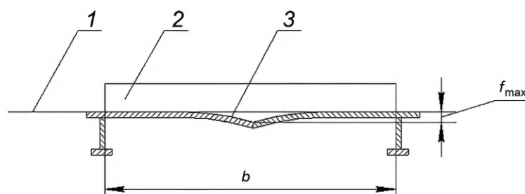
1 — номинальная поверхность; 2 — линейка; 3 — реальная поверхность; f_{\max} — максимальная стрелка прогиба; b — базовый размер
