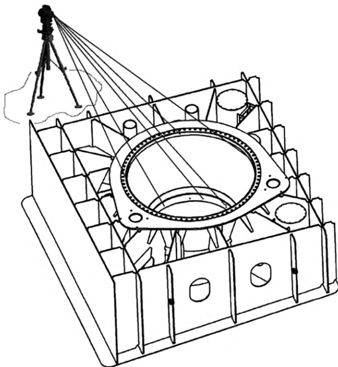
Рисунок В.3 — Определение геометрических параметров внутренней полости специализированного фундамента
