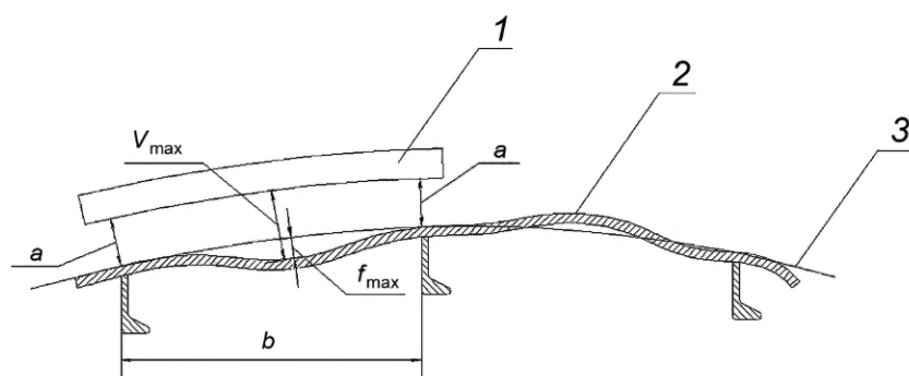
1 — шаблон; 2 — реальная поверхность; 3 — номинальная поверхность; a — расстояние от шаблона до номинальной поверхности; V_{\max} — максимальный зазор между шаблоном и реальной поверхностью; f_{\max} — максимальная стрелка прогиба; b — базовый размер
