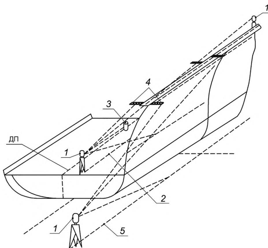
1 — теодолит; 2 — контрольные батоксы; 3 — риски горизонтальной базовой линии; 4 — марки; 5 — линия, параллельная ДП
