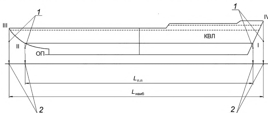
Рисунок А.13 — Проверка размеров корпуса судна по длине
