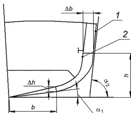
1 — теоретический обвод; 2 — фактический обвод
