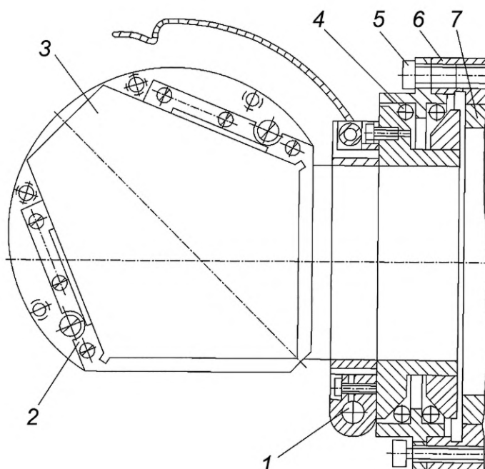
1 — петля; 2 — корпус; 3 — пентапризма; 4 — подшипник; 5 — регулировочный винт; 6 — хомут; 7 — труба теодолита
