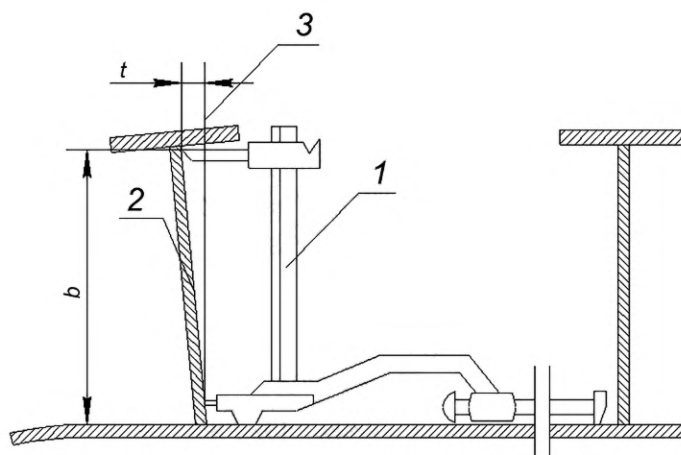
1 — угломер; 2 — реальная поверхность; 3 — номинальная поверхность; t — перекос между стенкой набора и обшивкой (настилом); b — базовый размер
