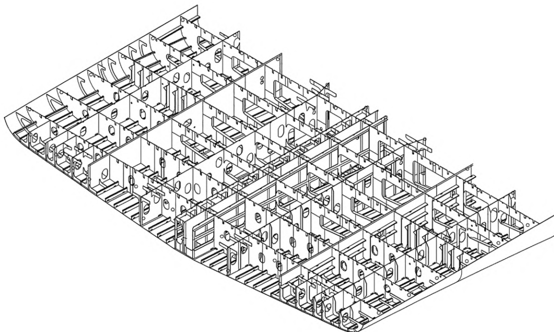
Рисунок А.18 — Объемная модель корпусной секции
