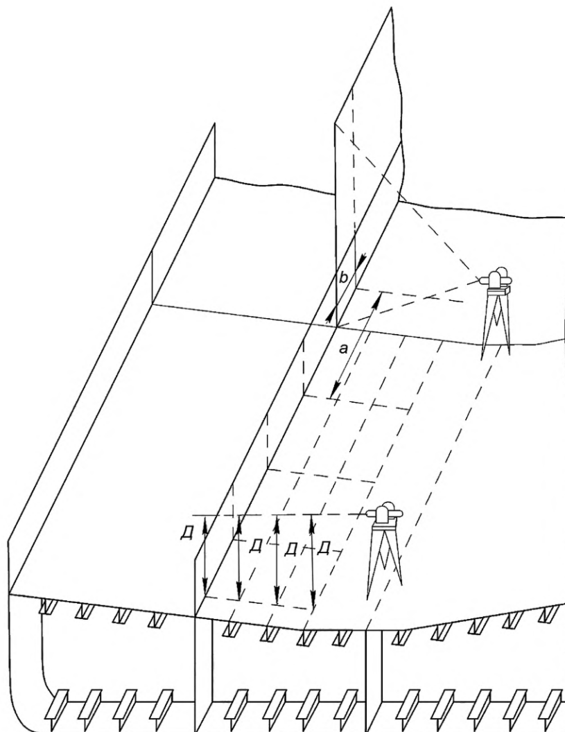
Рисунок А.22 — Снятие размеров для контуровки секции продольной переборки
