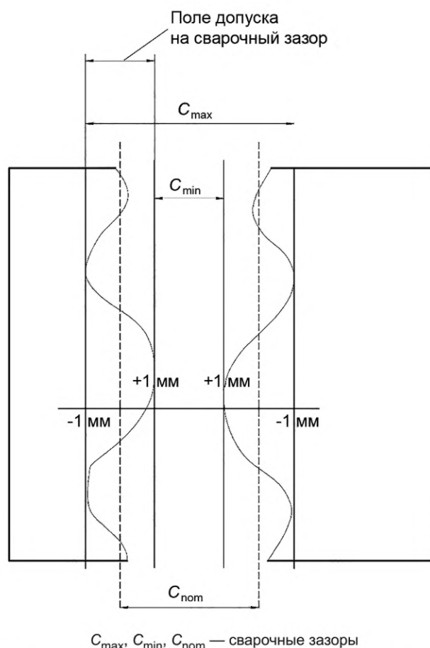
Рисунок А.15 — Анализ параметров сварочного зазора
