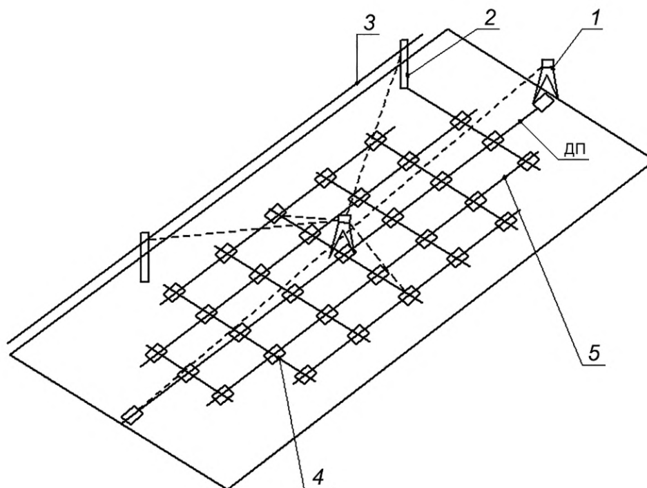
1 — теодолит (тахеометр); 2 — стойка; 3 — горизонтальная базовая линия; 4 — линия, перпендикулярная ДП; 5 — батокс
