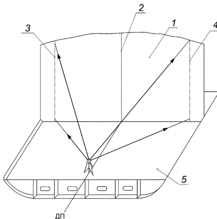
1 — поперечная переборка; 2 — средняя КЛ; 3, 4 — боковые КЛ; 5 — настил второго дна
