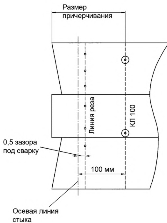
Рисунок А.19 — Схема нанесения линий причерчивания
