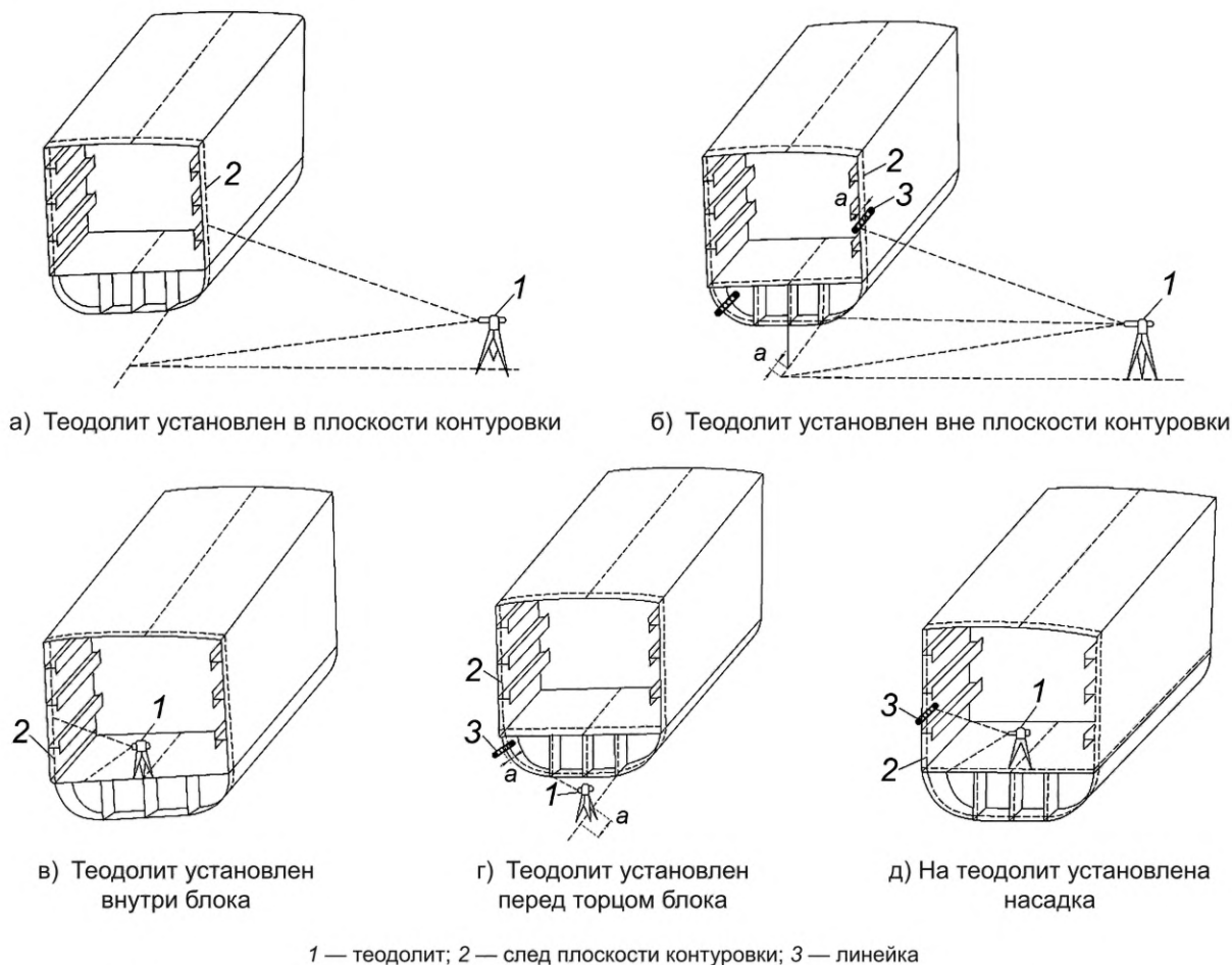
Рисунок А.24 — Варианты нанесения плоскости контуровки монтажных стыков блоков
