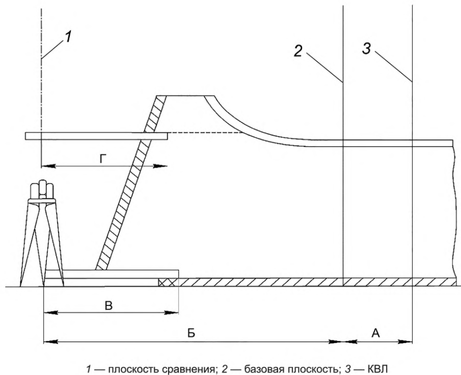
Рисунок А.23 — Контуровка секции продольной переборки
