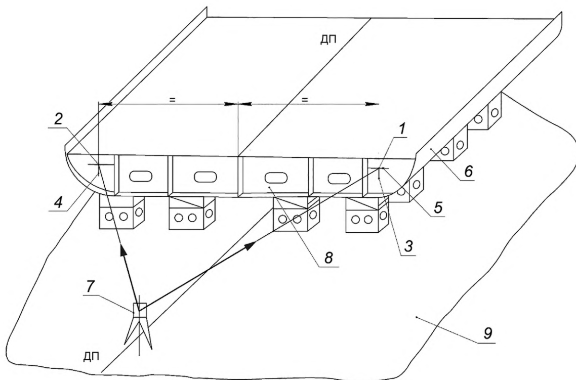
1, 2 — симметричные контрольные точки; 3, 4 — вертикальные КЛ; 5 — горизонтальная КЛ; 6 — днищевая секция; 7 — теодолит; 8 — крайний флор днищевой секции; 9 — ступельная плита
