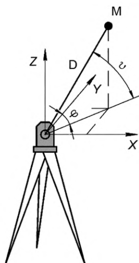
Рисунок А.14 — Линейно-угловая система измерения координат объективно выбранных линий стапеля и точек конструкций секций, строящихся на стапеле
