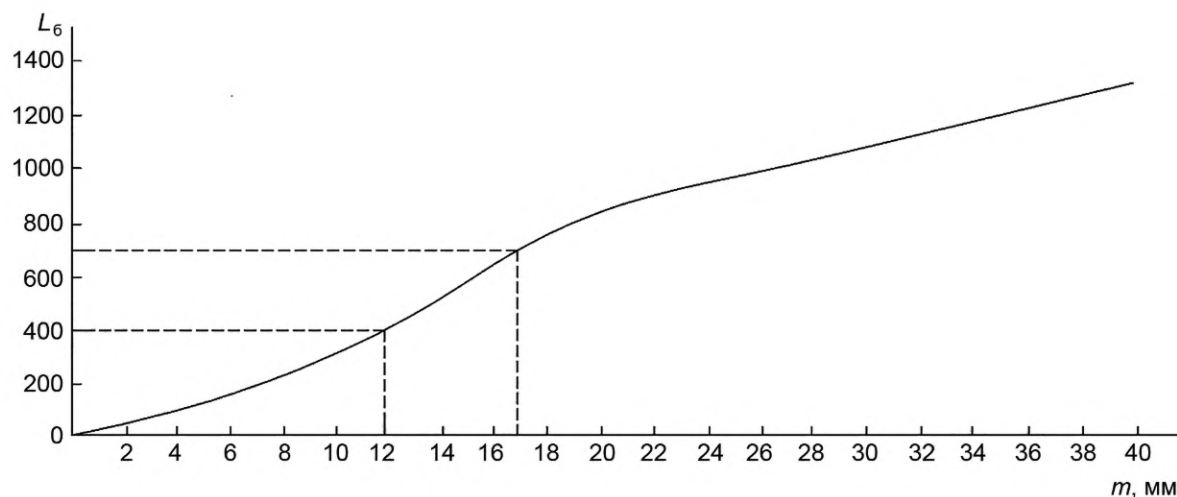
Рисунок В.2 — График зависимости длины свободного от сварки участка балки от размера несовпадения оснований смежных блоков
