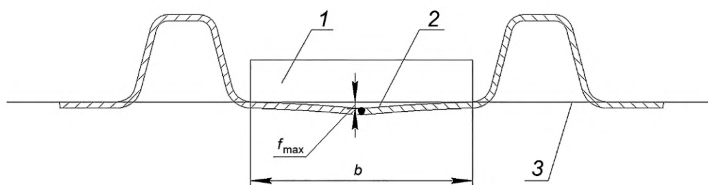
1 — линейка; 2 — реальная поверхность; 3 — номинальная поверхность; f_{\max} — максимальная стрелка прогиба; b — базовый размер
