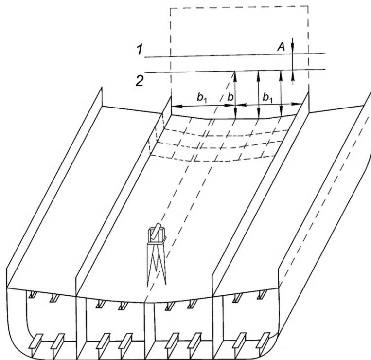
1 — КВЛ; 2 — базовая плоскость
