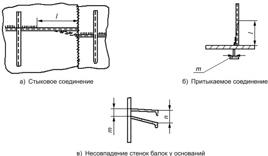
Рисунок В.1 — Несовпадение балок на монтажных соединениях
