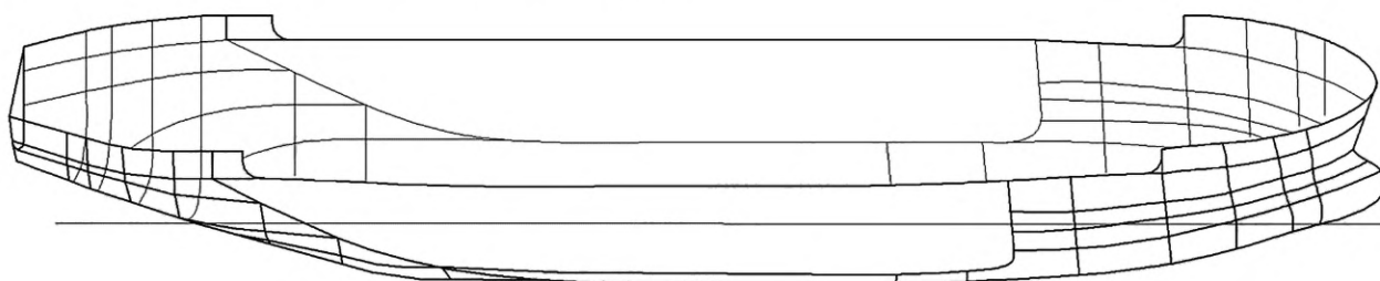
Рисунок А.17 — Каркасная пространственная модель корпуса судна
