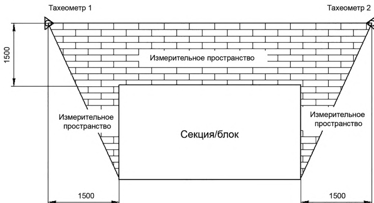
Рисунок А.16 — Схема создания измерительного пространства
