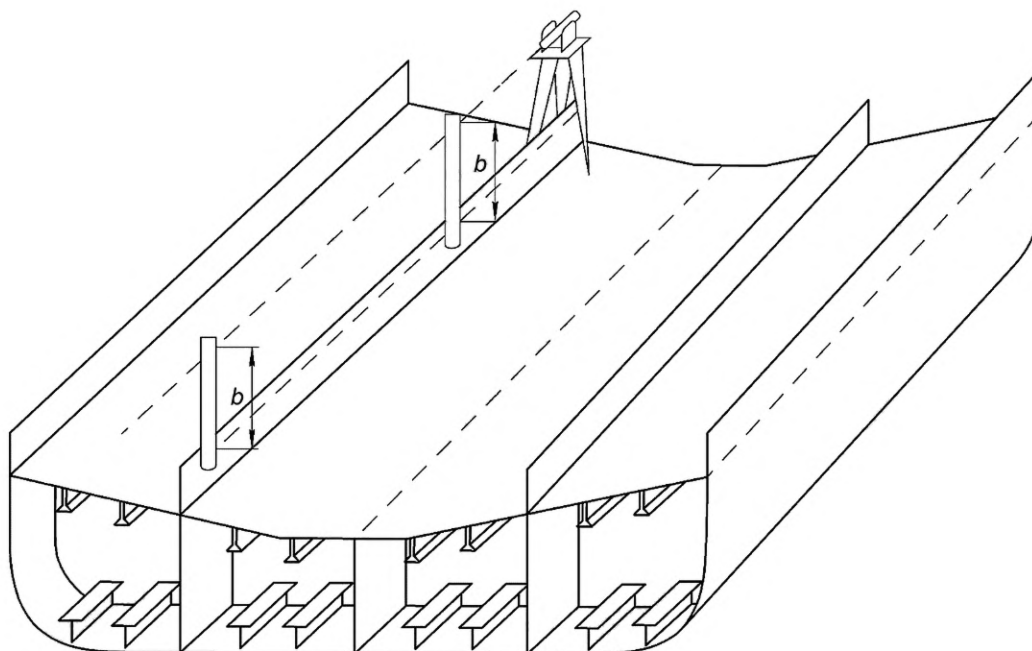
Рисунок А.21 — Контуровка комингса продольной переборки
