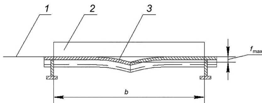
1 — номинальная поверхность; 2 — линейка; 3 — реальная поверхность; f_{\max} — максимальная стрелка прогиба; b — базовый размер
