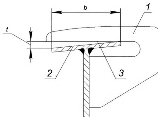
1 — малка; 2 — реальная поверхность; 3 — номинальная поверхность; t — перекос между пояском и стенкой набора; b — базовый размер
