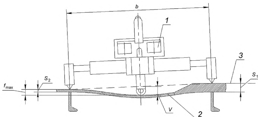
Рисунок 7 — Схема измерения стрелок прогиба обшивки (настила) в районе разных толщин с использованием рейки
