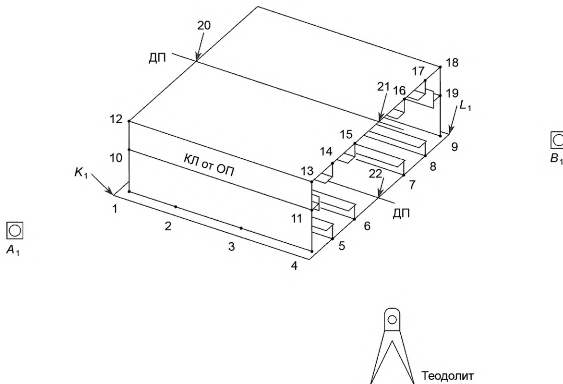
Рисунок А.26 — Схема расположения используемых баз, контролируемых точек и расположения используемого тахеометра или электронного теодолита
