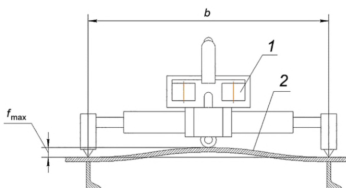
1 — бухтиномер; 2 — реальная поверхность; f_{\max} — максимальная стрелка прогиба; b — базовый размер
