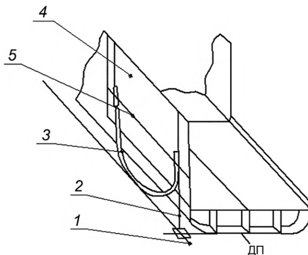
1 — базовая линия батокса; 2 — отвес; 3 — шланговый уровень; 4 — секция борта; 5 — КЛ
