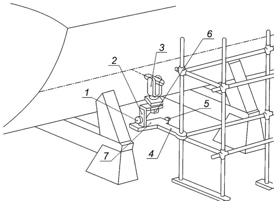
1 — маховик подъемной стойки; 2 — подъемная стойка; 3 — теодолит; 4 — кронштейн; 5 — установочный винт; 6 — стеновой винт; 7 — опорная площадка кронштейна
