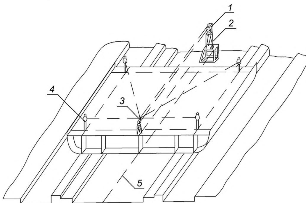
1 — излучатель; 2 — штатив; 3 — блок пентапризм; 4 — целевой знак; 5 — линия ДП, нанесенная на стапеле и на секции
