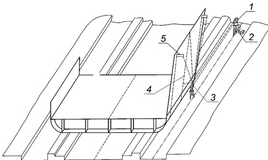
1 — излучатель; 2 — штатив; 3 — блок призм; 4 — линия контрольного шпангоута; 5 — целевой знак
