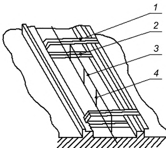
1 — рама; 2 — шергень; 3 — струна; 4 — отвес
