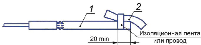
1 — устройство НСИ-Ш; 2 — инициируемый детонирующий шнур
