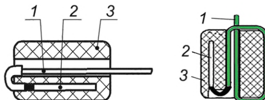
1 — волновод устройства; 2 — капсюль-детонатор с замедлением; 3 — шашка
