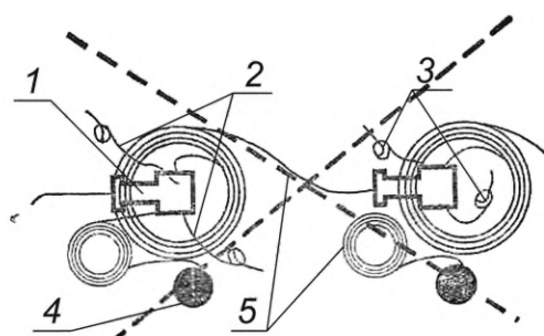
1 — монтажный соединитель; 2 — пассивная часть волновода; 3 — узел фиксирующий на пассивной части волновода; 4 — скважина; 5 — активная часть волновода
