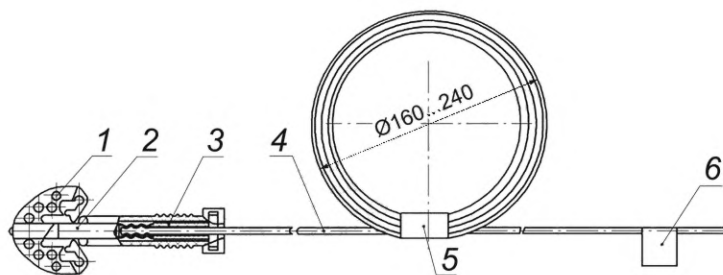
1 — монтажный соединитель (вариант исполнения); 2 — капсюль-детонатор с замедлением; 3 — втулка; 4 — волновод; 5 — бандероль; 6 — этикетка
