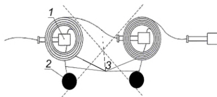
1 — монтажный соединитель; 2 — скважина; 3 — активная часть волновода
