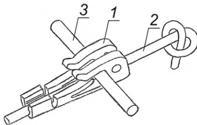
Рисунок В.4 — Схема инициирования устройств НСИ-Ш от детонирующего шнура с использованием соединителя
