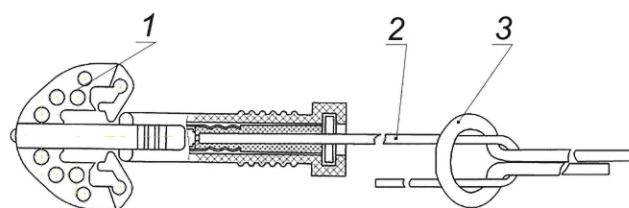
1 — монтажный соединитель; 2 — волновод; 3 — детонирующий шнур
