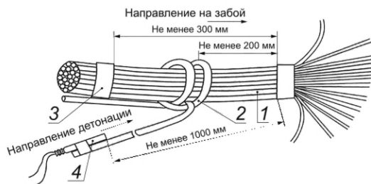
1 — волноводы иницируемых устройств; 2 — детонирующий шнур; 3 — изоляционная лента или проволока; 4 — электродетонатор
