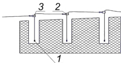
1 — капсюль-детонатор КД-С устройства НСИ-ПС; 2 — капсюль-детонатор КД-П устройства НСИ-ПС; 3 — устройство НСИ-Старт-В или НСИ-Старт-ВШ
