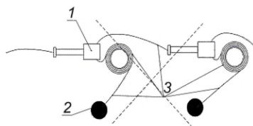
1 — монтажный соединитель; 2 — скважина; 3 — активная часть волновода
