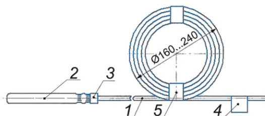
1 — волновод; 2 — капсюль-детонатор с замедлением; 3 — втулка короткая; 4 — этикетка; 5 — бандероль
