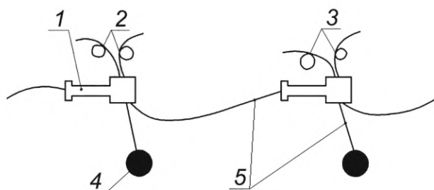
1 — монтажный соединитель; 2 — пассивная часть волноводов; 3 — узел фиксирующий на пассивной части волноводов; 4 — скважина; 5 — активная часть волноводов
