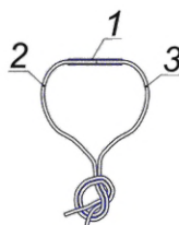
1 — втулка соединительная или отрезок трубки силиконовой; 2 — волновод устройств НСИ-Старт; 3 — ударно-волновая трубка (волновод)
