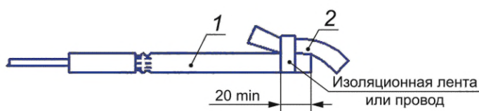
1 — устройство НСИ-С; 2 — инициируемый детонирующий шнур
