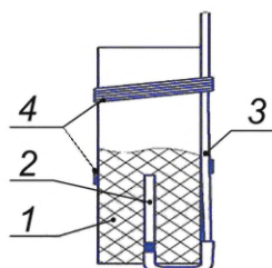
Рисунок Д.4 — Схема инициирования патрона капсюлечувствительного эмульсионного ВВ
