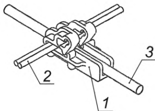
1 — соединитель; 2 — волновод иницируемого устройства; 3 — детонирующий шнур
