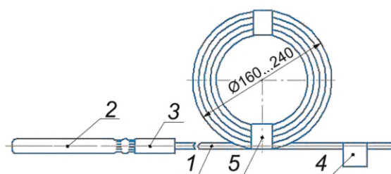
1 — волновод; 2 — капсюль-детонатор с замедлением; 3 — втулка; 4 — этикетка; 5 — бандероль
