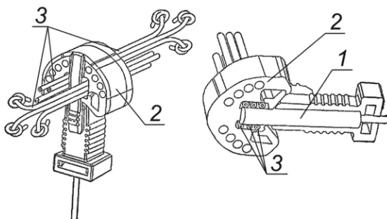
1 — капсюль-детонатор с замедлением КД-П; 2 — монтажный соединитель (пример исполнения); 3 — волноводы иницируемых устройств
