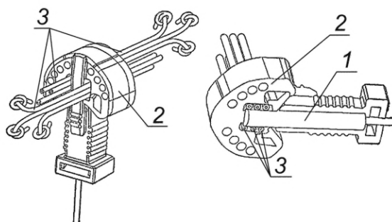
1 — капсюль-детонатор с замедлением инициирующего устройства; 2 — монтажный соединитель, 3 — волноводы инициируемых устройств
