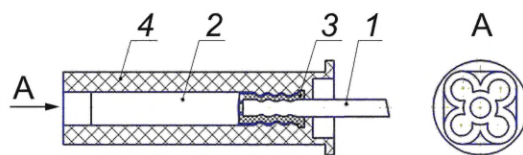
1 — волновод; 2 — капсюль-детонатор; 3 — втулка; 4 — соединитель для детонирующих шнуров (вариант исполнения)
