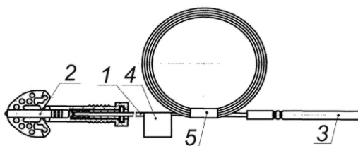
1 — волновод; 2 — монтажный соединитель (вариант исполнения) с капсюлем-детонатором КД-П; 3 — капсюль-детонатор Д-С; 4 — этикетка; 5 — бандероль
