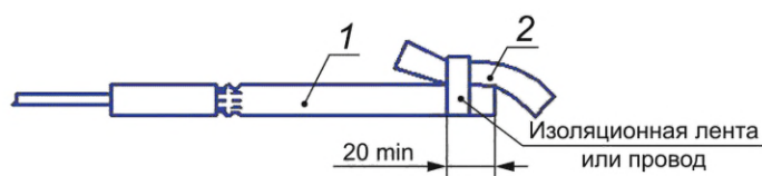
1 — устройство НСИ-С; 2 — инициируемый детонирующий шнур
