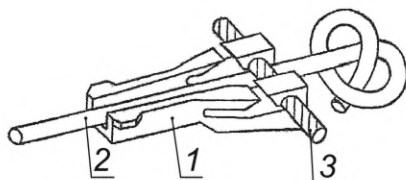
1 — соединитель; 2 — волновод иницируемого устройства; 3 — детонирующий шнур
