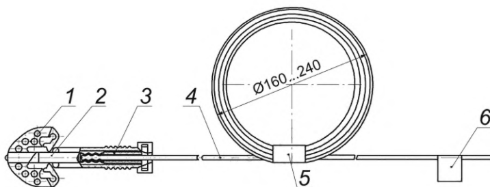
1 — монтажный соединитель (пример исполнения); 2 — капсюль-детонатор с замедлением; 3 — втулка; 4 — волновод; 5 — бандероль; 6 — этикетка
