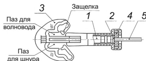
1 — капсюль-детонатор; 2 — втулка; 3 — соединитель (пример исполнения); 4 — стопорная вилка монтажного соединителя; 5 — волновод
