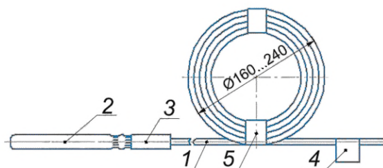
1 — волновод; 2 — капсюль-детонатор с замедлением; 3 — втулка соединительная; 4 — этикетка; 5 — бандероль
