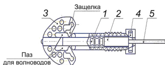
1 — капсюль-детонатор; 2 — втулка; 3 — монтажный соединитель (пример исполнения); 4 — стопорная вилка монтажного соединителя; 5 — волновод
