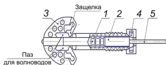
1 — капсюль-детонатор; 2 — втулка; 3 — монтажный соединитель для волновода (вариант исполнения); 4 — стопорная вилка монтажного соединителя; 5 — волновод
