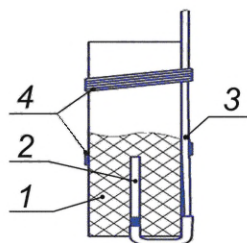
1 — патрон ВВ; 2 — капсюль-детонатор; 3 — волновод устройства; 4 — шпагат, лента клейкая
