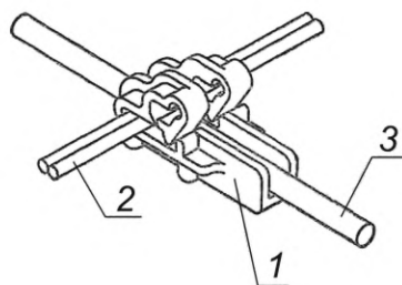
Рисунок В.5 — Схема инициирования устройств НСИ-Ш от детонирующего шнура с использованием соединителя
