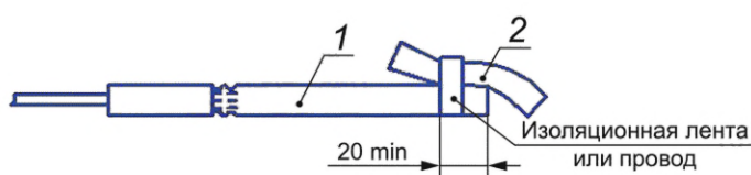
1 — устройство НСИ-Ш; 2 — иницируемый детонирующий шнур
