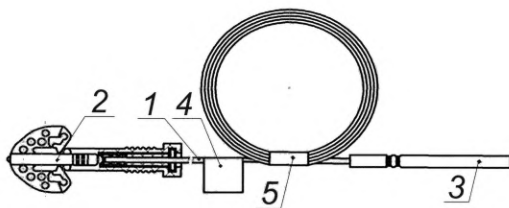
1 — волновод; 2 — монтажный соединитель с капсюлем-детонатором КД-П; 3 — капсюль-детонатор КД-С; 4 — этикетка; 5 — бандероль
