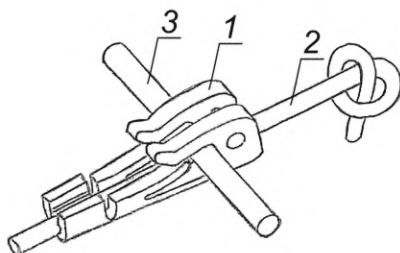
Рисунок 7 — Схема инициирования устройств НСИ от детонирующего шнура с использованием соединителя (вариант исполнения)
