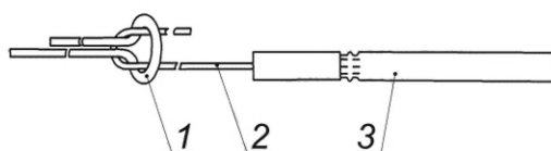
1 — иницирующий детонирующий шнур; 2 — волновод устройства; 3 — капсюль-детонатор с замедлением
