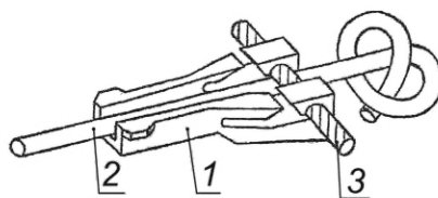
1 — соединитель; 2 — волновод инициируемого устройства; 3 — детонирующий шнур
