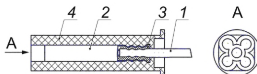
1 — волновод; 2 — капсюль-детонатор; 3 — втулка; 4 — соединитель (пример исполнения)
