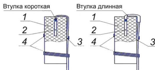
1 — патрон ВВ; 2 — капсюль-детонатор с замедлением; 3 — волновод устройства; 4 — проволока или шпагат, или изоляционная лента
