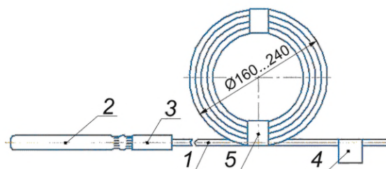
1 — волновод; 2 — капсюль-детонатор с замедлением; 3 — втулка длинная; 4 — этикетка; 5 — бандероль
