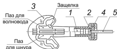
1 — капсюль-детонатор; 2 — втулка; 3 — соединитель универсальный (вариант исполнения); 4 — стопорная вилка монтажного соединителя; 5 — волновод
