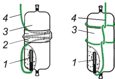
1 — капсюль-детонатор устройства НСИ-С; 2 — скотч; 3 — патрон капсюлечувствительного эмульсионного ВВ; 4 — волновод
