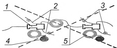
1 — монтажный соединитель; 2 — пассивная часть волновода; 3 — узел фиксирующий на пассивной части волновода; 4 — скважина; 5 — активная часть волновода
