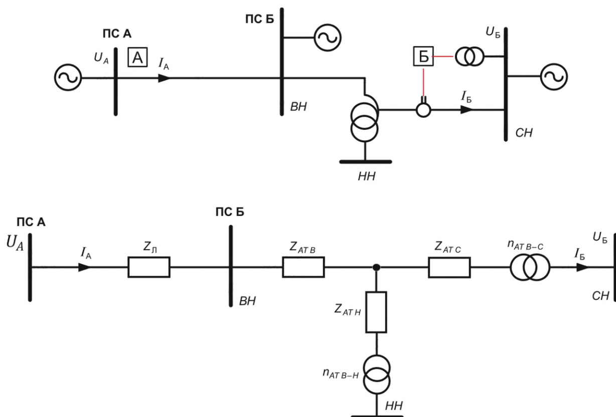
Рисунок Е.3 — Вариант схемы подключения ДЗ АТ к ТТ и ТН стороны СН
