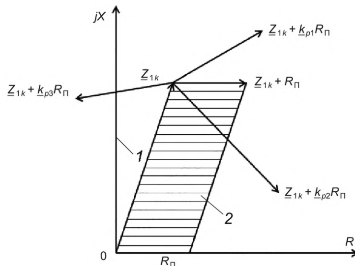
Рисунок Б.8 — Влияние доаварийного нагрузочного режима на дистанционные замеры при междуфазных КЗ через переходные сопротивления
