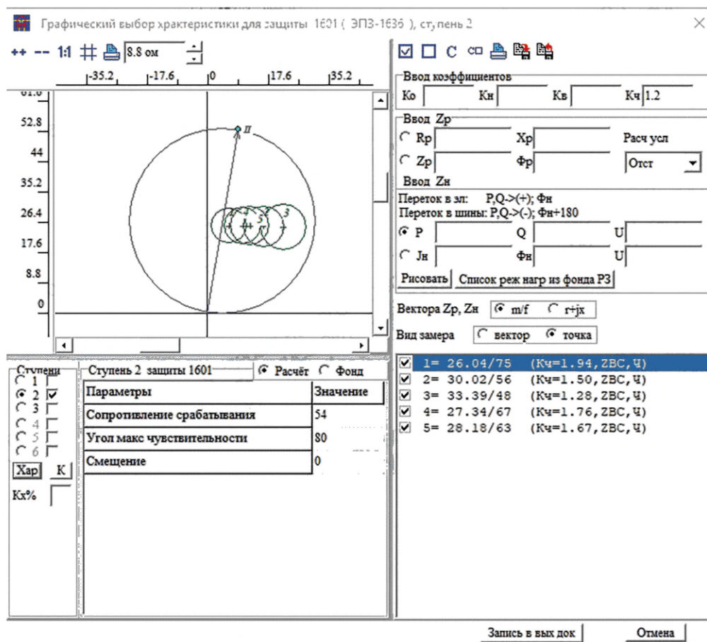
Рисунок 5.3 — Выбор круговой характеристики второй ступени ДЗ по чувствительности к междуфазным КЗ в конце ЛЭП
