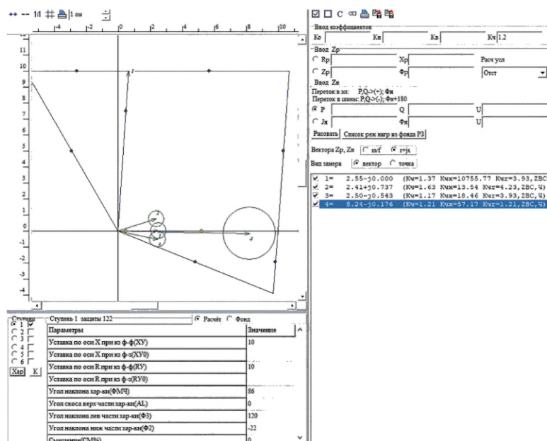
Рисунок 5.8 — Обеспечение чувствительности при КЗ в начале ЛЭП
