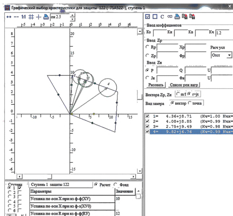
Рисунок 5.9 — Обеспечение чувствительности при КЗ в конце зоны охвата
