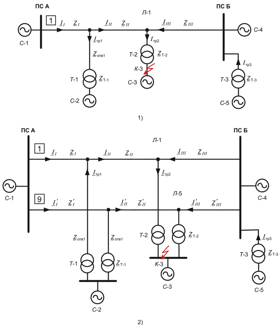
Рисунок 7.5 — Определение коэффициентов токораспределения при КЗ в точке К-3
