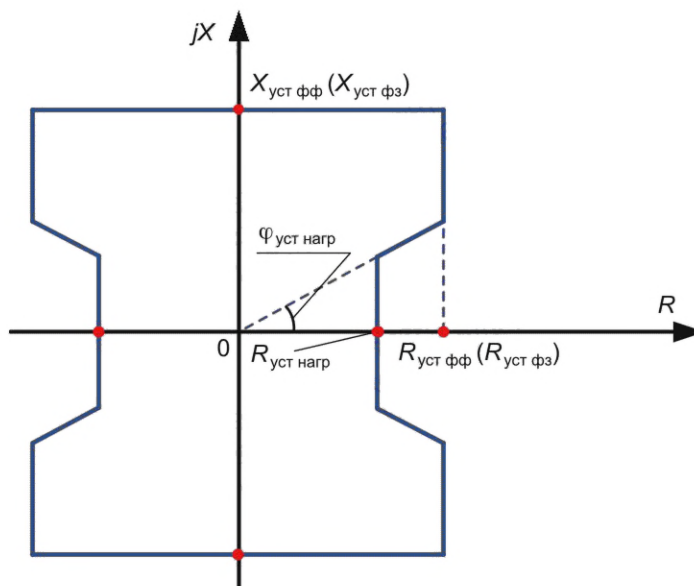
Рисунок 9.1 — Пример ненаправленной полигональной характеристики дистанционного пускового органа
