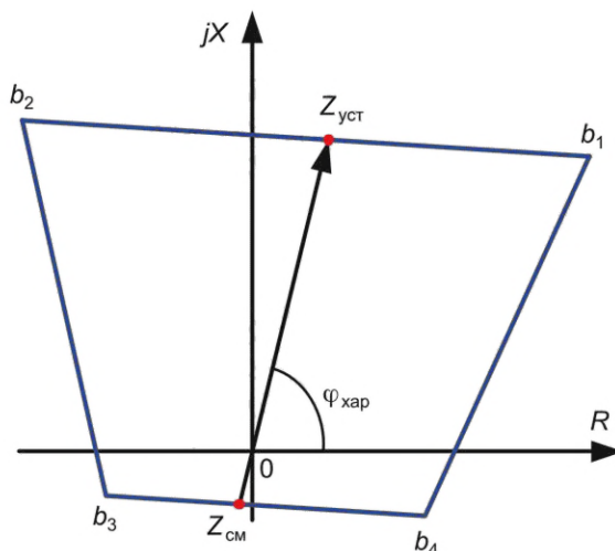
Рисунок А.2 — Пример направленной характеристики срабатывания в виде четырехугольника со смещением
