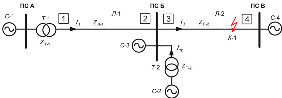
Рисунок 8.3 — Определение коэффициента токораспределения при КЗ в точке К-1
