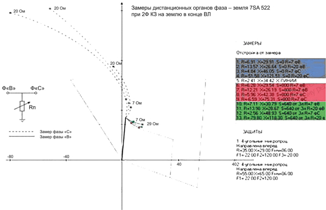
Рисунок Б.12 — Замеры Z_{B0} , Z_{C0} при двухфазном КЗ на землю BC0
