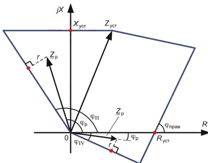
Рисунок 4.18 — Определение углов ограничения характеристики во втором и четвертом квадранте
