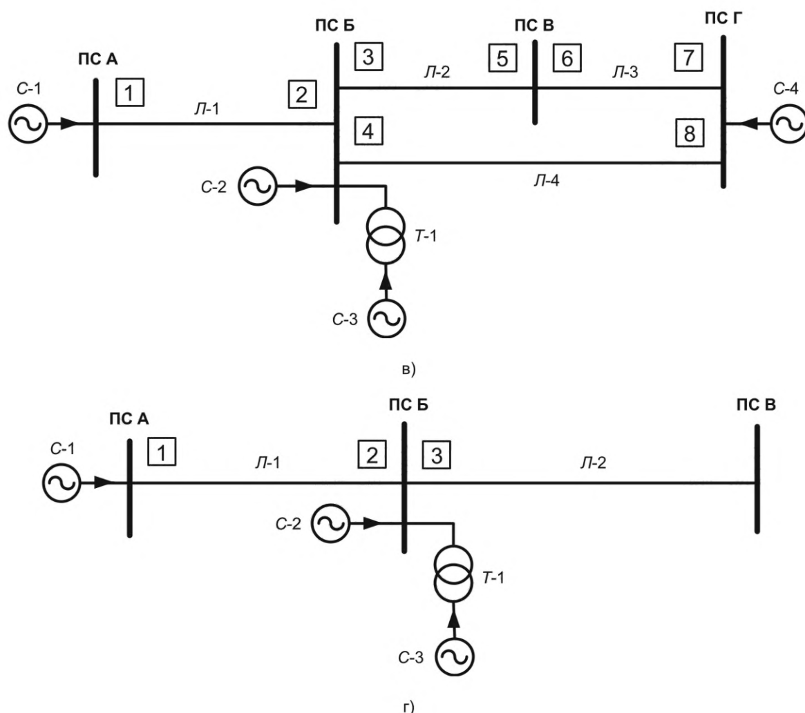
Рисунок 5.1 — Примеры типовых схем участков сети с одиночными ЛЭП с двусторонним питанием
