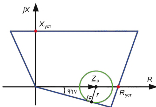
Рисунок 5.10 — Проверка чувствительности при КЗ в начале ЛЭП через переходное сопротивление
