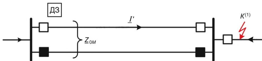
Рисунок Б.6 — Внешнее однофазное КЗ на землю A_0 для случая отключенной параллельной линии
