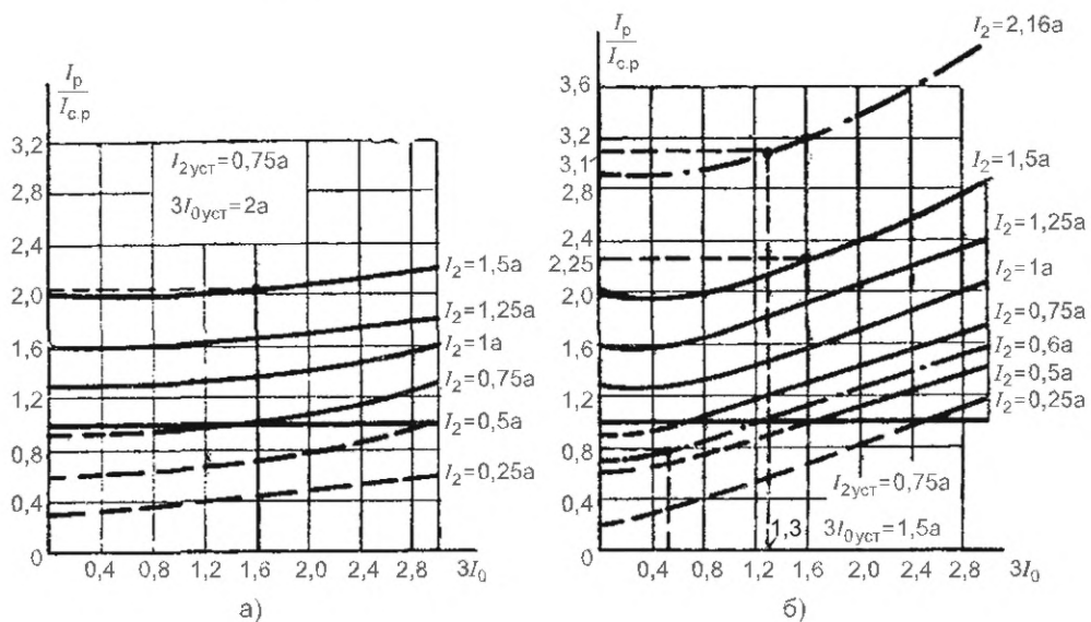
Рисунок 10.8 — Характеристики чувствительности пускового органа устройства БК типа КРБ-122
