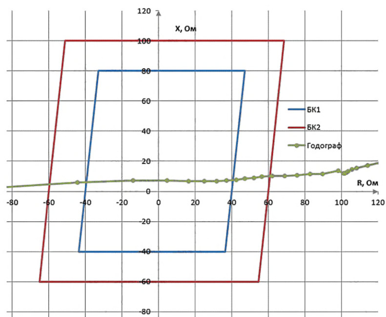
Рисунок 10.10 — Графический способ определения \Delta t_{\text{кач}}
