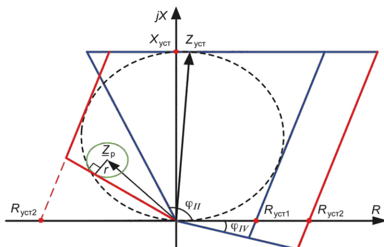
Рисунок 4.19 — Сравнительная проверка чувствительности ДО с полигональной и круговой характеристикой при КЗ в зоне дальнего резервирования
