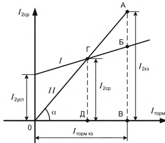
Рисунок 10.6 — Проверка чувствительности устройств БК типов КРБ-122, КРБ-124, КРБ-126
