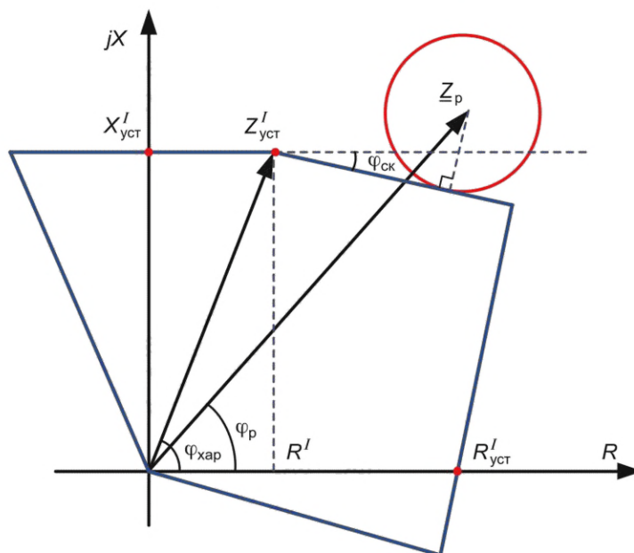
Рисунок 4.6 — Отстройка углом скоса верхней грани характеристики
