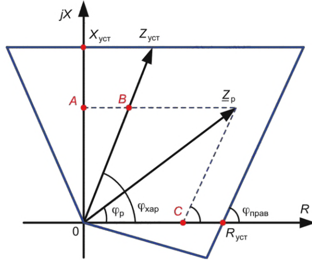
Рисунок 4.15 — Проверка чувствительности ДО с полигональной характеристикой
