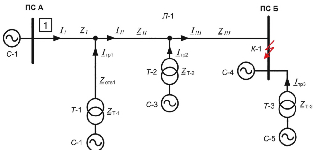
Рисунок 7.3 — Определение коэффициентов токораспределения при КЗ в точке К-1
