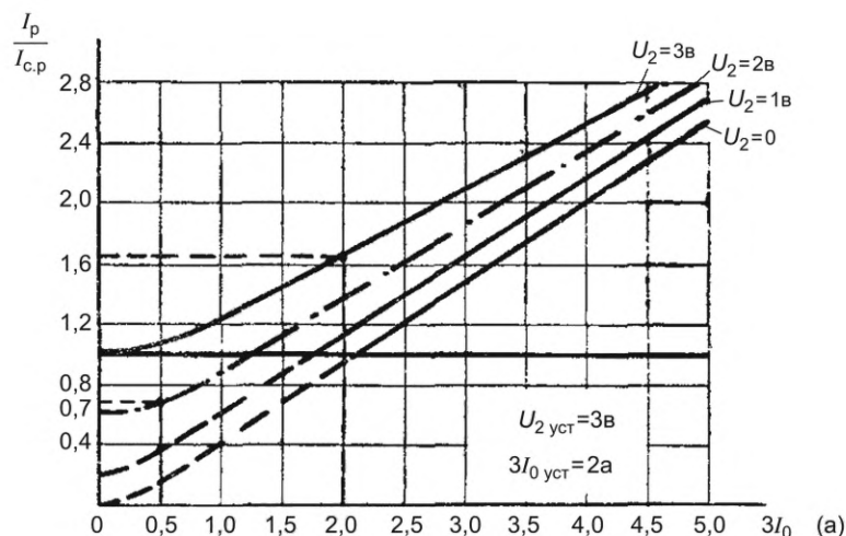
Рисунок 10.3 — Характеристики чувствительности устройства БК при качаниях типа КРБ-121
