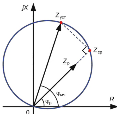
Рисунок 4.10 — Проверка чувствительности ДО с направленной круговой характеристикой, проходящей через начало координат
