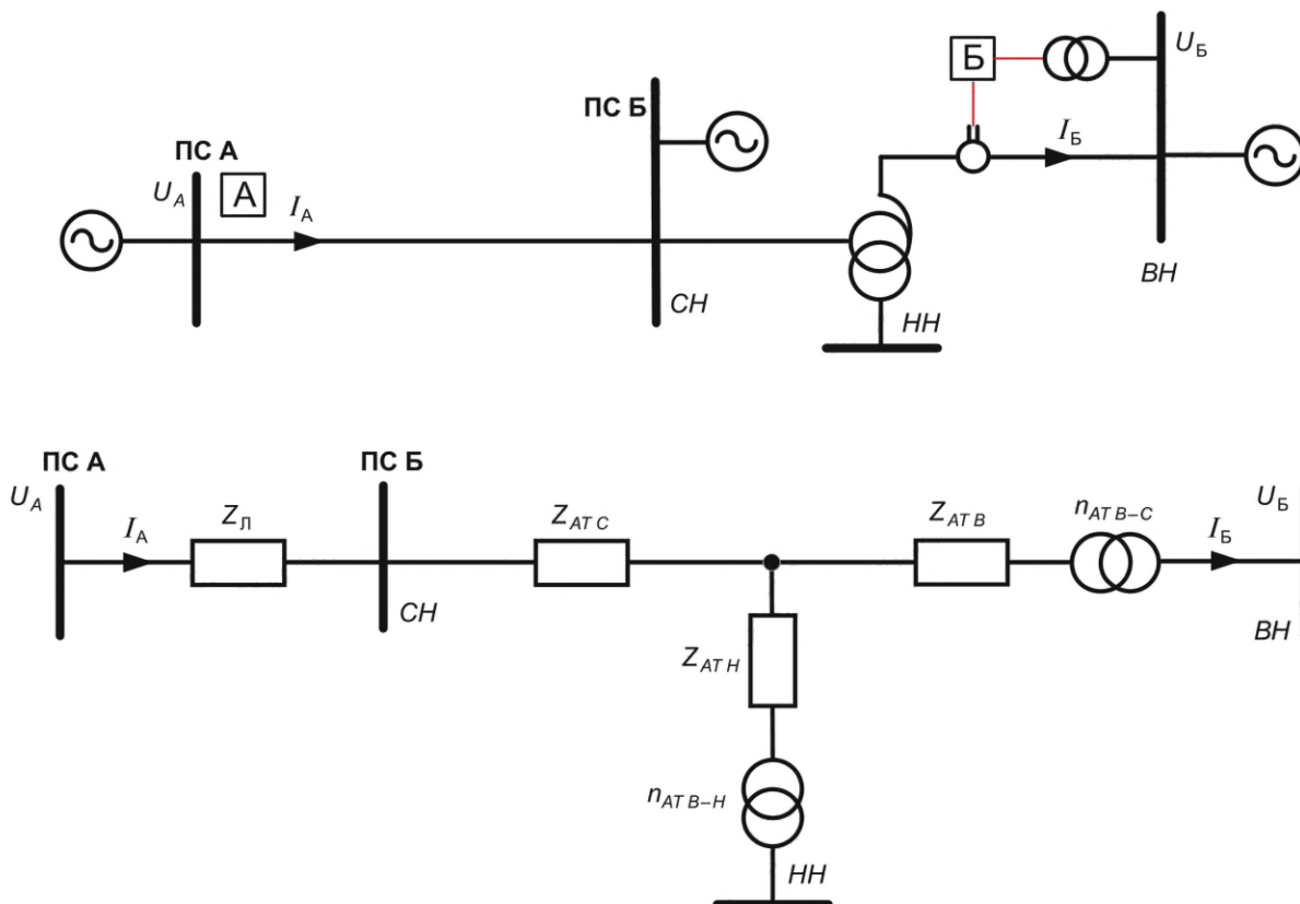
Рисунок Е.4 — Вариант схемы подключения ДЗ АТ к ТТ и ТН стороны ВН
