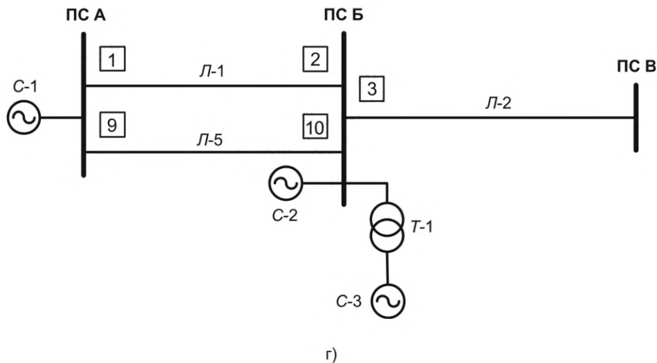
Рисунок 6.1 — Примеры типовых схем участков сети параллельных ЛЭП с двусторонним питанием
