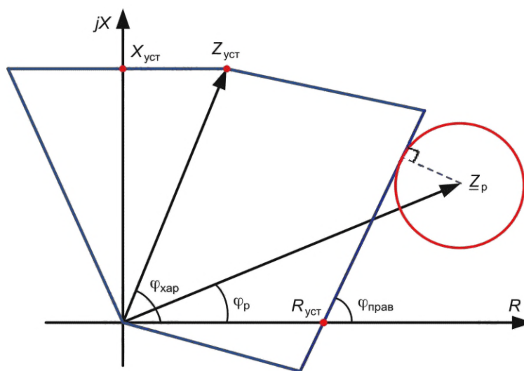
Рисунок 4.7 — Отстройка уставкой активного сопротивления и углом наклона правой боковой стороны характеристики
