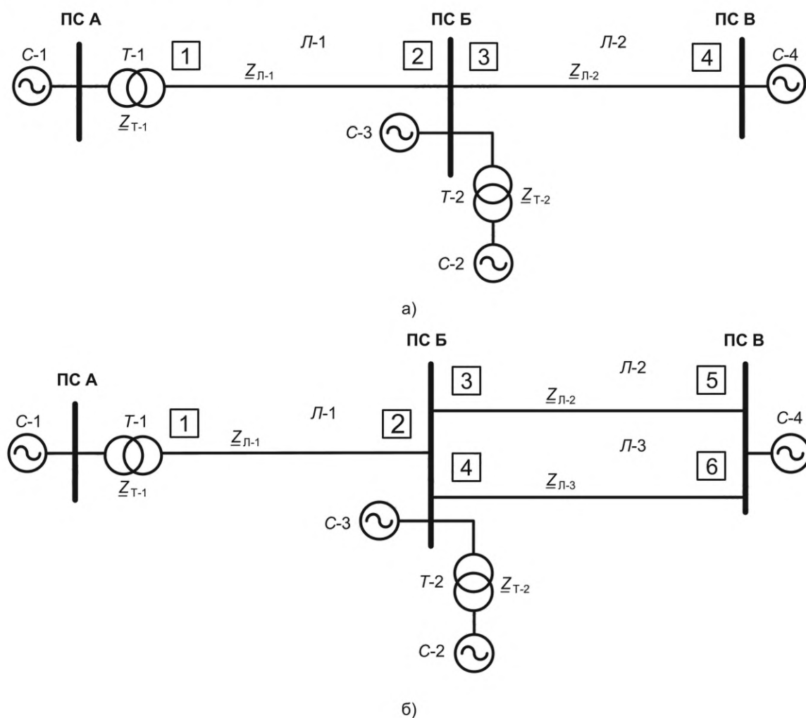
Рисунок 8.1 — Примеры типовых схем участков сети с ЛЭП, работающей по схеме блока Т (АТ) — линия
