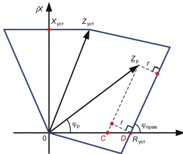
Рисунок 4.16 — Обеспечение чувствительности по активному сопротивлению срабатывания R_{уст}
