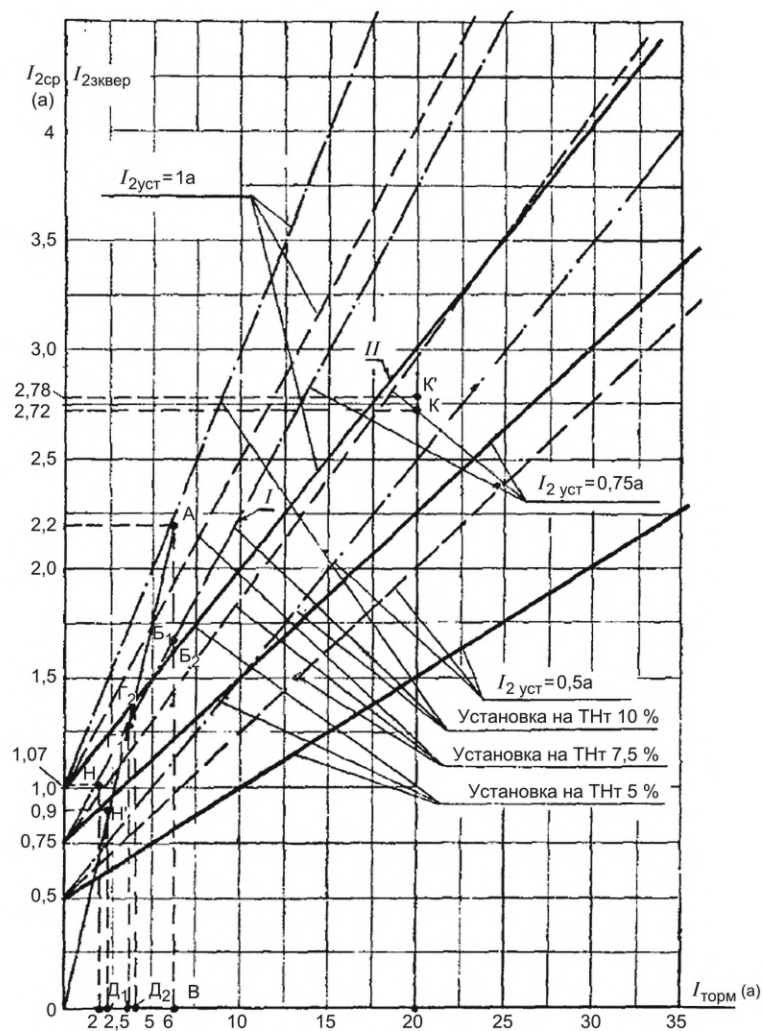
Рисунок 10.7 — Расчет устройства БК типа КРБ-122
