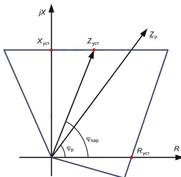
Рисунок 4.5 — Отстройка ДО с полигональной характеристикой
