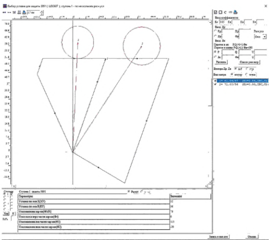
Рисунок 7.10 — Графический выбор параметров настройки ступени ДЗ по условию отстройки от КЗ на стороне НН Т
