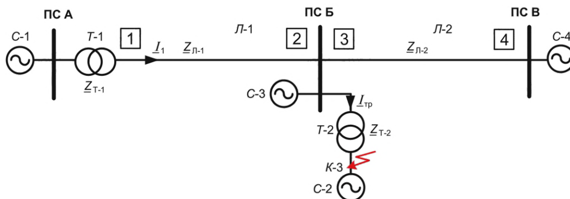
Рисунок 8.5 — Определение коэффициента токораспределения при КЗ в точке К-3
