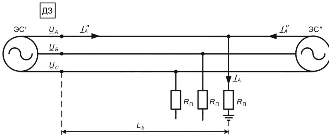
Рисунок Б.9 — Однофазное КЗ на землю через переходное сопротивление на ЛЭП с двухсторонним питанием
