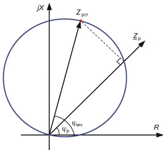
Рисунок 4.2 — Отстройка ДЗ с направленной круговой характеристикой, проходящей через начало координат
