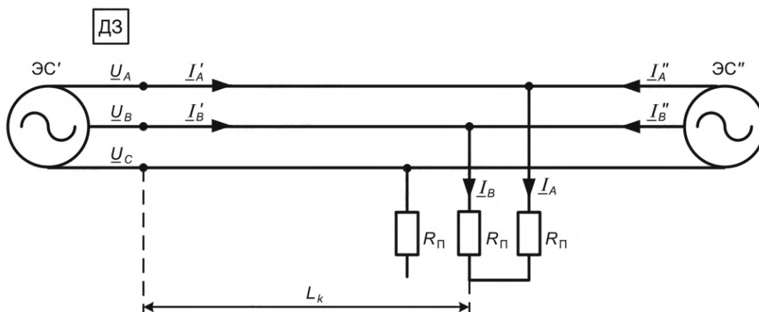
Рисунок Б.7 — Двухфазное КЗ через переходное сопротивление на ЛЭП с двухсторонним питанием
