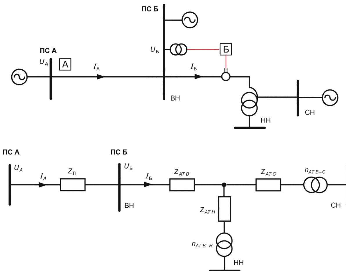
Рисунок Е.1 — Вариант схемы подключения ДЗ АТ к ТТ и ТН стороны ВН
