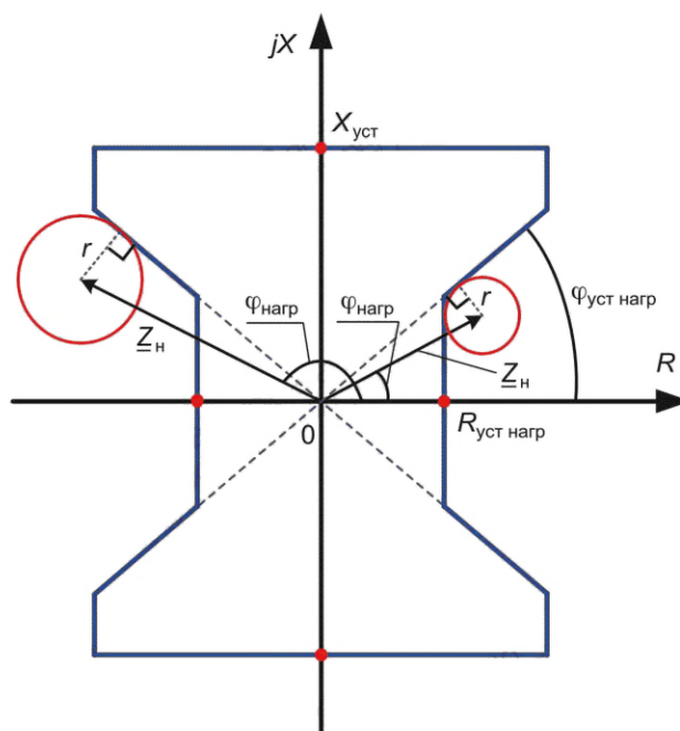
Рисунок 4.21 — Отстройка от нагрузочных режимов
