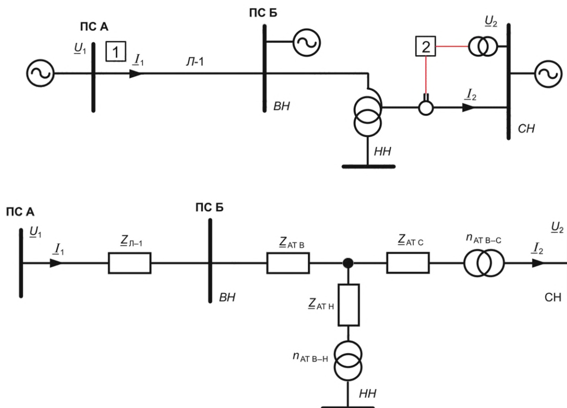
Рисунок 5.6 — Схема подключения ДЗ АТ к ТТ и ТН, установленным на стороне СН
