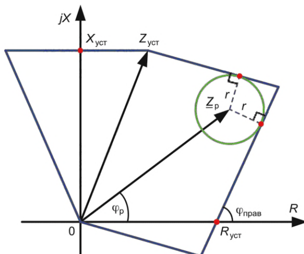
Рисунок 4.17 — Графический метод проверки чувствительности ДО с полигональной характеристикой
