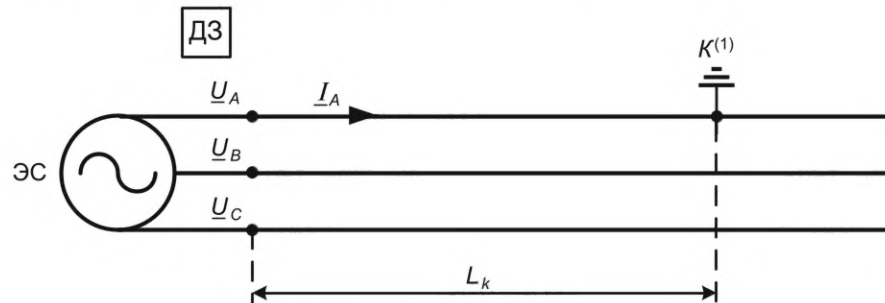
Рисунок Б.2 — Однофазное КЗ на землю
