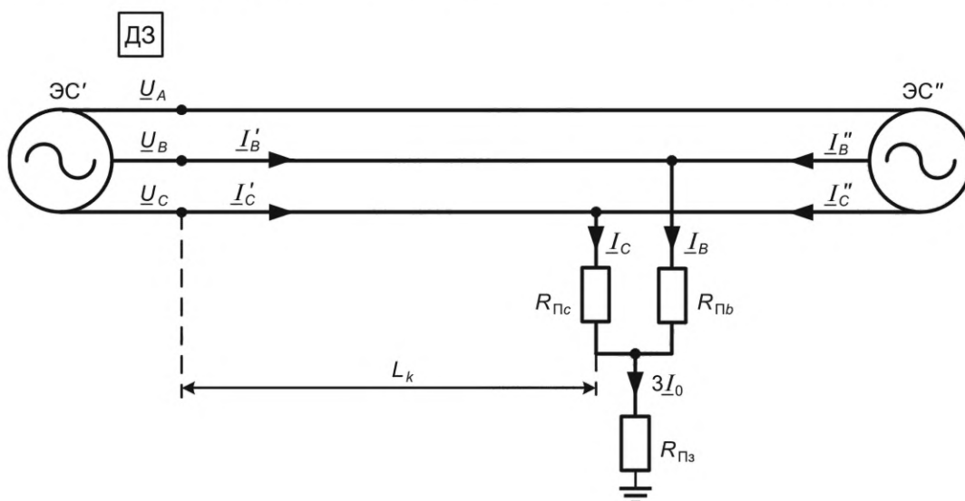
Рисунок Б.10 — Двухфазное КЗ на землю через переходное сопротивление на ЛЭП с двухсторонним питанием
