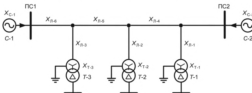
Рисунок Ж.1 — Схема сети для определения X_{T \text{ экв}}^{(k)}
