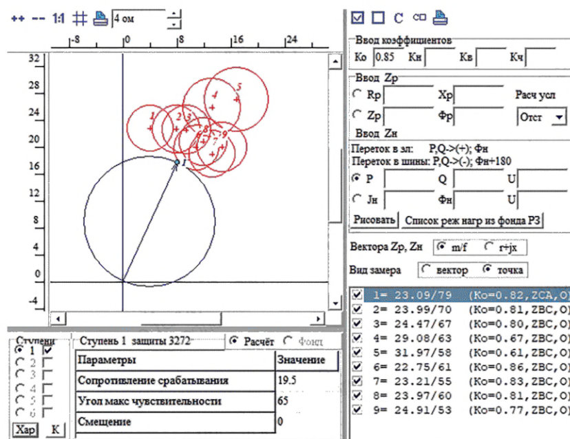
Рисунок 4.3 — Графический выбор параметров настройки ДО с круговой характеристикой
