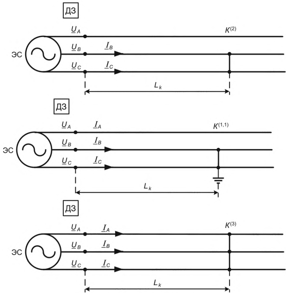
Рисунок Б.1 — Виды междуфазных повреждений на линии
