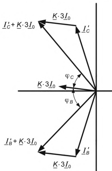
Рисунок Б.11 — Векторная диаграмма токов при двухфазном КЗ на землю
