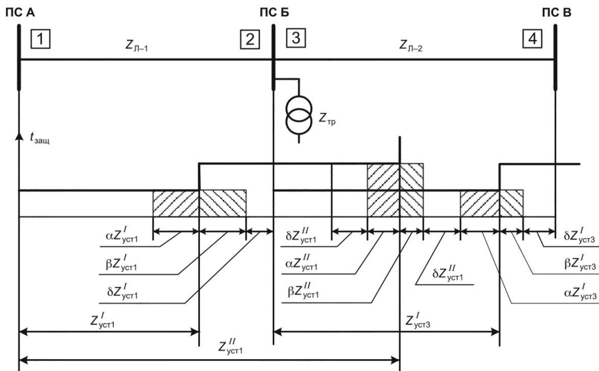
Рисунок 4.1 — Погрешности работы ДЗ
