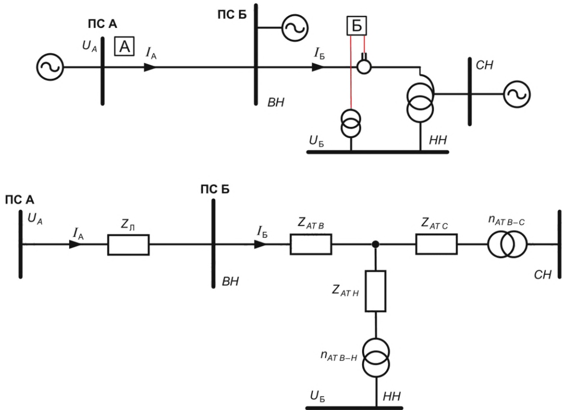
Рисунок Е.5 — Вариант схемы подключения ДЗ АТ к ТТ стороны ВН и ТН стороны НН
