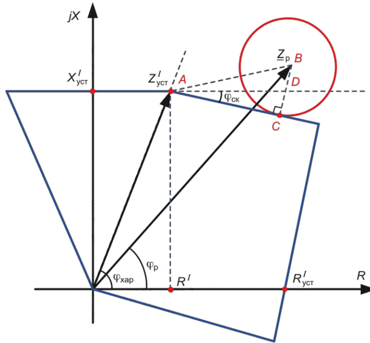
Рисунок В.1 — Графические построения для определения угла скоса
