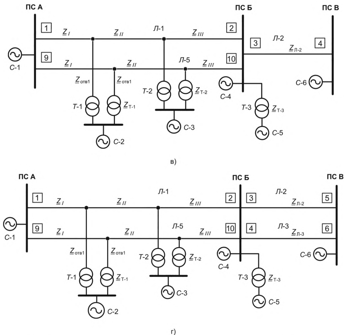
Рисунок 7.1 — Примеры типовых схем участков сети с одиночными и параллельными ЛЭП с двусторонним питанием при наличии ответвлений (отпаек)
