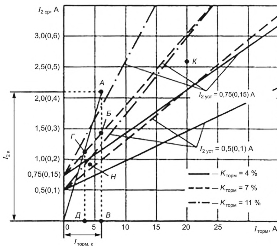
Рисунок 10.4 — Характеристики срабатывания устройства БК типа КРБ-122
