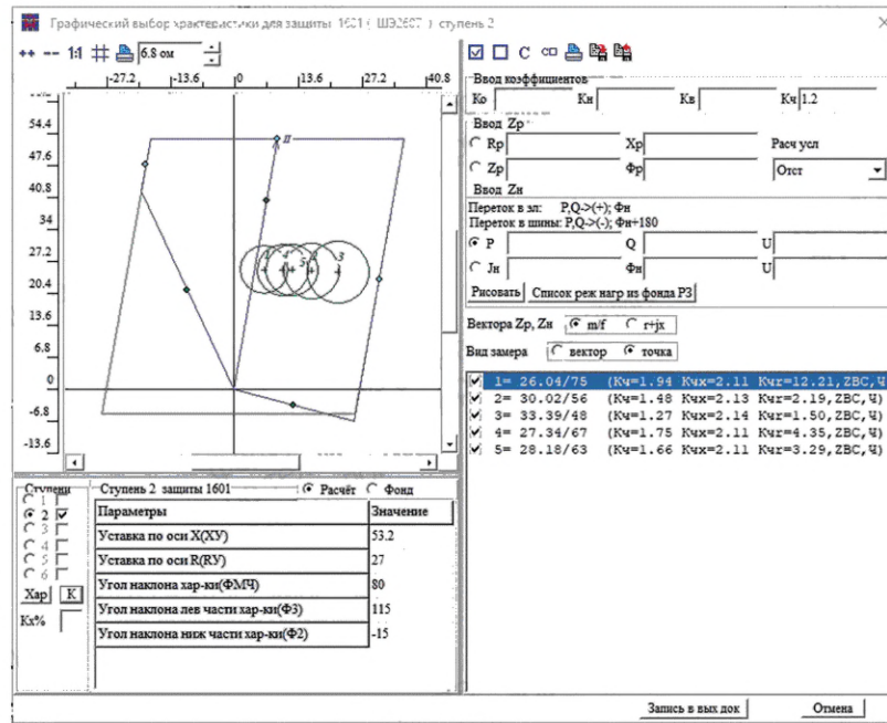
Рисунок 5.11 — Выбор полигональной характеристики срабатывания второй ступени по чувствительности к междуфазным КЗ в конце ЛЭП
