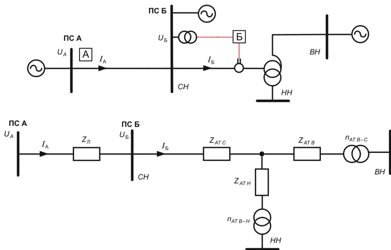
Рисунок Е.2 — Вариант схемы подключения ДЗ АТ к ТТ и ТН стороны СН
