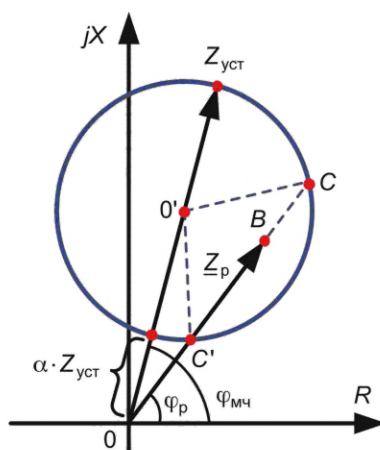
Рисунок 4.11 — Определение чувствительности ДО с круговой характеристикой со смещением по отношению к началу координат
