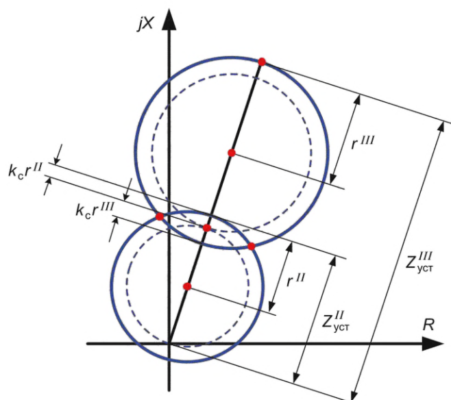
Рисунок 4.14 — Проверка зацепления ДО с круговыми характеристиками при наличии смещения
