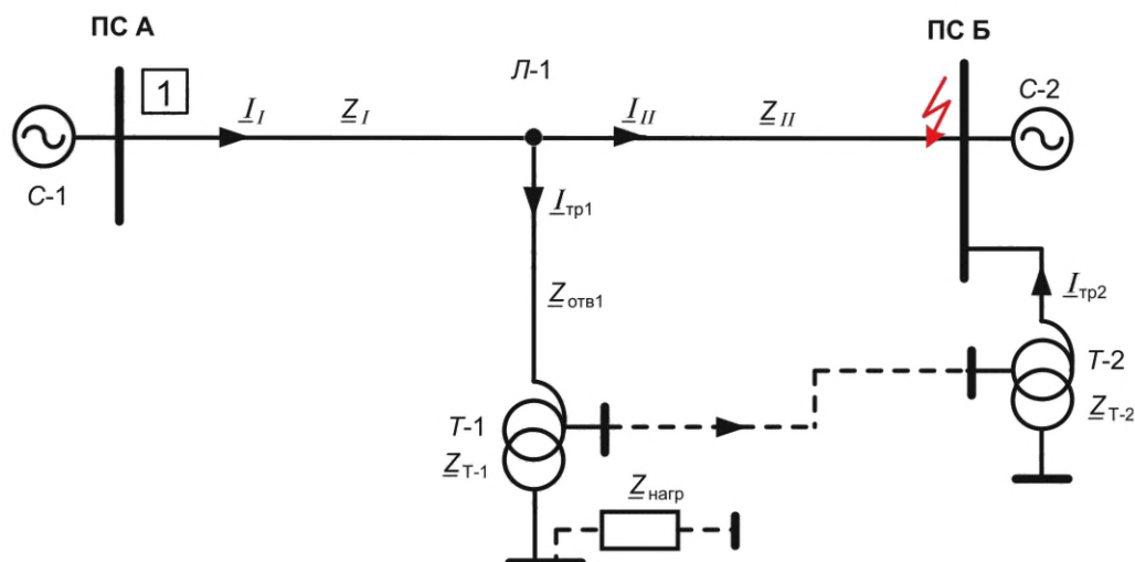
Рисунок 7.2 — Эффект «отрицательной подпитки» при КЗ на ЛЭП с ответвлением
