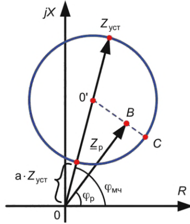
Рисунок 4.12 — Определение чувствительности ДО с круговой характеристикой со смещением по отношению к центру круговой характеристики
