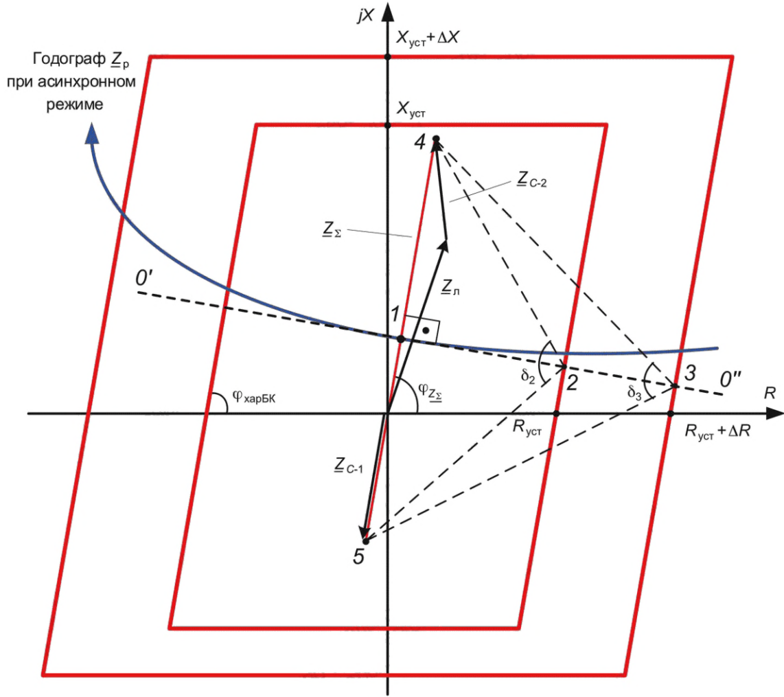
Рисунок 10.9 — Пересечение характеристик БК годографом асинхронного режима
