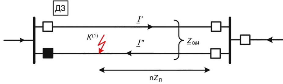
Рисунок Б.4 — Каскадное отключение однофазного КЗ на землю на параллельной линии
