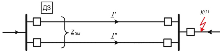
Рисунок Б.3 — Внешнее однофазное КЗ на землю, параллельные линии в работе
