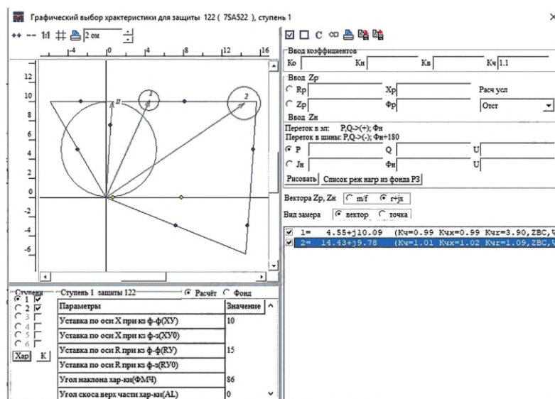
Рисунок 13.1 — Сравнение чувствительности круговой и полигональной характеристик ДЗ при КЗ через переходное сопротивление
