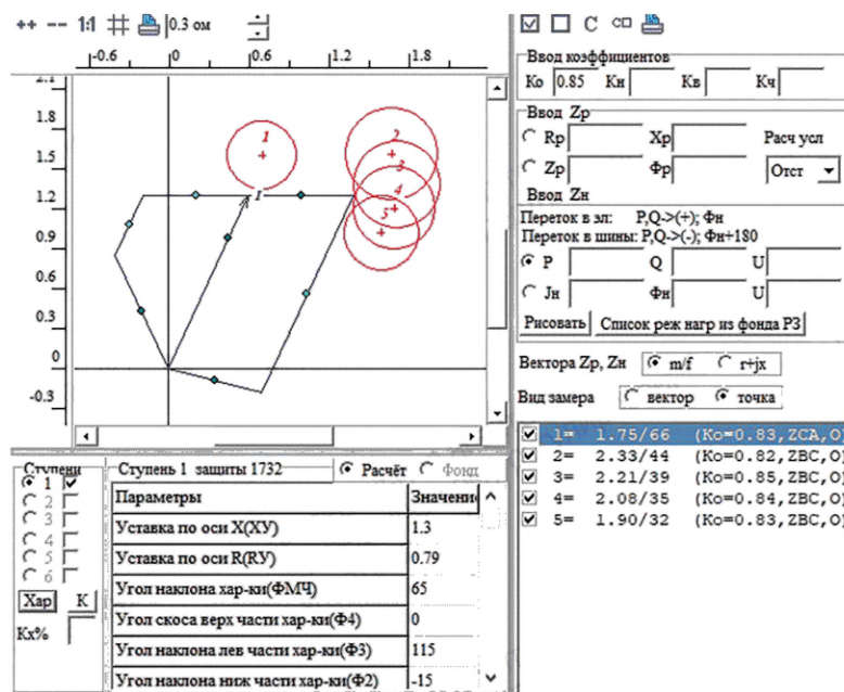
Рисунок 4.8 — Графический выбор параметров настройки ДО с полигональной характеристикой
