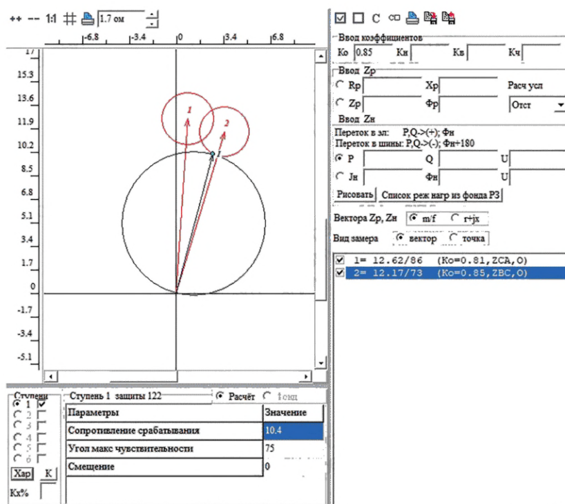
Рисунок 5.2 — Графический выбор параметров настройки ступени ДЗ с круговой характеристикой
