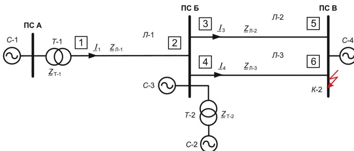
Рисунок 8.4 — Определение коэффициента токораспределения при КЗ в точке К-2
