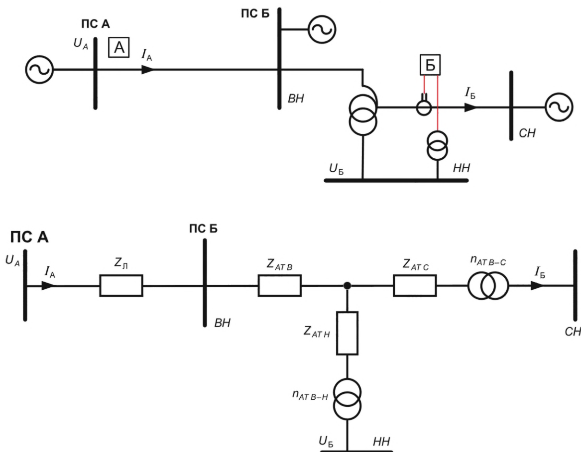
Рисунок Е.6 — Вариант схемы подключения ДЗ АТ к ТТ стороны СН и ТН стороны НН
