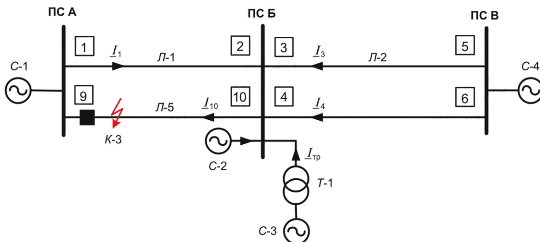
Рисунок 6.2 — Определение коэффициента токораспределения при КЗ в точке К-3
