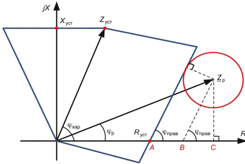
Рисунок В.2 — Графические построения для определения положения правой боковой стороны характеристики срабатывания
