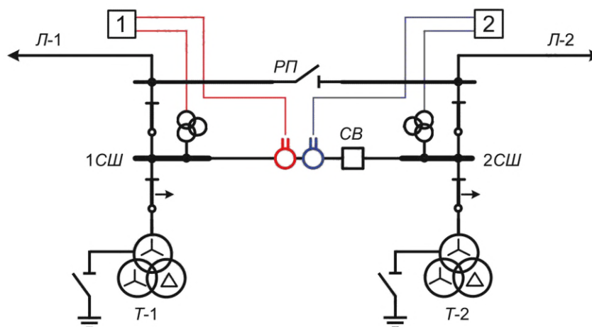
Рисунок 12.1 — Схема подключения ДЗ Л-1 и Л-2 к ТН и ТТ СВ
