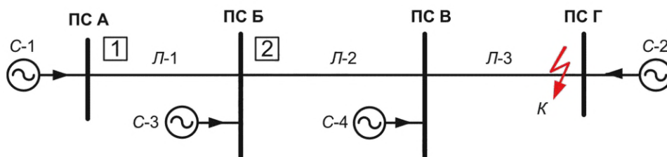
Рисунок 10.2 — Пример схемы сети ЛЭП с двусторонним питанием для расчета уставок устройства БК
