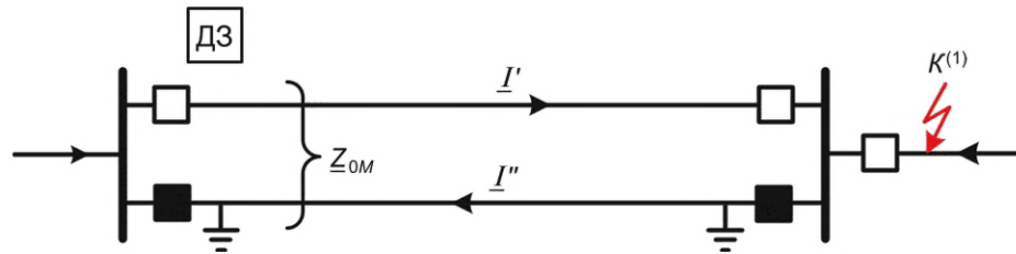
Рисунок Б.5 — Внешнее однофазное КЗ на землю A_0 для случая отключенной и заземленной параллельной линии
