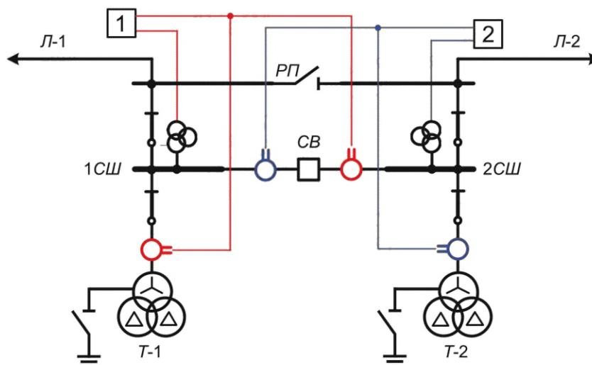
Рисунок 12.2 — Схема подключения ДЗ Л-1 и Л-2 на сумму ТТ СВ и ТТ силового трансформатора
