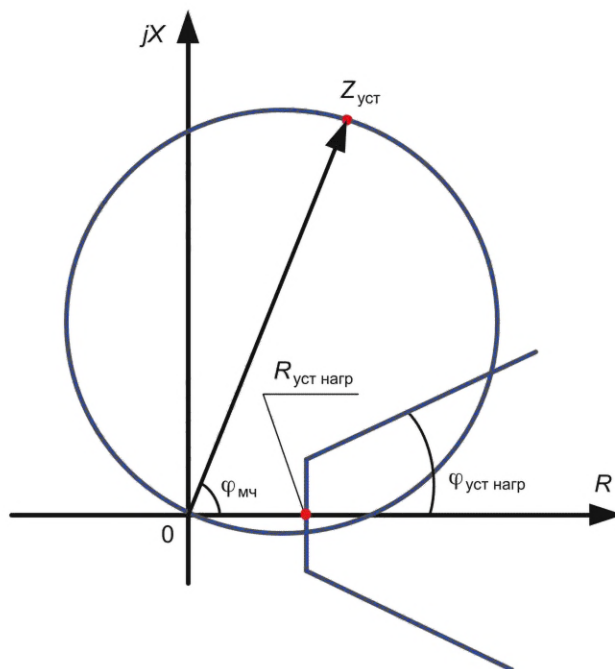
Рисунок А.3 — Пример направленной круговой характеристики с вырезом в области нагрузки
