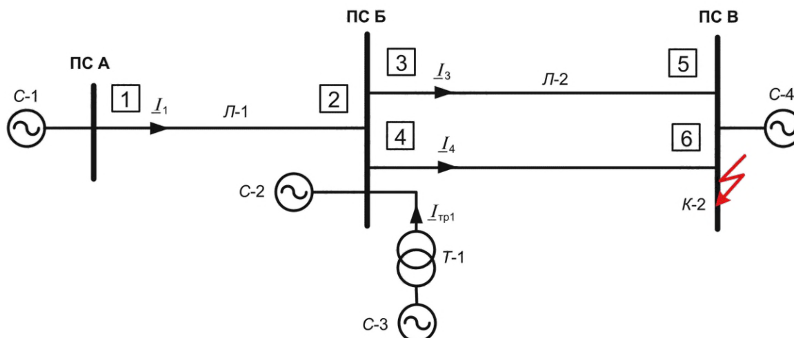
Рисунок 5.5 — Определение коэффициента токораспределения при КЗ в точке К-2
