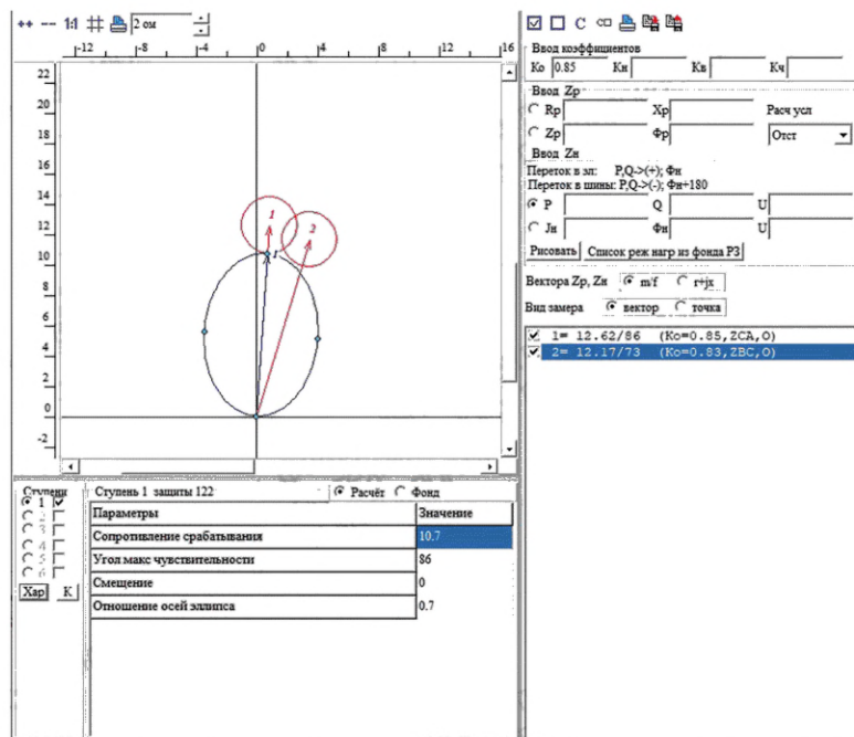
Рисунок 4.4 — Графический выбор параметров настройки ДО с характеристикой в виде эллипса
