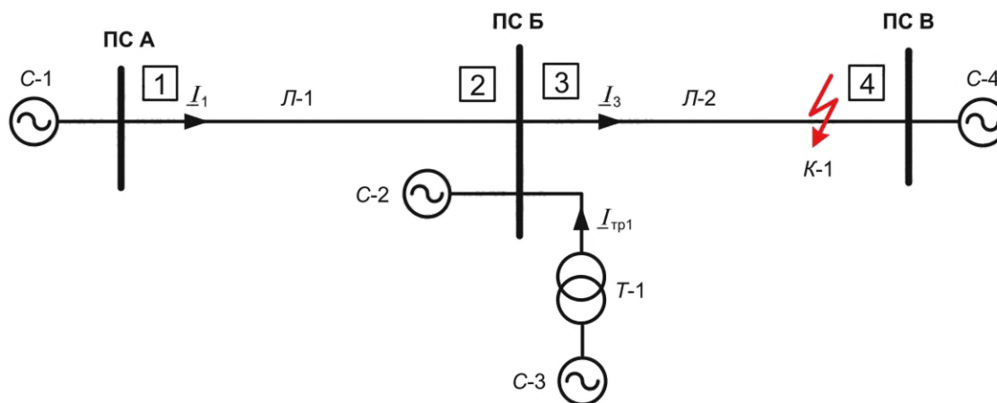
Рисунок 5.4 — Определение коэффициента токораспределения при КЗ в точке К-1
