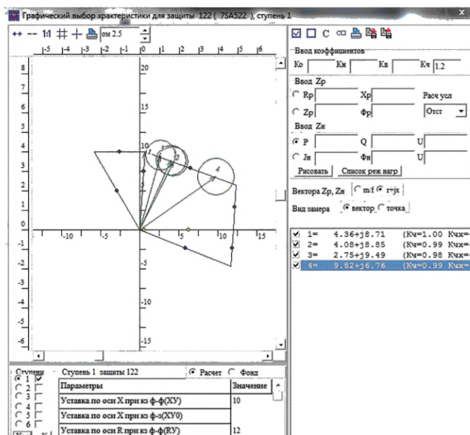
Рисунок 4.20 — Проверка обеспечения чувствительности при КЗ в конце зоны охвата по сопротивлению Z_{вст} или X_{вст}
