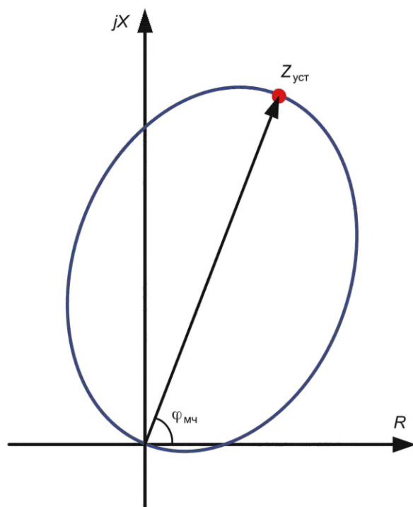
Рисунок А.4 — Пример направленной характеристики в виде эллипса
