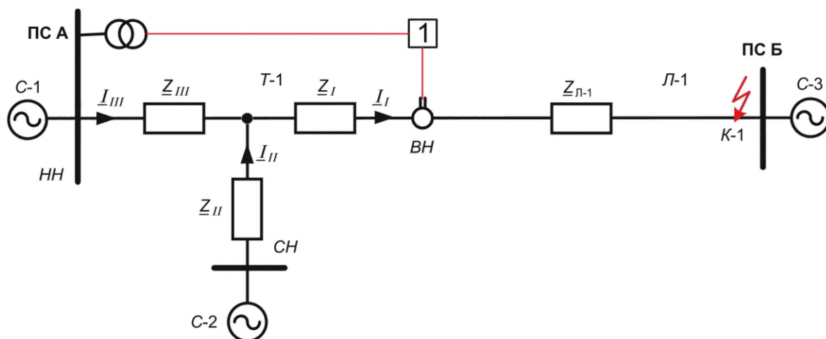
Рисунок 8.2 — Вариант схемы подключения ДЗ блока трехобмоточный Т (АТ) — линия к ТТ и ТН
