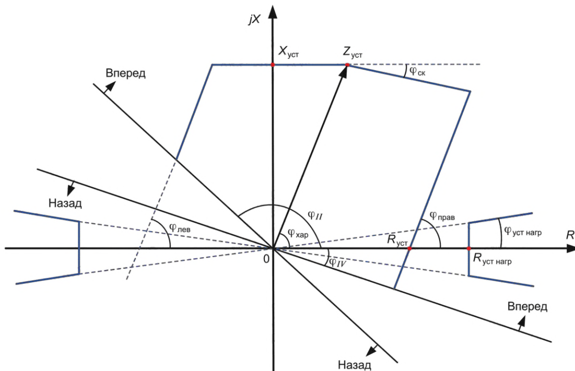
Рисунок А.1 — Пример направленной полигональной характеристики срабатывания
