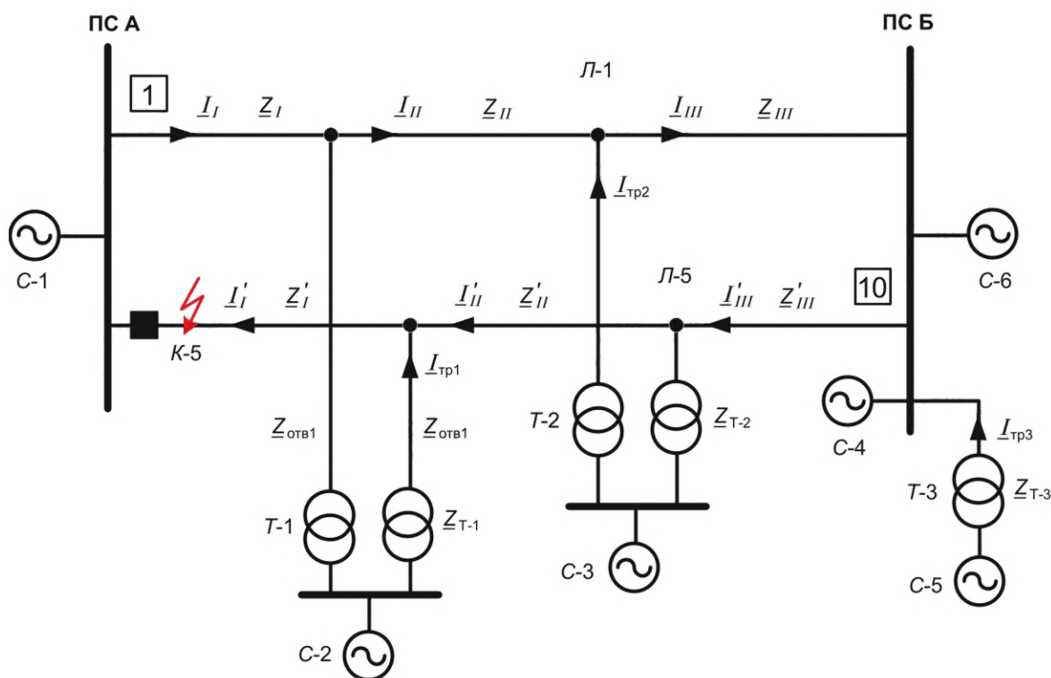
Рисунок 7.7 — Определение коэффициентов токораспределения для КЗ в точке К-5
