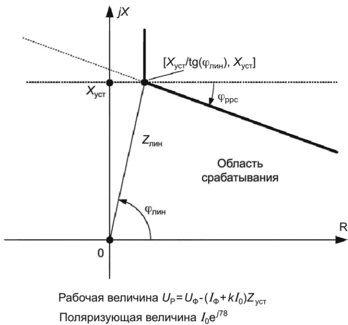
Рисунок Б.13 — Характеристика срабатывания реле реактивного сопротивления
