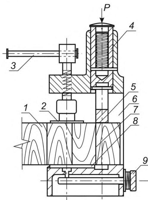
1 — образец; 2 — прижимная опора; 3 — рукоятка; 4 — пуансон; 5 — нож пуансона; 6 — корпус; 7 — клеевое соединение; 8 — передвижная опорная площадка; 9 — винт упора
