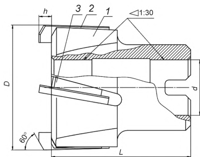
1 — корпус; 2 — нож по ГОСТ Р 72137; 3 — клин по ГОСТ 16859
