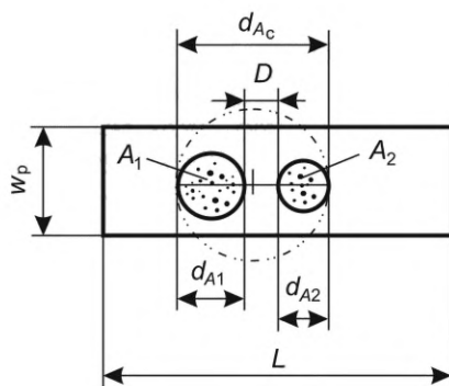
Рисунок С.1 — Скопление пор, D \leq d_{A2}
