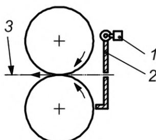
1 — концевой выключатель; 2 — панель отключения; 3 — обрабатываемый материал
