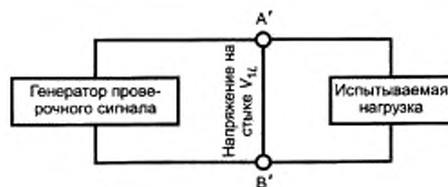
Рисунок 6 — Испытательная схема для измерения нагрузок по V.11
