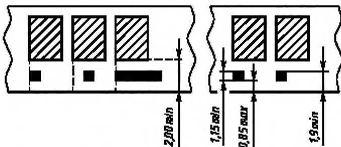
Рисунок 1 — Размещение счетной метки в зоне кодирования
