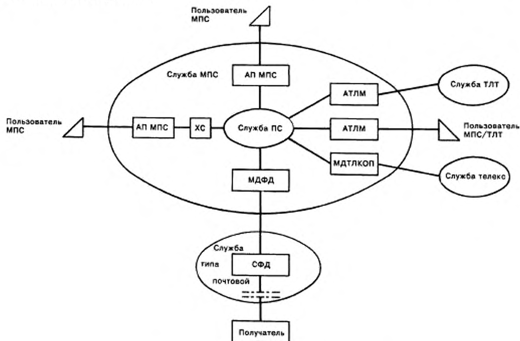
Рисунок 7 — Функциональная модель службы МПС
