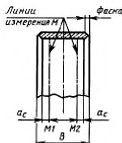
Рисунок 3 — Положение линий измерения
