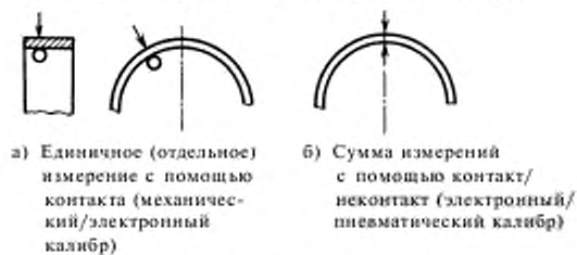
Рисунок 2 — Принцип измерения толщины стенки
