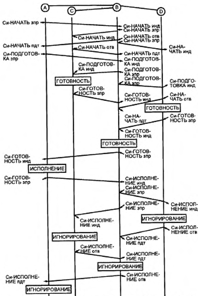
Рисунок С.4 — Последовательность примитивов — Исполнение атомарного действия Si-ПОДГОТОВКА
