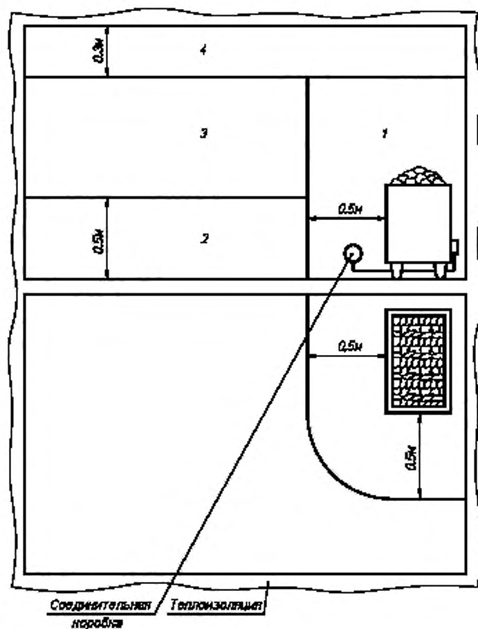
Рисунок 703А — Зоны температуры окружающей среды
