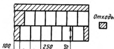
Рисунок 2 — Пример распределения прямоугольных проб
