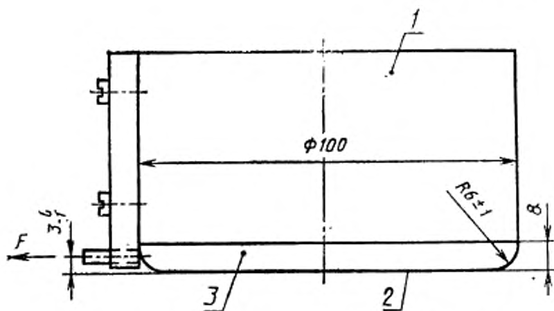
Рисунок 2 — Фрикционный цилиндр
