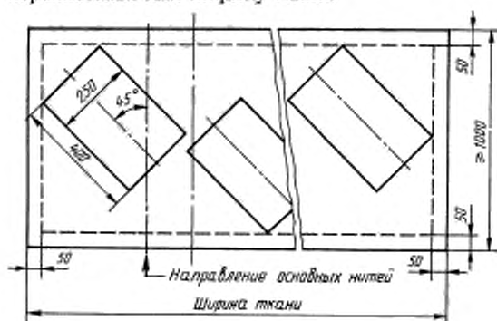
Рисунок 1 — Пример диагонально расположенных проб ткани из стекловолокна
