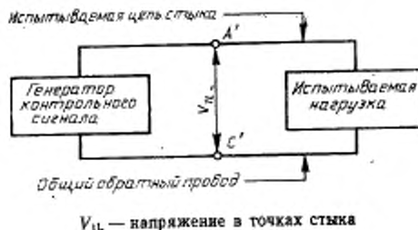
Рисунок 4 — Испытательная схема нагрузки V.10
