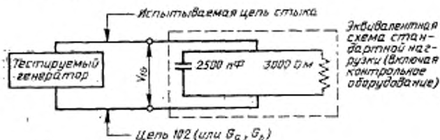
Рисунок 1 — Испытательная схема генератора V.28
