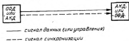
Рисунок 7 — Сигнал управления, синхронизации
