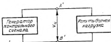
Рисунок 6 — Испытательная схема нагрузки V.11
