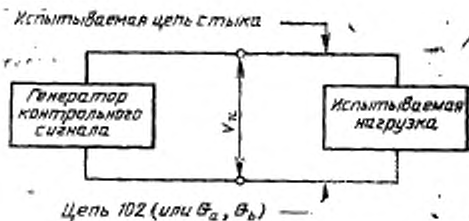
Рисунок 2 — Испытательная схема нагрузки V.28
