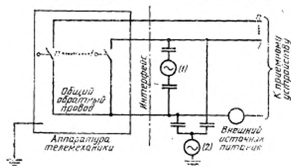
а) схема для пассивных двоичных выходных сигналов
