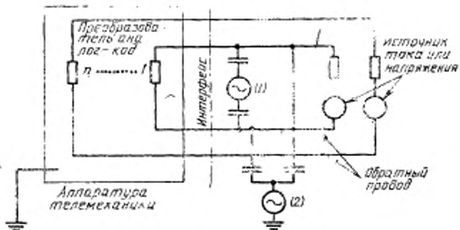
Схема для аналоговых входных сигналов
