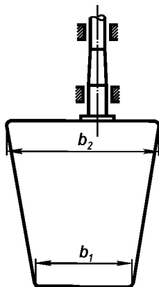
Рис. 1.2.1.5l. К определению ширины пера руля»;
