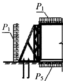
Рисунок 7.1а — Схема приложения динамической нагрузки на конструкции БВ У
