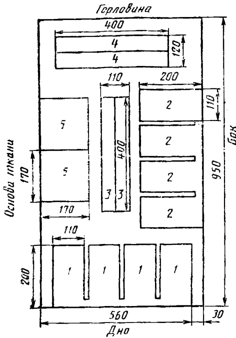
Схема раскроя мешка для испытаний
