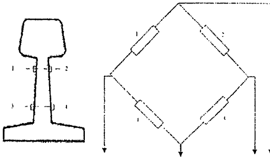
Рис. А.2. Схема измерения боковых сил тензорезисторами на шейке рельса
