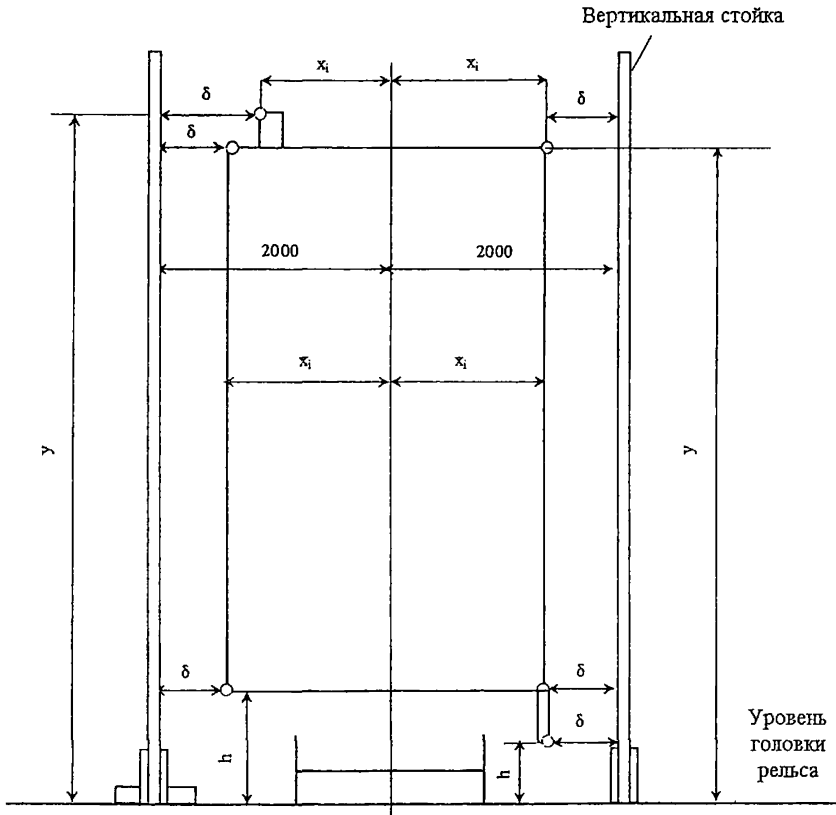
Рис. А.1. Схема измерения габаритных размеров
