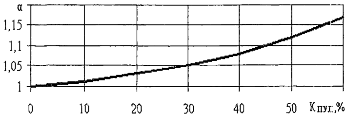
Рис. А.6. График для определения эквивалентного коэффициента, учитывающего пульсацию тока
