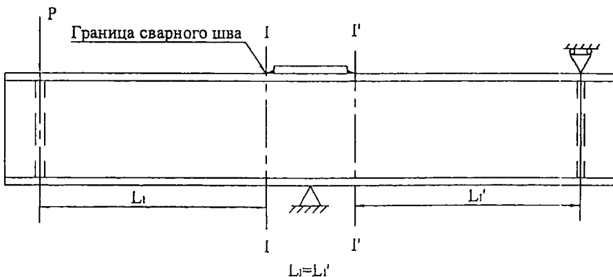
Рис. А.4. Схема нагружения типового сварного образца (точка приложения пульсирующей нагрузки Р может быть изменена в зависимости от конструкции стенда)
