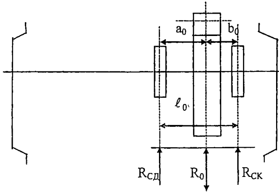
Рис. А.12. Схема для определения нагрузок на опорные подшипники тягового редуктора
