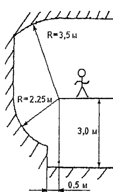
Рис. А.17. Минимально допустимое расстояние до частей электропоезда,
