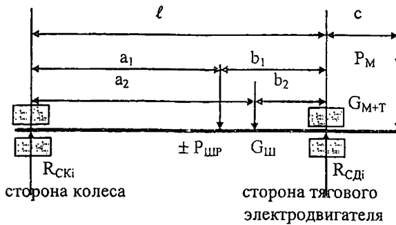
Рис. А.8. Схема для расчета нагрузок на подшипники ведущей шестерни
