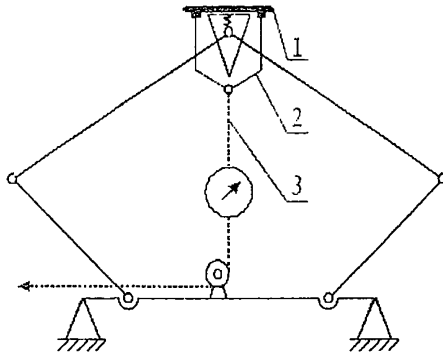
Рис. А.16. Схема для определения аэродинамической характеристики токоприемников: 1 – отрезок контактного провода; 2 – рамка; 3 – шнур.
