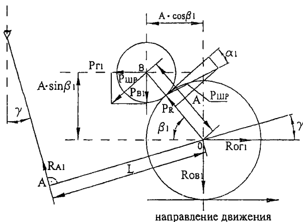
Рис. А.10. Схема нагружения опор редуктора в режиме тяги при движении колесной пары вперед
