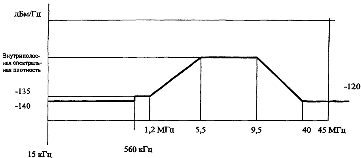
Рис.6.7а. Спектральная плотность мощности выходного сигнала
