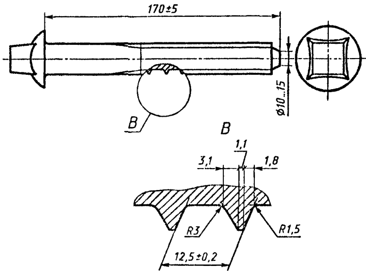
Исполнение 3 (применяется с пластмассовым дюбелем)
